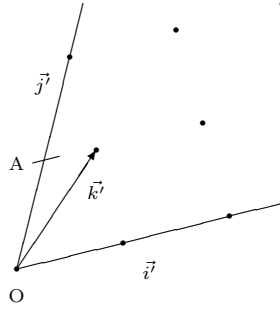
FIG. A.4 – Projection de \vec{k}' sur \vec{i}'_2
