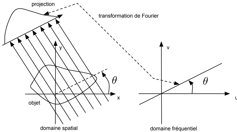
FIG. 3.1 – Représentation du théorème de la tranche centrale.
