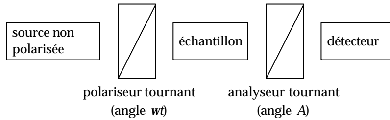
Figure 3 : schéma de principe d'un ellipsomètre à polariseur tournant.
