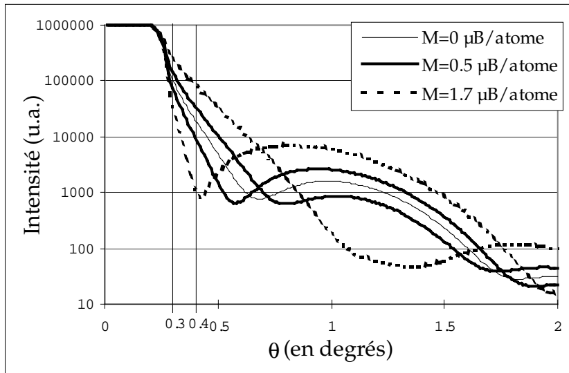
Figure 10 : réflectivité d'une tricouche Au(5nm)/Co(5nm)/Au(5nm) déposée sur verre. En trait fin, cas d'une aimantation nulle. Les signaux " up-up " et " down-down " se superposent. Lorsque l'aimantation augmente, une séparation des signaux (up-up) et (down-down) apparaît (trait gras, M = 0.5 \mu\text{B}/\text{atome} ); trait pointillé, M = M_{\text{sat}} = 1.7 \mu\text{B}/\text{atome} ).
