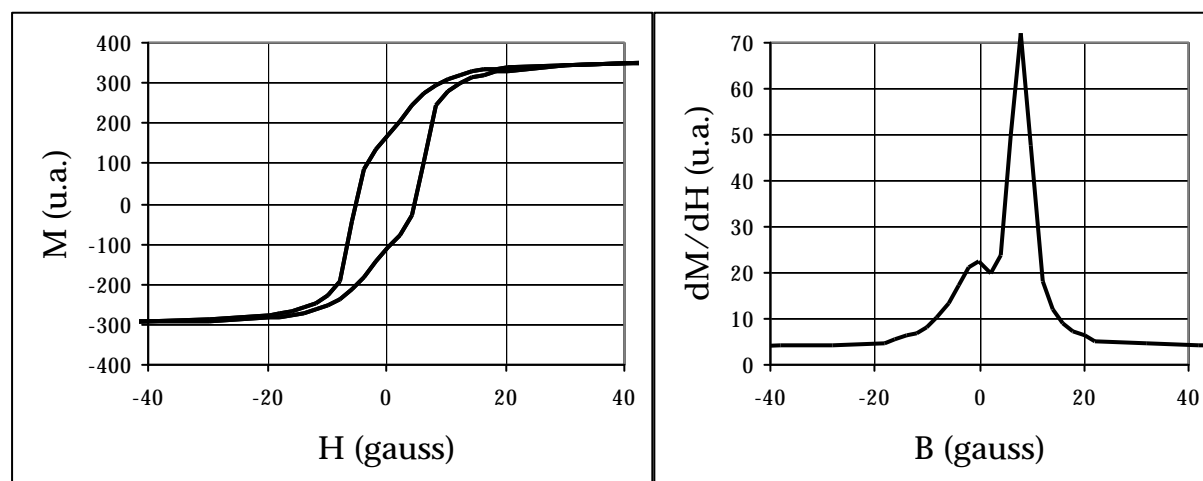
Figure 27 : à gauche, cycle d'hystérésis mesuré sur une tricouche Ni/Cu/NiFe (mesure par SQUID). A droite, la dérivée de l'aimantation par rapport au champ montre deux changements de pente suggérant que les deux couches sont magnétiquement découplées.
