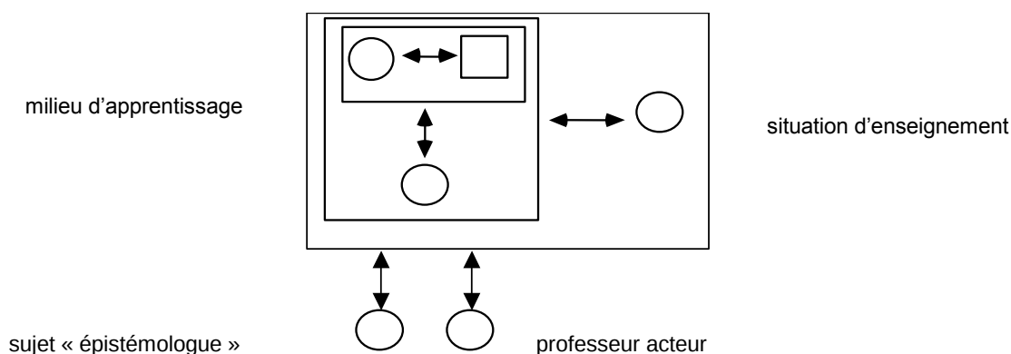
Figure 5 - La situation d'enseignement (Brousseau 1986)
