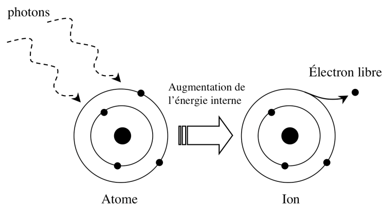
FIG. 7.4 - Ionisation par bombardement de photons.
