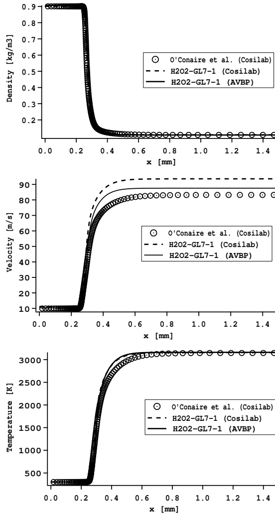
FIG. 6.9 - Profils de la densité, la vitesse et la température à travers la flamme, obtenus avec la cinétique complexe de O'Conaire et al. [42] (Cosilab) et la cinétique réduite H2O2-GL7-1 ( \phi=1.0 , T_0=300\text{K} , P_0=1.87\text{bar} ). ○ O'Conaire et al. ; - - - H2O2-GL7-1 (Cosilab) ; — H2O2-GL7-1 (AVBP).
