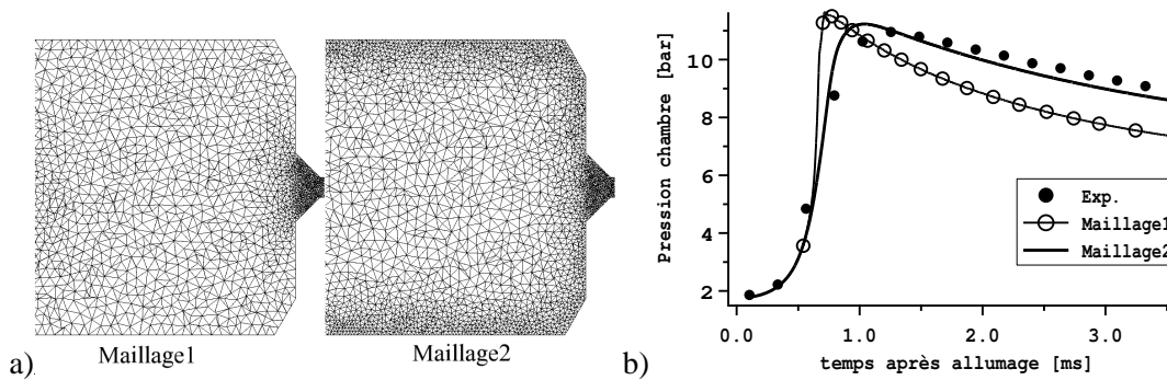
FIG. 8.33 - a) les deux maillages utilisés : Maillage1 : \Delta_{x|paroi} = 2\text{ mm} et Maillage2 : \Delta_{x|paroi} = 0,5\text{ mm} . b) Impact du raffinement à la paroi sur la pression chambre (lignes : simulations, symboles : expérience du DLR [180]).
