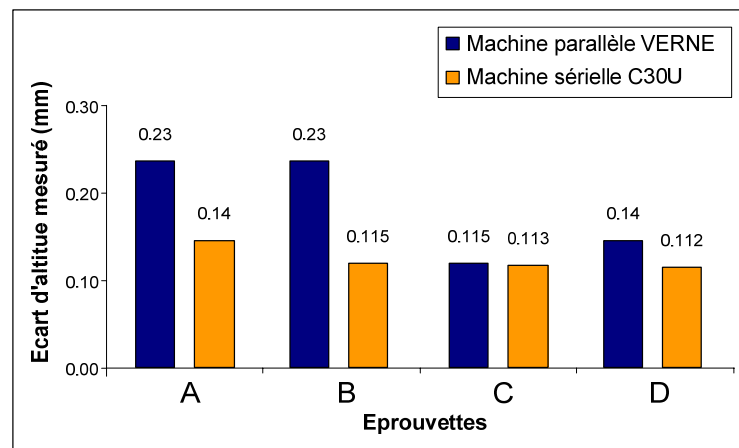
Figure 15 : Ecart mesurés sur chacune des éprouvettes
