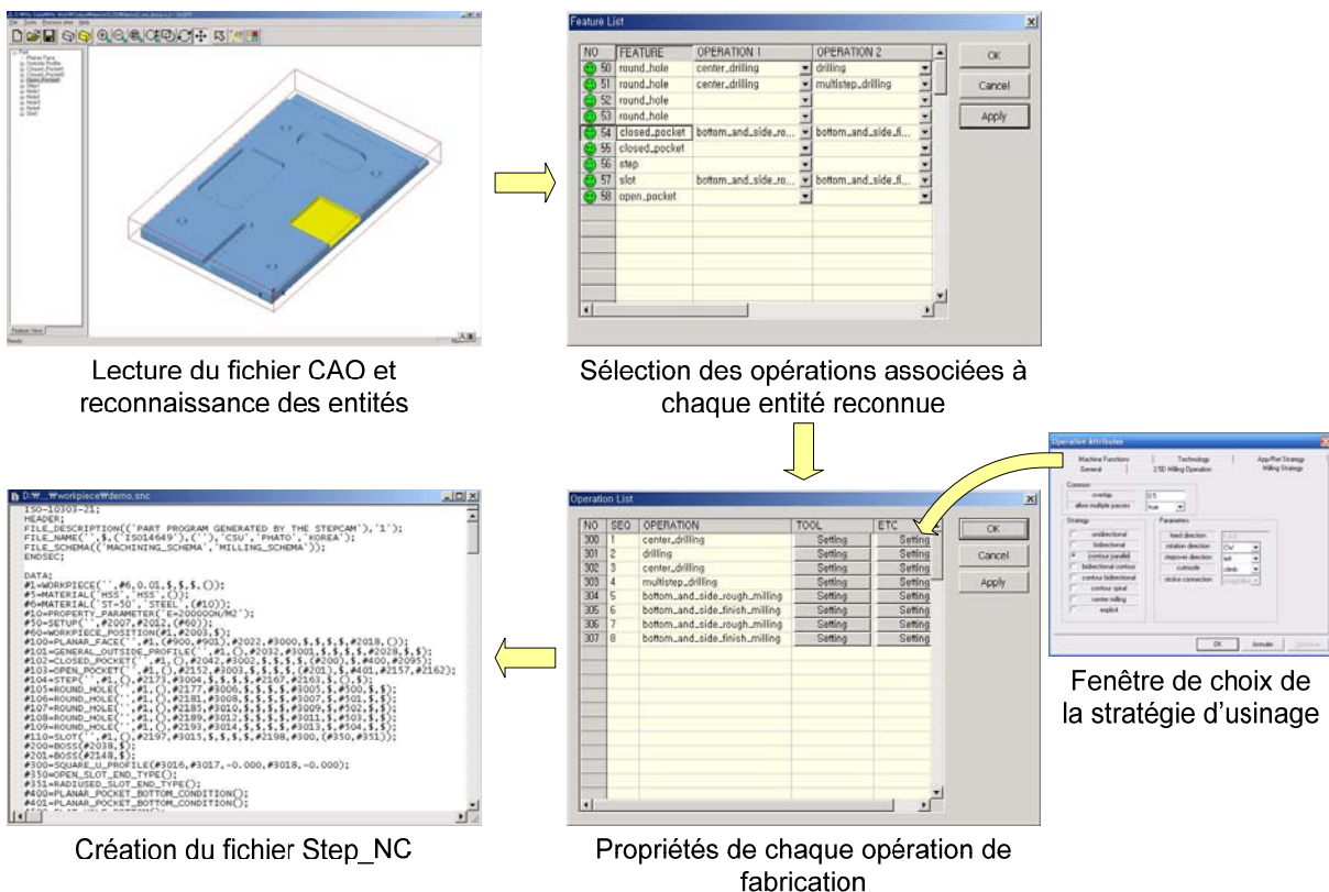
Figure 141 : Principe de fonctionnement du logiciel PosSFP [Suh2003]
