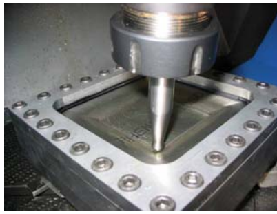
Figure 65 : Mise en œuvre du procédé
