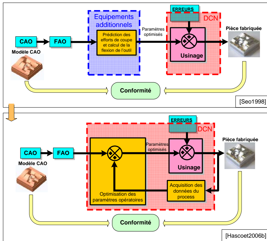
Figure 127 : Approches de programmation avancée de niveau 2
