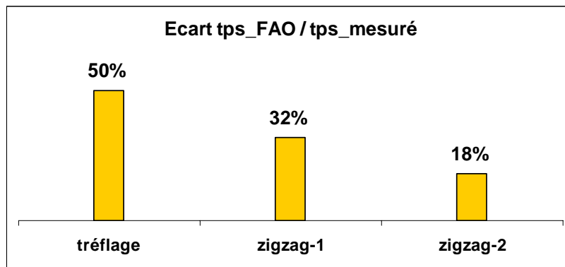
Figure 29 : Ecarts entre temps FAO et temps mesuré
