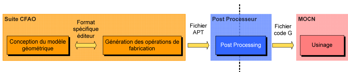
Figure 117 : Architecture de la chaîne numérique actuelle
