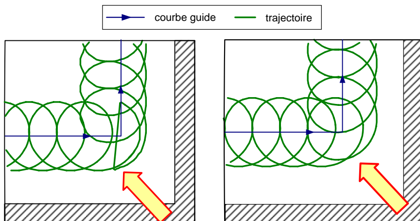
Exemple de trajectoire générée sans gestion des discontinuités de la courbe guide
