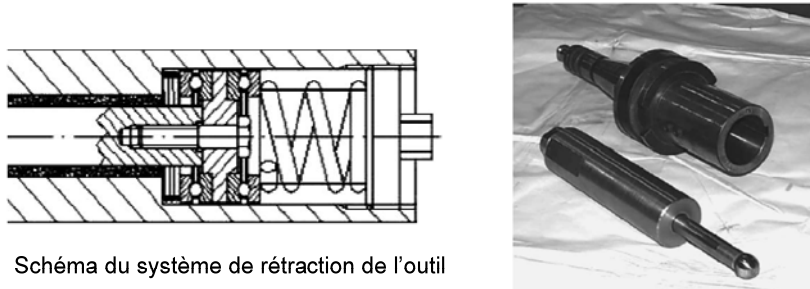
Figure 57 : Outil de formage rétractable [Ceretti2004]
