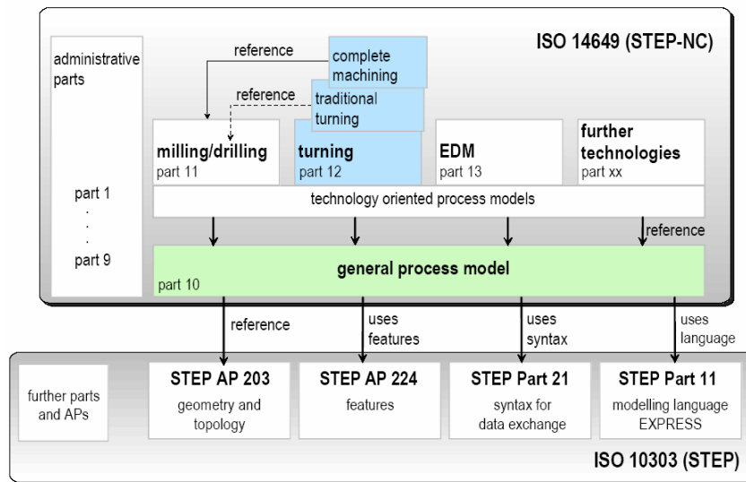
Figure 118 : Organisation de la norme ISO 14649 et relations avec l'ISO 10303
