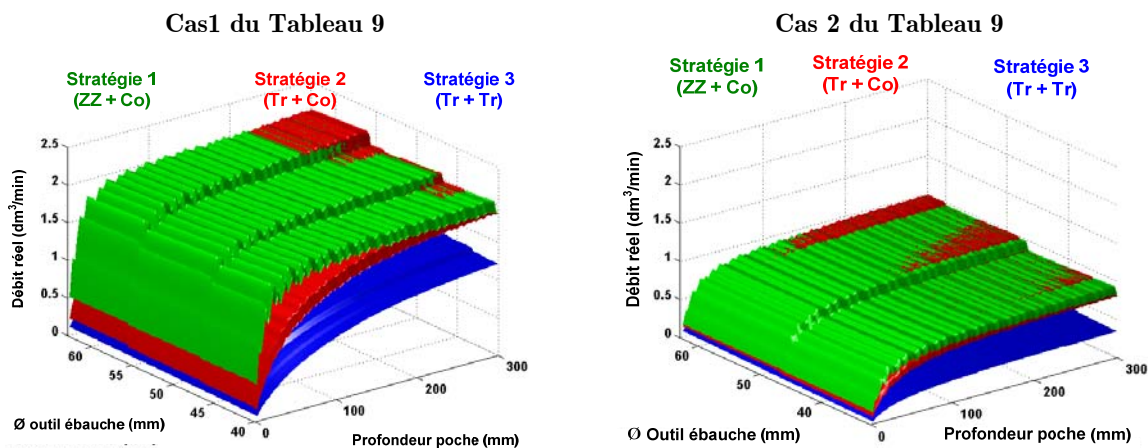
Figure 47 : Influence du diamètre de l'outil d'ébauche
