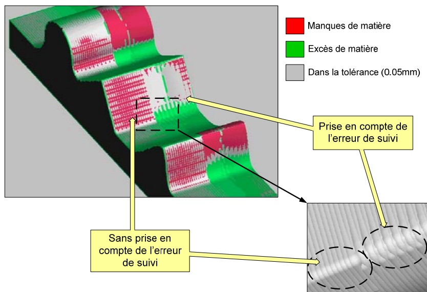
Figure 82 : Influence de l'erreur de poursuite
