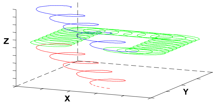
Figure 41 : Prise de passe trochoïdale entre deux couches
