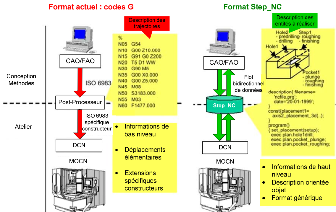
Figure 120 : Comparaison de l'ISO 6983 et de l'ISO 14649 [ESPRIT2000]
