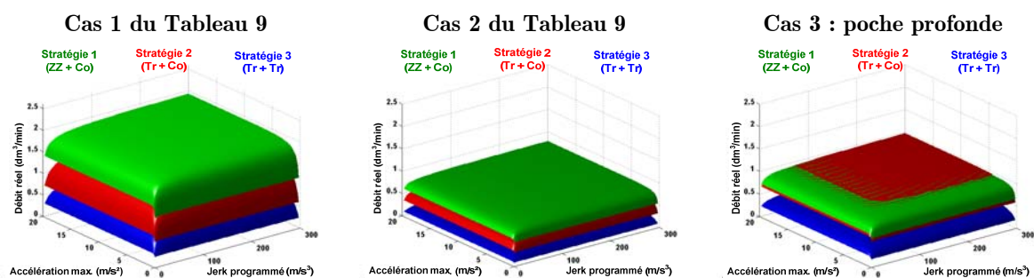
Figure 49 : Performances cinématiques
