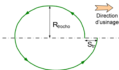
Figure 134 : Exemple de motif trochoïdal
