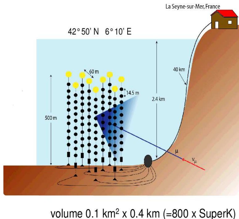
FIG. 2.3 – Représentation du télescope ANTARES : détection de lumière Cherenkov produite par propagation d'un muon dans l'eau
