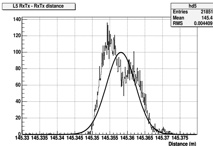
FIG. 3.21 – Distribution de la distance entre l'émetteur Ligne 5 et l'émetteur MILOM entre fin janvier et début avril 2007
