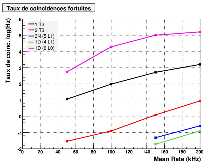
FIG. 5.12 – Taux de coïncidences fortuites en fonction du bruit de fond optique pour les différentes logiques comparées dans cette étude, pour un détecteur à 5 lignes.
