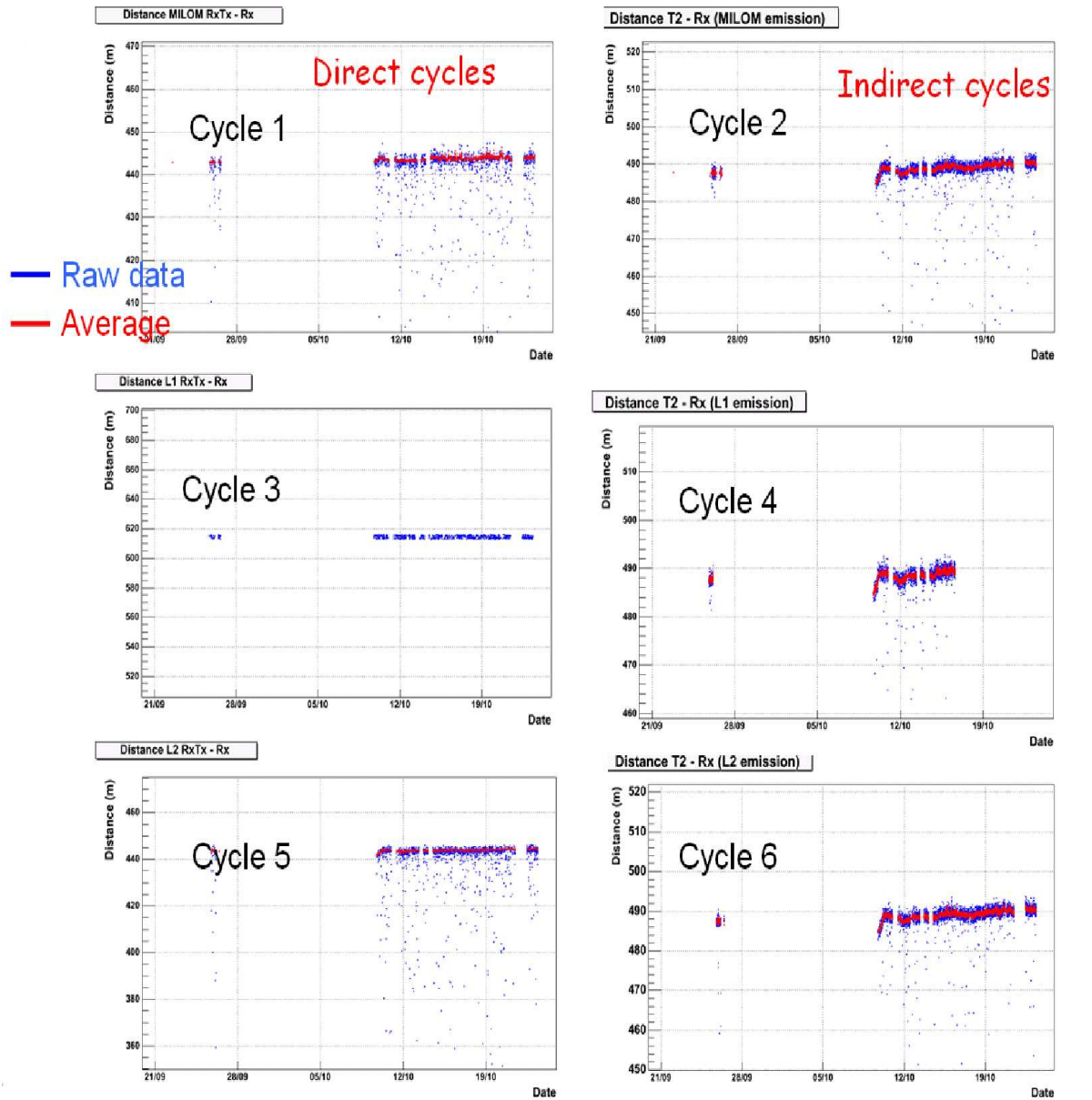
FIG. 3.16 – Comparaison des données brutes (bleu) et des moyennes glissantes correspondantes (rouge) converties en distances pour tous les cycles rapides dans une configuration similaire à celle de la figure précédente
