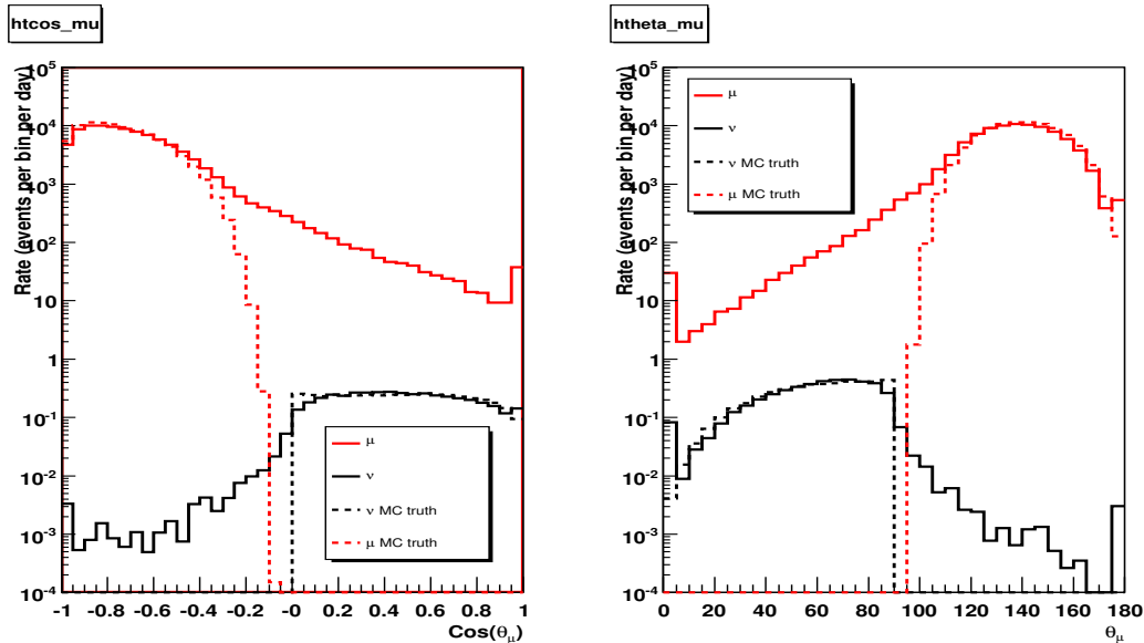
FIG. 5.21 – Cosinus des angles zénithaux (figure de gauche) et angles zénithaux (figure de droite) pour les traces ajustées des muons (en rouge), des neutrinos (en noir) et pour leur angle vrai (vérité MonteCarlo en pointillés) pour les événements reconstruits avec deux lignes minimum
