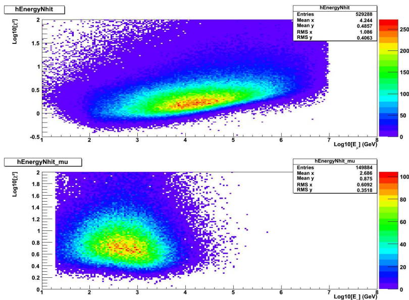
FIG. 5.27 – \chi^2 en fonction de l'énergie du muon pour les muons neutrinoiques en haut et les muons atmosphériques en bas (événements montants reconstruits au moins 6 hits sur 2 lignes)
