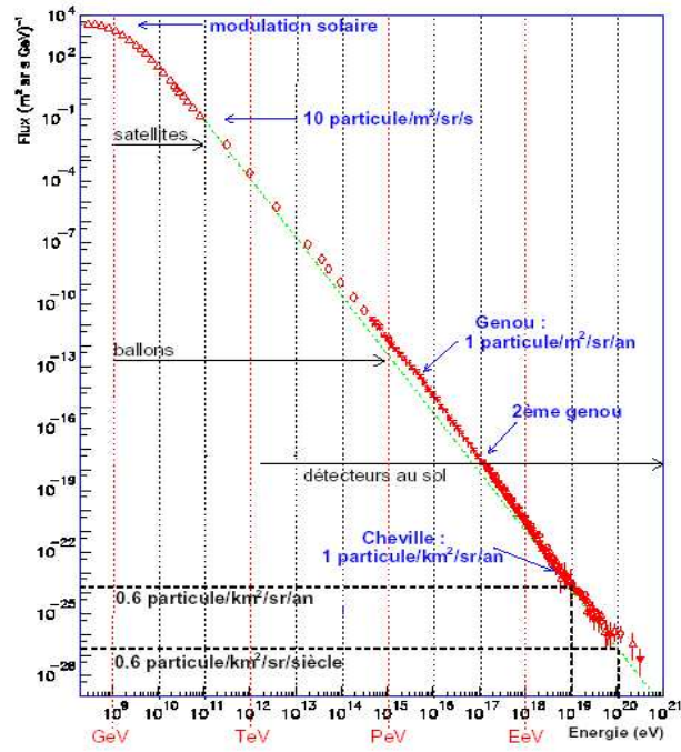
FIG. 1.3 – Spectre des rayons cosmiques
