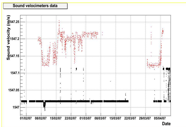
FIG. 3.19 – Vitesses du son mesurées par le célérimètre de la ligne 1 (en noir) et par celui de la MILOM après application de l'offset négatif de 0.245 m \cdot s^{-1} (en rouge) pendant une période de deux mois en 2007
