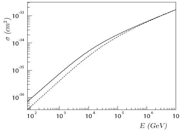
FIG. 1.10 – Section efficace de l'interaction du neutrino muonique en trait plein (antineutrino en trait pointillé) avec un nucléon [14]
