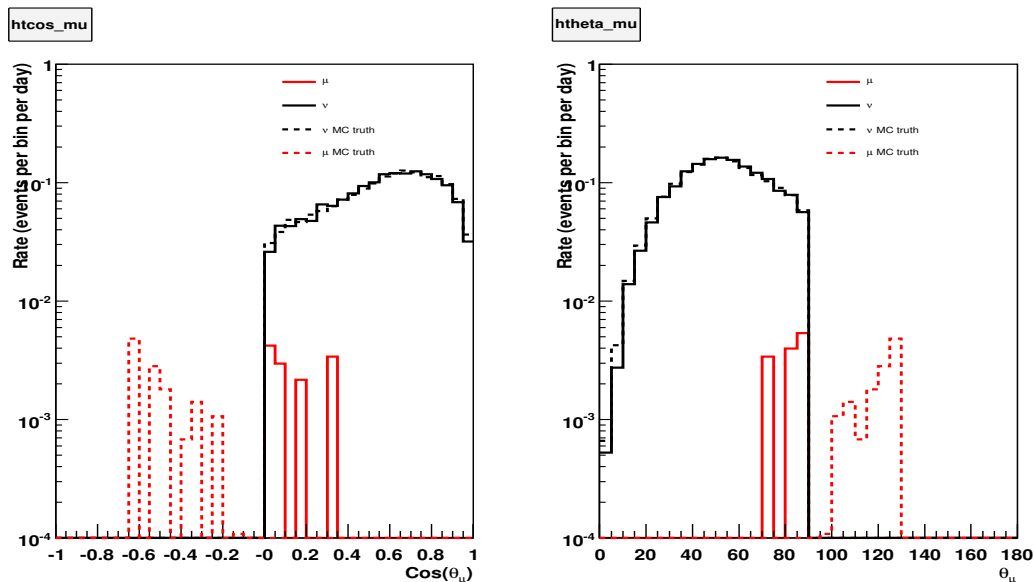
FIG. 5.30 – Cosinus des angles zénithaux (figure de gauche) et angles zénithaux (figure de droite) pour les traces ajustées des muons (en rouge), des neutrinos (en noir) et pour leur angle vrai (vérité MonteCarlo en pointillés) pour les traces montantes reconstruites avec \chi^2_{trace} < 1.45 et \chi^2_{point \text{ lumineux}} > 1.9
