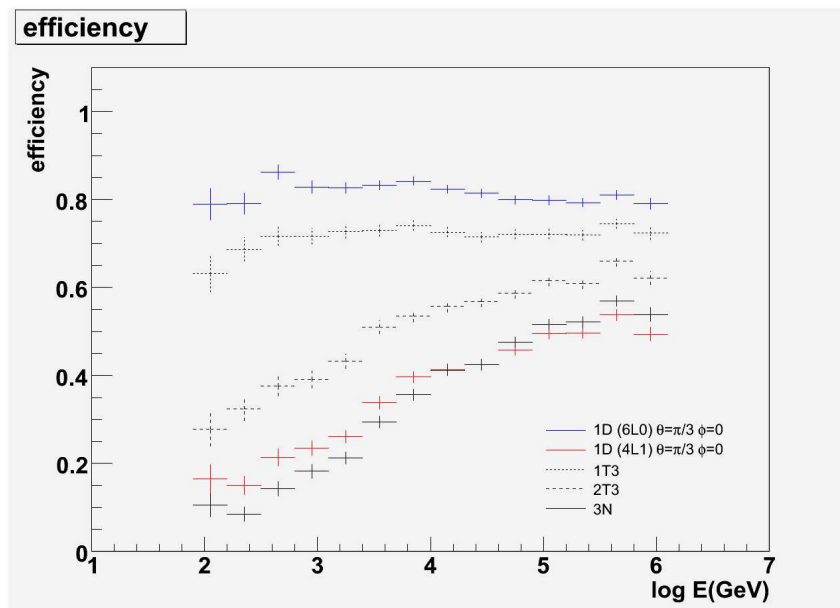
FIG. 5.8 – Comparaisons des efficacités des logiques de déclenchement 1D avec 6L0 (4L1), 1T3, 2T3 et 3N sur un échantillon d'événements simulés dans une direction fixe ( \theta = 60^\circ et \phi = 0^\circ ). La bonne direction est choisie comme direction d'application de la logique 1D pour les courbes noire et rouge.
