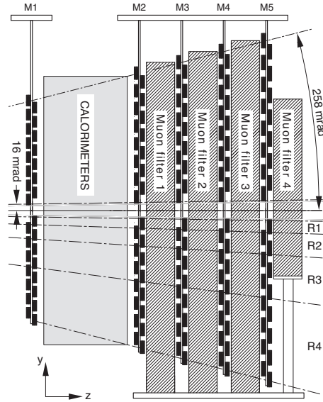
FIG. 2.21: Vue de côté du système à muons.
