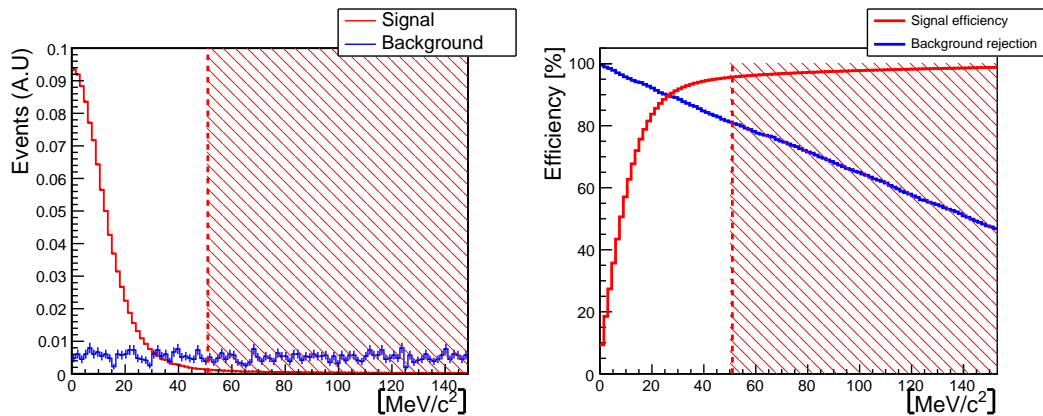
FIG. 4.7: Gauche : distribution de la différence de masse invariante des paires \mu^+ \mu^- avec la masse nominale du méson J/\psi après application de toutes les coupures de sélection du J/\psi pour le signal B^+ \rightarrow J/\psi K^+ (rouge) et pour le bruit de fond inclusif b\bar{b} (bleu). Droite : évolution de l'efficacité et du taux de réjection par rapport à la variation d'une coupure sur |M_{\mu\mu} - M_{J/\psi}| . La coupure choisie, |M_{\mu\mu} - M_{J/\psi}| < 51 \text{ MeV}/c^2 ( 3\sigma ), a une efficacité de 94,2% et un taux de réjection de 80,7%.
