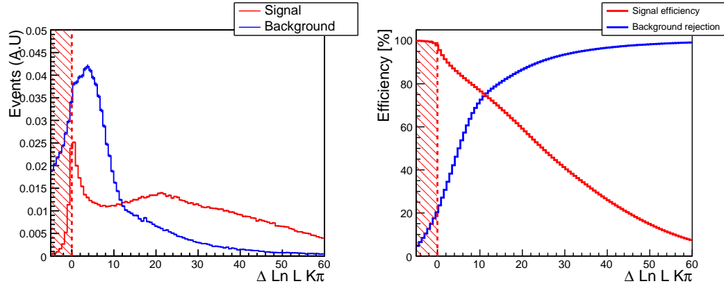
FIG. 4.8: Gauche : distribution du \Delta \ln \mathcal{L}_{K\pi} pour les kaons de signal B^+ \rightarrow J/\psi K^+ (rouge) et ceux de bruit de fond inclusif J/\psi (bleu). Droite : évolution de l'efficacité et du taux de réjection par rapport à la variation d'une coupure sur le \Delta \ln \mathcal{L}_{K\pi} . La coupure choisie, \Delta \ln \mathcal{L}_{K\pi} > 0 , a une efficacité de 95,4% et un taux de réjection de 20,3%.
