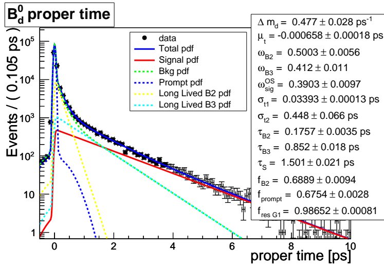
FIG. 5.12: Temps propre d'un exercice Monte-Carlo ajusté avec le modèle complet. Chaque contribution est représentée par une couleur différente. La Table 5.5 donne les valeurs ajustées des paramètres.
