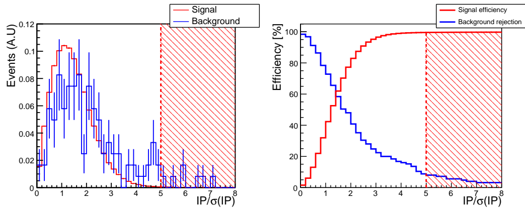
FIG. 4.14: Gauche : distribution des significances des paramètres d'impact du méson B^+ par rapport au vertex primaire IP/\sigma_{IP} pour les candidats B^+ de signal B^+ \rightarrow J/\psi K^+ (rouge) et de bruit de fond inclusif b\bar{b} (bleu). Droite : évolution de l'efficacité et du taux de réjection par rapport à la variation d'une coupure sur IP/\sigma_{IP} . La coupure choisie, IP/\sigma_{IP} < 5 , a une efficacité de 99,4% et un taux de réjection de 8,0%. Le bruit de fond inclusif J/\psi a un taux de réjection nul, c'est-à-dire que tous les événements passent cette coupure.
