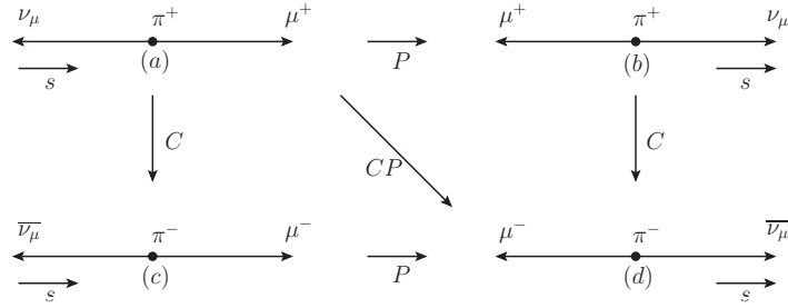
FIG. 1.1: Transformation suivant les symétries \mathcal{C} , \mathcal{P} , et \mathcal{CP} de la désintégration \pi^+ \rightarrow \mu^+ \nu_\mu .
