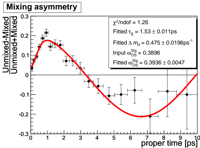
FIG. 5.7: Asymétrie de mélange des événements du lot B_{u,d} \rightarrow J/\psi X , ajustée par le modèle décrit dans ce chapitre. Le \chi^2/n\text{DoF} correspond à l'écart entre la courbe de la PDF et les données. La valeur \text{Input}\omega_{OS}^{\text{sig}} est celle de la fraction de mauvais étiquetage du côté opposé du signal mesuré dans la vérité Monte-Carlo.
