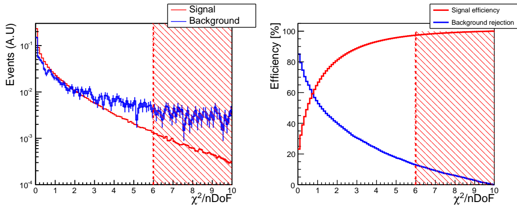
FIG. 4.6: Gauche : distribution de la qualité de vertex \chi_{\text{vtx}}^2/\text{nDoF} pour les candidats J/\psi de signal (rouge) et de bruit de fond (bleu) passant les coupures en impulsion transverse et celles des muons. Droite : évolution de l'efficacité et du taux de réjection par rapport à la variation d'une coupure sur la qualité de vertex \chi_{\text{vtx}}^2/\text{nDoF} . La valeur de coupure choisie, \chi_{\text{vtx}}^2/\text{nDoF} < 6 , a une efficacité de 97,3% et un taux de réjection de 12,7%.
