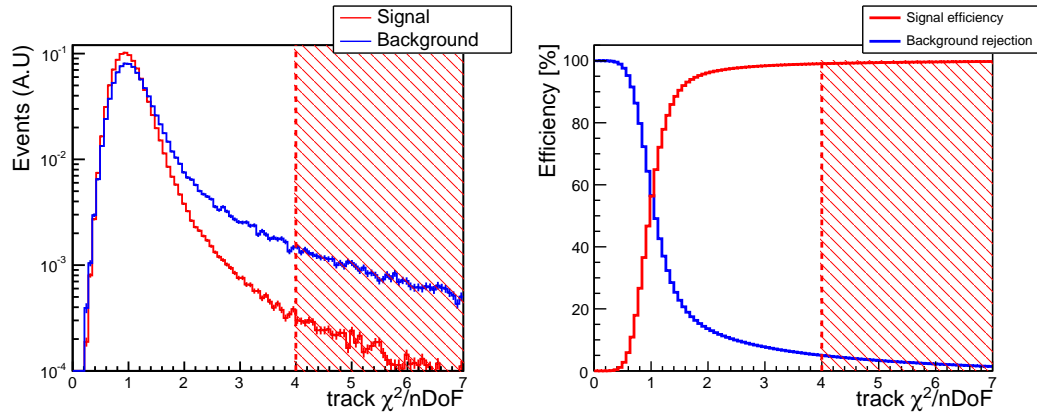
FIG. 4.10: Gauche : distribution de la qualité des traces \chi_{\text{trace}}^2/nDoF pour les kaons de signal B^+ \rightarrow J/\psi K^+ (rouge) et de bruit de fond inclusif J/\psi (bleu). Droite : évolution de l'efficacité et du taux de réjection par rapport à la variation d'une coupure sur la qualité de la trace. La coupure choisie, \chi_{\text{trace}}^2/nDoF < 4 , a une efficacité de 98,7% et un taux de réjection de 5,0%.
