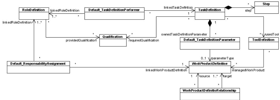
Figure 3-9. Méta-modèle de processus orienté activité de SPEM 2.0 – Method Content .
