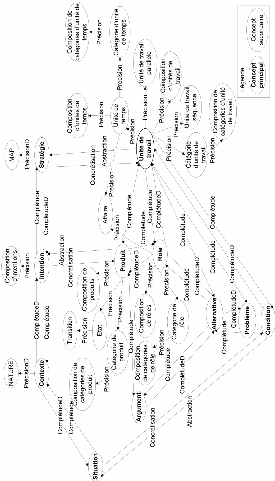
Figure 4-7. Graphe conceptuel.
