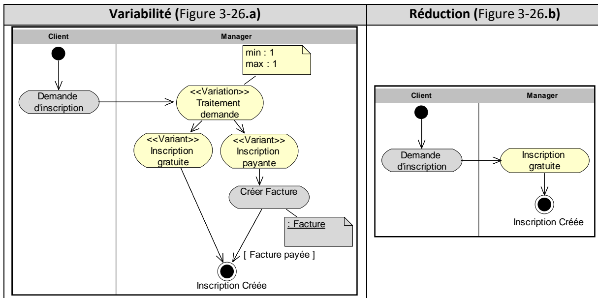
Figure 3-26 : Exemple d'une variation d'objets
