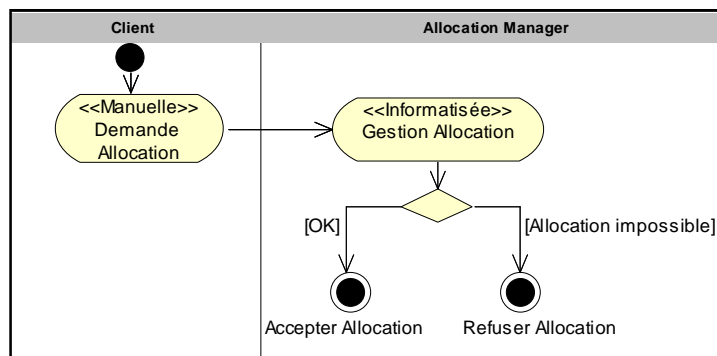
Figure 3-4 : Vue métier du CMP « Allocation de Ressource »
