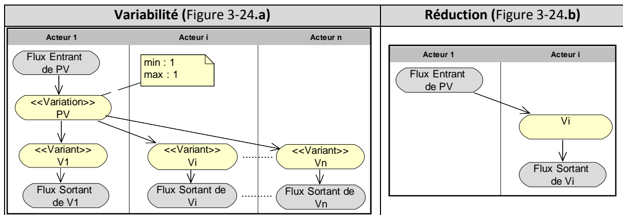
Figure 3-24 : Notations utilisées pour une variation des acteurs
