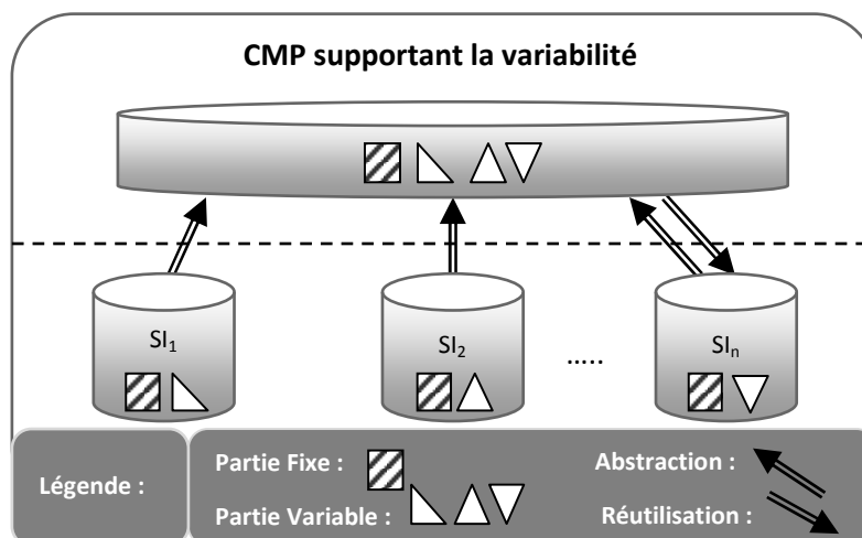
Figure 3-10 : Mécanisme d'abstraction / réutilisation des parties fixes et variables d'un CMP
