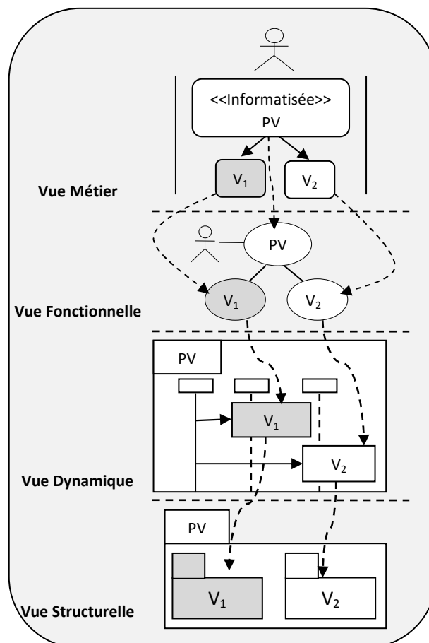
Figure 3-12 : Variabilité multi-vues
