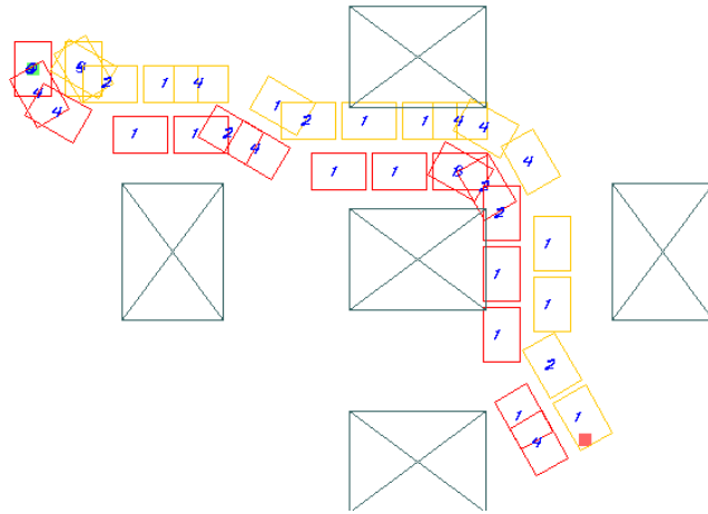
FIG. 6.13 – Séquence de pas en présence d'un grand nombre d'obstacles
