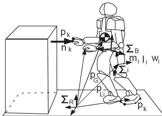
FIG. 3.15 – Exemple de posture où le robot a des contacts sur différents plans [Hirukawa 06]
