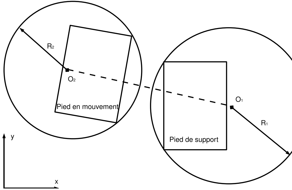
FIG. 3.17 – Les cylindres utilisés pour le calcul de distance afin d’éviter les auto-collisions des membres inférieurs du robot HOAP-3
