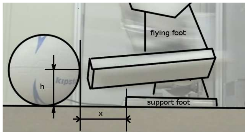
FIG. 5.1 – Schéma des paramètres ( x et h ) du coup de pied.
