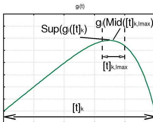
FIG. 4.10 – Représentation de l’approximation de \text{Sup}[g]_i([t]_k) par g_i(\text{Mid}[t]_{k, l_{max}} utilisé pour le calcul du gradient.
