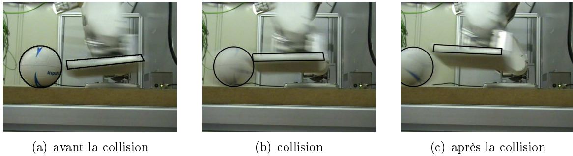
FIG. 5.4 – Représentation de l’impact pour un mouvement optimal avec la balle à x = 3cm au lieu de x = 1cm .
