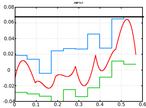
FIG. 4.9 – Planification garantie : Représentation d’une grandeur contrainte (le ZMP) : les encadrements de la fonction respectent les limites, donc la fonction continue les respectent.
