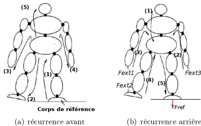
FIG. 3.5 – Principe de l'algorithme de Newton-Euler pour le calcul du modèle dynamique
