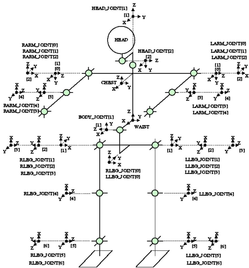
FIG. 3.20 – Représentation des degrés de liberté du robot HOAP-3.
