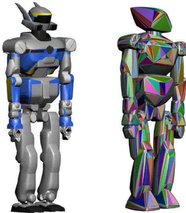
FIG. 3.16 – Le robot HRP-2 et ses volumes englobants [Escande 08]
