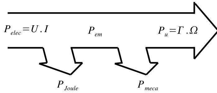
FIG. A.2 – Bilan de puissance d'un moteur à courant continu
