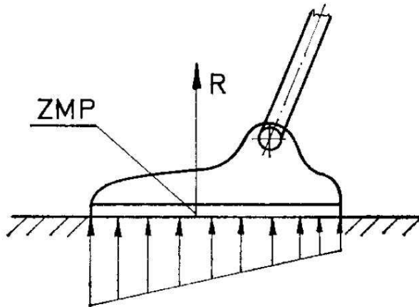
FIG. 3.12 – Définition du Zero Moment Point (ZMP) [Vukobratović 72]
