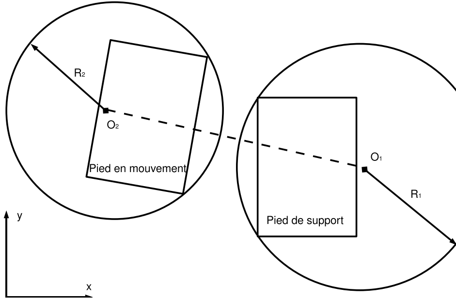
FIG. 3.17 – Les cylindres utilisés pour le calcul de distance afin d’éviter les auto-collisions des membres inférieurs du robot HOAP-3
