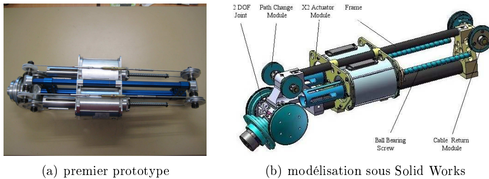
FIG. 3.2 – Représentation de l'actionneur par câble présenté dans [Olaru 09]
