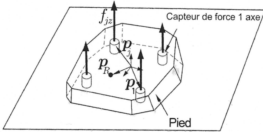
FIG. 3.13 – Définition des variables pour le calcul du ZMP (centre de pression) à partir de plusieurs capteurs de forces un axe
