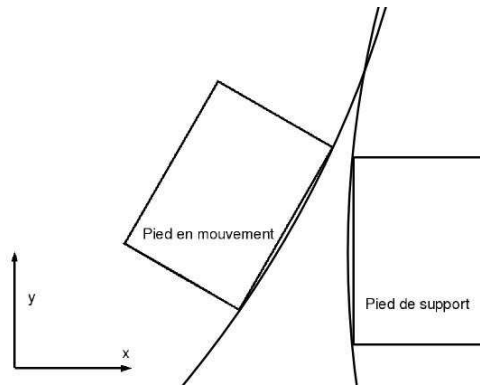
FIG. 3.18 – Les cylindres ayant des rayons importants peuvent s’intersecter alors que les pieds sont suffisamment éloignés
