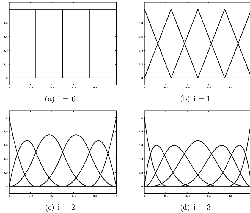
FIG. B.1 – Représentation des Fonctions B-splines
