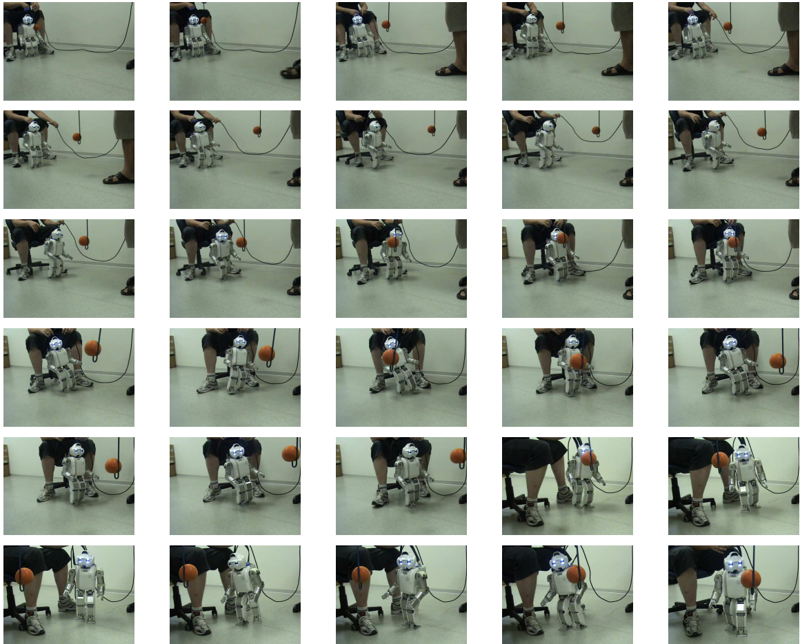
FIG. 6.16 – Expérimentation avec le robot HOAP-3.
