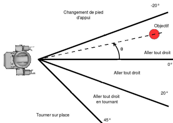
FIG. 6.8 – Algorithme directionnel pour le robot en appui sur le pied gauche.
