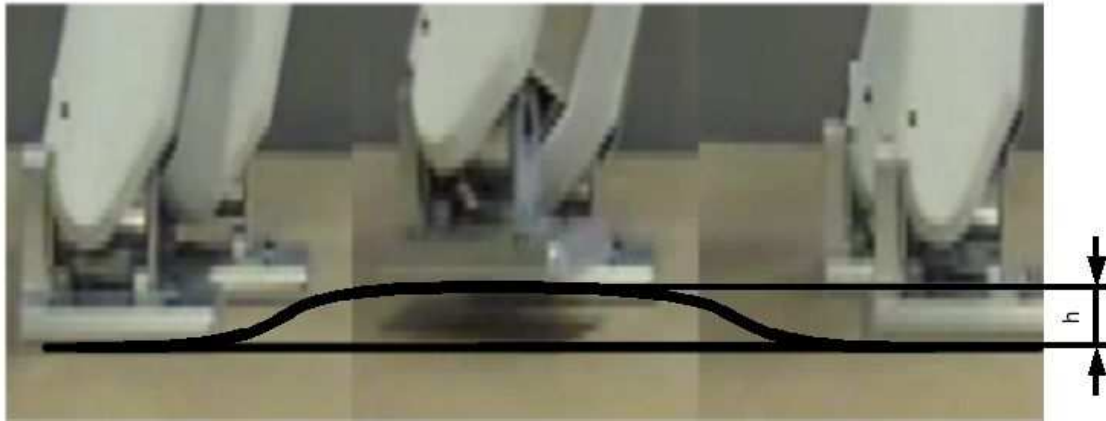
FIG. 4.4 – Représentation de la hauteur du pied pendant la phase de vol.
