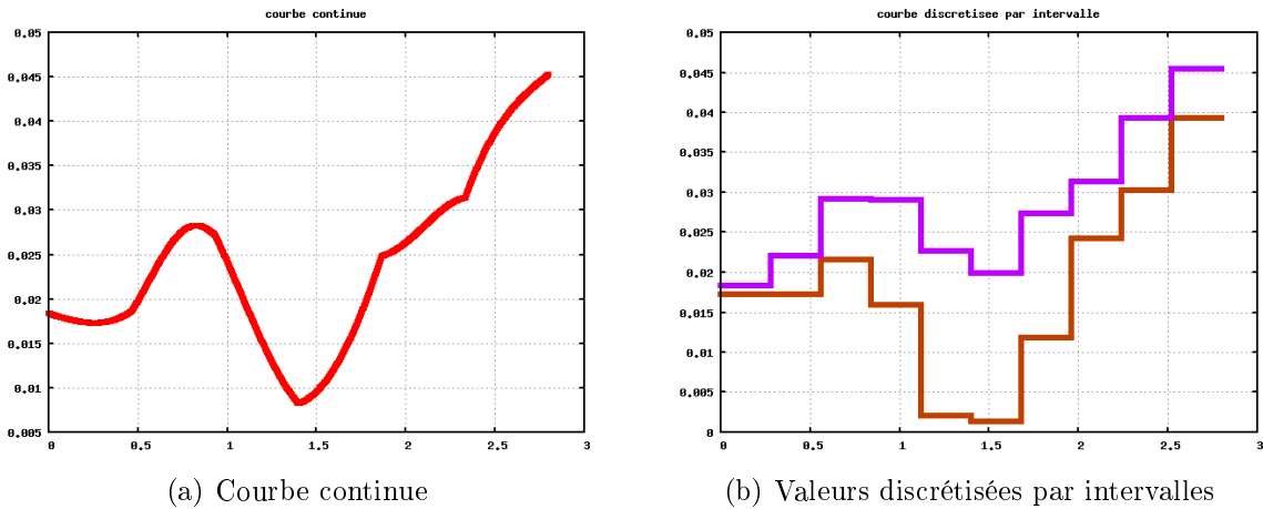
FIG. 4.8 – Discretisation garantie : la courbe continue est assimilée son encadrement pour plusieurs intervalles de temps.
