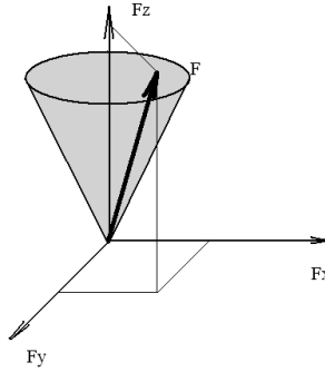
FIG. 3.8 – Représentation du cône de frottement.
