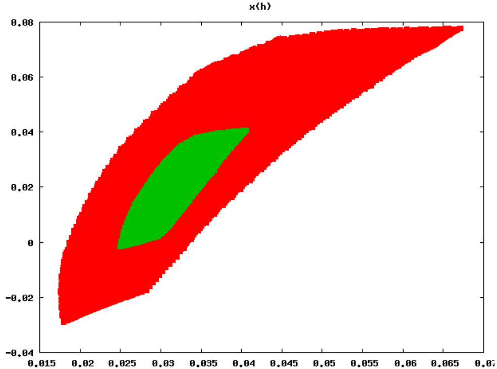
FIG. 5.7 – Représentation de l’ensemble des caractéristiques (x, h) pour les mouvements du sous-ensemble faisable avant l’expansion (en vert) et après l’expansion (en rouge) autour du mouvement optimal x = 1cm , h = 3cm . x en ordonnées et h en abscisse sont exprimé en mètre.
