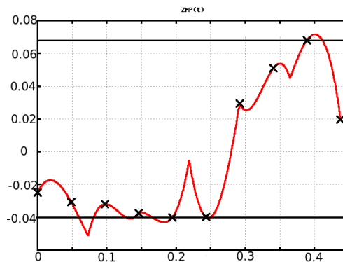
FIG. 4.6 – Représentation d'une grandeur contrainte (le ZMP), obtenue par une optimisation utilisant une grille de 10 instants.
