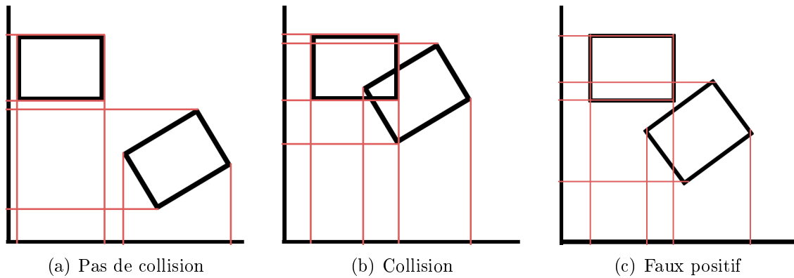
FIG. 6.6 – Test Simple : l’empreinte et l’obstacle sont projetés sur les axes
