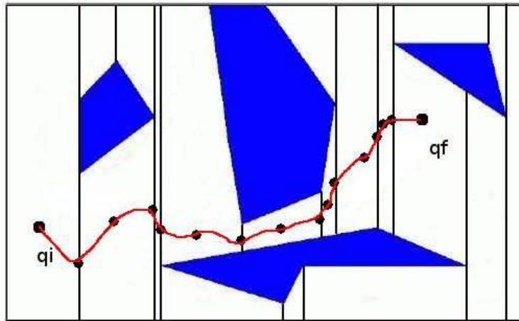
FIG. 2.3 – Décomposition de l'espace libre en sous-espaces
