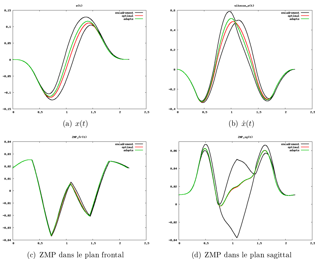
FIG. 5.8 – Représentation temporelle de plusieurs grandeurs pour le mouvement optimal, le mouvement adapté ainsi que l’ensemble des mouvements faisables appartenant à [\mathbb{X}] .
