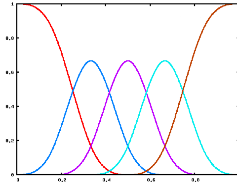
FIG. 3.1 – Représentation des fonctions de base
