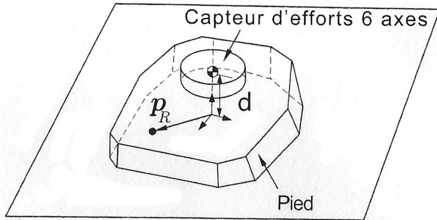
FIG. 3.14 – Définition des variables pour le calcul du ZMP à partir d'un capteur d'effort six axes
