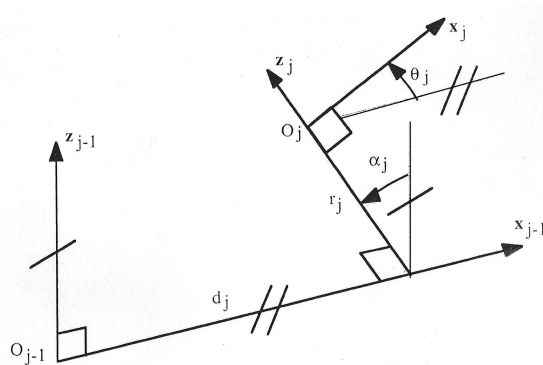
FIG. 3.4 – Représentation des paramètres géométriques de Denavit-Hartenberg [Khalil 02]
