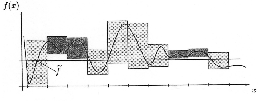
FIG. 4.7 – Optimisation utilisant l'Analyse par Intervalles [Hammer 93].
