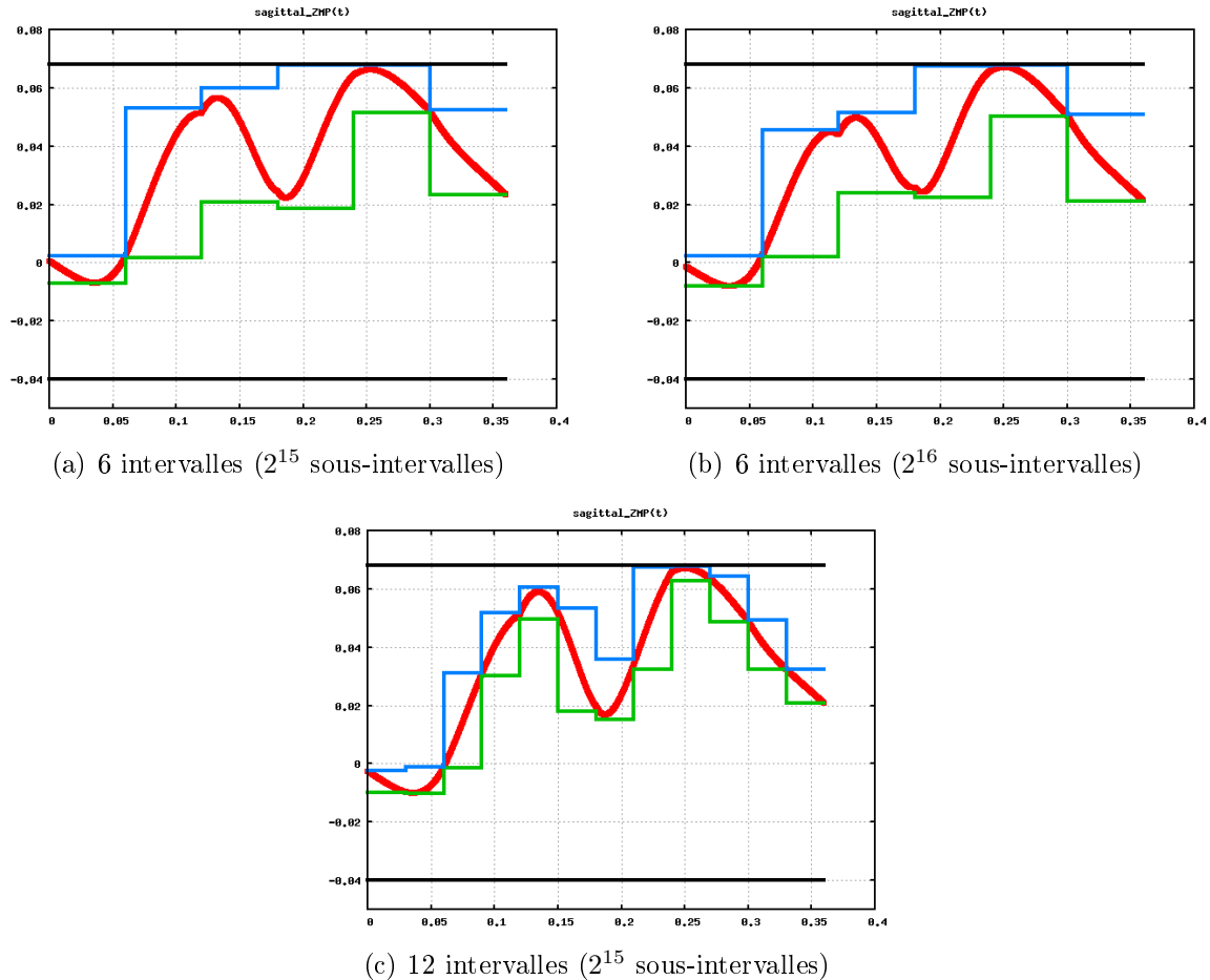
FIG. 4.12 – Représentation du ZMP dans le plan sagittal pour des optimisations utilisant la discrétisation garantie.
