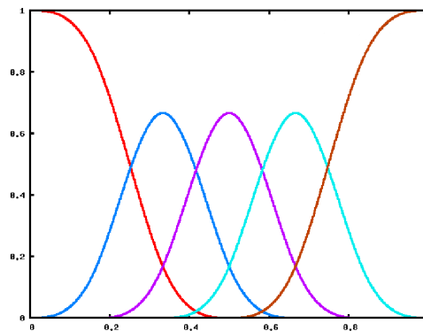
FIG. B.2 – Représentation des fonctions de base
