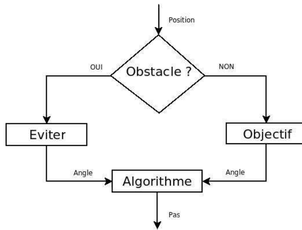
FIG. 6.10 – Algorithme incluant la détection d’obstacle.
