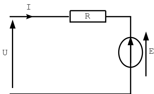
(a) modèle électrique
