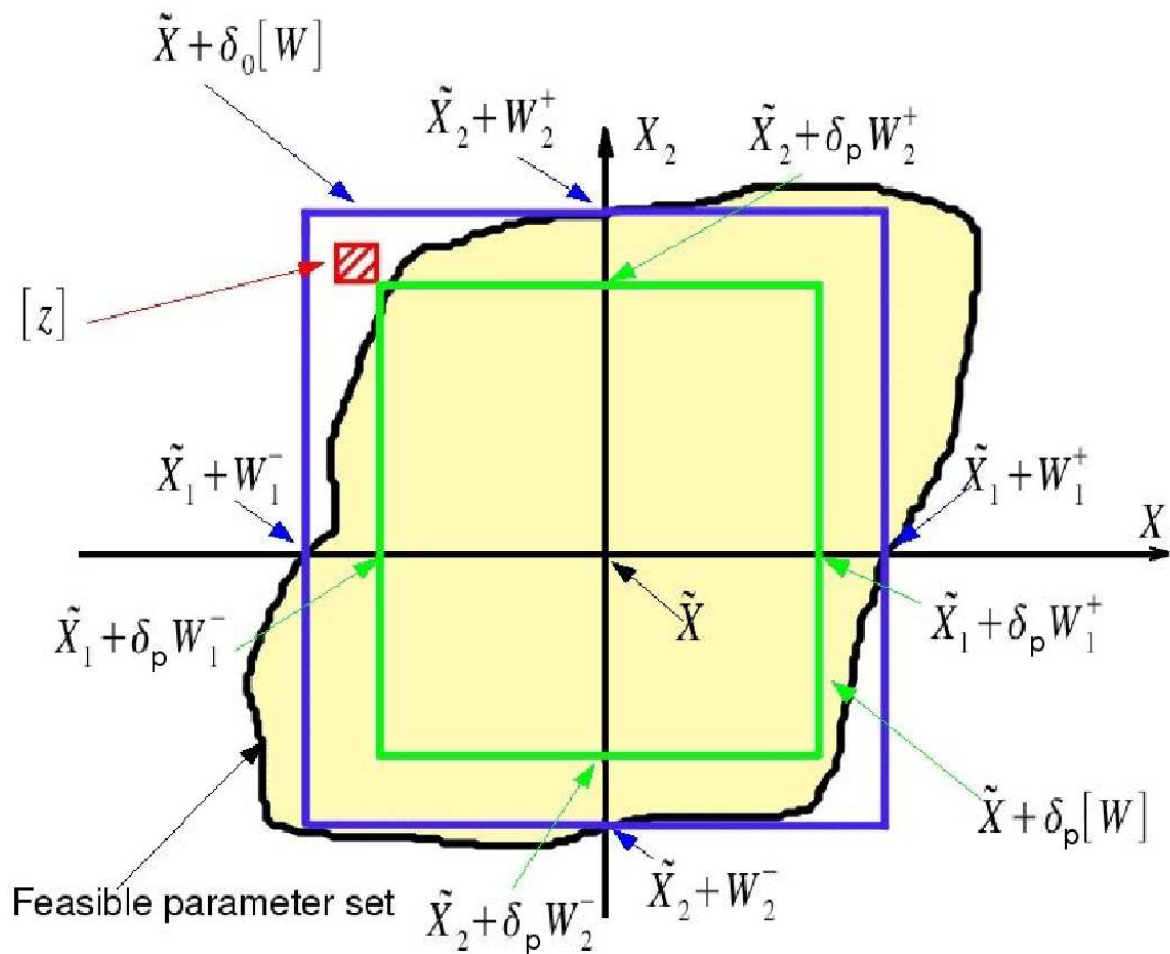
FIG. 5.5 – Exemple d'une ensemble faisable et de son approximation intérieure : [X]
