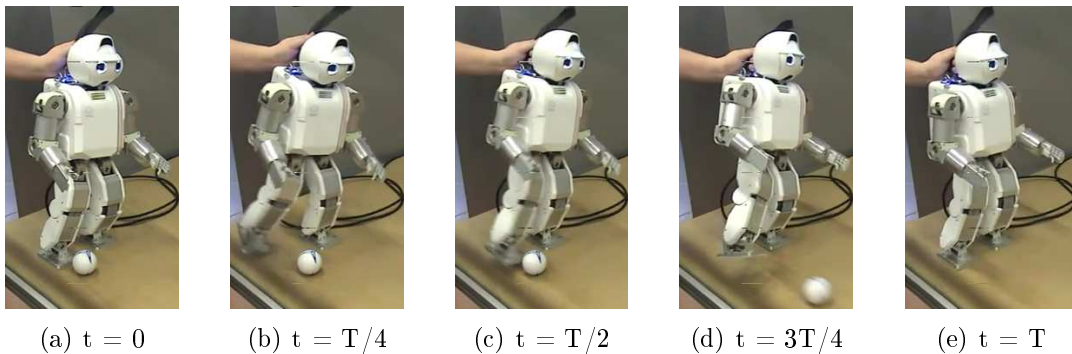
FIG. 4.3 – Exemple d’un mouvement de coup de pied
