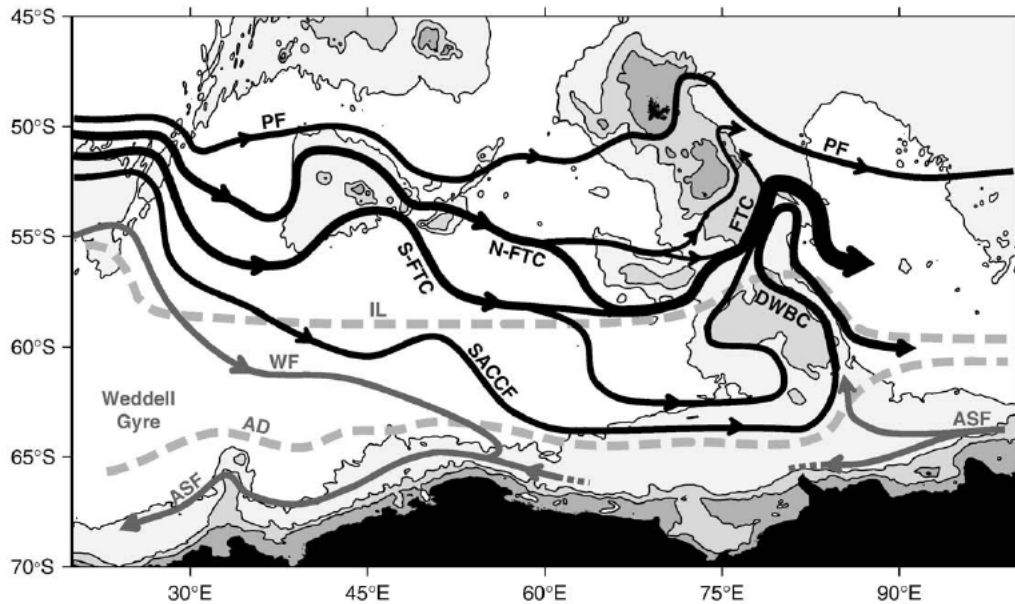
FIGURE 3.9: Schéma de la circulation océanique proposé par Roquet et al. [2009], à partir de l'analyse de données d'éléphants de mer combinées avec des données historiques et satellitaires.
