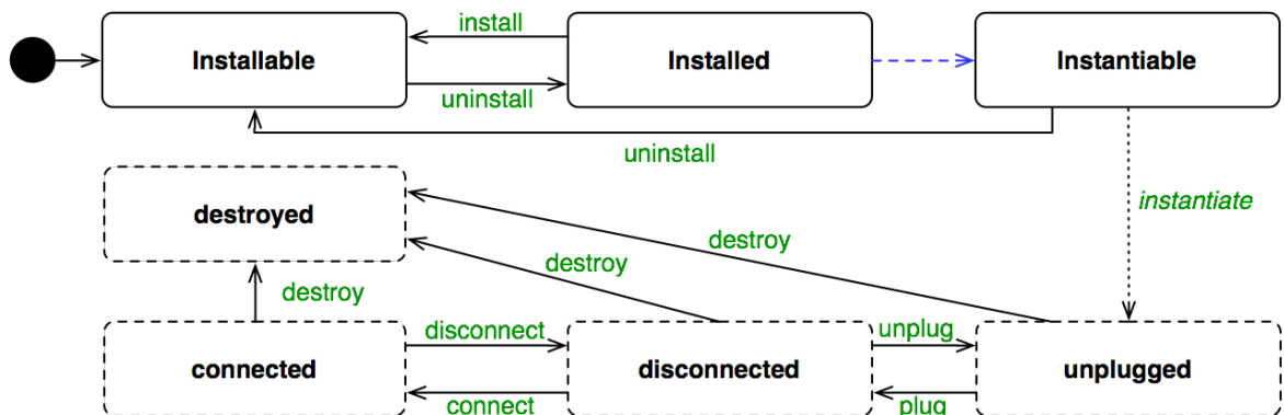
Figure V-9 Cycle de vie des extrémités de connecteurs Ethylene. Le disque noir pointe l'état initial. Les états dont l'encadrement est un trait continu s'inscrivent dans la phase « inerte ». Les états dont l'encadrement est un trait discontinu s'inscrivent dans la phase « instance ». Les flèches dont le trait est discontinu dénote une transition automatique. La flèche dont le trait est en pointillé dénote la création d'une nouvelle entité.
