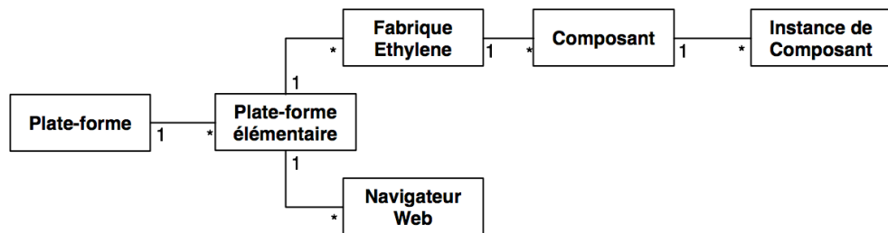
Figure VI-17 Modèle de plate-forme modifié pour intégrer l’approche Ethylene.
