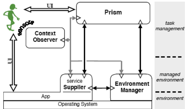
Figure III-11 Les composants d'Aura pour un environnement. [d'après Sousa05, p.42].
