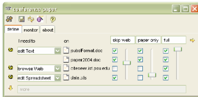
Figure III-12 Méta-IHM de Aura pour définir une tâche incluant une édition de texte (« edit text » avec les « materials » pubsFormat.doc et paper2004.doc), l'utilisation du web sur citeseer et d'un tableur. La partie droite de l'écran permet de spécifier des préférences.
