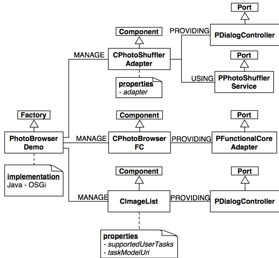
Figure VI-25 Spécification générale des composants ImageList , PhotoShufflerAdapter et PhotoBrowserFC et de leur fabrique.
