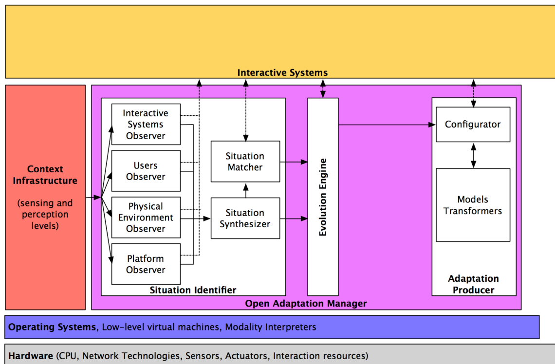
Figure V-4 Décomposition fonctionnelle : un premier affinage. Dans ce modèle en couches, les côtés supérieurs des boîtes offrent une API à destination des couches supérieures. Les flèches continues dénotent des échanges d'information et leur direction. Les flèches en pointillé indiquent les fonctions rendues accessibles par API aux couches supérieures.
