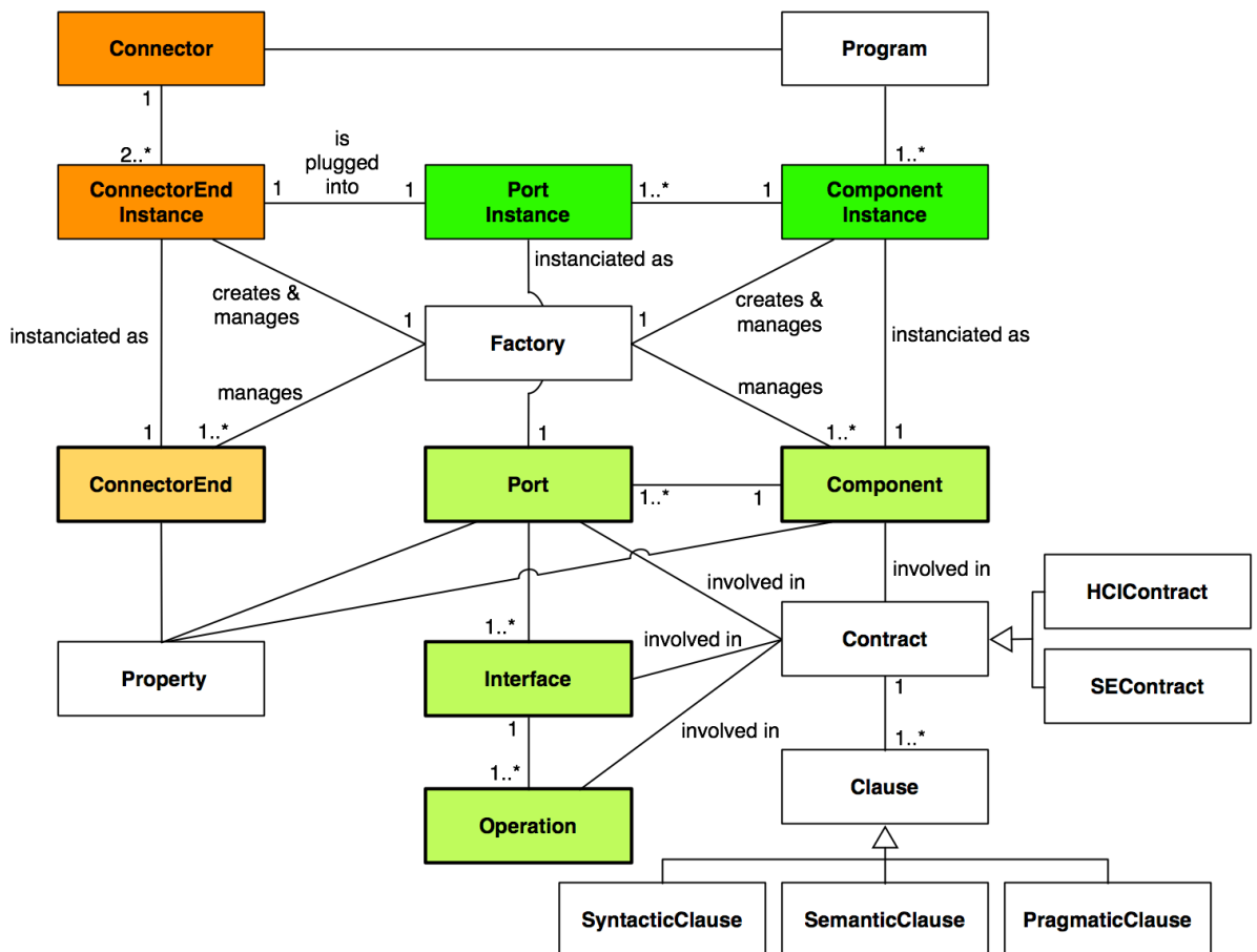
Figure V-8 Diagramme de classes du modèle Ethylene . Les boîtes colorées à encadrement épais modélisent les composants et connecteurs sous leur forme inerte. Les boîtes colorées à encadrement fin modélisent les instances de composants et de connecteurs. Les boîtes blanches modélisent les concepts périphériques. Les relations sans étiquette symbolisent la relation est composé de . Lorsque la cardinalité d'une relation n'est pas indiquée, cette cardinalité vaut *.
