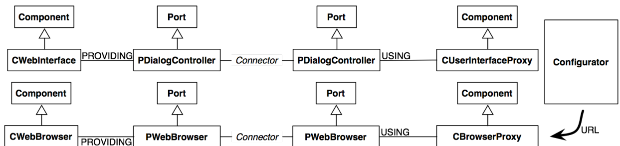
Figure VI-21 Assemblage d'un composant Web (CWebInterface), d'un composant navigateur web (CWebBrowser) et passage de l'URL de l'IHM de CWebInterface au navigateur.
