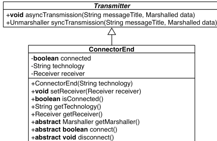
Figure VI-6 Attributs et méthodes de la classe ConnectorEnd.
