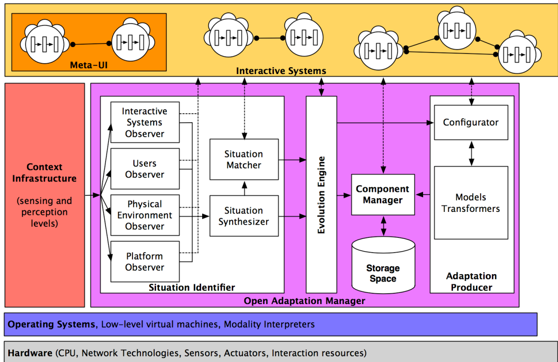
Figure V-5 Décomposition fonctionnelle : affinage final. La sémantique de cette figure est la même que dans la figure précédente. Les symboles en forme de fleur représentent des composants logiciels. Les segments terminés par de petits disques noirs symbolisent des liaisons entre composants.
