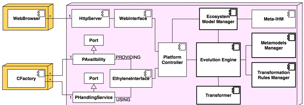
Figure VI-18 Architecture modifiée de l'infrastructure MARI qui intègre une interface d'accès aux technologies à composants conformes au modèle Ethylene.
