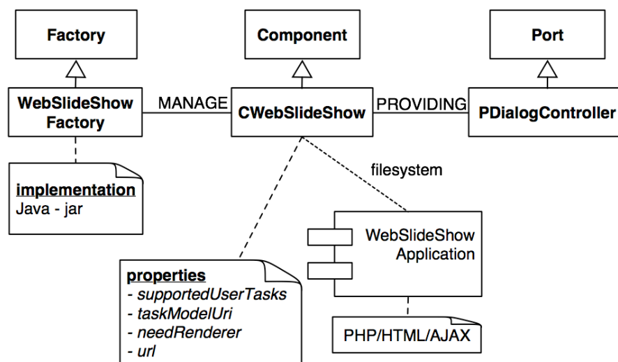
Figure VI-28 Spécification générale du composant WebSlideShow et de sa fabrique.
