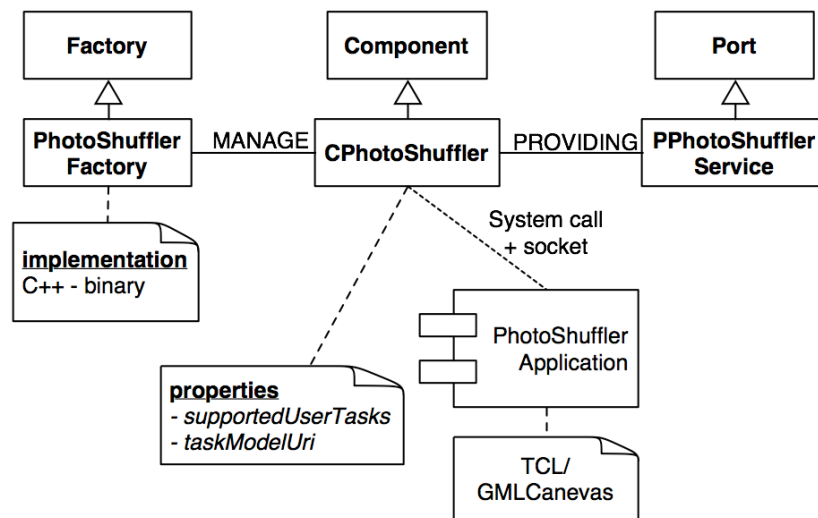
Figure VI-24 Spécification générale du composant PhotoShuffler et de sa fabrique.
