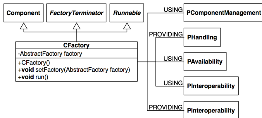
Figure VI-13 Spécification de l’encapsulation d’une fabrique concrète.
