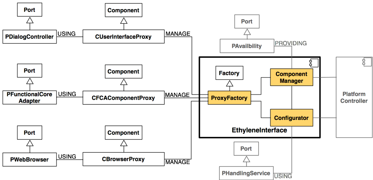
Figure VI-19 Détail du service « EthyleneInterface ». Ce service se décompose en trois fonctions : le gestionnaire de composant chargé d’assumer le rôle d’annuaire de composant, le configurateur chargé de la manipulation des instances de composants et une fabrique de composants mandataires destinés à l’interaction logique avec les composants IHM et les composants ANF.
