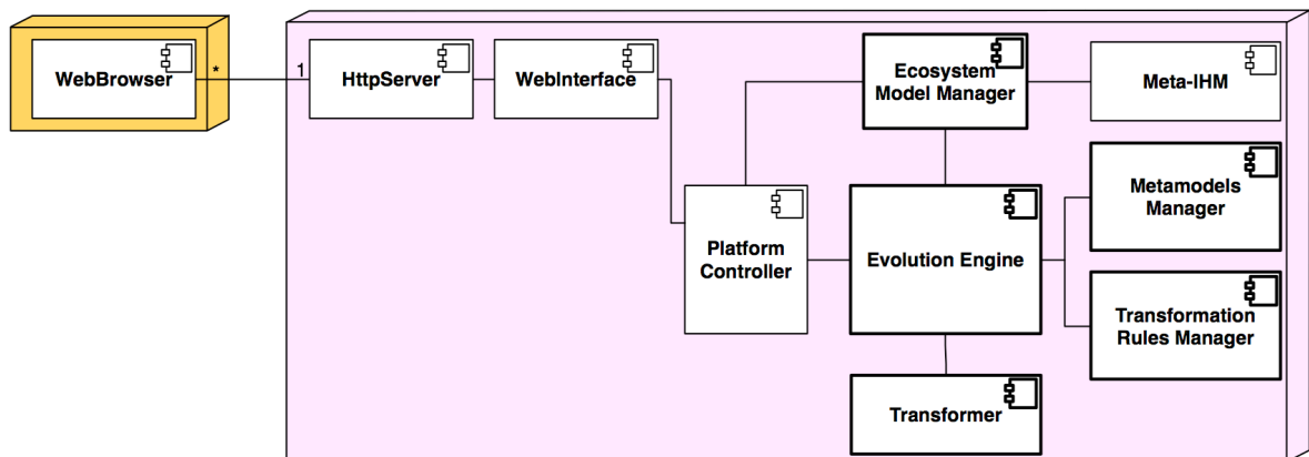
Figure VI-14 Architecture initiale de l'infrastructure MARI. Les services dont l'encadrement est épais forment le cœur fonctionnel de MARI. Les boîtes en « trois dimensions » représentent des plates-formes matérielles.
