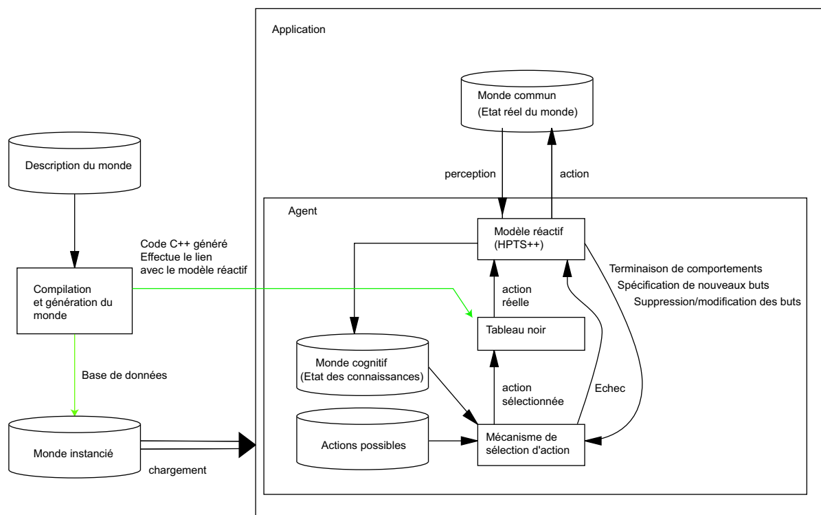
FIG. 4.1 – Architecture d'utilisation de BCOOL.
