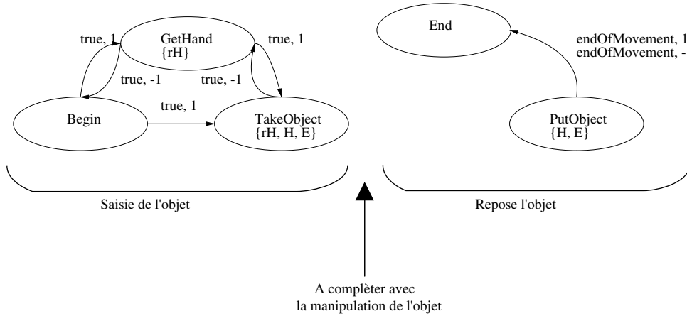
FIG. 3.14 – Patron d'automate de manipulation d'objet à une main.
