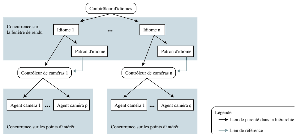
FIG. 5.15 – Architecture du système de cinématographie.
