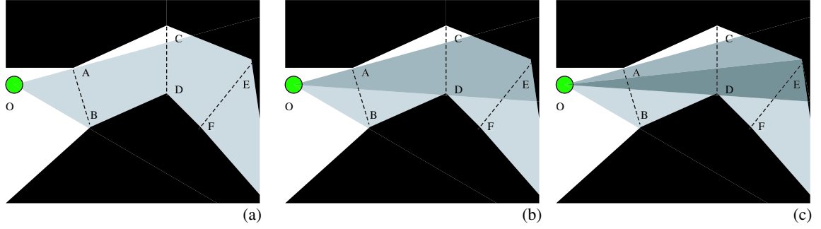
FIG. 2.4 – Calcul d'intersection des cônes de visibilité jusqu'à la limite de visibilité. Les trois niveaux de gris représentent les trois intersections successives.
