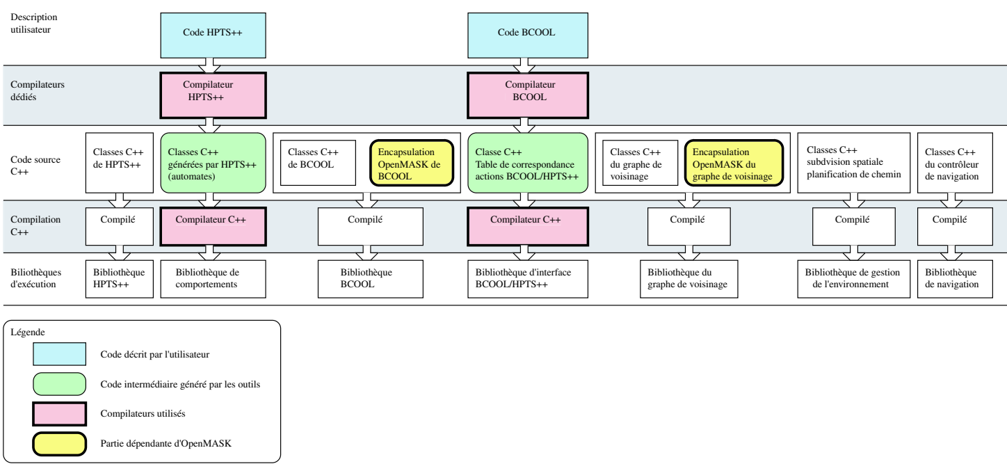
FIG. 5.1 – Insertion de l'architecture dans OpenMASK et interventions de l'utilisateur.
