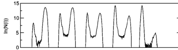
FIGURE 3.24: Histogrammes de l'intensité laser pour différents courants de pompe issus de [7].
