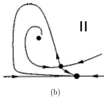
FIGURE 3.14: Excitabilité.
