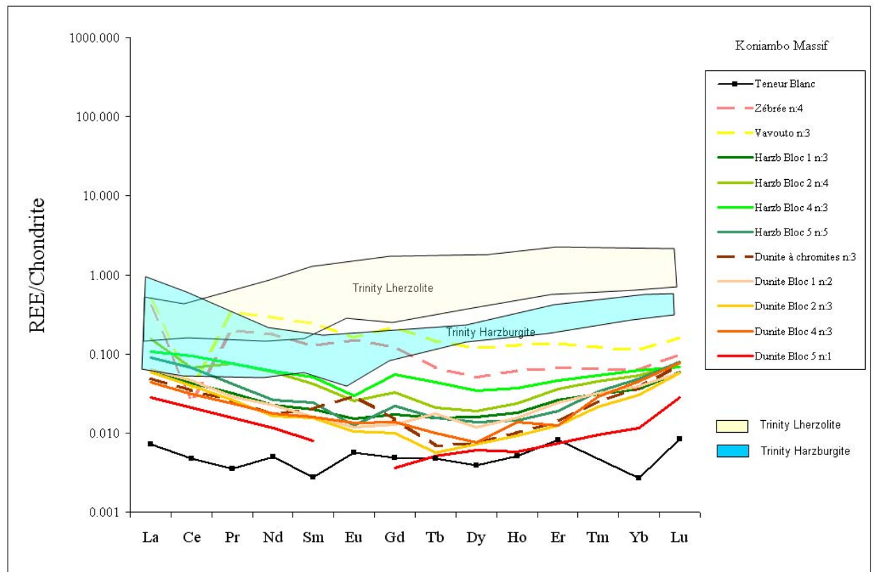
Figure 1.13: Spectres des terres rares (TR) normalisées aux chondrites pour l'ensemble des membres de la séquence ultramafique du massif du Koniambo incluant les péridotites à faciès Vavouto et à texture zébrée. Note : le trait noir représente la limite de détection des différentes TR telle qu'elle a pu être déterminée par la méthode d'analyse appliquée, « n » représente le nombre d'échantillons dans chaque catégorie. Pour fin de comparaison les résultats d'analyses pour des séquences ultramafique de l'ophiolite Trinity (USA) sont représentés (Gruau et al. , 1998).
