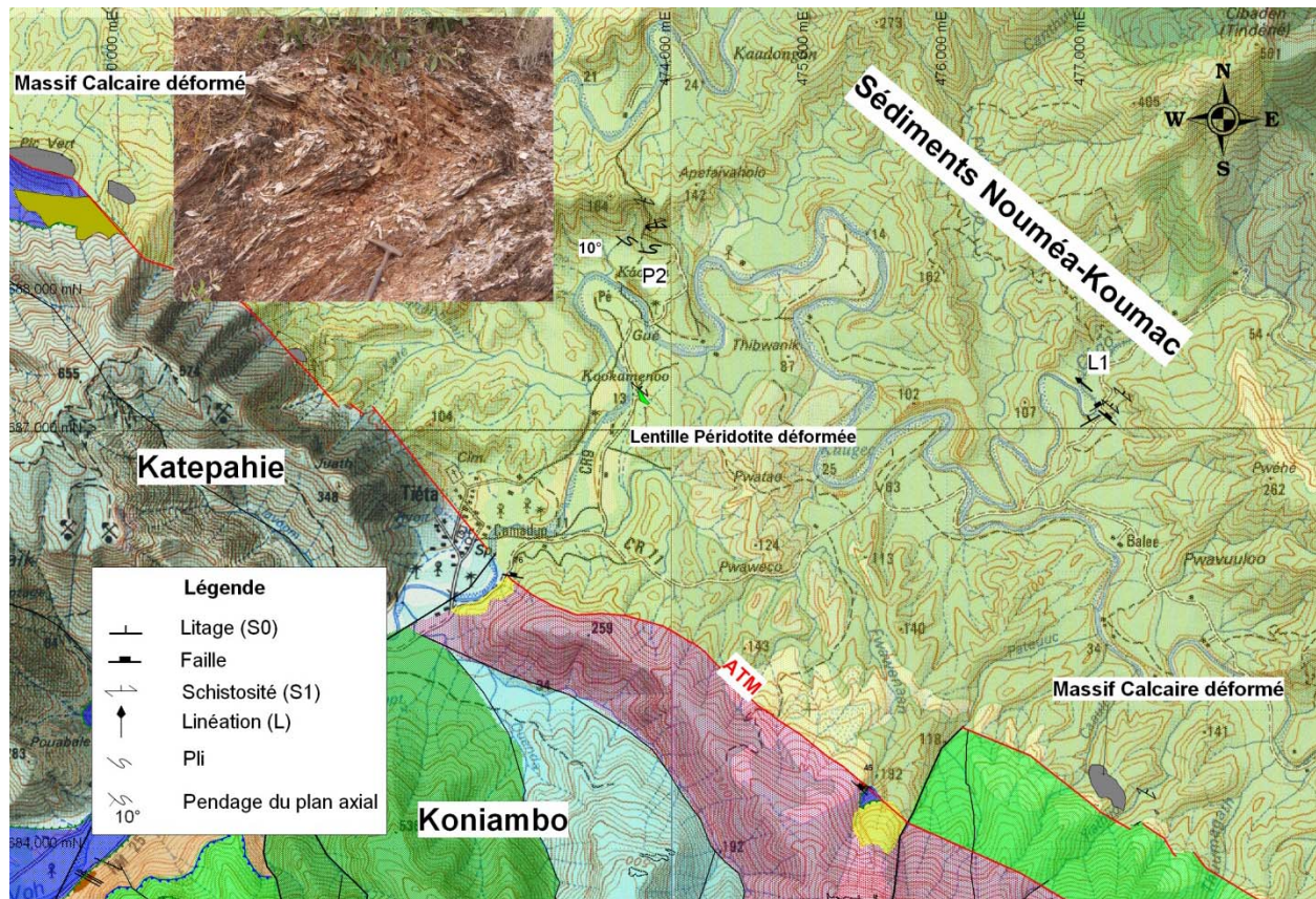
Figure 3.10: Détail structural au sein du corridor de déformation associé à l'ATM dans les sédiments de l'Unité Nouméa-Koumac. Charnière de plis (P2) avec plan axial orienté 095^\circ à pendage subhorizontal. Linéation d'étirement (L1) plongeant à 39^\circ vers le NO le long d'un plan de faille orienté 310^\circ/39^\circ , parallèle à l'ATM. Voir la légende de la Figure 3.2 pour le descriptif des unités géologiques.
