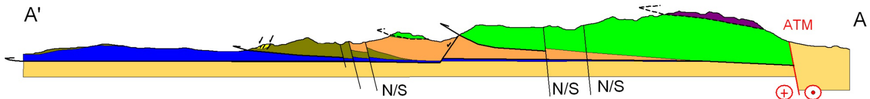
Figure 1.3: Coupe géologique de l'empilement tectonique des diverses unités et séquences formant le massif du Koniambo, A-A'; coupe ENE-OSO présentée sur la Figure 2.2.
