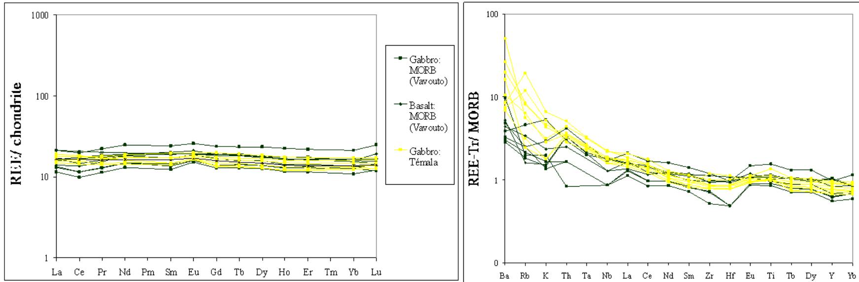
Figure 1.7: Diagrammes discriminants REE/chondrite (a) et REE-Tr/MORB (b) présentant l'affinité tholéiitique de type MORB enrichie en éléments LIL pour les gabbros de la région de Témala. Les gabbros et basaltes MORB de Vavouto sont présentés pour comparaison.
