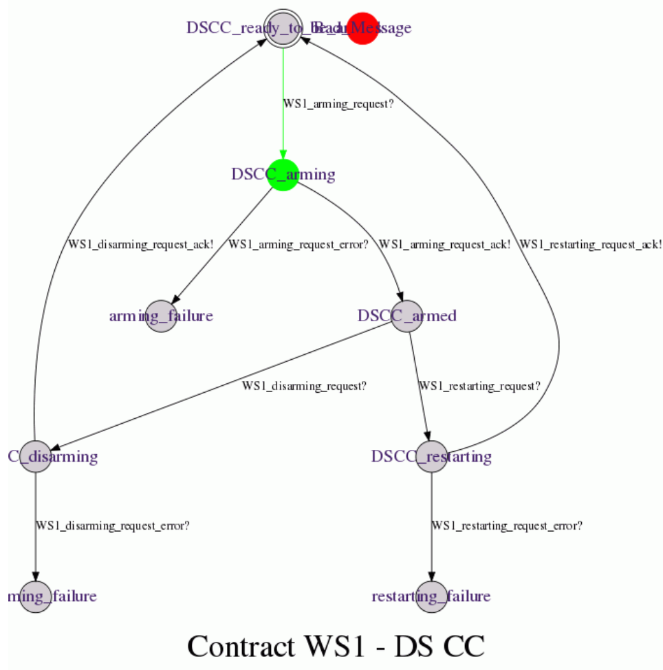
Figure 64 : détection de la réception d'un message erroné.
