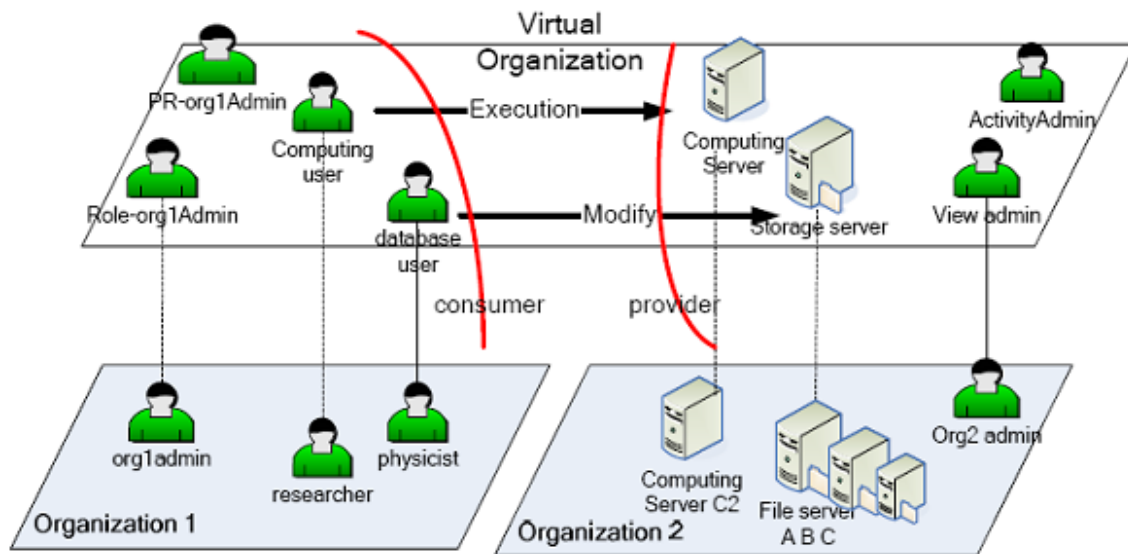
Figure 22 : Le modèle OrBAC au sein d'un environnement sous forme de grille [Nasser, 2006].
