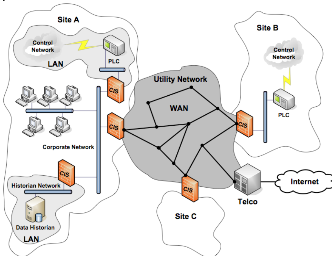
Figure 39 : Architecture CRUTIAL d'une infrastructure d'information critique.
