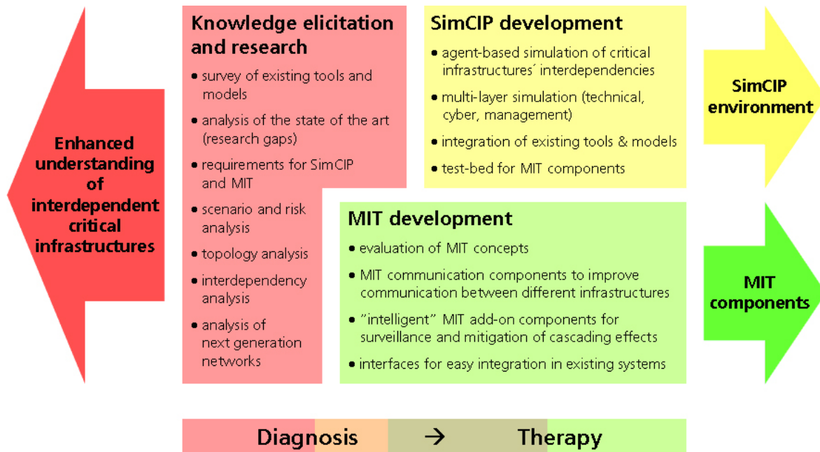
Figure 8 : Architecture générale du projet IRRIS.
