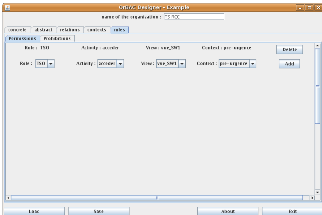
Figure 53 : Spécification d'une règle de contrôle d'accès avec l'outil OrBAC Designer.
