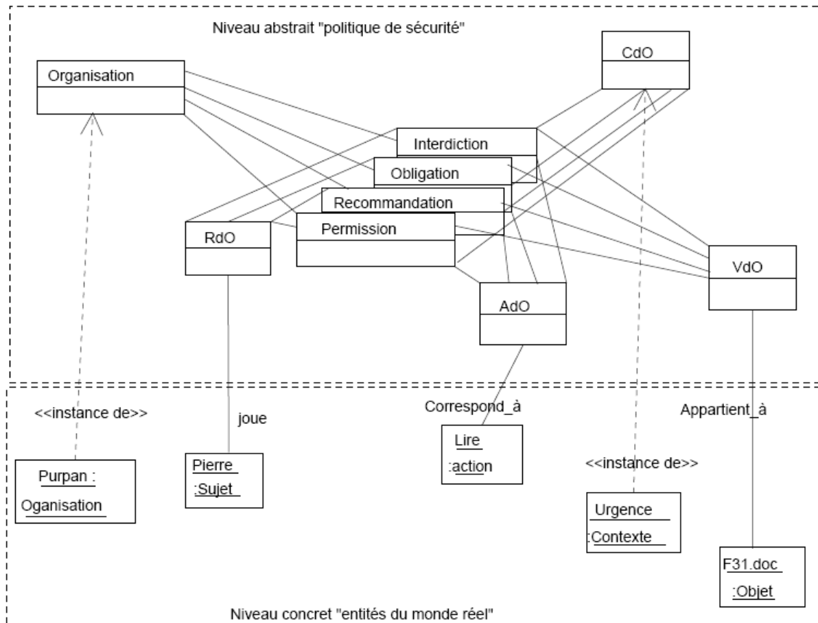
Figure 20 : Exemple d'instanciation d'une règle de sécurité Multi-OrBAC.
