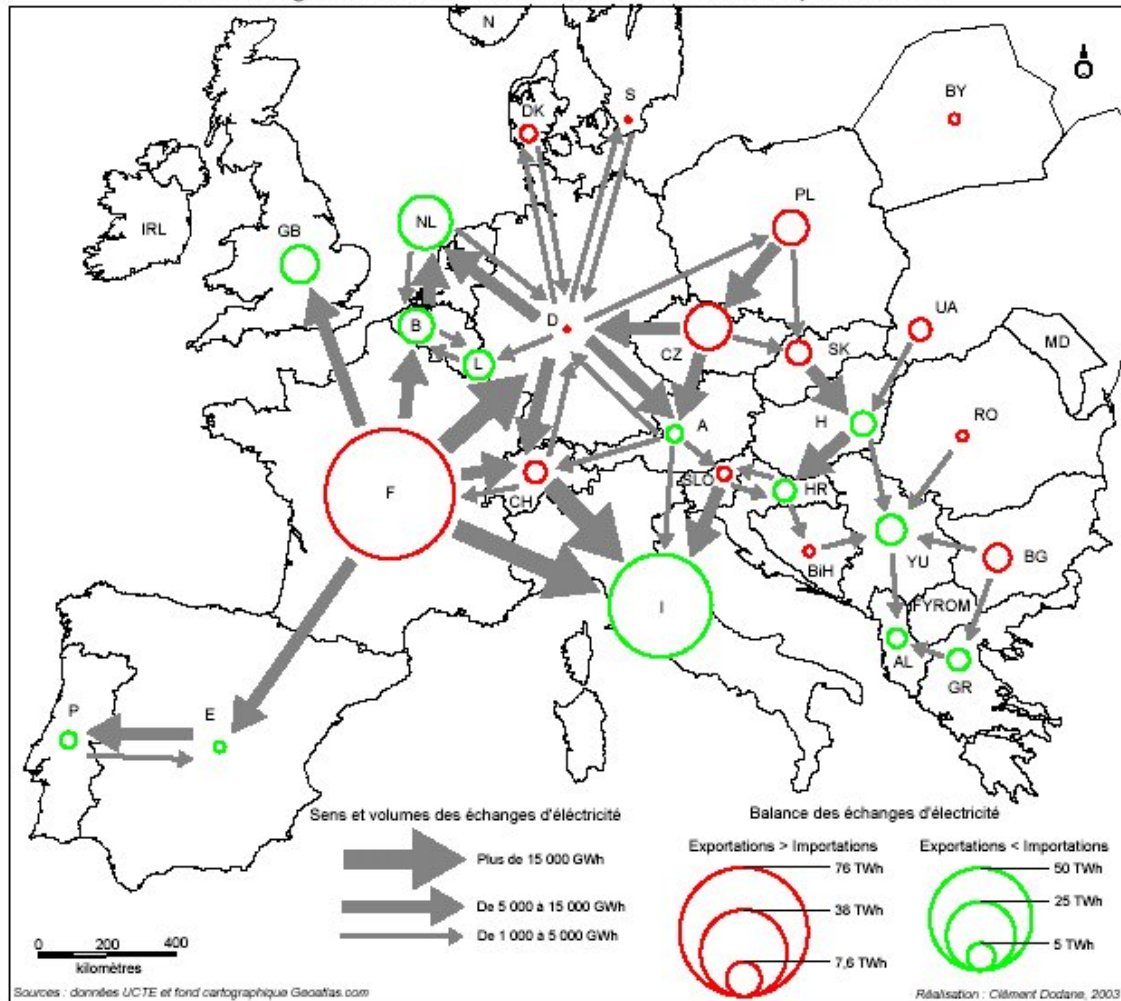
Figure 7 : Interdépendances entre les réseaux électriques européens 2 .
