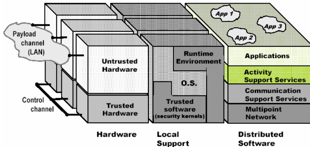
Figure 9 : Architecture des nœuds CRUTIAL.
