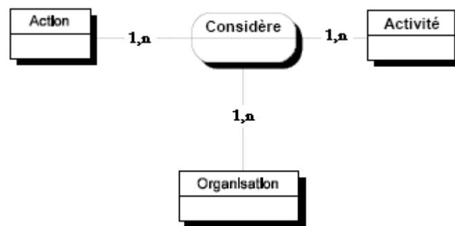
Figure 14 : La relation « Considère ».
