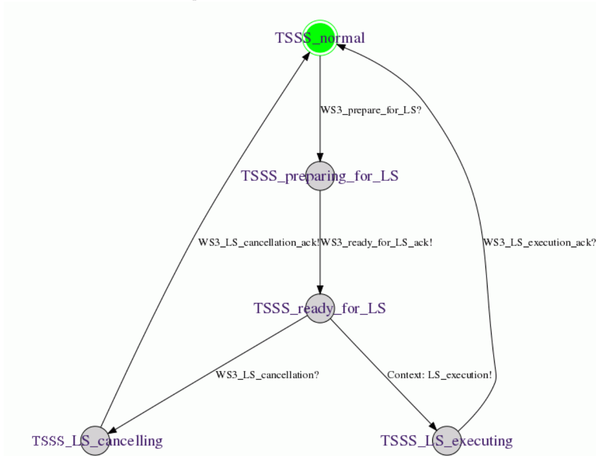
Figure 70 : Automate de SW3-préparation_de_délestage au niveau du TS SS.
