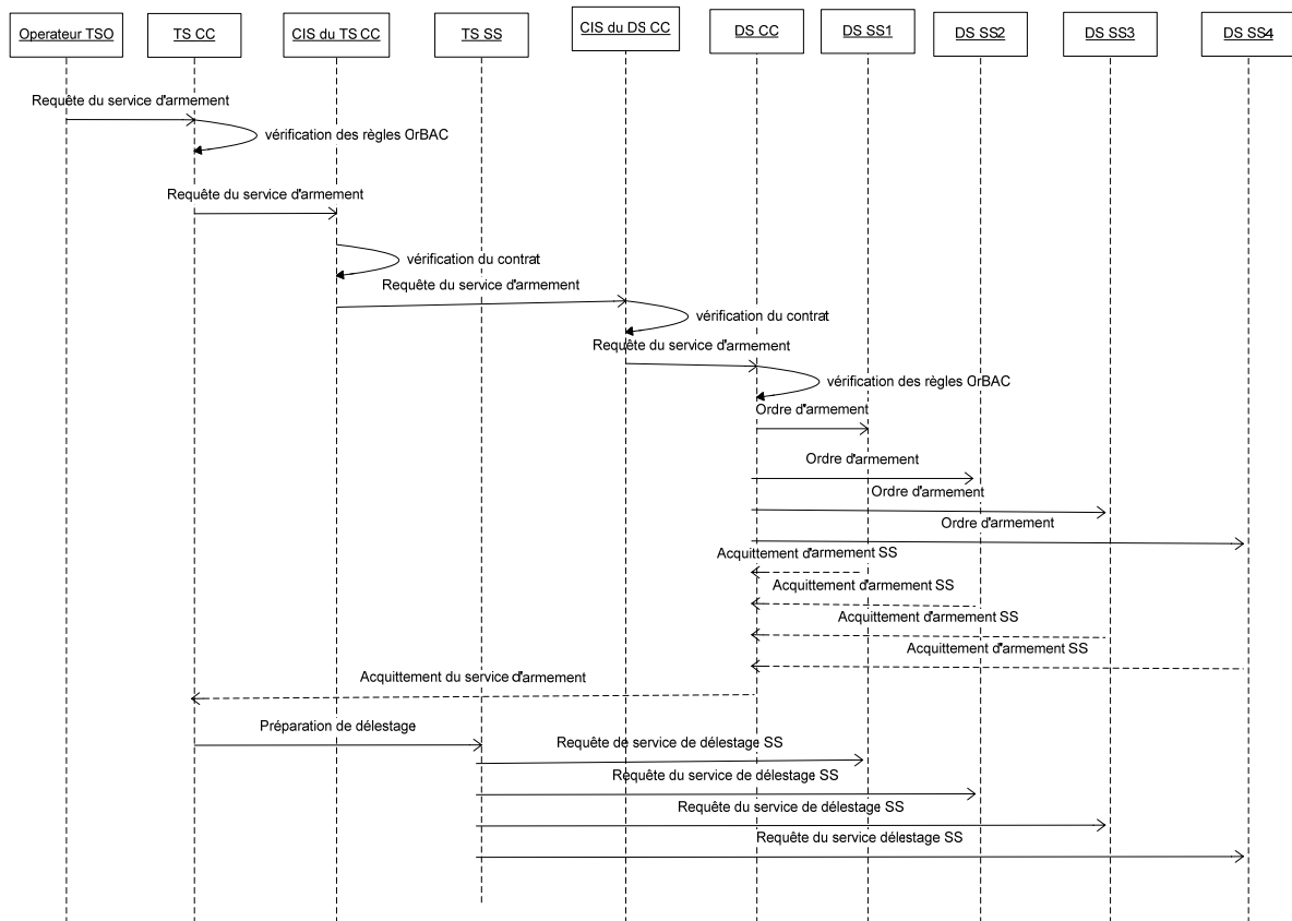
Figure 46 : Application du modèle PolyOrBAC au scénario de délestage.
