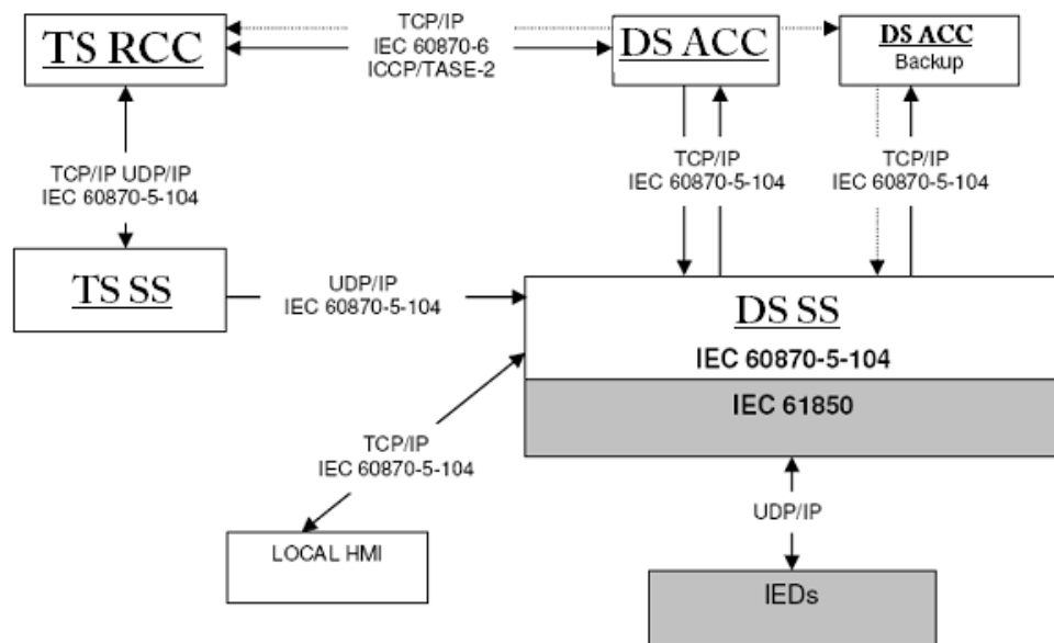
Figure 36 : Les flux d'information et protocoles de communication [Garrone et al., 2007].
