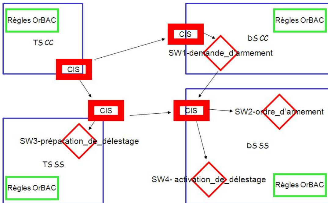
Figure 40 : Application du modèle PolyOrBAC au scénario de déstage.
