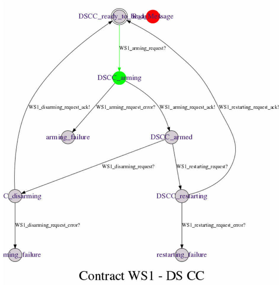
Figure 68 : Le contrat signale la réception d'un message erroné.
