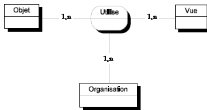
Figure 13 : La relation « Utilise ».
