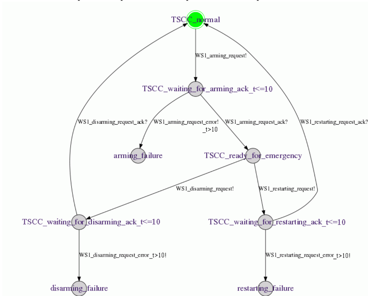
Figure 42 : Automate de SW1-demande_d'armement au niveau du TS CC.
