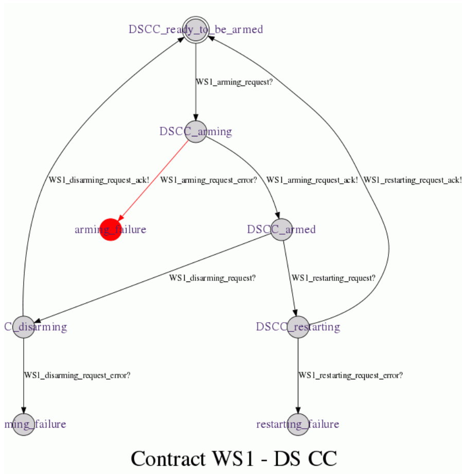
Figure 66 : Contrat dans un état d’erreur après un timeout.
