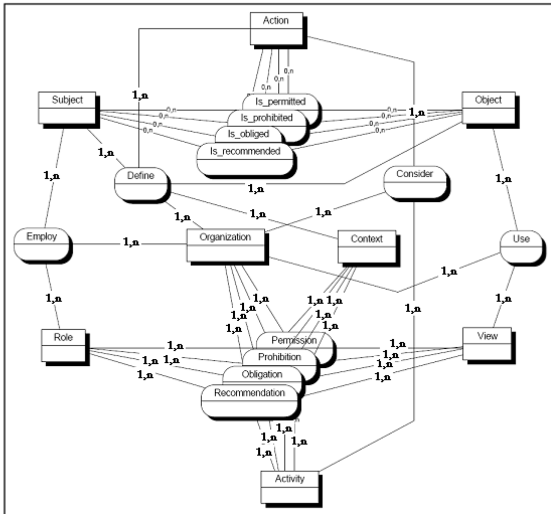
Figure 16 : Structure du modèle OrBAC [Abou El Kalam et al. , 2003].
