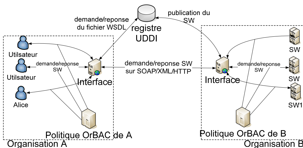
Figure 26 : L'architecture de l'approche PolyOrBAC.
