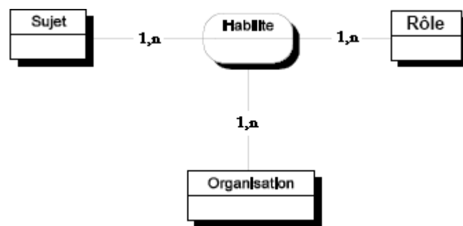
Figure 12 : La relation « Habilite ».
