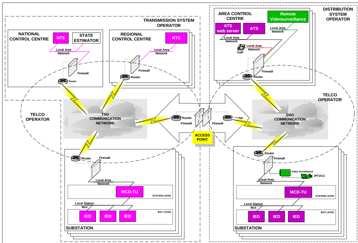
Figure 35 : Système de contrôle à distance des TSO et DSO [Garrone et al., 2007].
