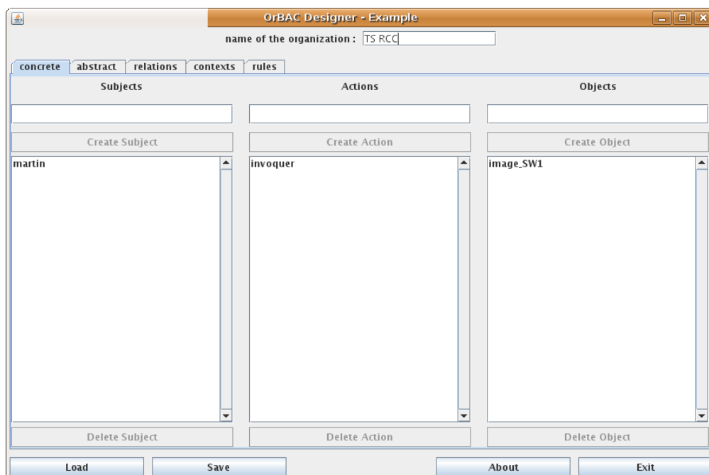
Figure 51 : Outil OrBAC Designer : niveau concret.
