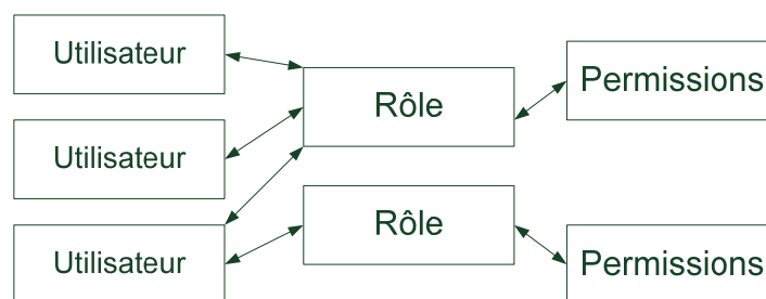
Figure 10 : Positionnement de la notion de rôle dans le fonctionnement de RBAC.
