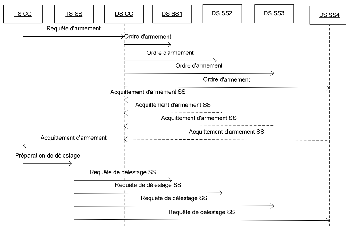
Figure 38 : Diagramme de séquence du scénario de délestage.
