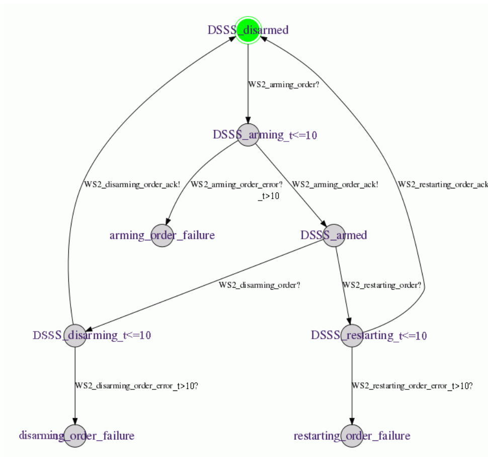
Figure 45 : Automate pour WS2-arming-order au niveau du DS SS.
