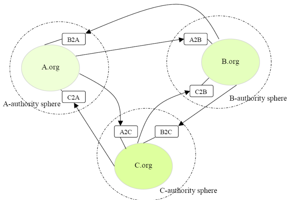
Figure 23 : Fonctionnement du modèle O2O [Coma 2006].
