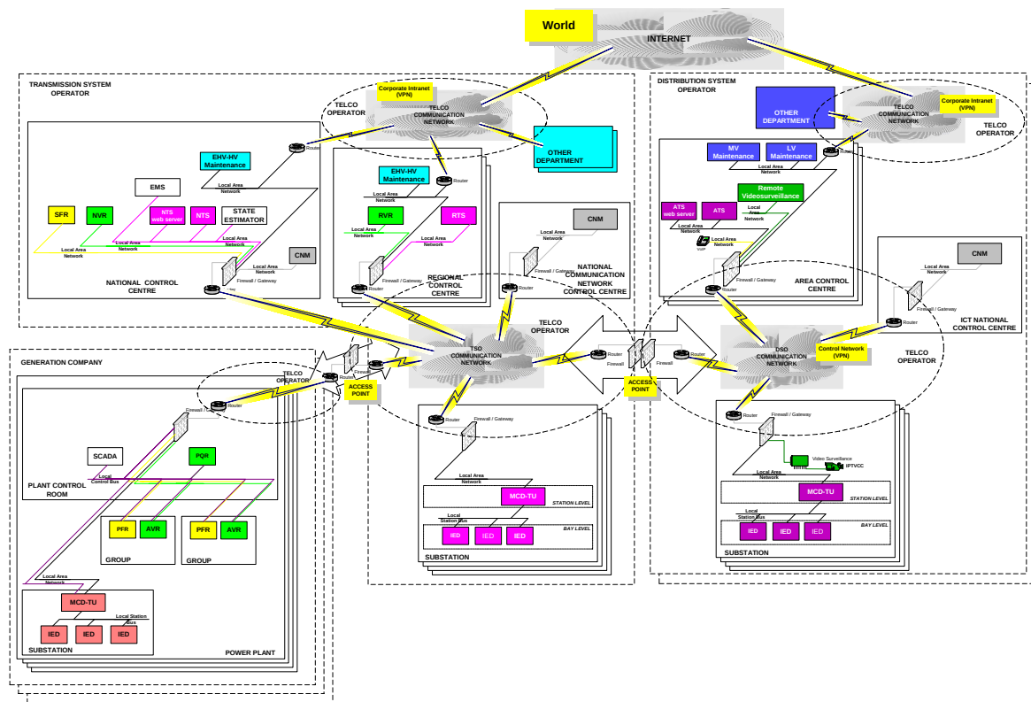
Figure 33 : Infrastructure d'information et de communication d'une IPE [Garrone et al., 2007]
