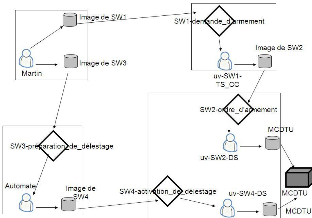
Figure 41 : Application des notions d'image de service Web et d'utilisateur virtuel au scénario.
