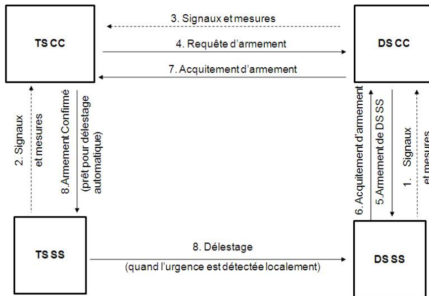
Figure 37 : Signaux et mesures échangés dans le scénario de délestage.
