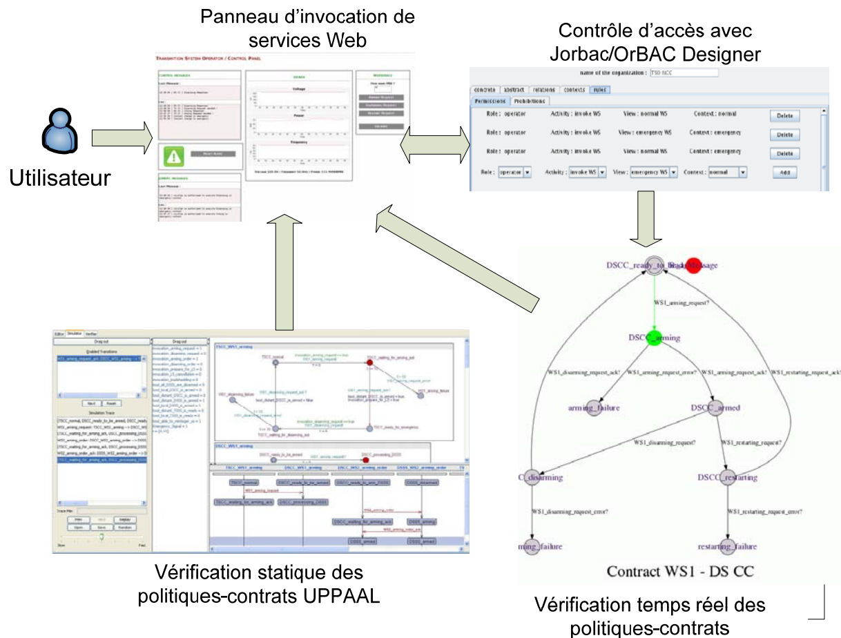
Figure 48 : Plateforme PolyOrBAC.
