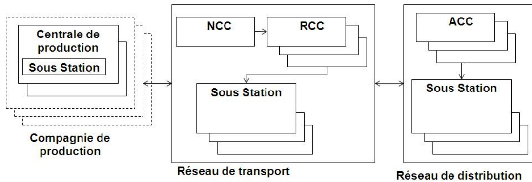
Figure 34 : Architecture générale d'une IPE.
