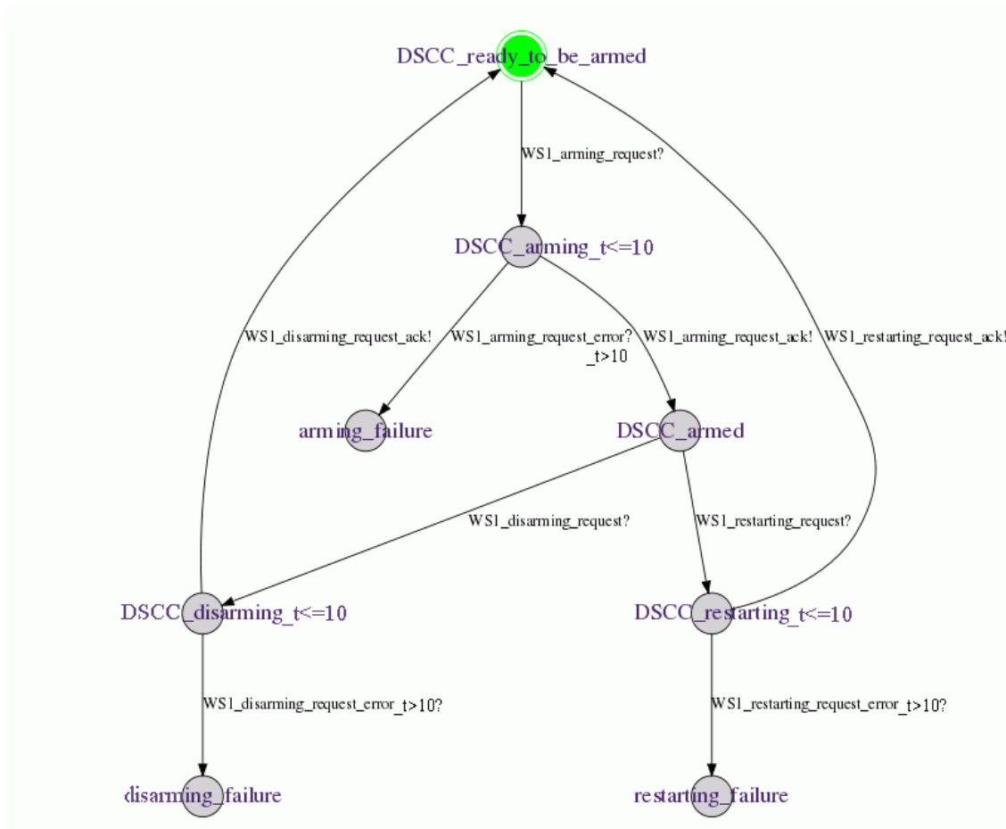
Figure 43 : Automate de SW1-demande_d'armement au niveau du DS CC.
