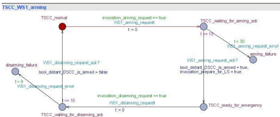
Figure 55 : Exemple d'automate temporisé pour la représentation de politiques-contrats.
