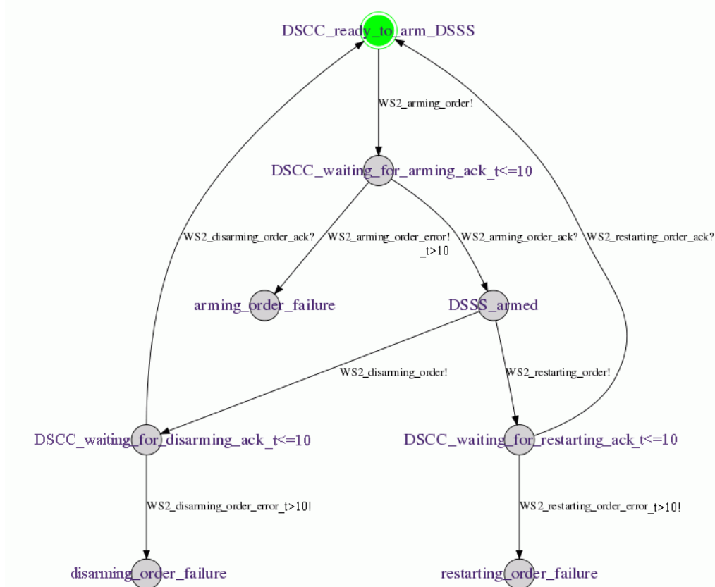
Figure 44 : Automate pour SW2-ordre_d'armement du côté du DS CC.
