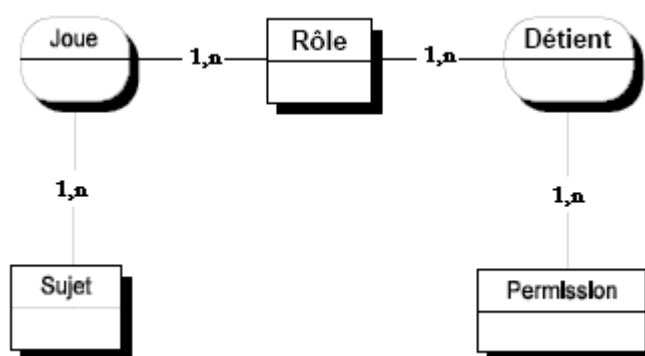
Figure 11 : La relation « détient » et la relation « joue »
