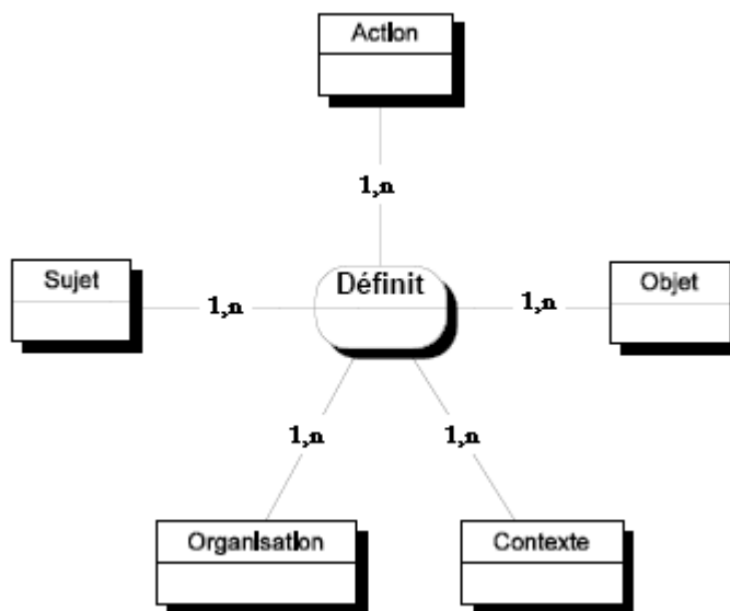
Figure 15 : La relation « Définit ».
