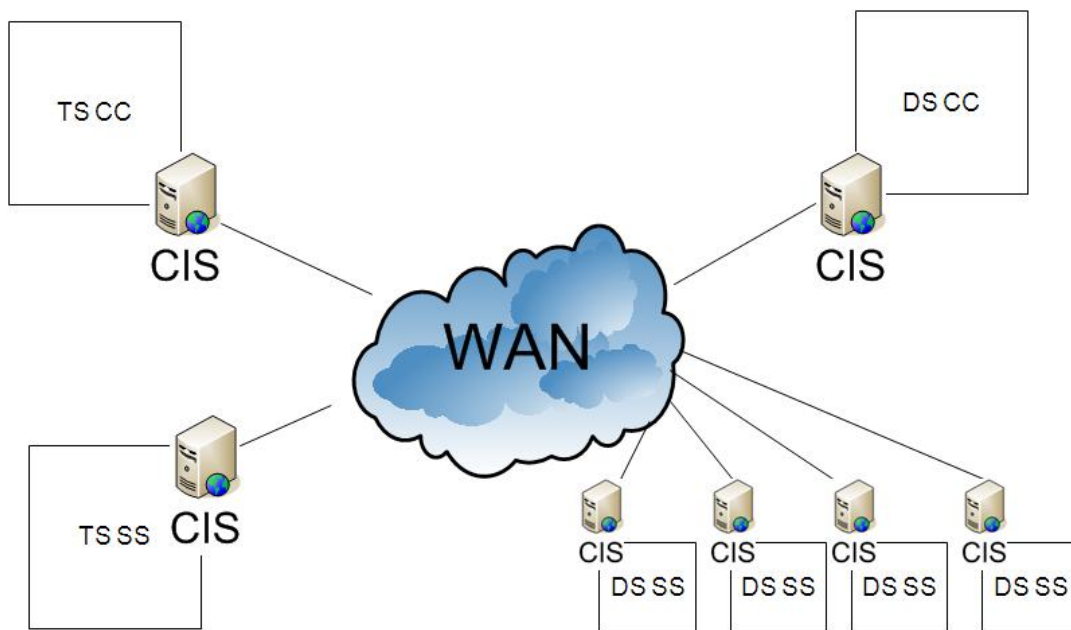
Figure 47 : Organisations et CIS au sein de l'IIC considérée.
