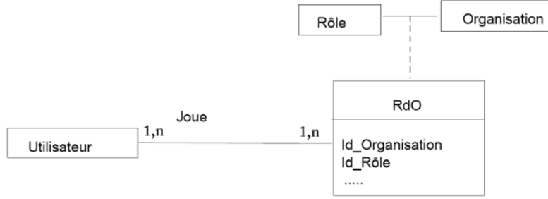
Figure 19 : Ébauche du diagramme de classe pour la classe-association RdO.
