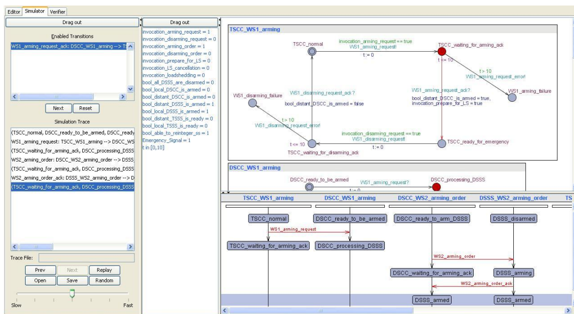
Figure 54 : Vérification statique des politiques-contrats grâce aux automates temporisés.
