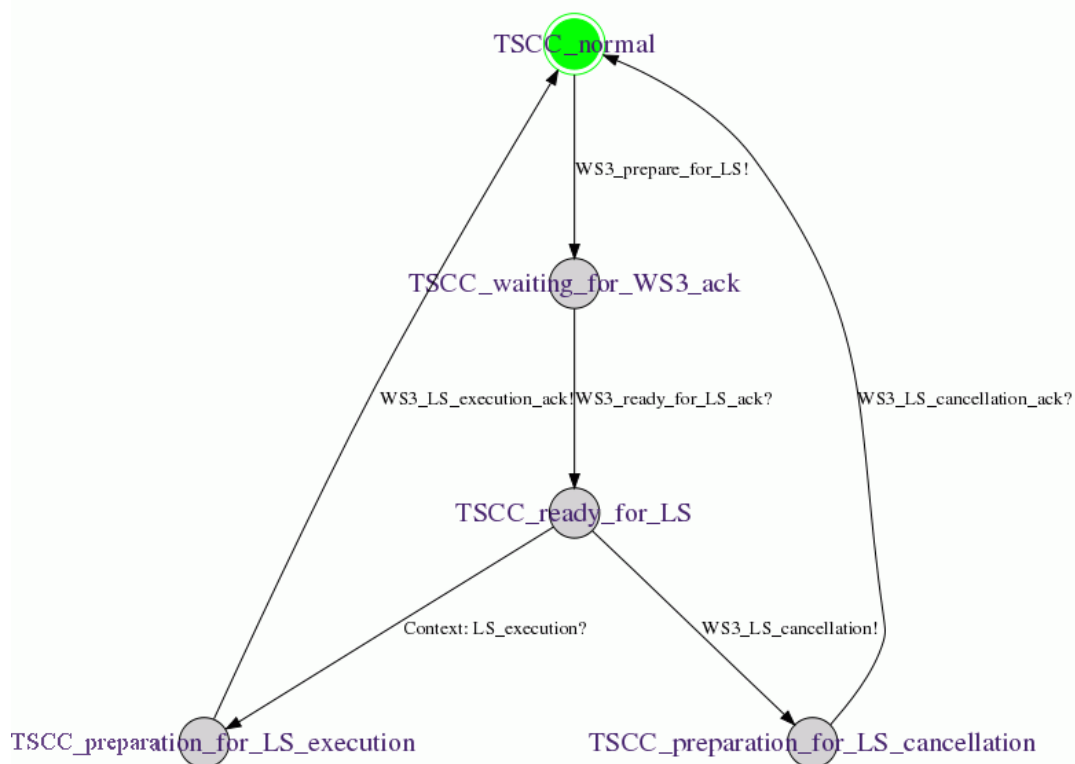
Figure 69 : Automate de SW3-préparation_de_déstage au niveau du TS CC.
