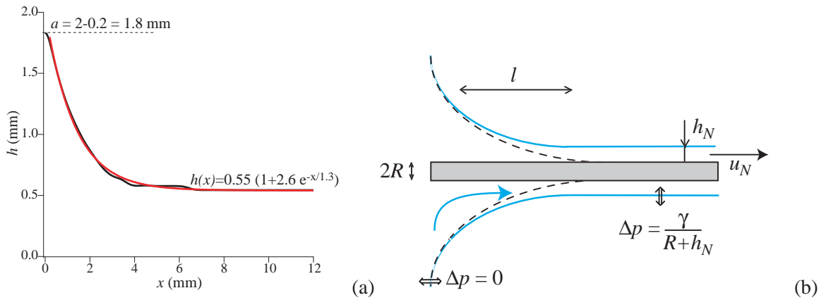
Fig. 2.11. Ménisque à la sortie de la vanne : (a) profil expérimental (en noir) et courbe d'ajustement (en rouge). (b) Notations, surpressions en différents points et mouvement du fluide. La courbe pointillée correspond au ménisque statique (obtenu en l'absence de mouvement).
