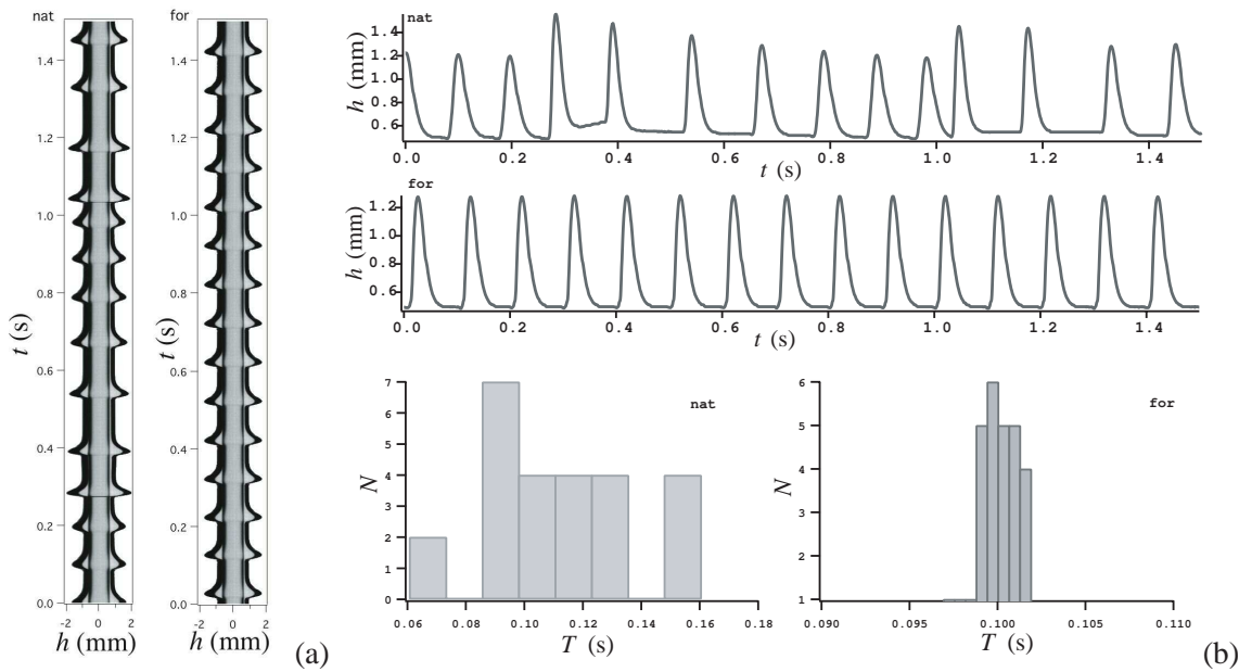
Fig. B.5. Resultats obtenus avec la caméra perpendiculaire à l'écoulement. (a) Images obtenues sans et avec forçage ; (b) signal h(t) et histogramme des périodes correspondants sans et avec forçage.
