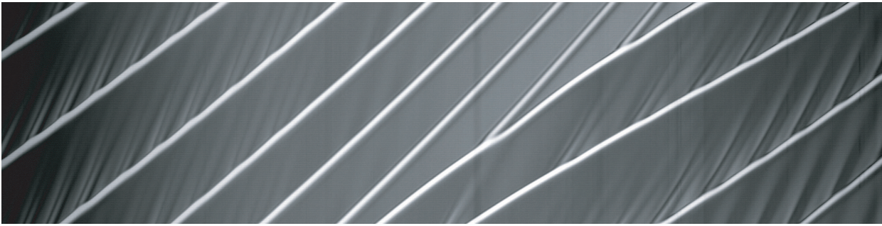
Fig. 4.33. Diagramme spatio-temporel (durée : 1s) en bas de la fibre ( 63\text{ cm} < x < 88\text{ cm} ) obtenu pour R=0.32\text{ mm} ( R/l_c=0.21 ) et h_N=0.48\text{ mm} ( \alpha_N=1.5 ). Présence d'oscillations régulières entre les gouttes ( \lambda \approx 5.8\text{ mm} \approx \lambda_{RP} \approx 5.4\text{ mm} ) alors que l'on est à fort débit et pas dans le mode goutte à goutte.
