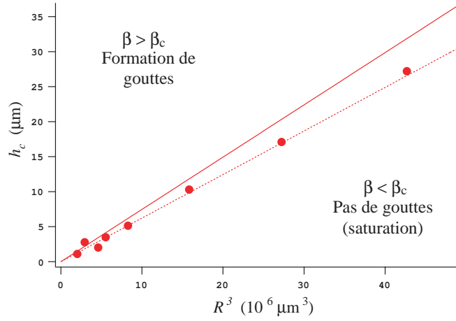
Fig. 3.17. Expérience de D. Quéré (81) du fil tiré hors d'un bain : épaisseur critique h_c en-deçà de laquelle l'instabilité sature. La transition est donnée par la loi (3.12) qui s'écrit aussi h_c = (a/l_c^2)R^3 . Points expérimentaux obtenus par D. Quéré (81), ligne pointillée : ajustement expérimental ( a=1.4 ) et ligne continue : loi obtenue par (46) ( a=1.68 ).
