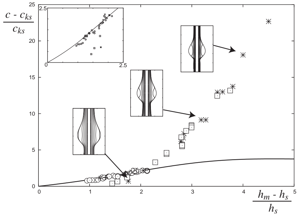
Fig. 6.2. Vitesse c normalisée par la vitesse à la surface du substrat (c - c_{ks})/c_{ks} en fonction de l'amplitude (h_m - h_s)/h_s : \circ R=0.475 mm, + R=0.45 mm, \times R=0.35 mm, \square R=0.25 mm, * R=0.2 mm. Profils et lignes de courant obtenus numériquement à partir du modèle WRIBL pour une fibre de rayon R=0.2 mm. Encart : zoom sur les faibles amplitudes.
