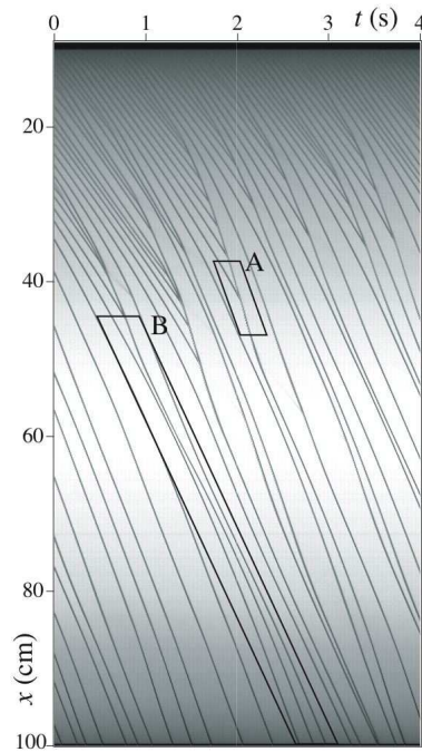
Fig. 5.1. Evolution naturelle le long de la fibre : diagramme spatio-temporel pour R=0.35 mm, h_N=0.85 mm. Interactions fortes : A coalescence, B répulsion.
