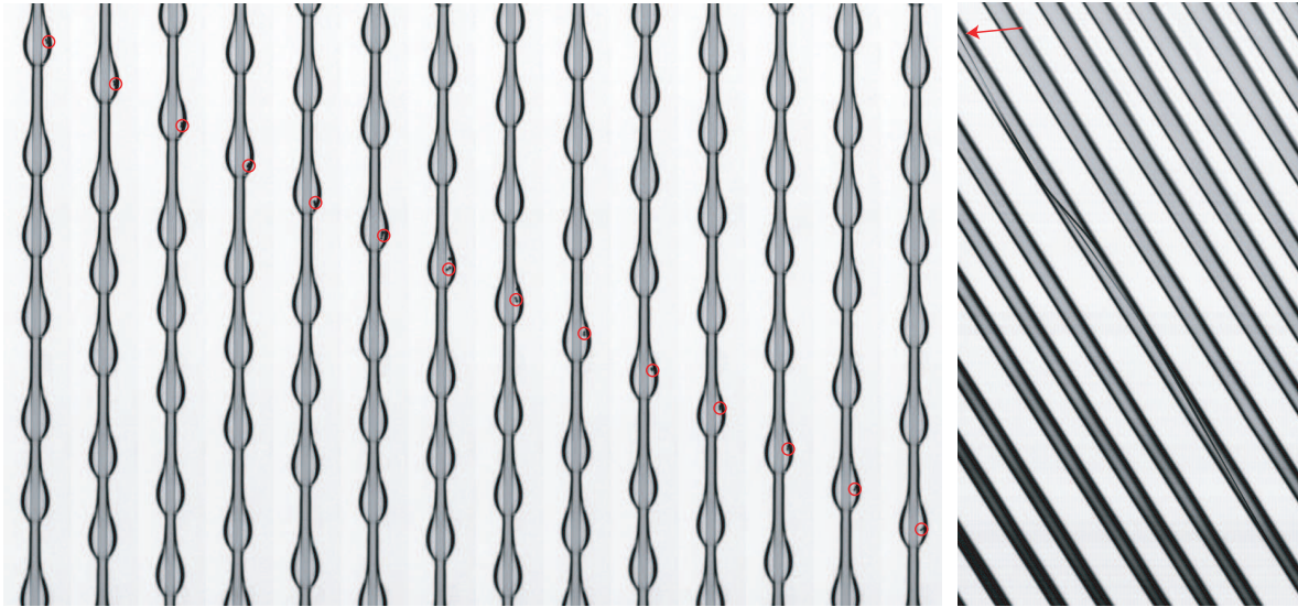
Fig. 4.35. Une goutte : succession d'images et diagramme spatio-temporel. Cette fois, les gouttes sont en gris et l'espace entre les gouttes (film très mince) est représenté en blanc. La flèche indique la particule que l'on suit.
