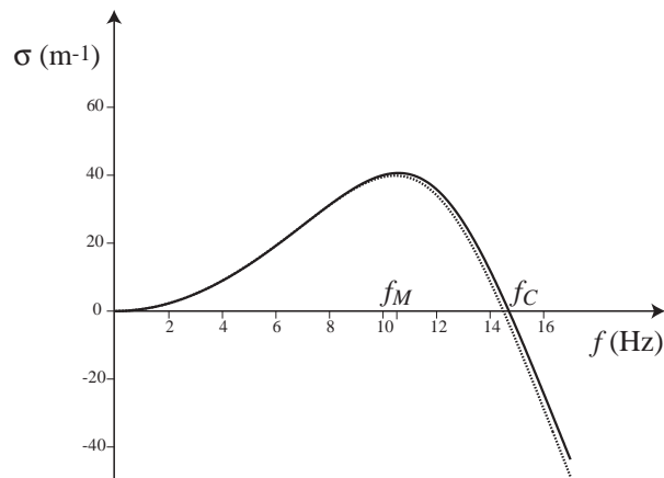
Fig. 4.5. Taux de croissance pour R=1.5 mm, h_N=0.87 mm ( Re=1.4 ). Ligne continue : solution des équations d'Orr-Sommerfeld. Ligne pointillée : solution du modèle WRIBL.
