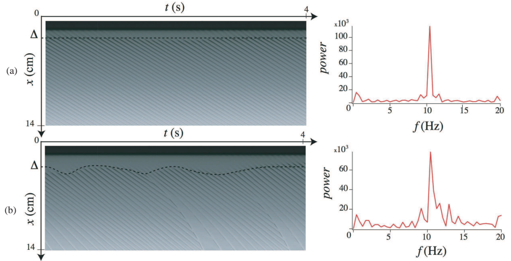
Fig. 3.2. Diagrammes spatiotemporels (à gauche) et spectres de la fréquence prise à l'apparition des ondes f(x = \Delta) correspondants (à droite) pour R = 0.32 mm, V50 , pour un régime régulier (a) et un régime irrégulier (b). (a) : Q = 0.067 g/s, h_N = 0.56 mm, \Delta = 1.83 \pm 0.03 cm, f = 10.4 \pm 0.8 Hz; (b) : Q = 0.090 g/s, h_N = 0.6 mm, \Delta = 2.07 \pm 0.23 cm, f = 10.8 \pm 2.5 Hz.
