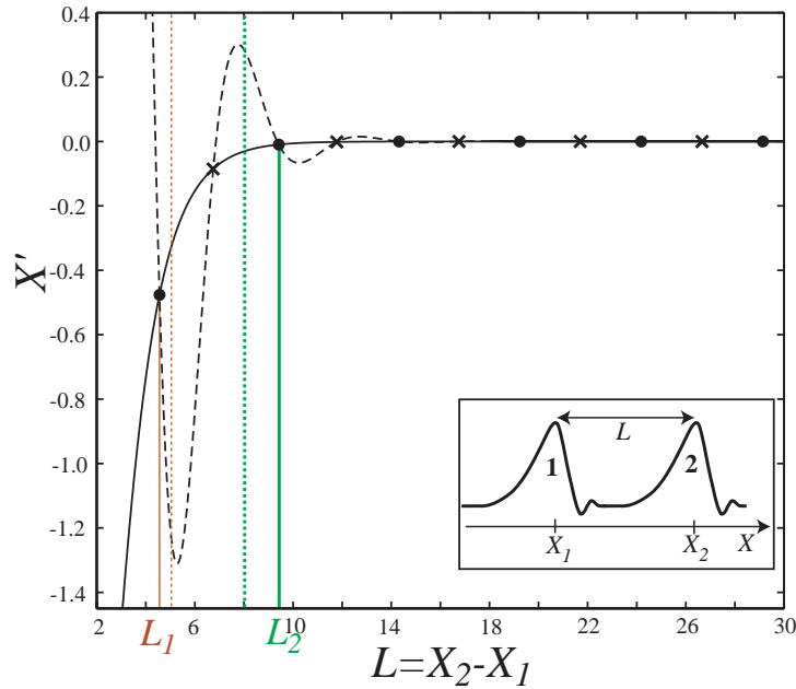
Fig. 5.14. Evolution de S_1 (ligne pleine) et S_2 (ligne pointillée) en fonction de la distance L entre deux pulses pour \delta_d = 0.4 . \bullet : état lié stable, \times : état lié instable. Les lignes pleines verticales indiquent les distances L_1 (rouge, fin) et L_2 (vert, épais) des deux premiers états liés. Les lignes verticales pointillées représentent les valeurs L_0 prises pour expliquer une attraction (rouge, fin) et une répulsion (vert, épais) (voir dans le texte ci-dessous).
