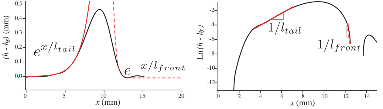
Fig. 4.21. Détermination expérimentale des longueurs de queue l_{tail} et de front l_{front} . Exemple donné sur la figure : R=0.475 mm, h_N=0.61 mm, f_{for}=5 Hz. On trouve l_{tail}=1.25 mm et l_{front}=0.33 mm.
