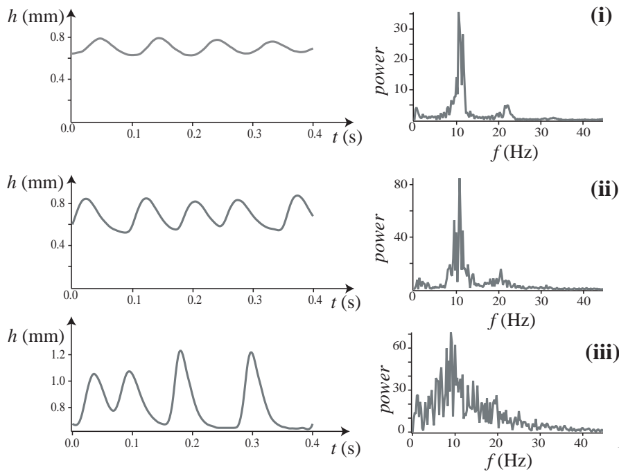
Fig. 4.4. Evolution de l'épaisseur pour R=1.5 mm, h_N=0.8 mm, sans forçage, à (i) x = 8 cm, (ii) x = 30 cm et (iii) x = 45 cm ; spectres temporels correspondants.
