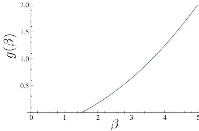
Fig. 3.16. Evolution de la partie imaginaire de \omega_0 en fonction du paramètre \beta .
