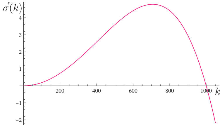
Fig. 3.11. Taux de croissance pour R = 0.5 \text{ mm} , h_N = R , huile V50 ( \eta = 48 \text{ mPa.s} , \gamma = 20.8 \text{ mN/m} , \rho = 963 \text{ kg/m}^3 ).
