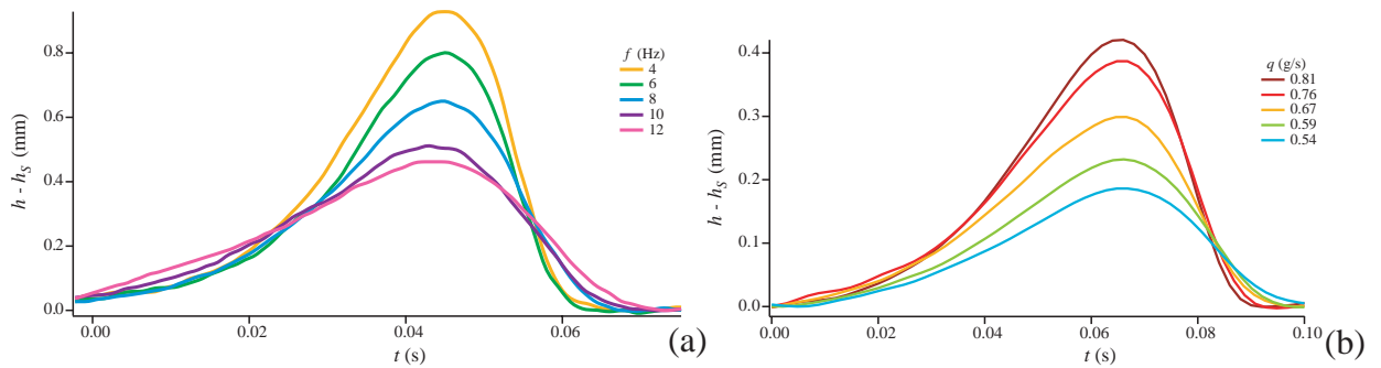
Fig. 4.15. Profils expérimentaux (en temps) pour R=1.5 mm, (a) h_N=0.87 mm et différentes fréquences ; (b) f=10 Hz et différents débits.
