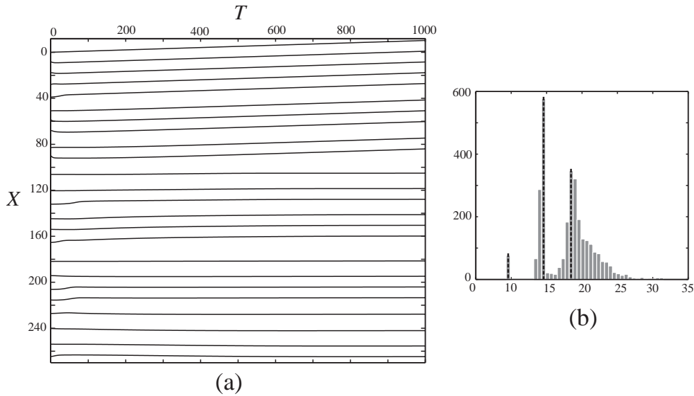
Fig. 5.15. (a) Diagramme spatio-temporel obtenu numériquement en résolvant le système (5.7) pour \delta_d = 0.4 , dans le référentiel en mouvement à la vitesse c_\delta . (b) Histogramme des distances entre pulses obtenu en faisant des statistiques sur 3000 pulses à t=1000 . La distribution initiale des distances a été prise gaussienne, de moyenne 18 et de largeur 3.
