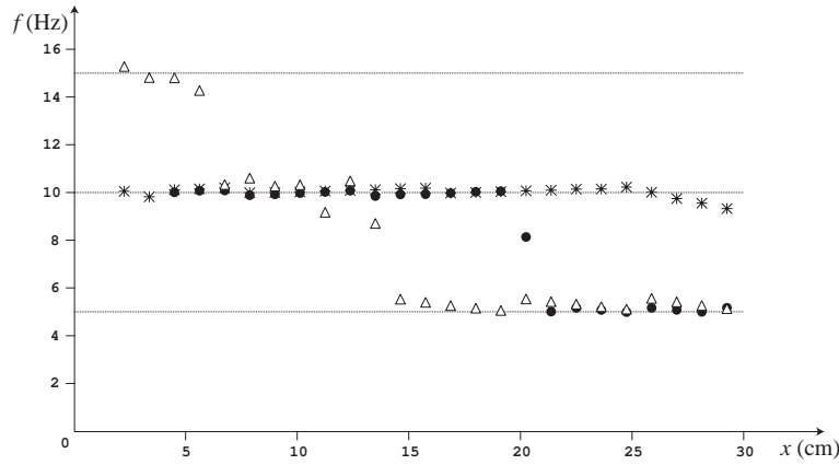
Fig. 4.8. Evolution de la fréquence en fonction de la position x sur la fibre pour R = 1.5 mm ( R/l_c = 1 ) et : (*) h_N = 0.87 mm ( \alpha_N = 0.58 ) et f_{for} = 10 Hz; (●) h_N = 0.87 mm ( \alpha_N = 0.58 ) et f_{for} = 5 Hz; ( \Delta ) h_N = 1.14 mm ( \alpha_N = 0.76 ) et f_{for} = 5 Hz. Ces trois situations correspondent aux cas présentés sur la figure 4.7(a),(b),(c) respectivement.
