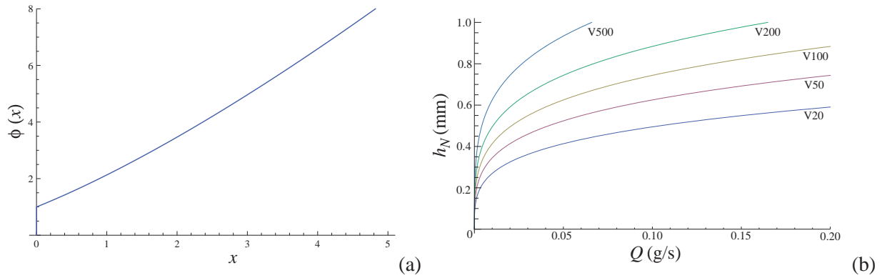
Fig. 2.8. (a) Evolution de la fonction géométrique \phi(x) et (b) évolution de h_N en fonction du débit calculée à partir de la relation (2.4) pour R=0.2 mm et différentes viscosités.
