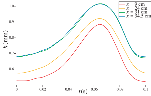
Fig. 4.12. Profils expérimentaux pour R=1.5 mm, h_N=0.87 mm et f_{for}=10 Hz à différentes altitudes le long de la fibre.
