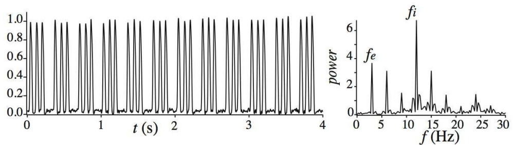
(d): Signal temporel en sortie de l'écoulement ( x=50 cm) extrait du diagramme spatio-temporel. Amplitude normalisée h/h_m et spectre correspondant.
