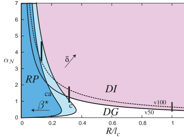
Fig. 4.1. Carte des régimes. Les segments verticaux correspondent aux gammes de paramètres principalement explorées dans cette section. Dans la zone bleue notée RP et délimitée par la frontière (c) \beta^* = 1 , l'instabilité de Rayleigh-Plateau domine. La zone bleue foncée, délimitée par la frontière (ca) \beta^* = 1.507 , correspond à la région où l'instabilité est absolue. Dans la zone rose notée DI et délimitée par les frontières V50/V100 \delta = 1 , l'inertie domine. La zone blanche notée DG correspond à la région où l'écoulement domine.
