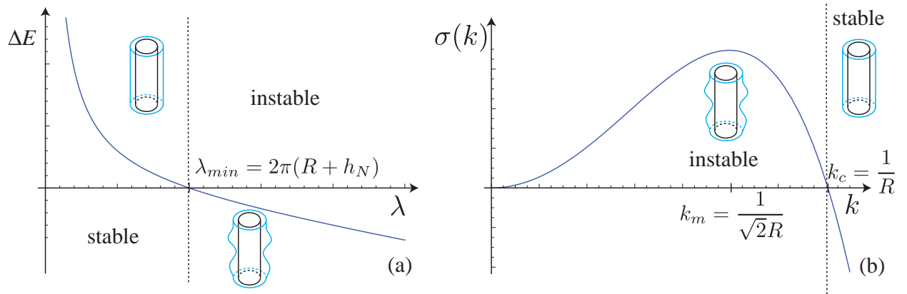
Fig. 2.20. Stabilité d'un film liquide sur une fibre sans effet de la gravité : (a) Evolution de la différence d'énergie \Delta E entre un cylindre liquide non déformé et un cylindre liquide ondulé en fonction de la longueur d'onde \lambda . La ligne pointillée verticale indique la transition entre la région stable dans laquelle le film liquide reste plat ( \Delta E > 0 , déformer l'interface est coûteux en énergie) et instable dans laquelle le film se déstabilise ( \Delta E < 0 , il est plus favorable de déformer le cylindre) ; (b) Evolution du taux de croissance \sigma en fonction du nombre d'onde k . La ligne pointillée verticale indique la transition entre la région instable ( \sigma > 0 , les perturbations de l'interface sont amplifiées) et la région stable ( \sigma < 0 , les perturbations de l'interface sont amorties).
