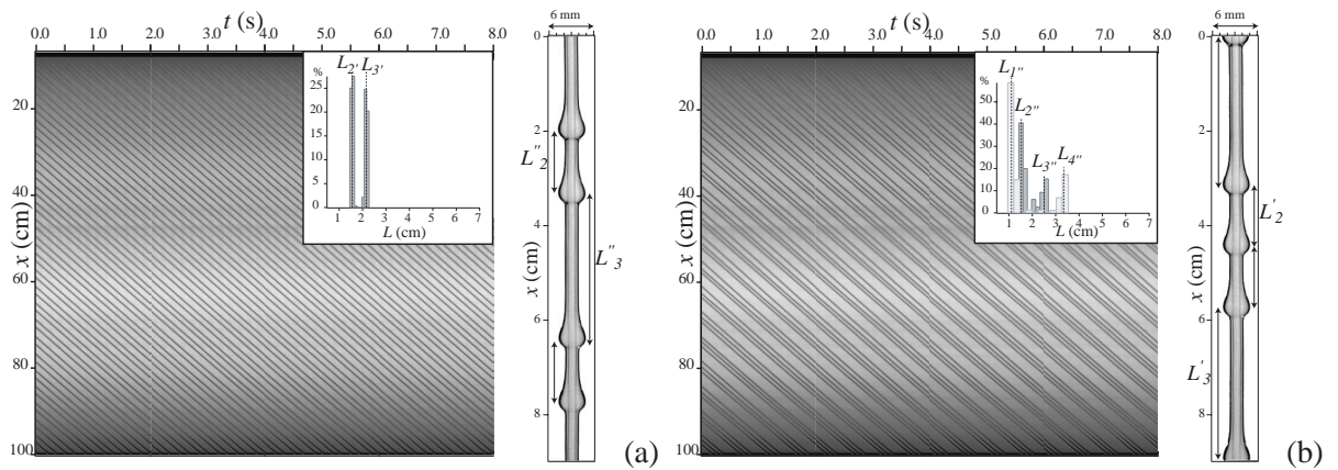
Fig. 5.10. Etats liés forcés : photos de l'écoulement à x \sim 90 cm, diagramme spatio-temporel et histogrammes des distances entre pulses (par rapport au nombre total de pulses) en bas de la fibre 1.20 \text{ m} < x < 1.40 \text{ m} , pour R=0.45 \text{ mm} , We=18 , Re=0.56 et différents signaux en entrée : (a) état lié 2-pulses et (b) état lié 3-pulses.
