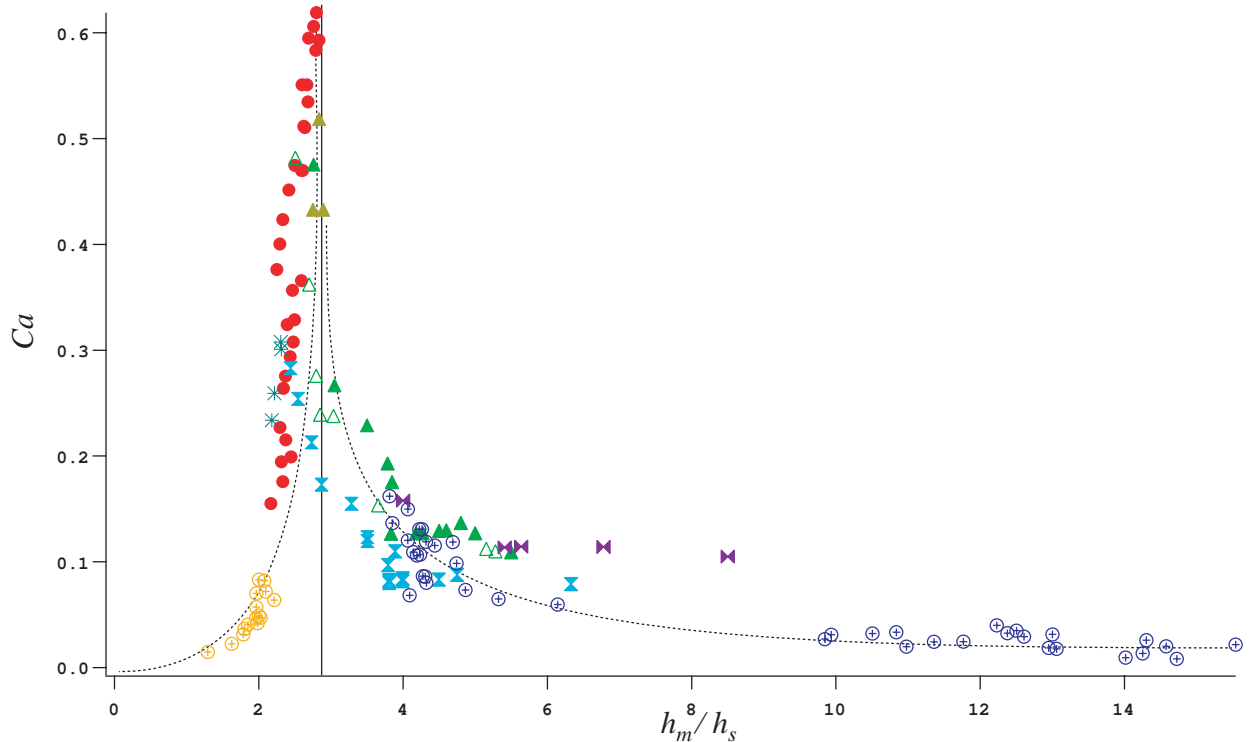
Fig. 6.19. Nombre capillaire Ca en fonction de l'amplitude h_m/h_s pour R=0.475 mm, V50 ( \bullet ), R=0.2 mm, V100 ( \blacktriangle ), R=0.2 mm, V500 ( \triangle ), R=0.25 mm, V100 ( \blacktriangledown ), R=0.175 mm, V100 ( \blacktriangleright ), R=0.45 mm, V50 ( * ), R=0.35 mm, V50 ( \blacktriangle ); R=0.45 mm, V500 ( \oplus ), R=0.2 mm, V500 ( \oplus ). Les lignes pointillées sont là pour guider l'œil et symbolisent les deux tendances observées; la ligne en trait plein verticale indique l'amplitude à laquelle ces deux tendances se rejoignent.
