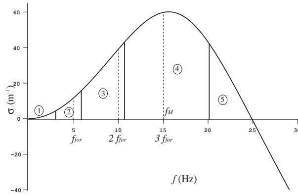
Fig. 4.11. Taux de croissance pour h_N=1.14 mm, \alpha_N = 0.76 , R/l_c = 1 . Les lignes pointillées représentent l'expérience de la figure 4.7(c).
