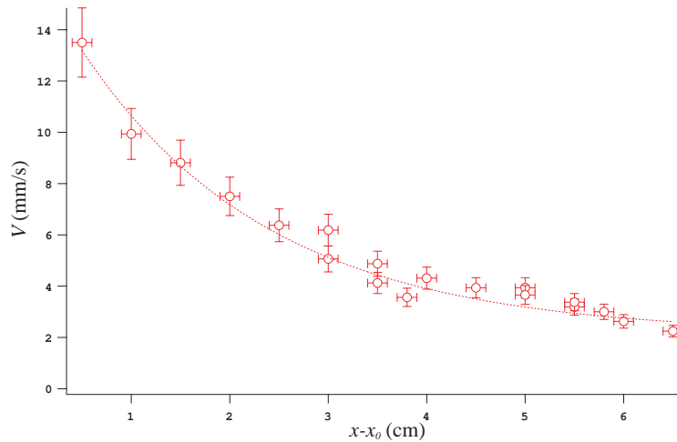
Fig. 6.7. Vitesse d'une goutte d'huile V100 de volume \Omega=9 \text{ mm}^3 glissant sur une fibre sèche de rayon R=0.2 \text{ mm} en fonction de sa position x - x_0 .
