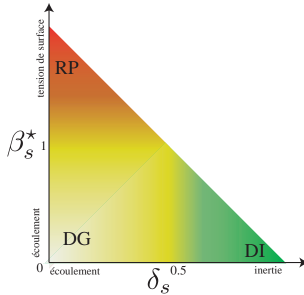
Fig. 4.24. Diagramme de phase des différents régimes dans le plan (\beta_s^*, \delta_s) . En augmentant \beta_s^* , on passe d'un régime dominé par l'écoulement (DG, en jaune) à un régime dominé par la tension de surface (RP, en rouge). En augmentant \delta_s , on passe du régime DG à un régime où l'inertie domine (DI, en vert).
