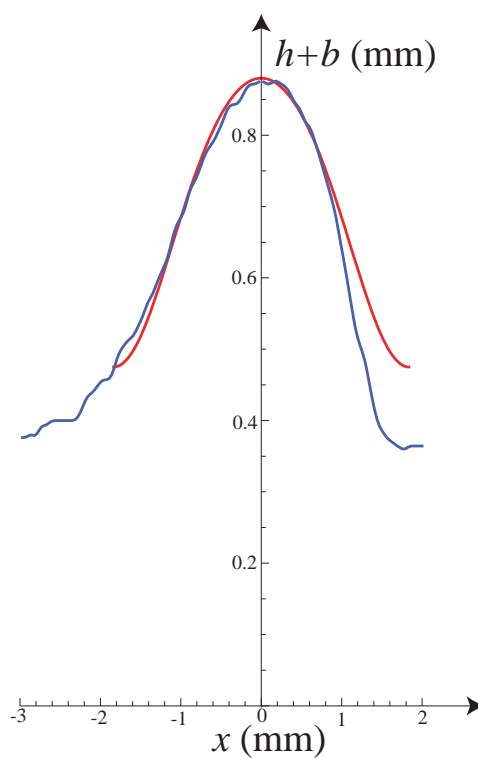
Fig. 3.27. Comparaison entre le profil d'une goutte sur une fibre horizontale calculé sans gravité (rouge) et profil expérimental (bleu) sur une fibre de rayon R=0.2 mm pour une goutte en mode global stable.
