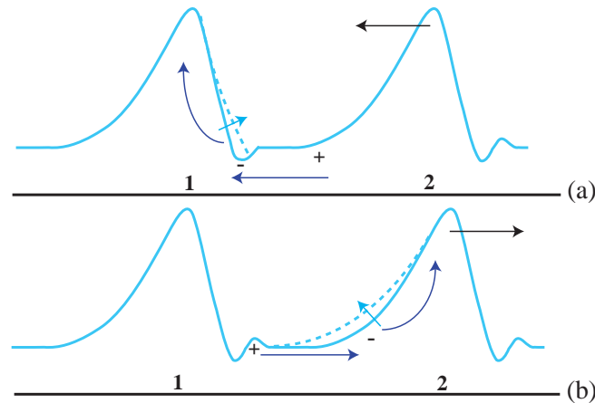
Fig. 5.7. (a) : Attraction de deux ondes ; (b) : Répulsion de deux ondes. Les mouvements relatifs des ondes (flèches noires) sont donnés dans le référentiel en mouvement de l'onde 1.
