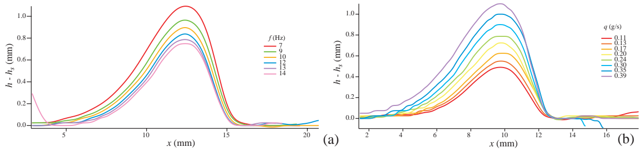
Fig. 4.14. Profils expérimentaux (en espace) pour R=0.475 mm, (a) h_N=0.87 mm et différentes fréquences ; (b) f=7 Hz et différents débits.
