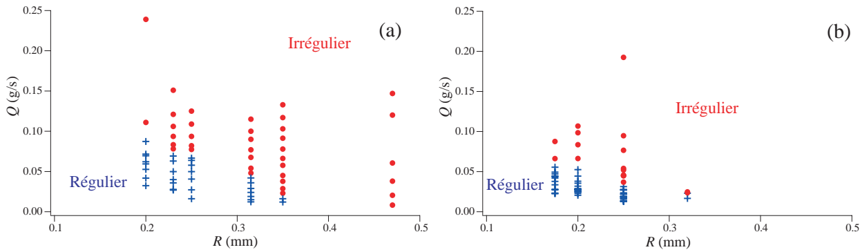
Fig. 3.5. Débits réguliers (croix bleues) et irréguliers (ronds rouges) pour différents rayons de fibre et de l'huile V50 (a) et V100 (b).
