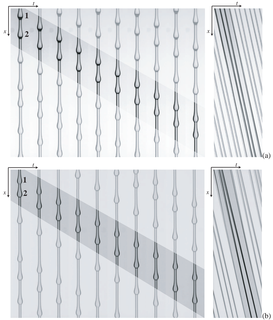
Fig. 5.6. (a) Attraction : R = 0.35 \text{ mm} , h_N = 0.85 \text{ mm} , V50 (hauteur sur la fibre : 9 cm) et (b) repulsion : R = 0.35 \text{ mm} , h_N = 0.92 \text{ mm} , V50 (hauteur sur la fibre : 7 cm). Chronophotographie réalisée en prenant une image toutes les 0.08 s. Diagramme spatio-temporel correspondant.
