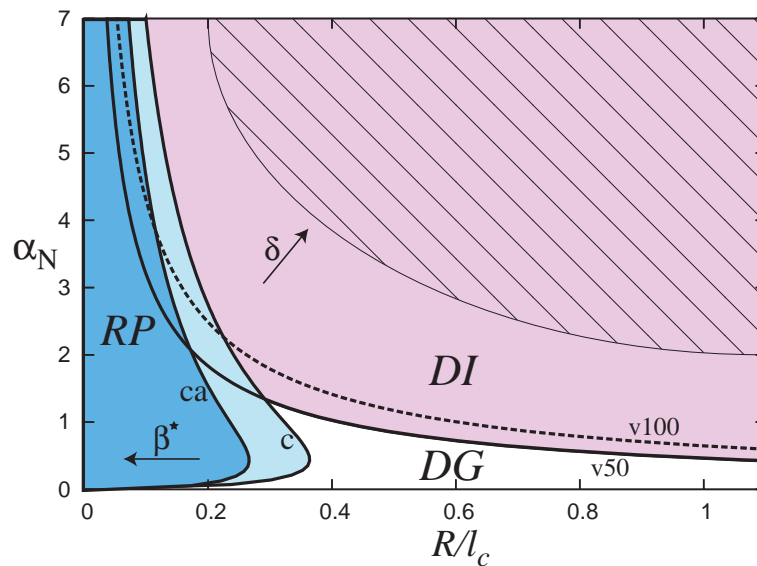
Fig. 3.32. Carte des régimes dans le plan (\alpha_N, R/l_c) pour les huiles V50 et V100. Les courbes correspondent à \beta^* = 1 (c), \beta^* = \beta_{ca}^* = 1.507 (ca) et \delta = 1 (labels v50 et v100). La partie hachurée correspond aux épaisseurs importantes que l'on ne peut pas atteindre expérimentalement, et est donnée par R + h_N \simeq l_c . Les différentes régions sont précisées dans le texte.
