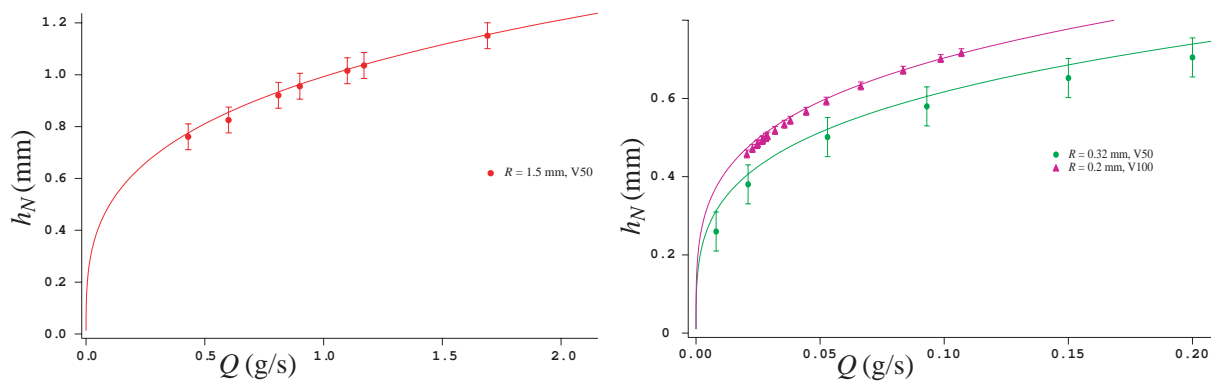
Fig. 2.9. Mesures de l'épaisseur initiale h_N en fonction du débit : résultats expérimentaux (points) et calcul à partir de la relation (2.4) (trait plein).
