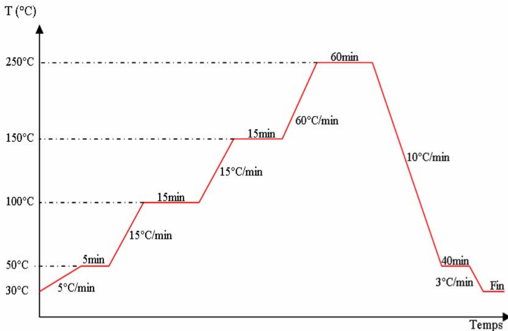
Figure 40. Cycle thermique du recuit de durcissement du BCB
