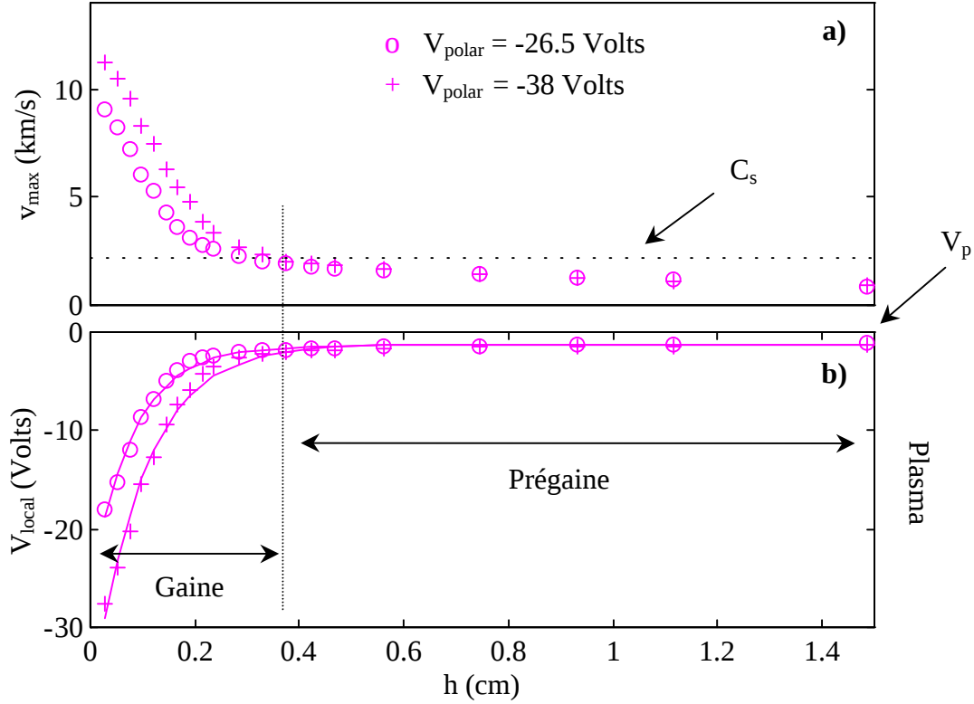
Figure III.14 : a) Vitesse des ions b) Profils de potentiel
