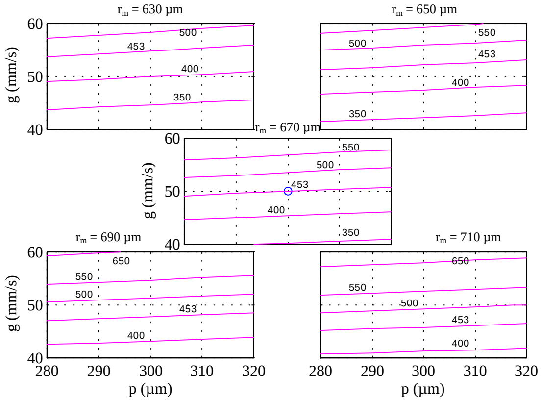
Figure IV.6 : Evolution de \lambda_S en fonction de r_m , p , q
