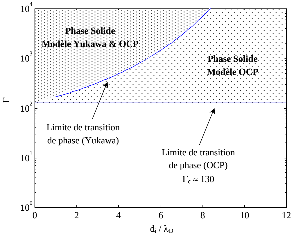
Figure V.12 : Diagramme de transition de phase pour le modèle OCP et Yukawa
