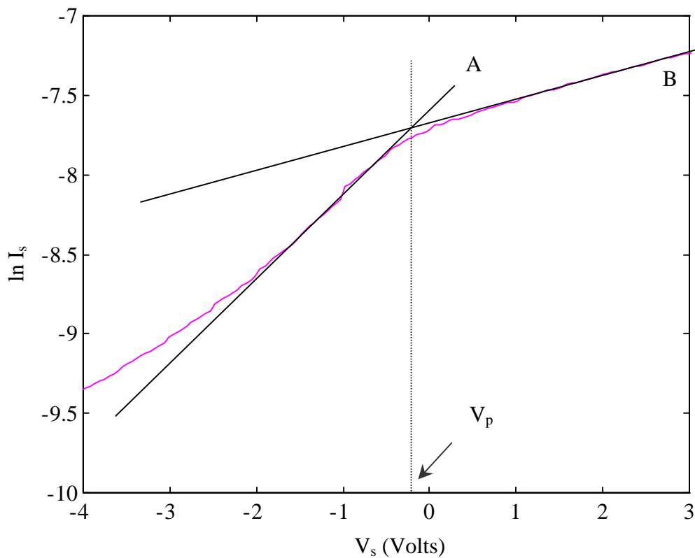
Figure II.8 : Détermination graphique du potentiel plasma
