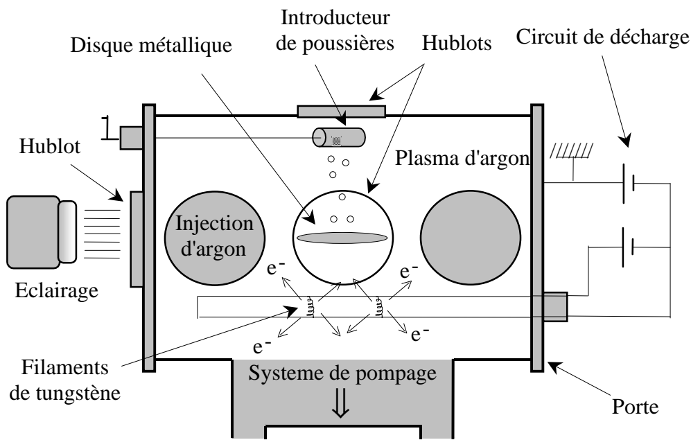
Figure II.1 : Dispositif expérimental
