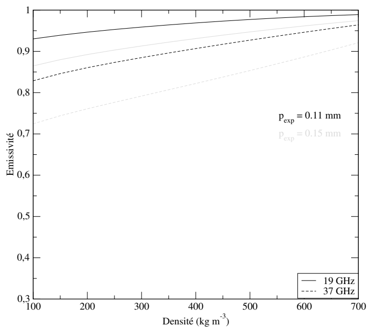
(a) MEMLS
