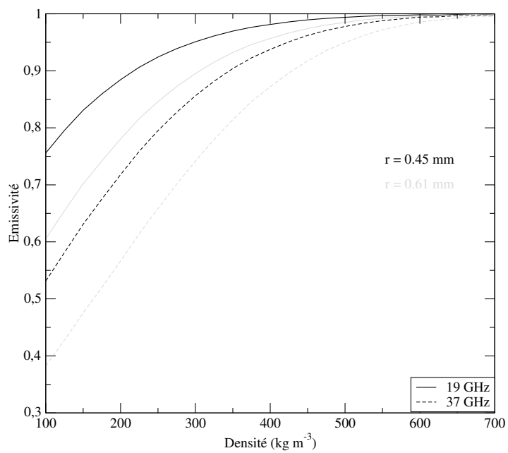
(b) DMRT-ML
