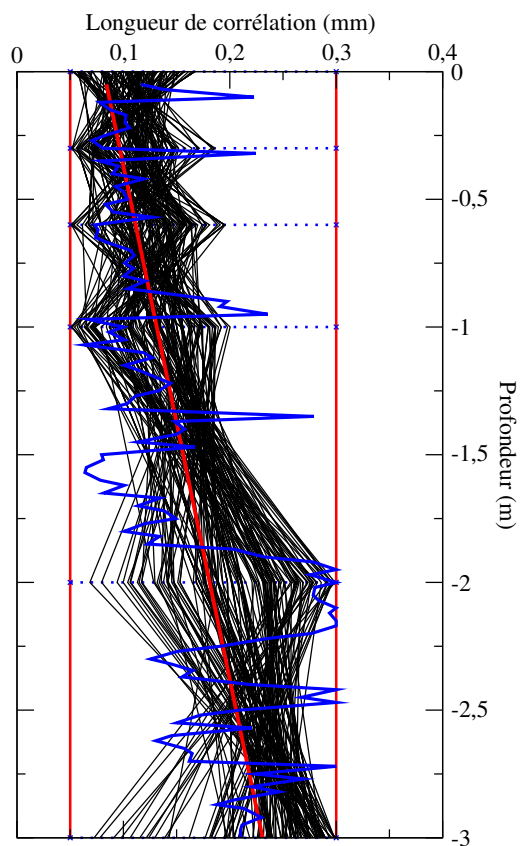
FIG. 4.14 – Evolution de la taille des grains estimée par la méthode de Monte Carlo sur les trois premiers mètres, ainsi que l'évolution du profil de taille de grains dérivée de la mesure de réflectance IR (profil bleu). La régression linéaire de ce dernier profil est présentée en rouge.
