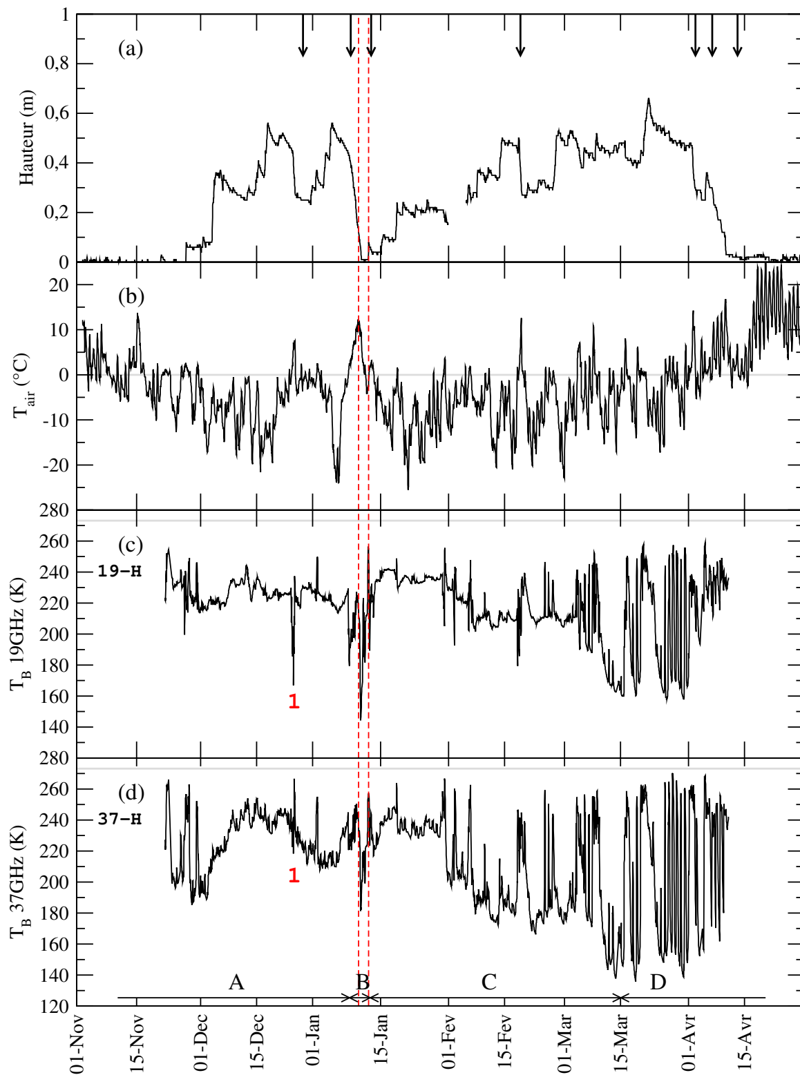
FIG. 8.5 – Evolutions temporelles de la hauteur de neige mesurée par la sonde à ultra-sons (a), de la température de l'air (b) et des températures de brillance mesurées par le radiomètre au sol à 19 GHz (c) et 37 GHz (d) en polarisation horizontale .
