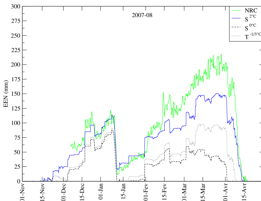
FIG. 7.9 – Evolution de l'EEN (en mm) mesurée par le NRC (trait vert) et modélisée par Crocus pour trois paramétrisations de la phase des précipitations, S^{2^\circ C} (trait continu bleu), S^{0^\circ C} (trait interrompu) et T^{-1/3^\circ C} (trait pointillé).
