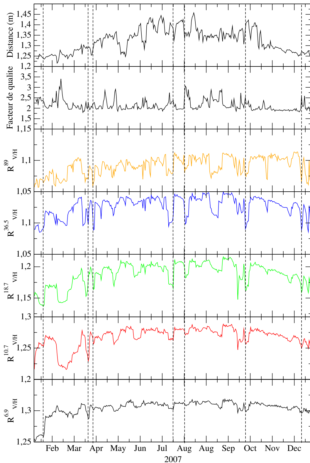
FIG. 6.14 – Evolution temporelle en 2007 de la distance capteur-surface et du facteur de qualité mesurés par un capteur à ultra-sons à Dôme C (les deux panneaux du haut). Les panneaux suivant correspondent au rapport de températures de brillance.
