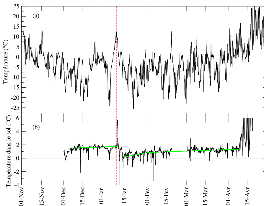
FIG. 8.3 – Evolutions de la température de l'air mesurée à 2 m (a) et de la température mesurée à 4 cm dans le sol (b).
