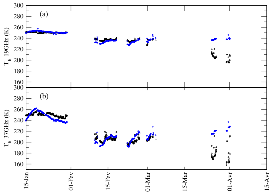
FIG. 8.15 – Evolution des températures de brillances observées (noir) et modélisées (bleu) à 19 GHz (a) et 37 GHz (b), en polarisation verticale sur les périodes de la phase C où le manteau neigeux est dans sa majorité sec.
