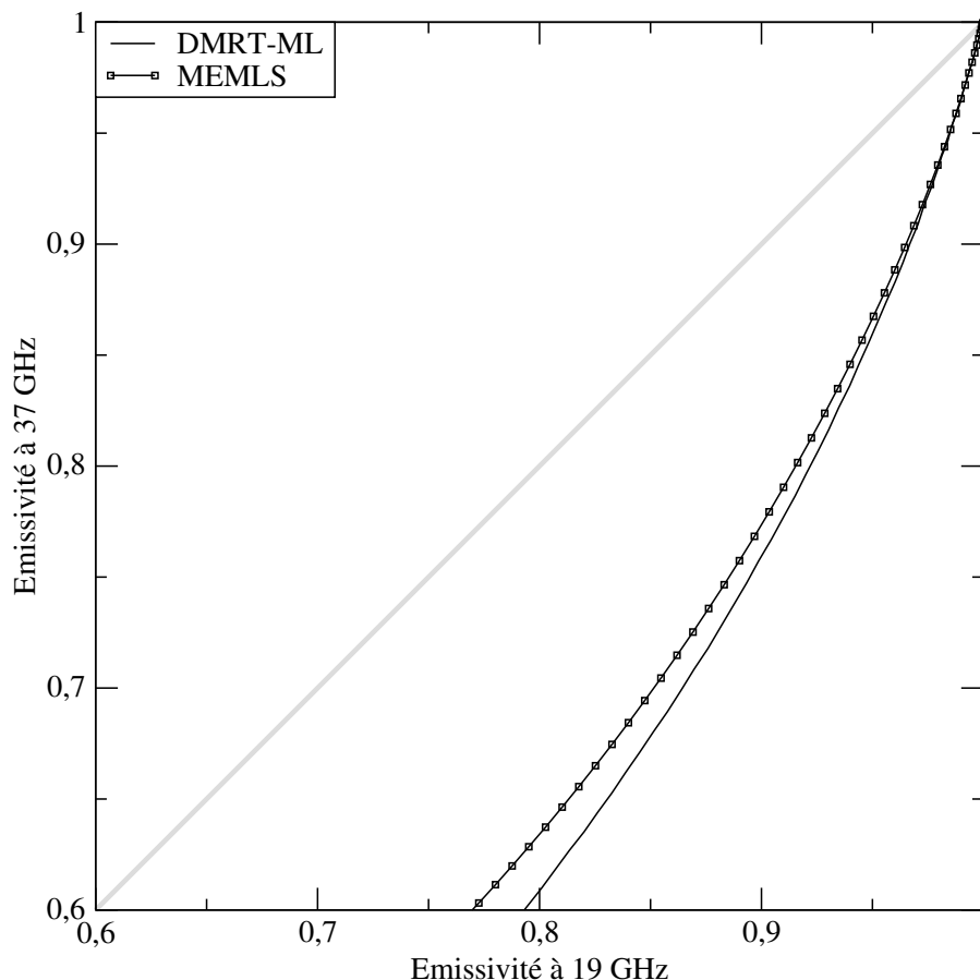
FIG. 3.9 – Evolution des émissivités en polarisation verticale à 37 GHz en fonction de celle à 19 GHz pour différentes tailles de grains. Lorsque la taille de grains est petite, les émissivités sont élevées aux deux fréquences. Lorsque la taille de grains augmente, les émissivités diminuent (Figure 3.8).
