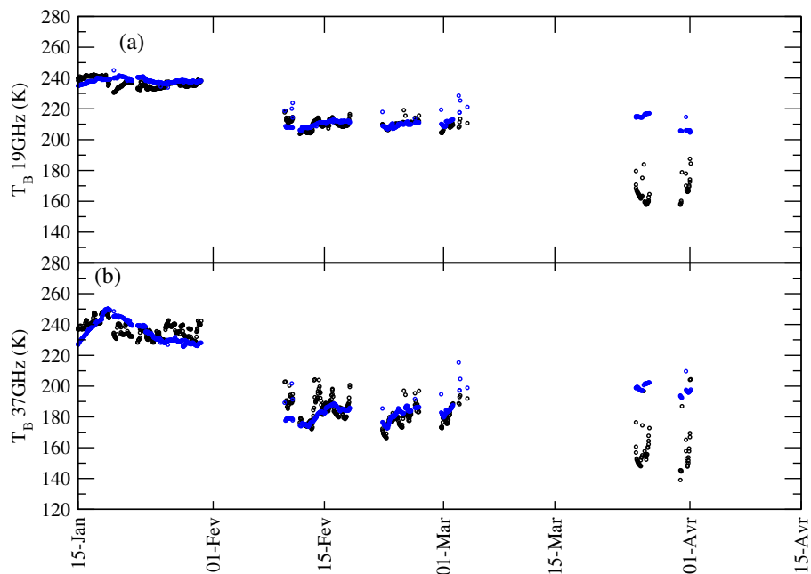
FIG. 8.16 – Evolution des températures de brillances observées (noir) et modélisées (bleu) à 19 GHz (a) et 37 GHz (b), en polarisation horizontale sur les périodes de la phase C où le manteau neigeux est dans sa majorité sec.
