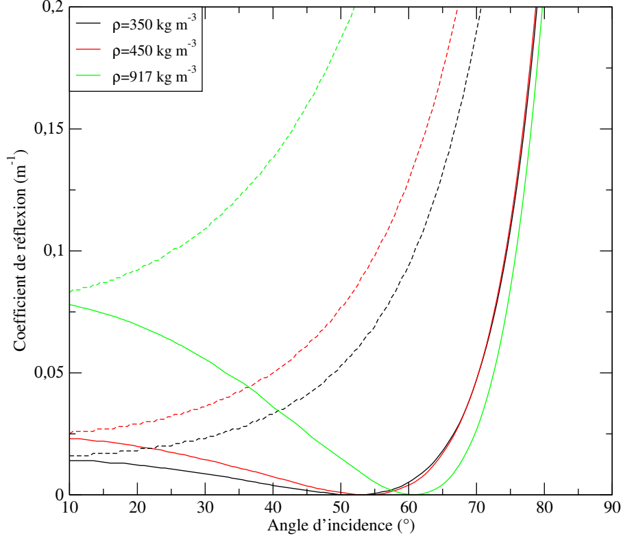
FIG. 3.2 – Evolution des coefficients de réflexion de l'onde polarisée horizontalement (courbe pointillée) et verticalement (courbe continue) en fonction de l'angle d'incidence pour différentes densités (350, 450 et 917 kg m -3 ).
