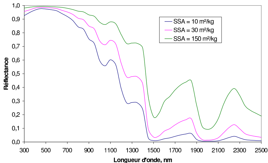
FIG. 2.7 – Réflectance de la neige dans le domaine spectral 300-2500 nm pour trois valeurs de SSA, 150, 30 et 10 \text{ m}^2 \text{ kg}^{-1} (de haut en bas). Evolutions modélisées par J.-C. Gallet (LGGE) avec le modèle DISORT.
