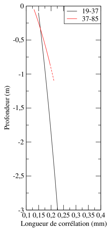
FIG. 5.11 – Profil de longueur de corrélation déduit du spectre d'émissivité à 19,3 et 37 GHz (noir) et du spectre d'émissivité à 37 et 85,5 GHz (rouge).
