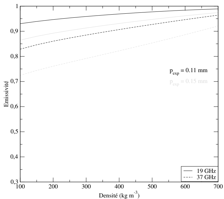
(a) MEMLS
