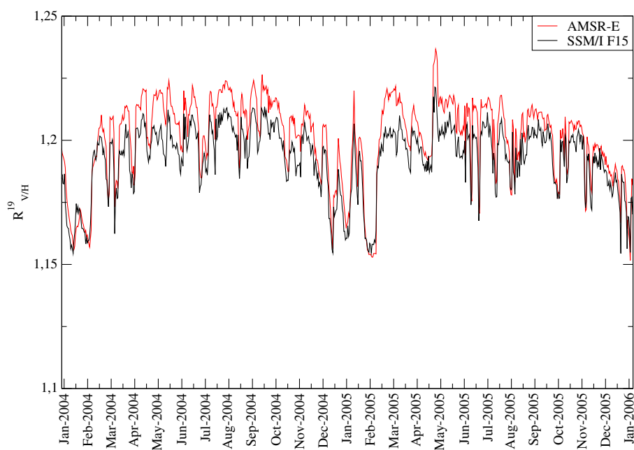
FIG. 6.12 – Evolutions temporelles, à Dôme C entre 2004 et 2006, du rapport entre les températures de brillance polarisées verticalement et horizontalement, à 19,3 et 18,7 GHz, mesurées respectivement par SSM/I F15 (noir) et AMSR-E (rouge).
