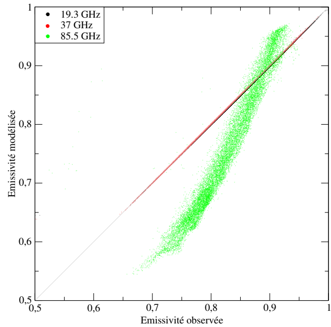
FIG. 5.10 – Graphique des émissivités modélisées, à partir du profil de taille de grains déduit de l'inversion du spectre d'émissivité à 19,3 et 37 GHz, en fonction de celles observées, à 19,3 (noir), 37 (rouge) et 85,5 GHz (vert).
