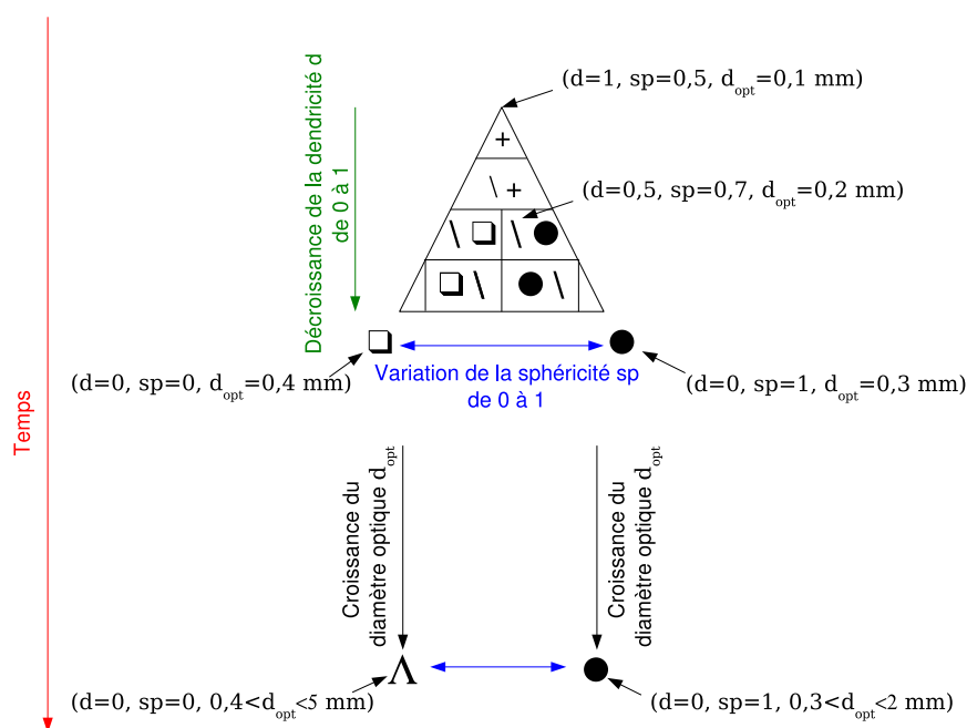
FIG. 2.9 – Evolution des variables de la taille de grains de Crocus, dendricité/sphéricité et sphéricité/taille, au cours de la métamorphose. d , sp et d_{opt} symbolise respectivement la dendricité, la sphéricité et le diamètre optique. Les symboles permettent le lien entre les variables descriptives continues de Crocus et la classification des grains de neige de Colbeck et al. (1993). Cette figure a été adaptée de la figure 1 de Brun et al. (1992).
