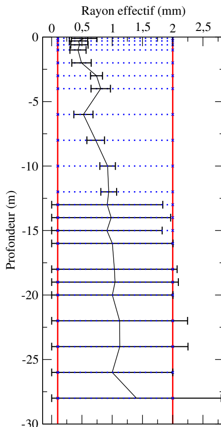
FIG. 4.16 – Evolution de la taille de grains moyenne avec la profondeur. Les barres d’incertitude représentent l’écart-type des 295 profils moyennés. La gamme de taille de grains possible lors de l’estimation avec DREAM est représentée par les lignes verticales rouges. Les lignes horizontales en pointillé bleues représentent la répartition des profondeurs auxquelles sont tirées aléatoirement les tailles de grains.
