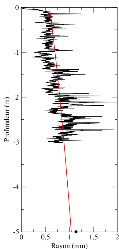
FIG. 5.9 – Profil du rayon effectif déduit des photographies IR prises à Dôme C jusqu'à 3 m de profondeur (courbe noire), et utilisé pour modéliser les températures de brillance avec DMRT-ML dans le Chapitre 4. Le point noir à 5 m correspond à la taille de grains en dessous de 3 m de profondeur estimée lors du test de sensibilité (Chapitre 4). Le profil déduit de l'inversion du spectre d'émissivité à 19,3 et 37 GHz correspond à la droite rouge.
