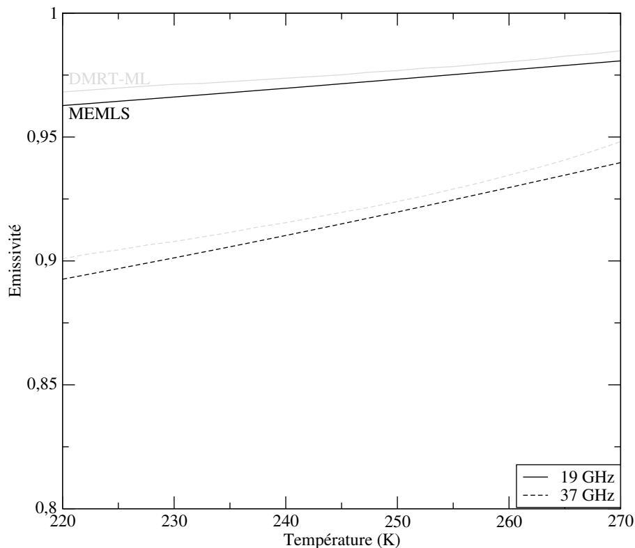
FIG. 3.11 – Evolution des émissivités en polarisation verticale à 19 GHz (trait continu) et 37 GHz (trait interrompu) modélisées avec MEMLS (noir) et DMRT-ML (gris) en fonction de la température. La densité du manteau est de 350 \text{ kg m}^{-3} , le rayon de DMRT-ML égal 0,45 \text{ mm} et la longueur de corrélation exponentielle vaut 0,11 \text{ mm} .
