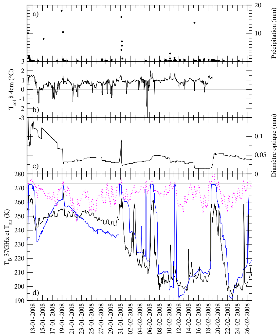
FIG. 8.14 – Evolutions, entre le 12 janvier et le 26 février 2008, de la hauteur d'eau précipitée (a), de la température à 4 cm dans le sol (b), du diamètre optique moyen des grains modélisé par Crocus (c), des températures de l'air (trait pointillé) et des températures de brillance mesurées (noir) et modélisées (bleu) (d).
