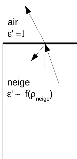
FIG. 6.2 – Représentation d'un manteau dont la densité est constante et où la seule interface, discontinuité de constante diélectrique \epsilon , est avec l'atmosphère. \epsilon' est la partie réelle de la constante diélectrique.
