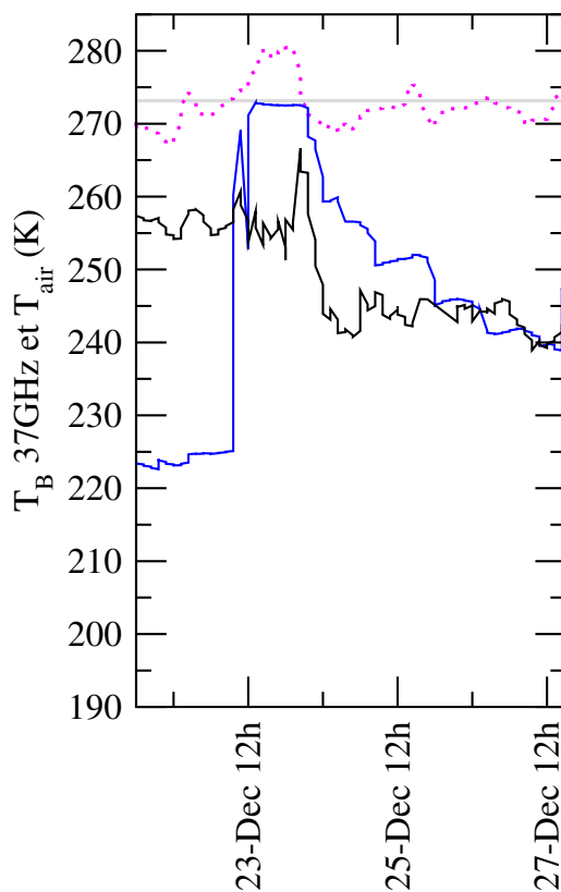
FIG. 8.11 – Evolution des températures de brillance observées (trait noir) et modélisées avec Crocus-MEMLS (trait bleu) en polarisation verticale à 37 GHz et de la température de l'air (trait pointillé).
