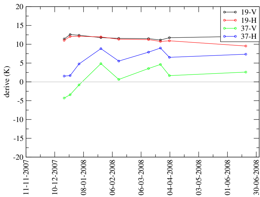
FIG. H1 – Evolutions temporelles des dérives du radiomètre pour les quatre canaux.
