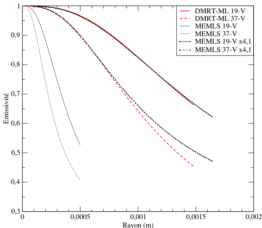
FIG. 3.8 – Evolution de l'émissivité d'un manteau neigeux homogène en fonction de la taille des grains, modélisée avec MEMLS (courbes noires) et DMRT-ML (courbes rouges). La conversion longueur de corrélation - rayon optique avec \beta=0,75 rapporte des rayons optiques sous estimant beaucoup l'émissivité (courbes noires sans symbole) par rapport à DMRT-ML. En multipliant le rayon optique ainsi calculé par 4,1, des émissivités assez similaires sont modélisées avec MEMLS (courbes noires avec symboles) et DMRT-ML (courbes rouges).
