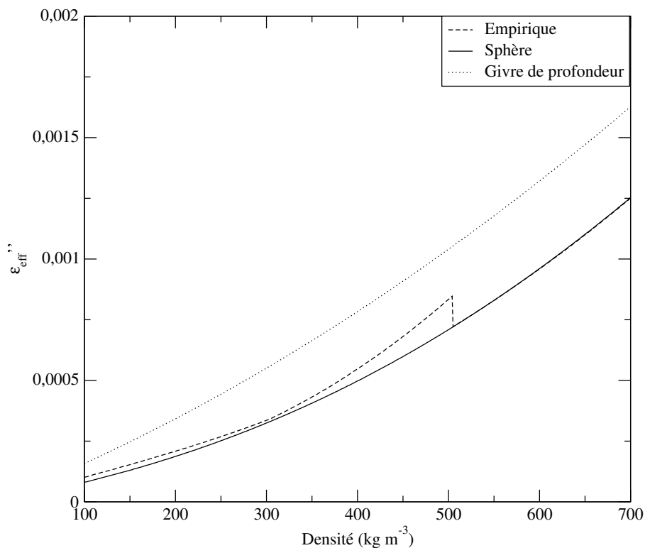
FIG. 3.6 – Evolution de la partie imaginaire de la constante diélectrique effective de la neige modélisée par MEMLS suivant trois types de paramétrisations, une empirique pour représenter la neige naturelle, et deux semi-empiriques avec des géométries de grains représentant des sphères ou du givre de profondeur (des cristaux creux).
