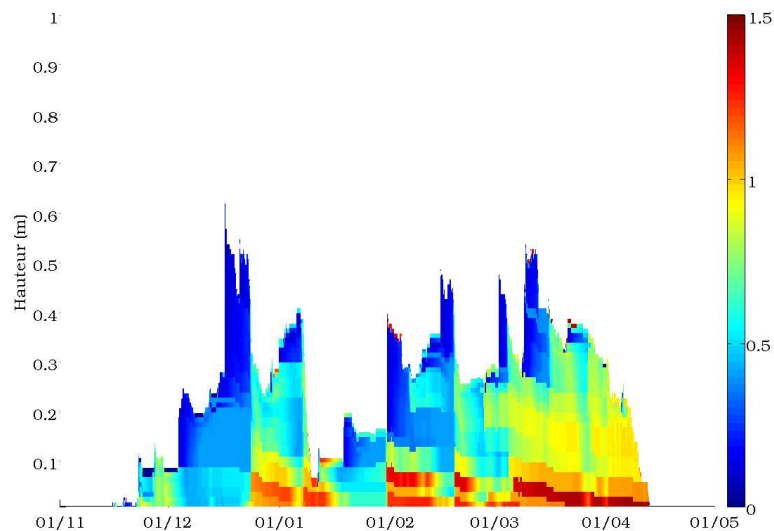
FIG. 8.13 – Evolutions verticale et temporelle du diamètre optique (mm) dans le manteau modélisé par Crocus du 1 er novembre au 1 er mai.
