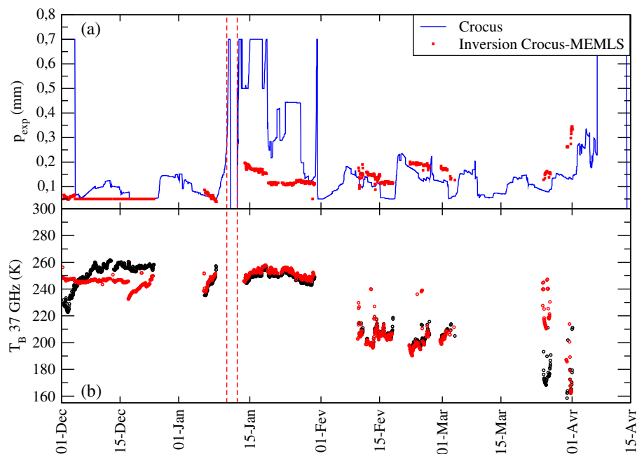
FIG. 8.17 – Evolutions temporelles de la longueur de corrélation exponentielle calculées à partir des profils de diamètre optique modélisés par Crocus (trait continu) et inversées à partir des températures de brillance observées, sur un manteau sec, en considérant un manteau homogène en taille de grains (carré) (a). Evolutions des températures de brillance observées (noir) et modélisées avec les modèles couplés Crocus-MEMLS et le profil de taille de grains uniforme estimé par inversion des observations (rouge) (b).
