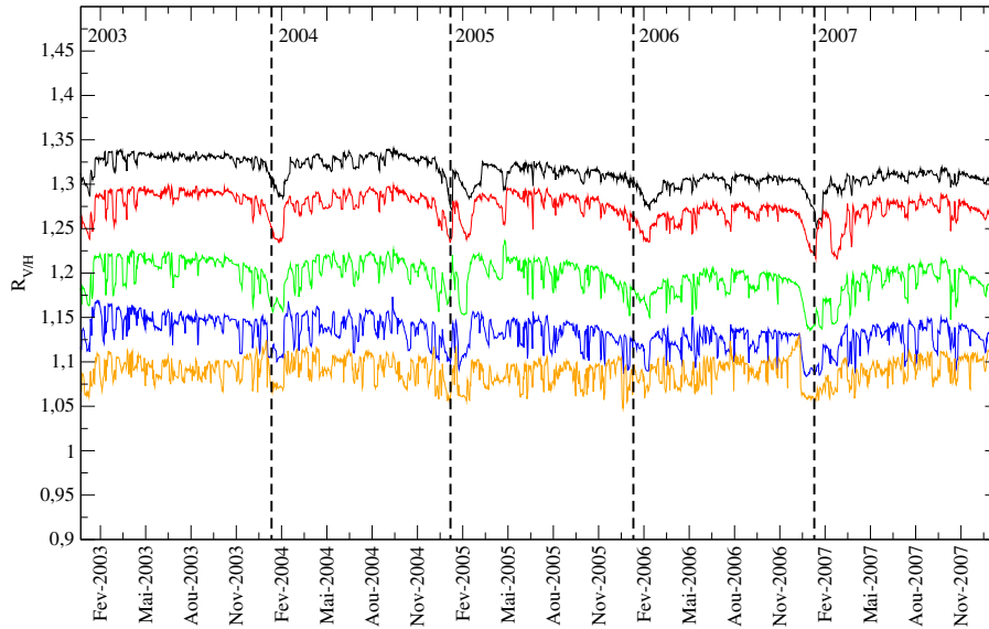
FIG. 6.10 – Evolution temporelle, à Dôme C entre 2003 et 2007, du rapport entre les températures de brillance polarisées verticalement et horizontalement, à 6,9, 10,7, 18,7, 36,5 et 89 GHz (de haut en bas).
