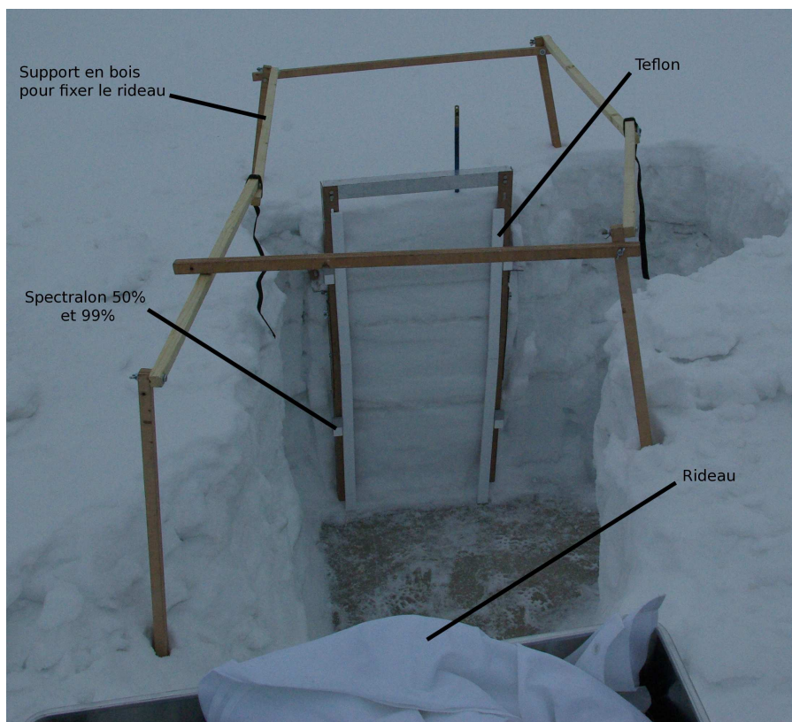
FIG. 2.8 – Photographie du dispositif pour mesurer la réflectance IR de la face du puits avec un appareil photographique modifié. Les photographies sont prises sous une lumière diffuse obtenue avec un rideau translucide placé sur le support en bois. Sur la face du puits sont placées des références calibrées (Spectralon 50% et 99%) ainsi que des barres de Téflon. Photographie prise le 27 février 2008 à Sept-Iles, Québec (L. Brucker).
