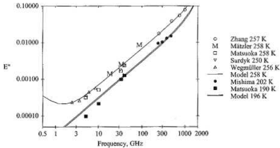
FIG. 3.5 – Comparaison de la partie imaginaire de la constante diélectrique de la glace ( \epsilon''_{glace} ) mesurée (symboles) et calculée (lignes) pour des fréquences comprises entre 0,5 et 2000 GHz à 196 K (symboles pleins) et 258 K (symboles ouverts). Figure extraite de Mätzler (2006) (Fig 5.11 p. 459).
