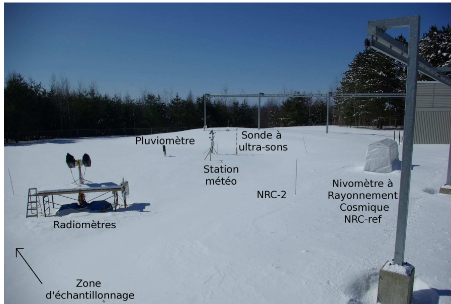
FIG. III.2 – Photographie de la disposition des instruments de mesures de la station SIRENE. Le Nivomètre à Rayonnement Cosmique (NRC) NRC-2 est enterré. Photographie prise le 23 mars 2008.
