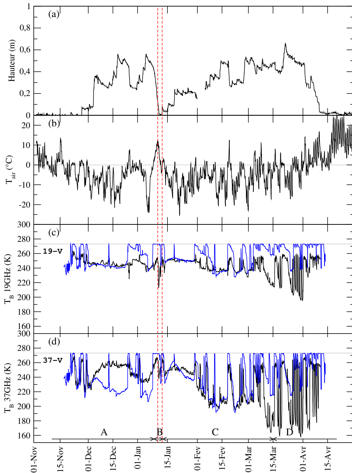
FIG. 8.8 – Evolution sur la saison 2007-08 de la hauteur de neige (a), de la température de l'air (b) et des températures de brillance observées (courbes noires) et modélisées avec Crocus-MEMLS (courbes bleues) en polarisation verticale à 19 GHz (c) et 37 GHz (d).
