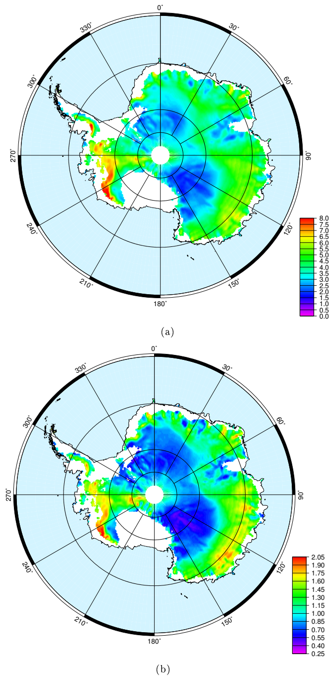
FIG. 5.12 – Carte des profondeurs de pénétration (en mètre) à 19,3 GHz (a) et 37 GHz (b) calculées avec MEMLS et le profil de longueur de corrélation déduit du spectre d'émissivité à 19,3 et 37 GHz.
