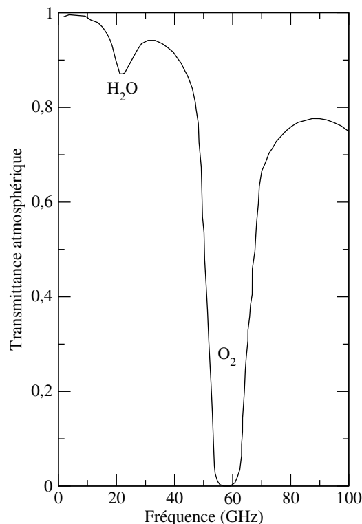
FIG. 3.1 – Transmittance atmosphérique représentant les fenêtres et les bandes d'absorption entre 1 et 100 GHz.
