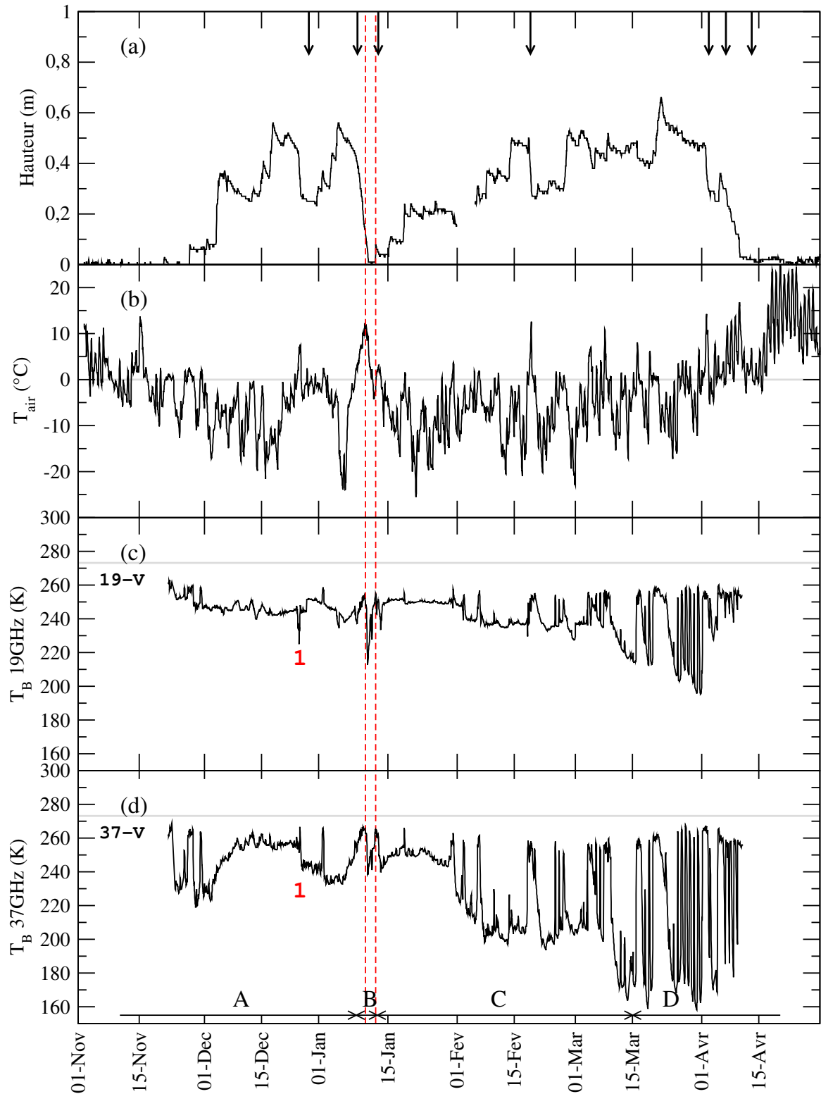
FIG. 8.4 – Evolutions temporelles de la hauteur de neige mesurée par la sonde à ultra-sons (a), de la température de l'air (b) et des températures de brillance mesurées par le radiomètre au sol à 19 GHz (c) et 37 GHz (d) en polarisation verticale .
