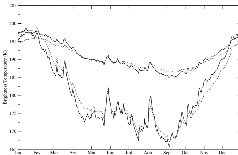
FIG. 4.15 – Evolution temporelle de la température de brillance observée avec AMSR-E (trait continu) et modélisée par MEMLS (trait interrompu), à 18,7 GHz (en haut) et 36,5 GHz (en bas). Contrairement à la Figure 4.10, le profil de taille de grains utilisé ici est estimé par une méthode de Monte Carlo.
