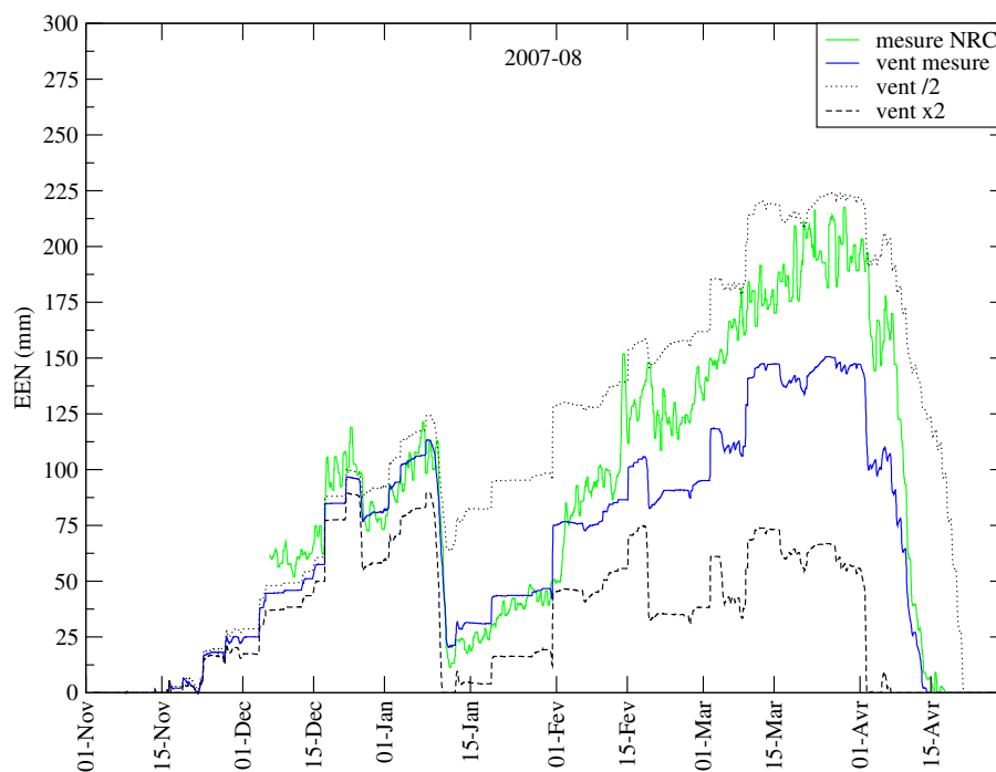
FIG. 7.10 – Evolution de l'EEN (en mm) mesurée par le NRC (trait vert) et modélisée par Crocus pour trois vitesses de vent différentes : mesurée (trait continu), divisée par 2 (trait pointillé) et multipliée par 2 (trait interrompu).
