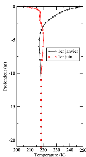
FIG. 4.1 – Profils de température mesurés avec 35 thermomètres à Dôme C le 1 er janvier 2007 (ronds) et le 1 er juin 2007 (carrés), jusqu'à 21 m de profondeur.
