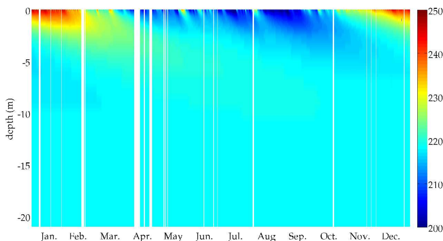
FIG. 4.11 – Evolution horaire de la température de la neige (en Kelvin) à Dôme C au cours de l'année 2007, de la surface jusqu'à 21 m de profondeur. Les traits blancs verticaux sont des manques dans la série de mesures.
