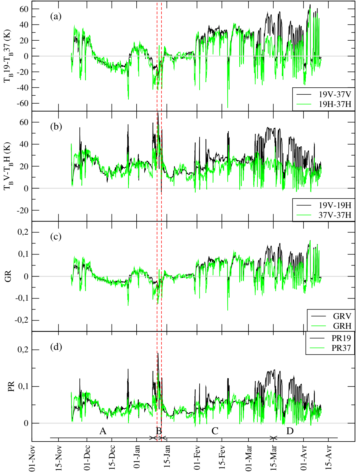
FIG. 8.6 – Evolutions temporelles de l'écart entre les fréquences (a), l'écart entre les polarisations (b), du gradient de fréquence GR^* (c) et du gradient de polarisation PR^* (d).
