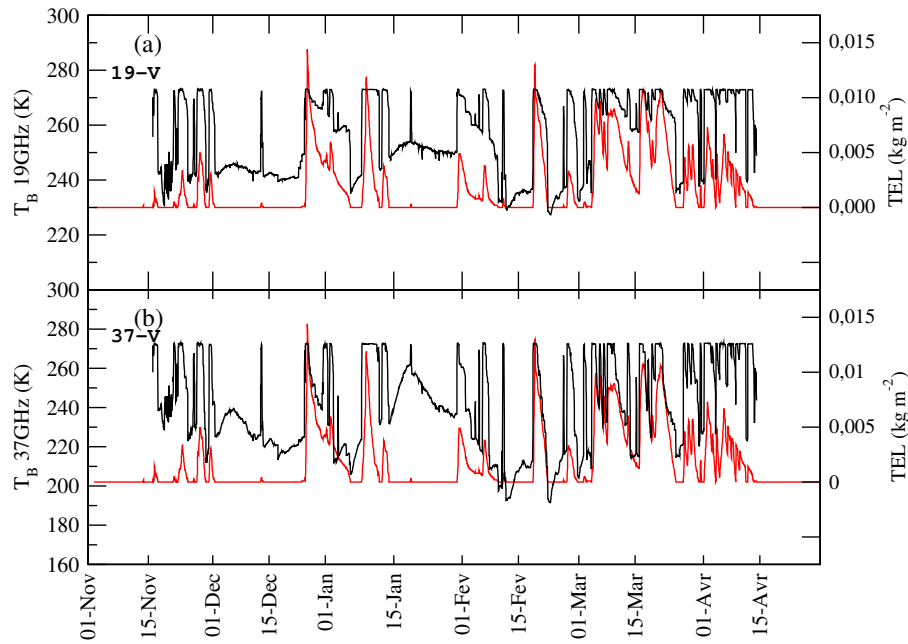
FIG. 8.12 – Evolutions des températures de brillance modélisées (noir) à 19 GHz (a) et 37 GHz (b) et de la TEL totale du manteau modélisée par Crocus (rouge).
