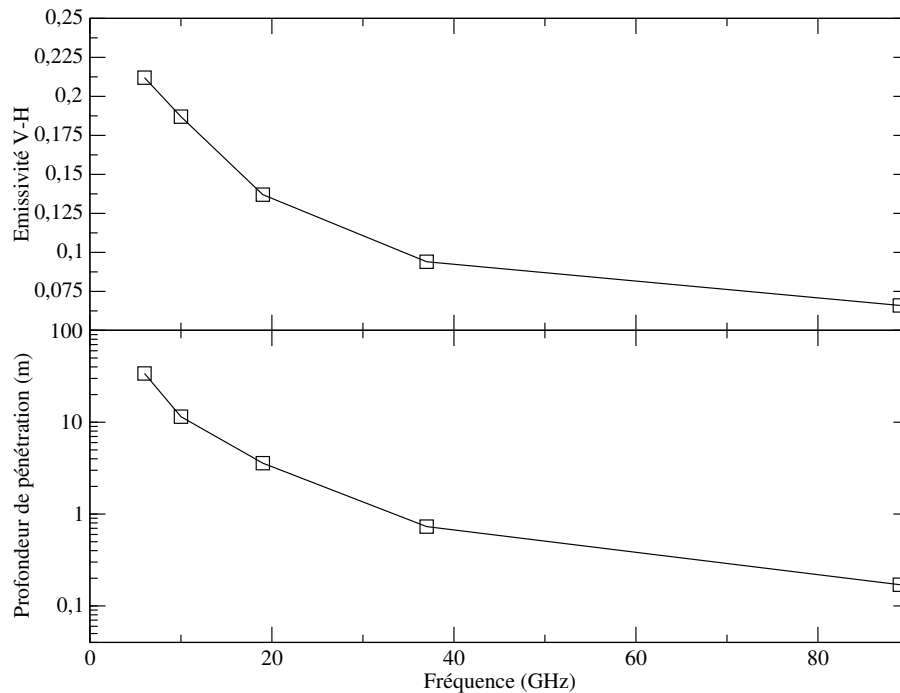
FIG. 6.9 – Spectre, à Dôme C, de l'écart d'émissivité entre les polarisations verticale et horizontale (en haut) et de la profondeur de pénétration (en bas).
