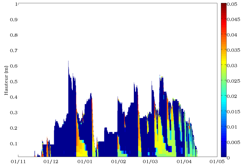
FIG. 8.10 – Evolutions verticale et temporelle de l'humidité ( \text{g cm}^{-3} ) dans le manteau modélisé par Crocus du 1 er novembre au 1 er mai.
