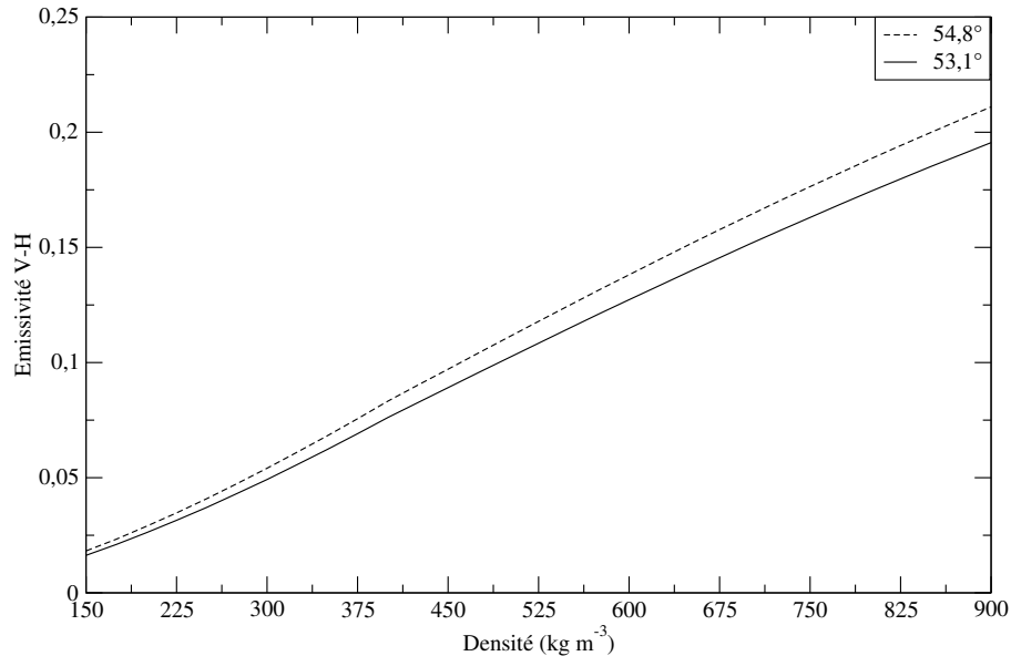
FIG. 6.3 – Evolution de l'écart d'émissivité entre les polarisations verticale et horizontale, pour un manteau homogène, en fonction de la densité. L'évolution est calculée avec les équations de Fresnel pour un angle d'incidence de 53,1° (SSM/I) et 54,8° (AMSR-E).
