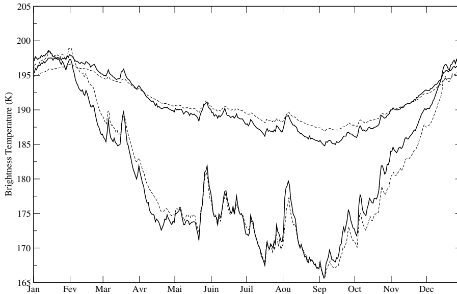
FIG. 4.10 – Evolution temporelle de la température de brillance observée avec AMSR-E (trait continu) et modélisée par MEMLS (trait interrompu), à 18,7 GHz (en haut) et 36,5 GHz (en bas). Le profil stratigraphique de taille de grains utilisé par MEMLS provient des photographies IR.
