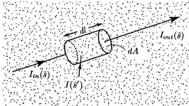
FIG. 3.4 – Représentation d'un milieu rempli d'un grand nombre de particules où se trouve un volume cylindrique, de longueur dl , contenant des particules. I est l'intensité énergétique interagissant avec le volume. Le volume cylindrique a son axe dans la direction \hat{s} (figure 7.1.1, Tsang et al., 2000b).
