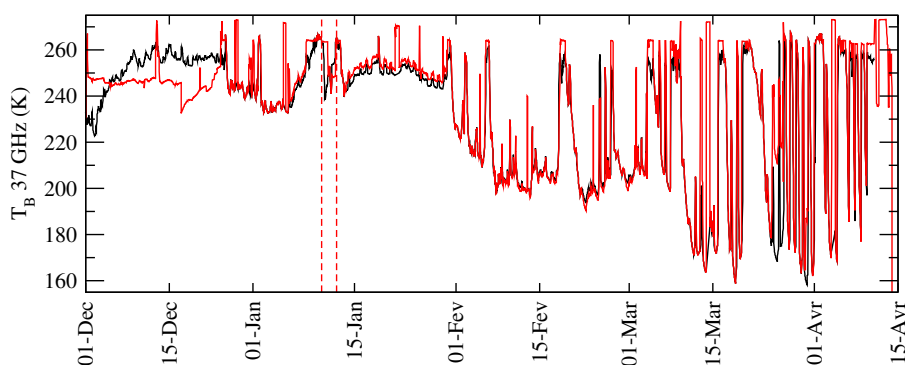
FIG. 8.18 – Evolution sur toute la saison de la température de brillance observées (noir) et modélisées avec les modèles couplés Crocus-MEMLS et le profil de taille de grains uniforme estimé par inversion des observations.
