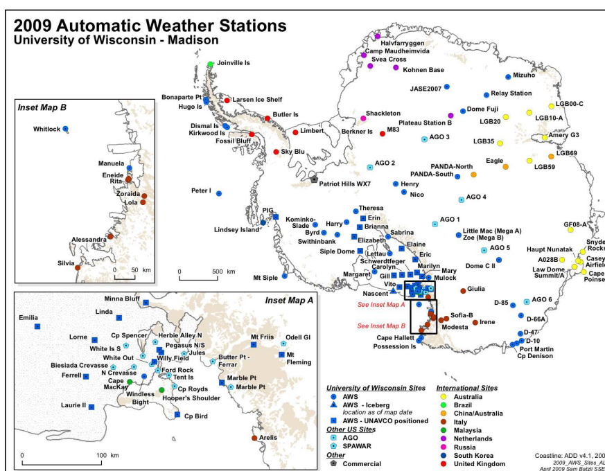
FIG. 1.2 – Carte de la localisation des stations météorologiques automatiques en Antarctique. Figure extraite de http://amrc.ssec.wisc.edu .
