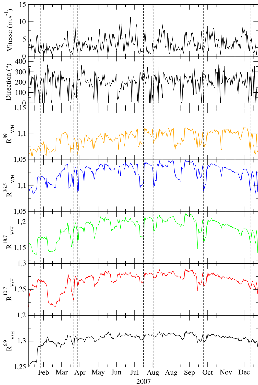
FIG. 6.13 – Evolution temporelle en 2007 de la vitesse et direction du vent mesurées par la station automatique de Dôme C (les deux panneaux du haut). Les panneaux suivant correspondent au rapport de températures de brillance.
