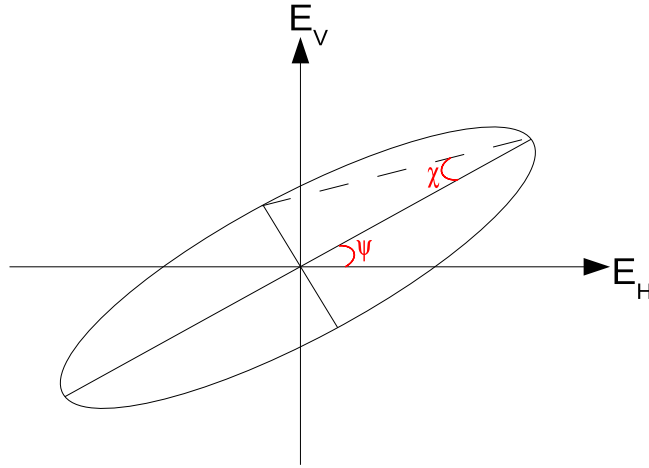
FIG. 6.1 – Schématisation de la forme d'une polarisation, elliptique, circulaire ( \chi=45^\circ ) ou linéaire ( \chi=0^\circ ). Lorsque l'onde est linéaire, la polarisation est verticale pour \psi=90^\circ ou horizontale pour \psi=0^\circ ou \psi=180^\circ .
