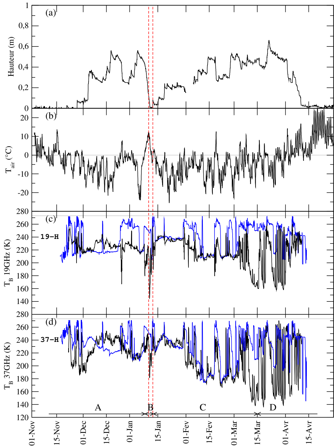
FIG. 8.9 – Evolution sur la saison 2007-08 de la hauteur de neige (a), de la température de l'air (b) et des températures de brillance observées (courbes noires) et modélisées avec Crocus-MEMLS (courbes bleues) en polarisation horizontale à 19 GHz (c) et 37 GHz (d).
