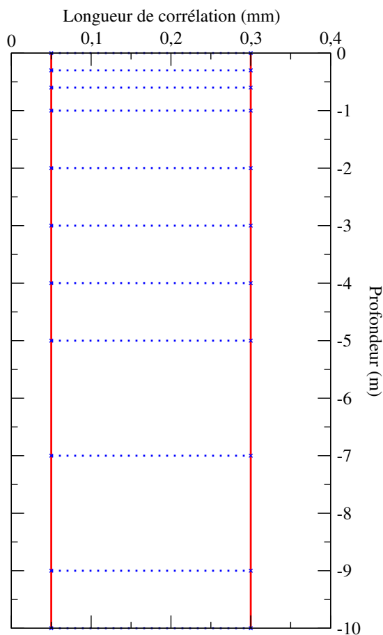
FIG. 4.12 – Caractéristiques du profil de taille de grains utilisé par la méthode de Monte Carlo pure. La gamme de taille de grains possible lors de l'estimation du profil est 0,05 mm - 0,3 mm, et est représentée par les lignes verticales rouges. Les lignes horizontales en pointillé bleues représentent la répartition des profondeurs auxquelles sont tirées aléatoirement les tailles de grains.
