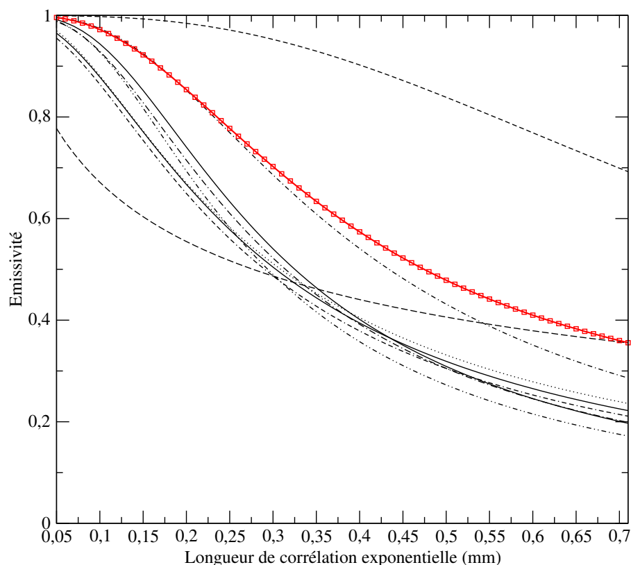
FIG. 3.7 – Evolution de l'émissivité d'un manteau neigeux homogène en fonction de la longueur de corrélation pour les 11 paramétrisations empiriques du coefficient de diffusion (courbes noires) et la paramétrisation théorique basée sur l'approximation de Born améliorée (courbe rouge avec les carrés).
