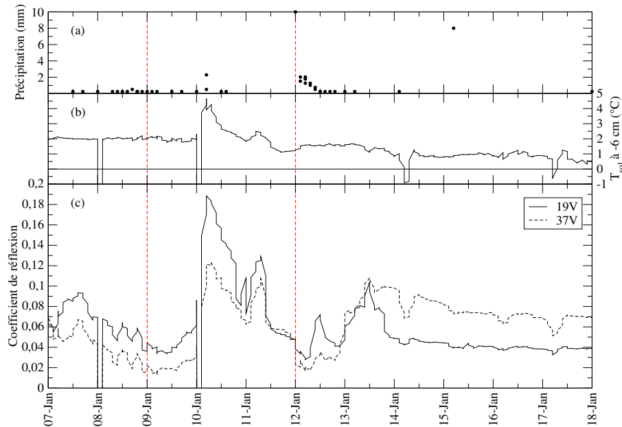
FIG. 8.7 – Evolutions sur la période du 7 au 18 janvier de la quantité de précipitation mesurée (a), de la température à 6 cm de profondeur dans le sol (b) et des coefficients de réflexion calculés avec l'Equation 8.2 (c).
