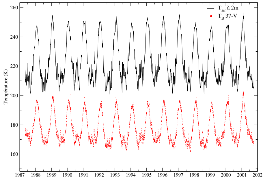
FIG. 1.3 – Evolutions temporelles, à Dôme C entre juin 1987 et 2002, de la température de l’air à 2 m mesurée par la station automatique (trait continu noir) et de la température de brillance acquise à 37 GHz en polarisation verticale mesurée par les radiomètres micro-ondes Special Sensor Microwave/Imager (SSM/I) F8, F11 et F13.
