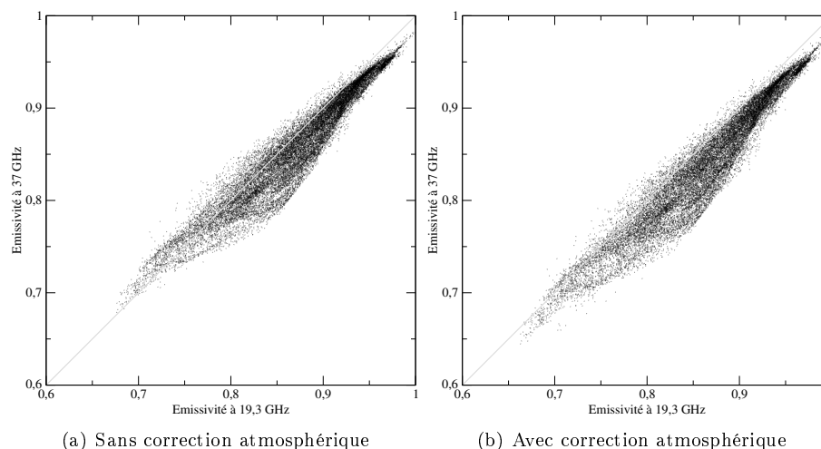
FIG. 3.12 – Émissivité moyenne, à 37 GHz en fonction de celle à 19,3 GHz, de chaque pixel observé hors des zones de fonte en Antarctique. Les émissivités sont calculées sans (a) et avec (b) correction atmosphérique.
