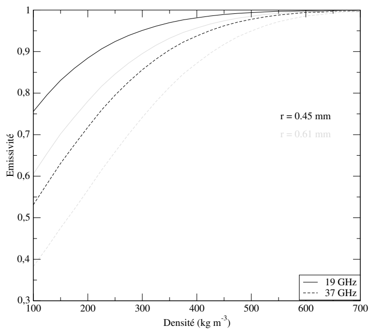
(b) DMRT-ML
