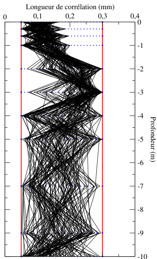
FIG. 4.13 – Résultat de l'estimation des profils de taille de grains par la méthode de Monte Carlo, afin que l'évolution temporelle de la température de brillance soit prédite avec une RMSE moyenne inférieure à 3 K. 150 profils sont présentés.
