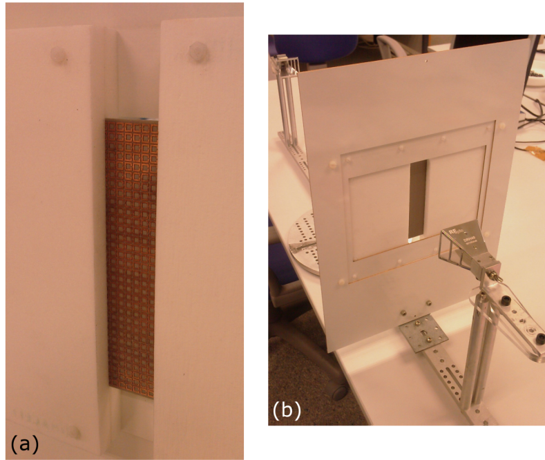
FIGURE 4.28 – (a) Vue d'une des couches de SRR constituant le prototype, dans son support. (b) Vue d'ensemble du banc en transmission, comportant deux antennes cornet large bande pour une caractérisation de 4 à 40 GHz. Le matériau blanc visible sur les deux vues est une mousse (Rohacell) d'indice proche de 1 dans la gamme micro-ondes.
