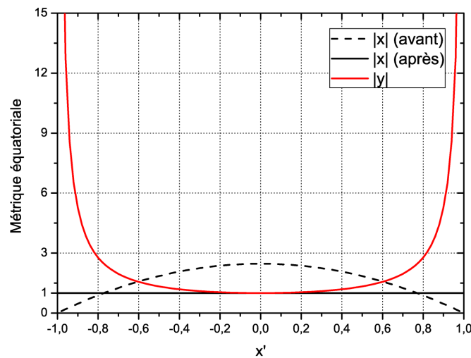
FIGURE 5.30 – Métriques au niveau de l'équateur ( y' = 0 ) en fonction de la position. Pour la métrique |x| , les valeurs avant (tirets noirs) et après (courbe noire) modification de la fonction de Mercator sont représentées.
