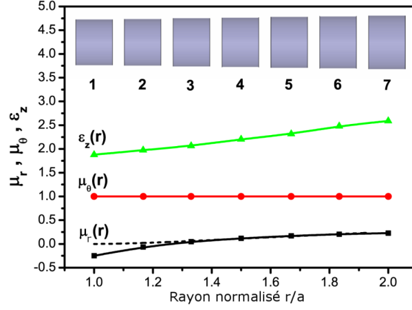
FIGURE 5.4 – Paramètres matériau à la fréquence de fonctionnement (580 GHz) en fonction de la position dans le revêtement, pour le dimensionnement retenu. Pour chacune des 7 couches le cylindre constituant la cellule élémentaire est représenté au-dessus des courbes. Pour le paramètre \mu_r , la courbe en pointillés indique les paramètres initialement visés.
