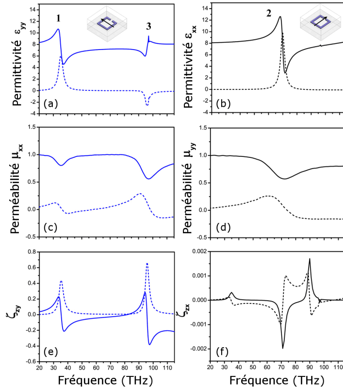
FIGURE 4.20 – Evolutions fréquentielles des paramètres effectifs de permittivité (a-b), de perméabilité (c-d) et de bianisotropie (e-f) d'une cellule du réseau MIR, obtenues par intégration des champs à partir deux simulations d'orientation \phi = 0^\circ (a,c,e) et \phi = 90^\circ (b,d,f). Les traits continus et les pointillés représentent respectivement les parties réelles et imaginaires des paramètres.
