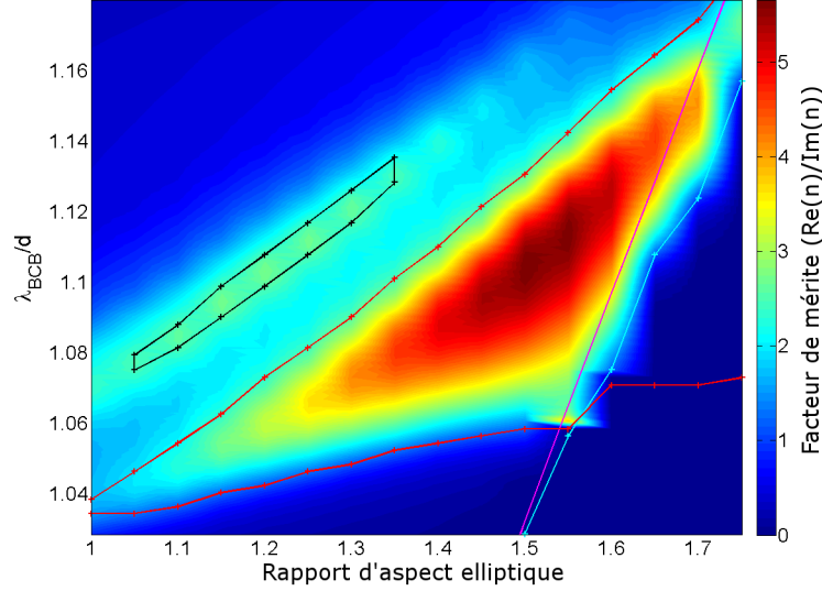
FIGURE 4.43 – Carte d'évolution du facteur de mérite de l'indice en fonction du rapport d'aspect elliptique et de la longueur d'onde dans le BCB ( \lambda_0/n_{BCB} normalisée par la période d du réseau. Les deux courbes rouges et noires délimitent les zones où la perméabilité est négative respectivement dans la première et la seconde zone de Brillouin de la pile. Les courbes cyan et rose indiquent respectivement la fréquence plasma électrique et la fréquence de coupure (analogue à une fréquence plasma) théorique pour un guide elliptique de mêmes dimensions que les ouvertures. Sur chaque courbe les croix indiquent les cas effectivement simulés (les courbes et la carte de couleurs sont interpolées). (N.B. : les écarts de fabrication sur les épaisseurs décrits au 4.3.2.2 sont inclus dans cette étude paramétrique.)
