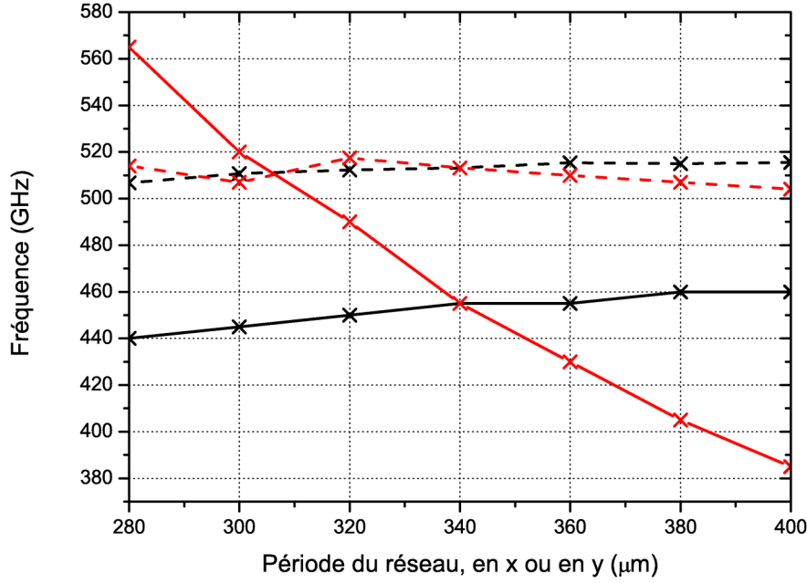
FIGURE 4.40 – Evolution de la fréquence plasma électrique (tirets) et de la fréquence de résonance magnétique (traits continus) extraites par inversion de Fresnel de simulations de lames de 5 cellules, en fonction de la période en y lorsque la période en x est fixée à 340 \mu\text{m} (courbes rouges) et en fonction de la période en x lorsque la période en y est fixée à 340 \mu\text{m} (courbes noires). Les cas simulés correspondent aux croix, les lignes servant uniquement de guides pour les yeux. (N.B. : les écarts de fabrication sur les épaisseurs décrits au 4.3.2.2 sont inclus dans cette étude paramétrique.)
