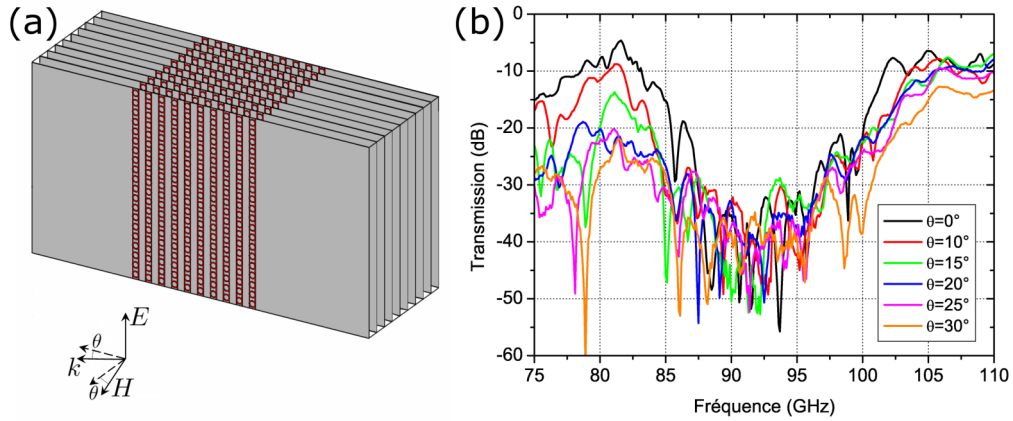
FIGURE 3.27 – (a) Schéma du prototype en bande W montrant l'angle d'incidence \theta et (b) spectres de transmission en amplitude mesurés, en fonction de cet angle. La flèche indique le sens des angles d'incidence croissants (de 0 à 30^\circ par pas de 5^\circ ).
