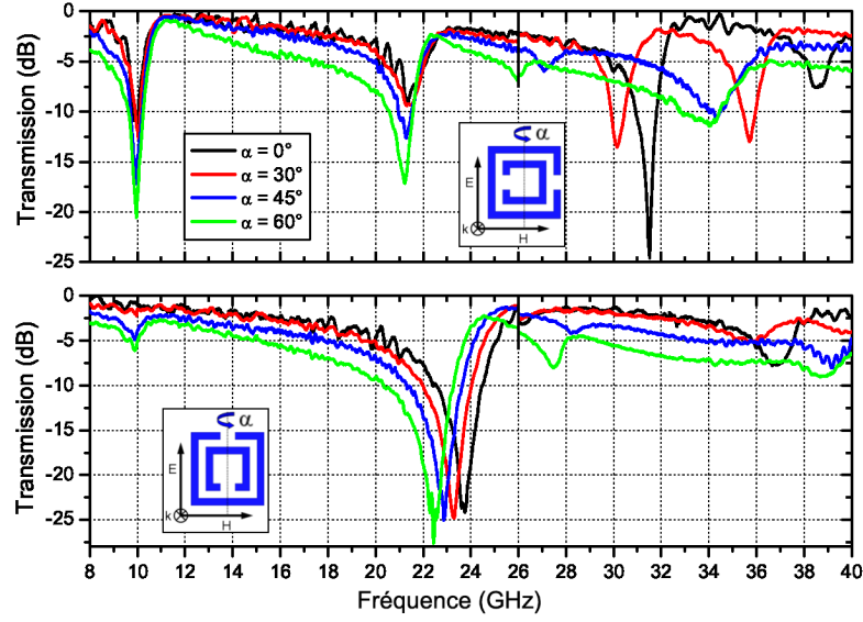
FIGURE 4.7 – Spectres expérimentaux de l’amplitude de la transmission à travers le réseau planaire de ECSR entre 8 et 40 GHz, en polarisation TE, pour différents angles d’incidence \alpha et pour deux orientations du réseau par rapport au champ électrique (en insert).
