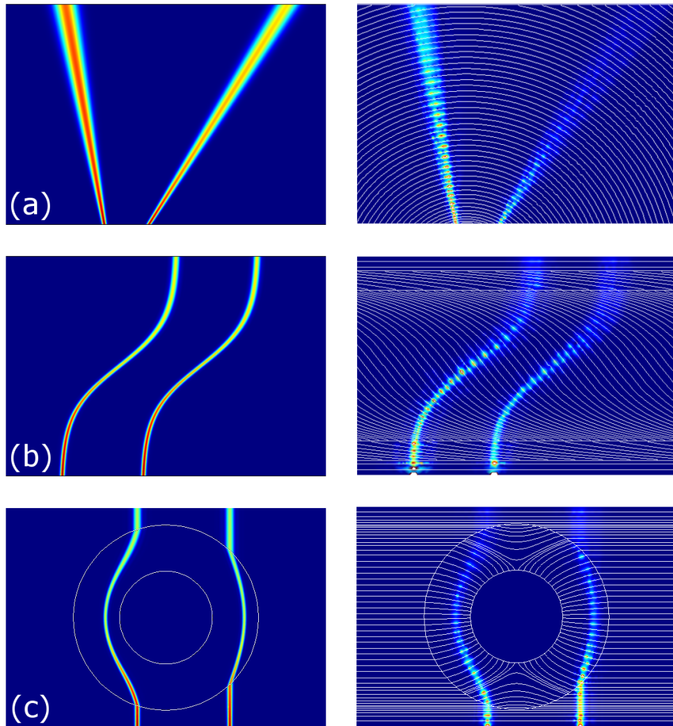
FIGURE 5.25 – Cartes d’amplitude normalisée du champ magnétique dans les dispositifs d’agrandissement (a), de translation (b) et d’évitement de zone (c), utilisant un matériau homogène présentant les paramètres effectifs requis (après simplification) (colonne de gauche) et incluant la microstructuration sous forme de couches conformées alternativement diélectriques et métalliques (colonne de droite).
