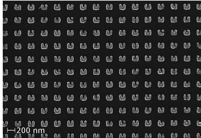
FIGURE 4.14 – Vue au microscope électronique d'un détail du prototype NIR.
