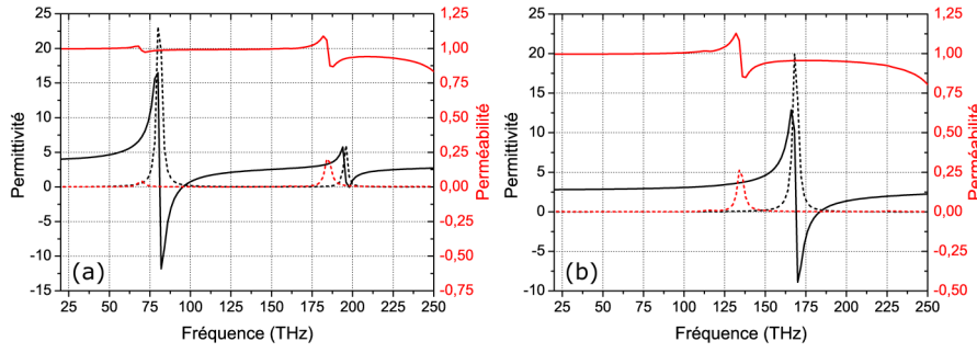
FIGURE 4.26 – Spectres de permittivité (en noir) et de perméabilité (en rouge) complexes (partie réelle et partie imaginaire respectivement en traits continus et en pointillés, extraits par intégration des champs pour la cellule de la figure 4.22 symétrisée (voir légende de la figure 4.23), pour les orientations de réseau \phi = 0^\circ (a) et \phi = 90^\circ (b), telles qu’elles ont été définies au 4.2.2.
