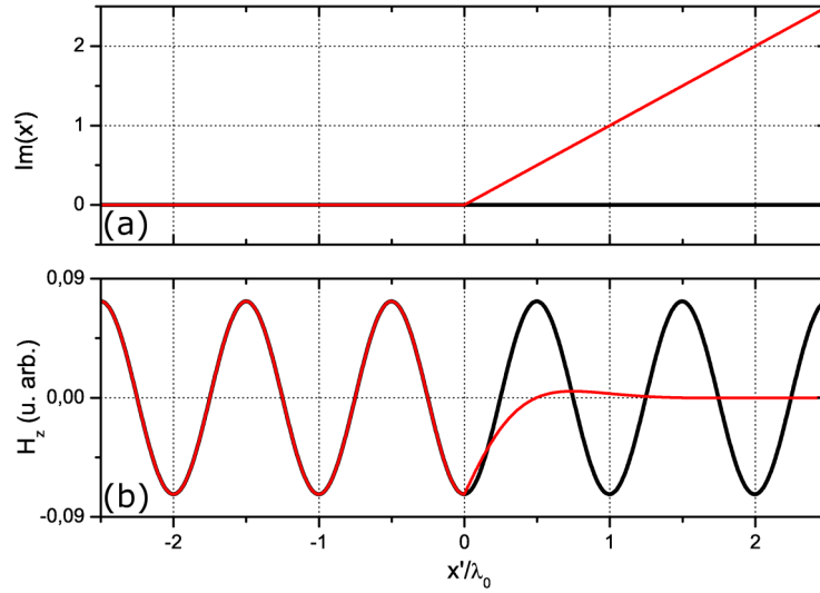
FIGURE 2.13 – (a) Partie imaginaire de la coordonnée x' dans l'interprétation topologique et (b) relevé correspondant du champ H_{z'} dans la direction x' dans l'interprétation matériau, en l'absence de transformation (courbes noires) et avec la transformation de l'équation 2.25 (courbes rouges).
