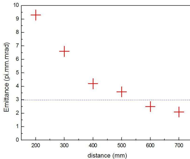
Figure 77 : Emittance en fonction de la distance. La pression du gaz est de 5.10^{-2} mbar. Les ions ^{133}\text{Cs}^+ sont à une intensité de 1 \mu\text{A} . Le potentiel RF est de 10 \text{ kV}_{pp} à 5.42 \text{ MHz} .
