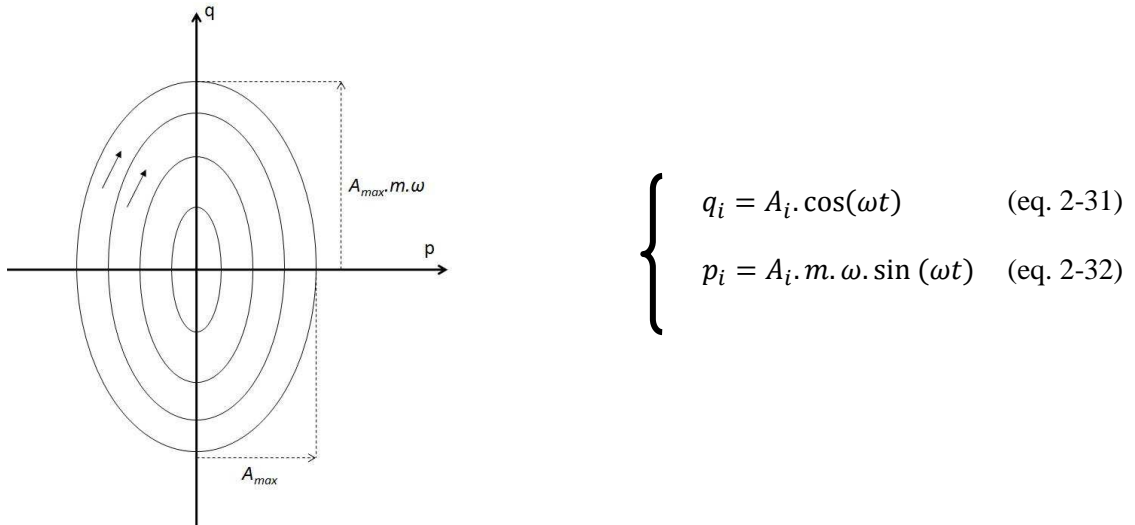
Figure 21 : Évolution de l'espace de phase de particules soumises à un potentiel RF.
