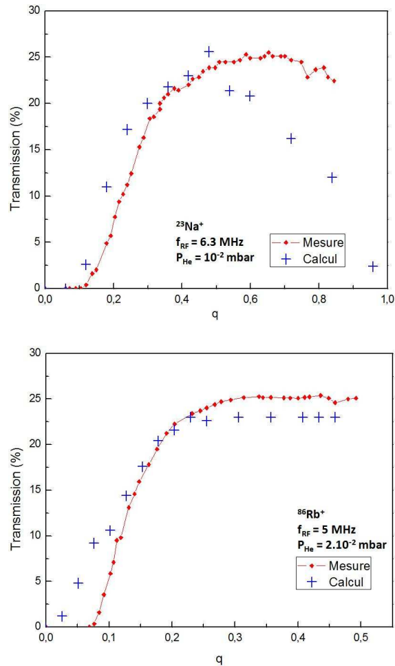
Figure 58 : Évolution de la transmission en fonction de l'amplitude RF pour ^{23}\text{Na}^+ (à gauche) et ^{87}\text{Rb}^+ (à droite).
