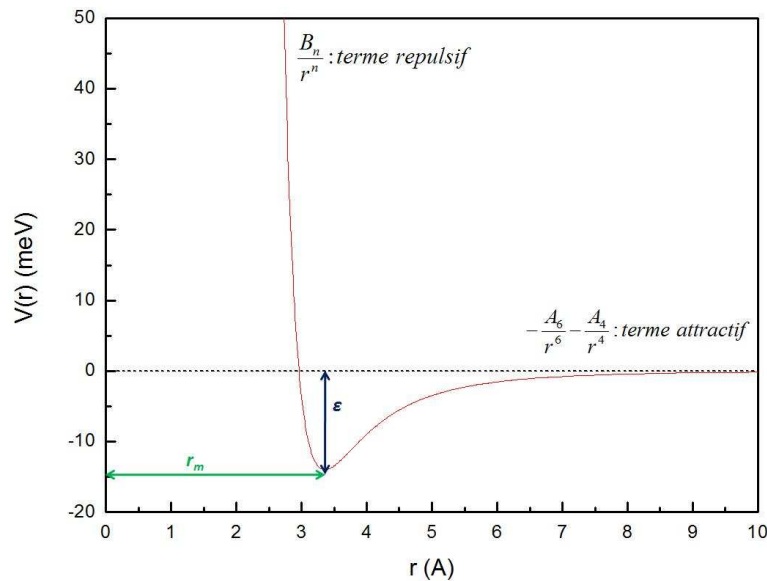
Figure 23 : Puits de potentiel pour ^{133}\text{Cs}^+ sur He. \varepsilon est la profondeur du puits de potentiel et r_m , sa position.
