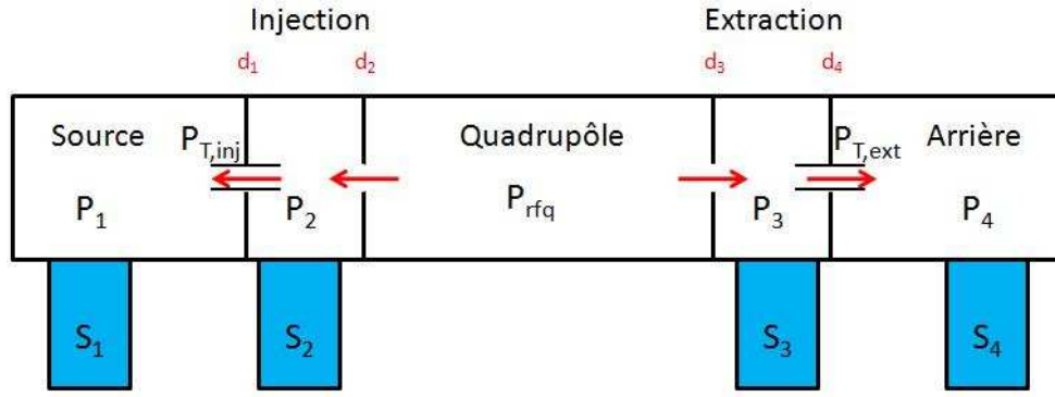
Figure 87 : Système considéré pour la phase 2
