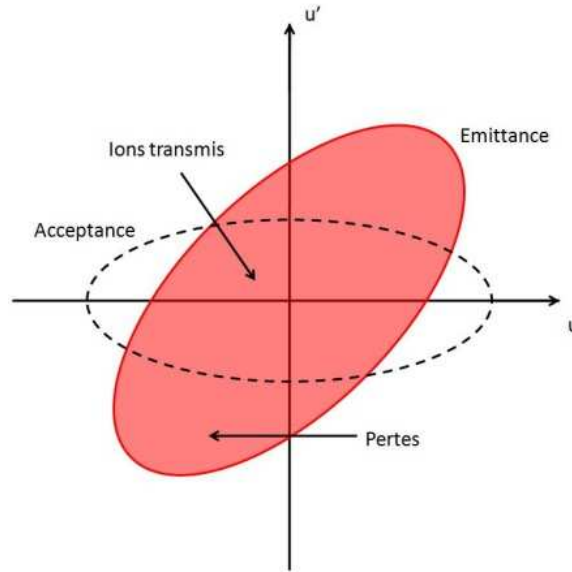
Figure 7 : Comparaison entre l'émission du faisceau et l'acceptance de l'appareil.
