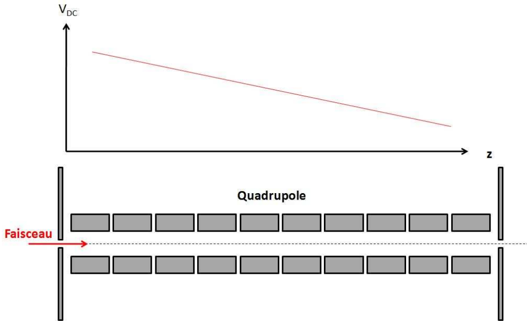
Figure 31 : Application du potentiel de guidage sur le quadripôle. Ceci est obtenu par l'application de potentiel continu sur un quadripôle segmenté.
