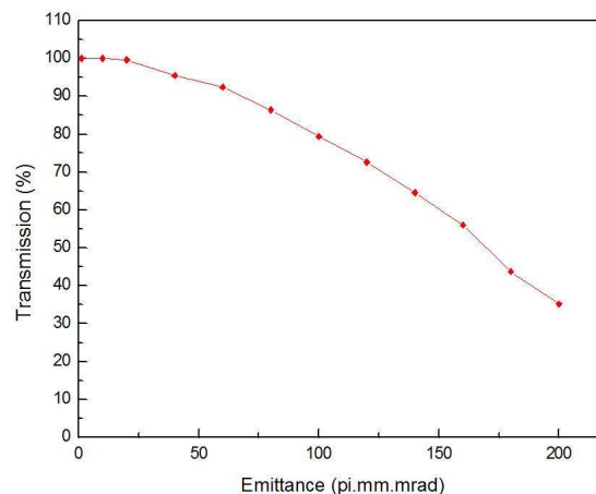
Figure 73 : Cas de la focalisation de faisceaux de Césium 133 Cs + à 60 keV à 1 μA sans l'application du potentiel RF. La transmission est calculée juste derrière l'orifice d'entrée du quadripôle. La plateforme HT est à 59900 V.
