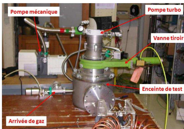
Figure 51 : Système de vide
