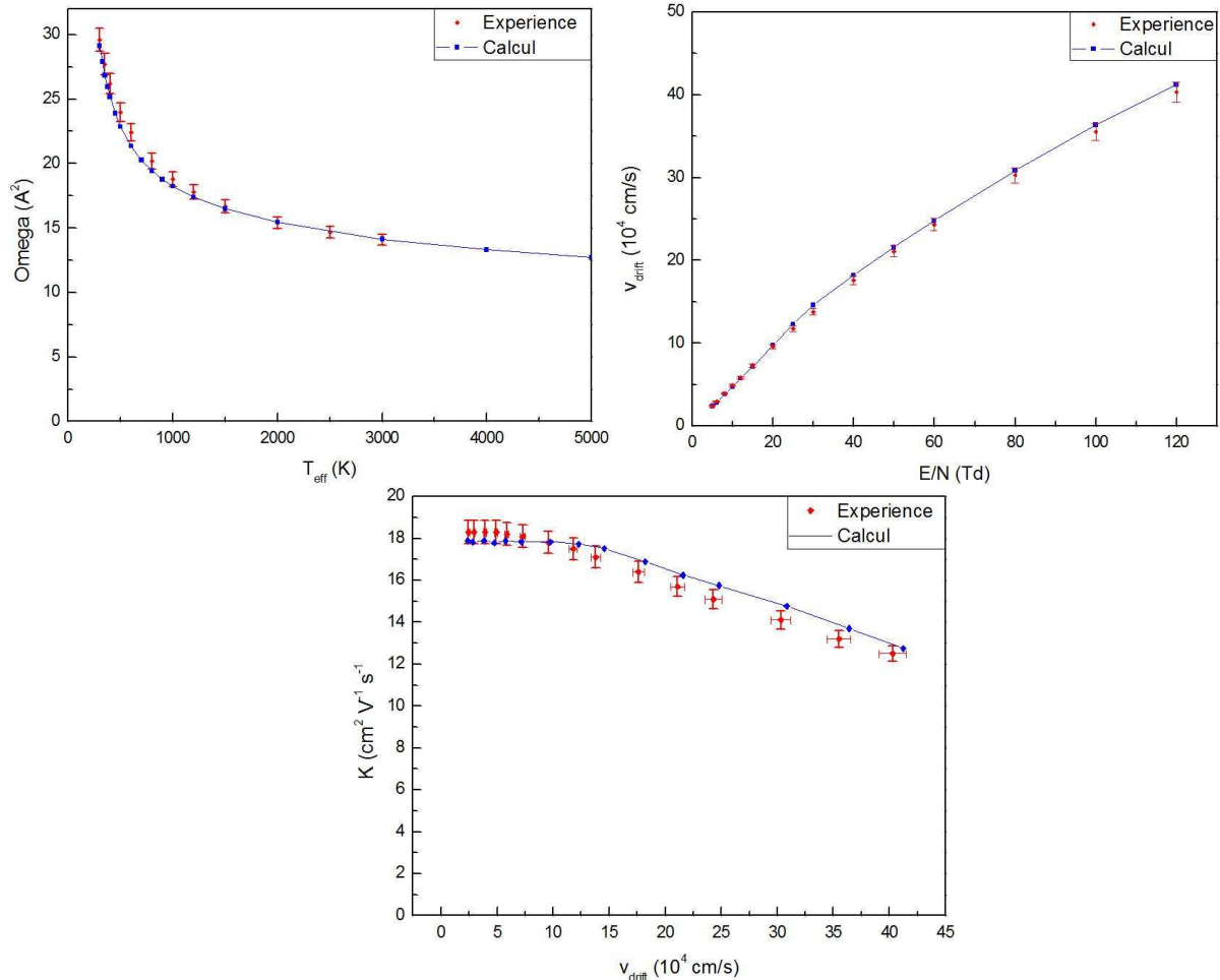
Figure 24 : Comparaison entre le calcul et les données expérimentales [Eli78] pour \text{Cs}^+ sur He.
