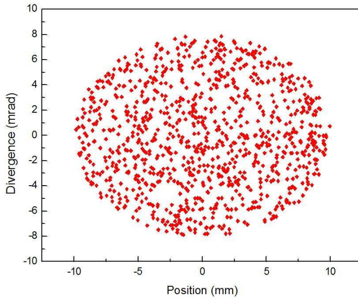
Figure 69 : Faisceau-type de 80 \pi .mm.mrad utilisé comme référence.
