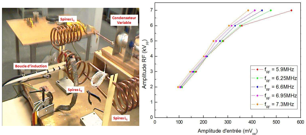
Figure 92 : Banc de test du système RF de SHIRaC-Phase2 : en haut, le résonateur avec la boucle d'induction, les trois branches et le condensateur variable, (en bas), les potentiels RF obtenus.
