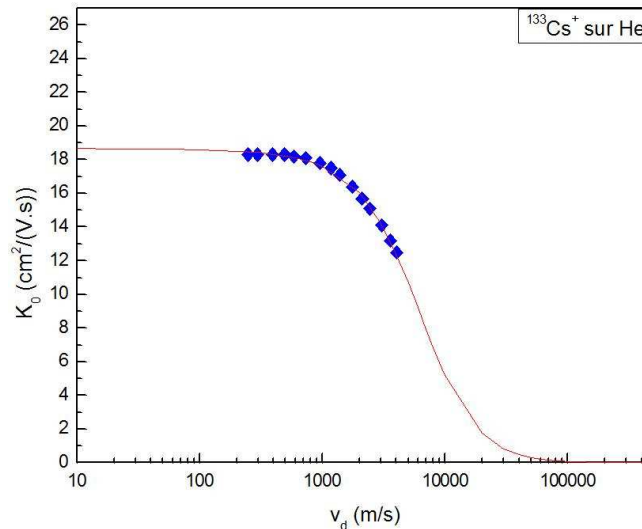
Figure 22 : Constante de mobilité en fonction de l'énergie de l'ion pour des ions Cs^+ interagissant avec des atomes d'Hélium.
