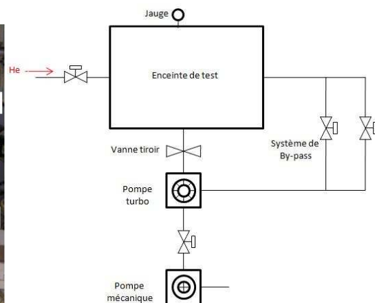
Figure 51 : Système de vide
