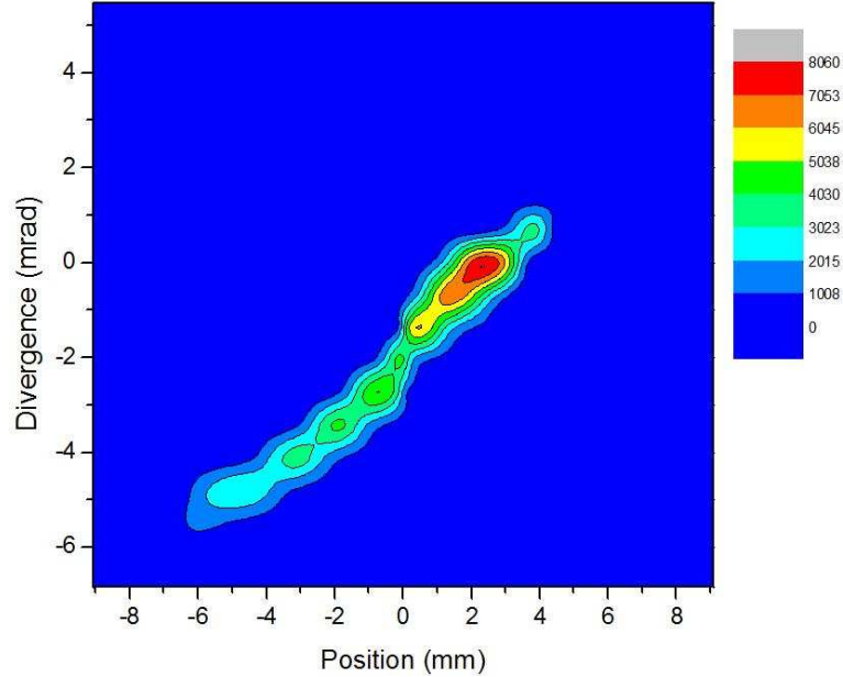
Figure 66 : Diagramme d'émission pour un faisceau refroidi avec SHIRaC-Phase1 et mesuré avec un emittance-metre à balayage électrostatique [Bac00]. Le potentiel RF est de 1800V pp à 5MHz. La pression d'Hélium est de 10^{-2} mbar. L'emittance est de 2 \pi \cdot \text{mm} \cdot \text{mrad} à 60 keV.
