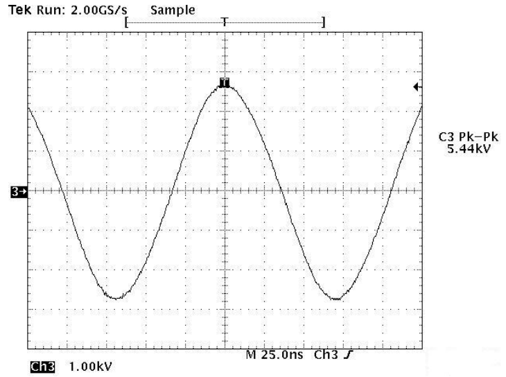
Figure 39 : A gauche, la boucle d'induction est placée dans le résonateur ce qui assure le couplage entre les circuits primaire et secondaire. L'oscillogramme à droite représente la plus haute amplitude RF obtenue au banc d'essai avec une capacité de 68 pF à la place du résonateur.
