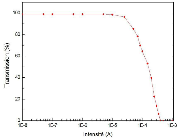
Figure 72 : Transmission en fonction de l'intensité pour un faisceau 133 Cs + de 80 π.mm.mrad à 60 keV. La transmission est calculée juste derrière l'orifice d'entrée du quadripôle.
