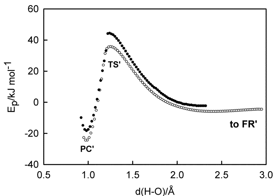
FIG. 5.6 – Oxydation du méthane-thiol par HO_2^\bullet : trajectoires de réaction du chemin a en phase gazeuse (cercles blancs) et en phase aqueuse (cercles noirs). Les courbes ont été calculées au niveau UB3LYP/6-311+G(d,p) en scannant la surface d'énergie potentielle en fonction de la distance d_{O-H_S} .
