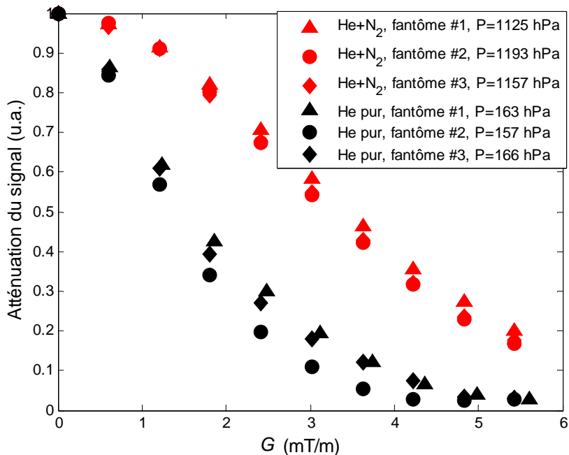
Figure 4-15 Atténuation du signal dans les trois fantômes en fonction du gradient de diffusion G appliqué sur l'axe X pour des pressions similaires. Deux séries de données sont montrées, une est acquise pour l'hélium dans l'azote à P = 1158 \pm 34 hPa et l'autre pour l'hélium pur à P = 162 \pm 26 hPa.
