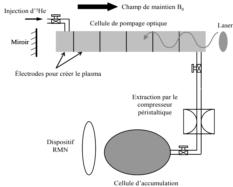
Figure 3-1 Schéma détaillé du polariseur.
