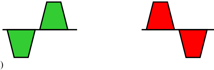
Figure 3-32 (a) Gradient de diffusion avec polarité (-/+), appelée m ; (b) gradient de diffusion avec polarité (+/-), appelée p.
