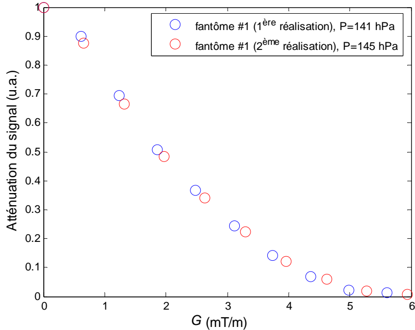
Figure 4-8 Atténuation du signal expérimentale en fonction du gradient de diffusion G appliqué le long de l'axe Z. Les pressions P sont similaires avec P = 141 hPa pour la première réalisation du fantôme #1 et P = 145 hPa pour la deuxième réalisation.
