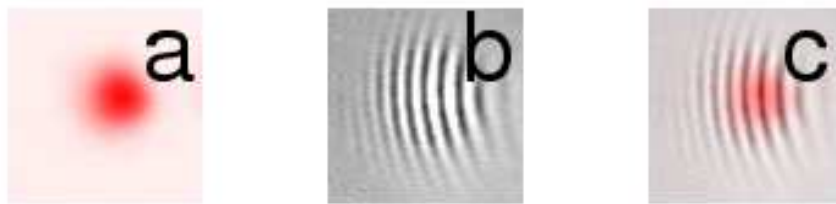
FIGURE 2.34 – a) Profil d'intensité d'un soliton de cavité (image colorée en rouge). b) Interférogramme du même soliton de cavité de la figure a) avec une onde de référence. Le réseau de frange caractérise la phase du soliton. c) Somme de a) et b). Nous observons peu de déviations dans les lignes d'intensité indiquant que le profil de phase des solitons de cavité change peu suivant le rayon de la structure.
