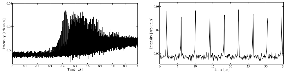
FIGURE 4.9 – Intensité émise par une structure laser lors de l'allumage. À gauche : Nous observons la totalité du transitoire. À droite : Zoom de ce transitoire (autour de 0.4 \mu\text{s} ). Le transitoire est caractérisé par un comportement pulsé à l'ISL de la cavité externe. I_{L1} = 278.8\text{mA} , I_{L2} = 15\text{mA} , \Delta T^o = -6.8^\circ\text{C} , \text{ISL} \sim 250\text{MHz} .
