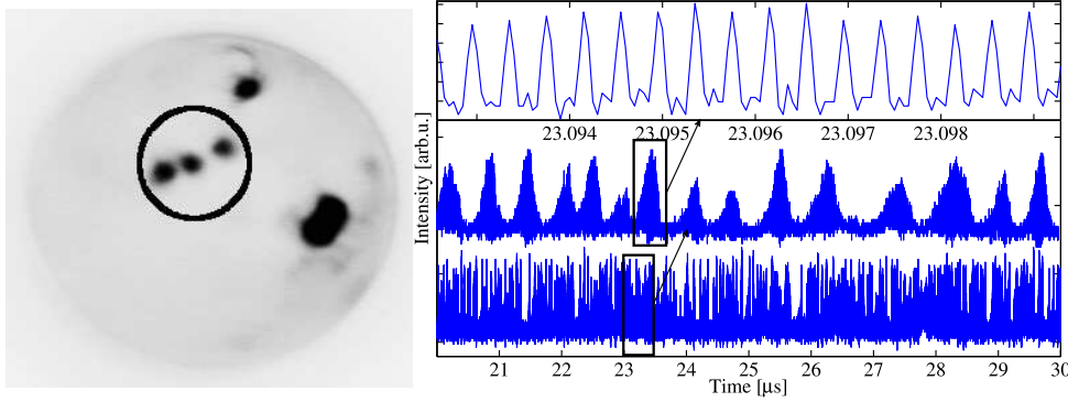
FIGURE 4.19 – À gauche : Champ proche du milieu amplificateur. Le cercle noir indique la zone d'espace où se passe le comportement temporel présenté à la figure de droite. Le signal temporel est constitué de paquets de pulses. Ce régime est connu pour être une combinaison de l'effet de verrouillage de mode passif et de l'effet de Q-switching.
