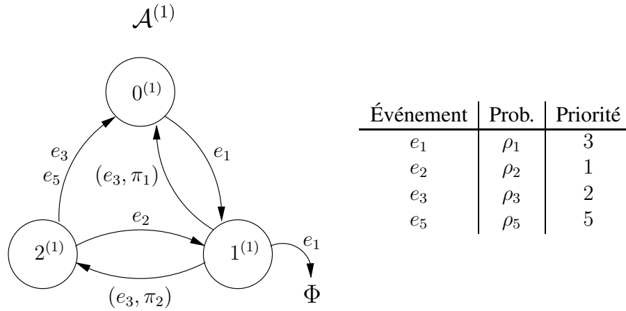
FIG. 7.4 – Représentation graphique de l’automate \mathcal{A}^{(1)}
