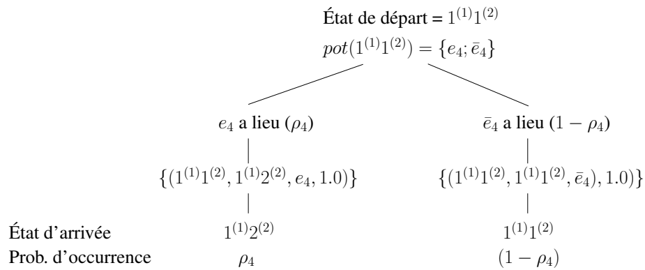
FIG. 7.19 – Construction des chaînes de transitions globales pour l'état 1^{(1)1^{(2)}}
