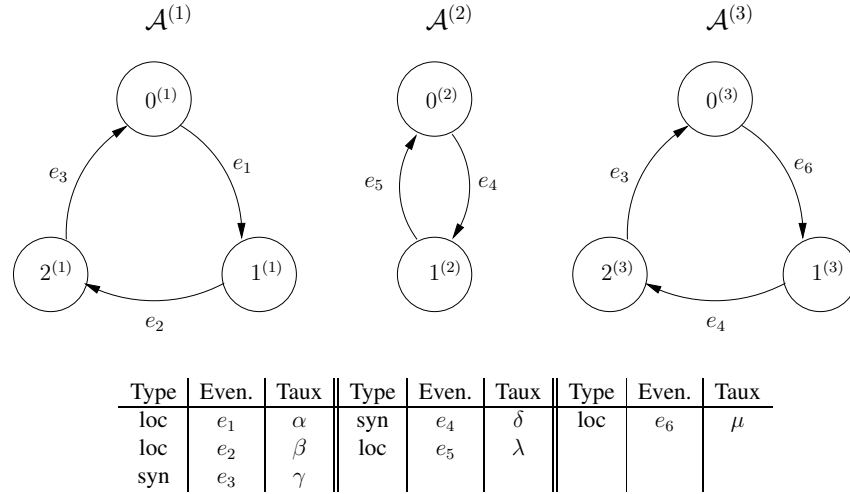
FIG. 2.2 – Modèle SAN avec événements synchronisants
