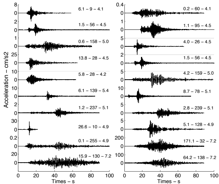
Figure 6: Exemples d'accélérogrammes extraits de la base de données du Réseau Accélérométrique Permanent RAP ( http://www-rap.obs.ujf-grenoble.fr ), montrant la variabilité du mouvement sismique en fonction de la distance, de la magnitude et des conditions de site.
