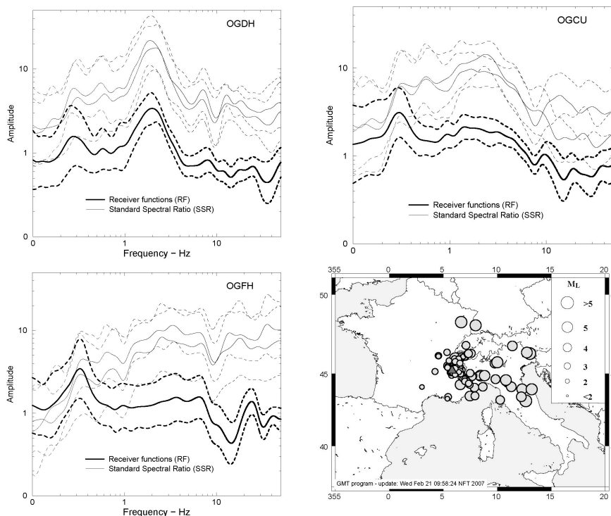
Figure 21: Amplification du mouvement du sol à trois stations du réseau accélérométrique permanent RAP installées dans le bassin grenoblois (stations OGCU, OGDH et OGFH). Les rapports spectraux selon la méthode proposée par Borchardt [44] ont été calculés par rapport à la station au rocher OGMU, en utilisant les enregistrements de la base de données du RAP représentés en carte. Les traits continus représentent la valeur moyenne des rapports (moyenne des composantes horizontales) et les discontinus les écarts-types. Seuls les enregistrements pour lesquels le rapport signal/bruit est supérieur à 3 ont été conservés (d'après [149]).
