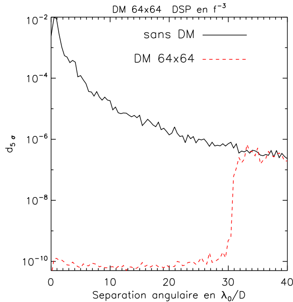
FIG. IV.1.5 – Détection à 5\sigma avant (trait continu noir) et après (tirets rouges) convergence de la boucle de correction en lumière monochromatique. Le défaut initial est de 20 nm rms avec une DSP en f^{-3} .
