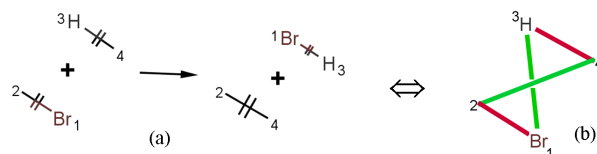
FIG. 6.14: Cœur (a) et graphe de réaction équivalent (b) de la réaction de la figure 6.11
