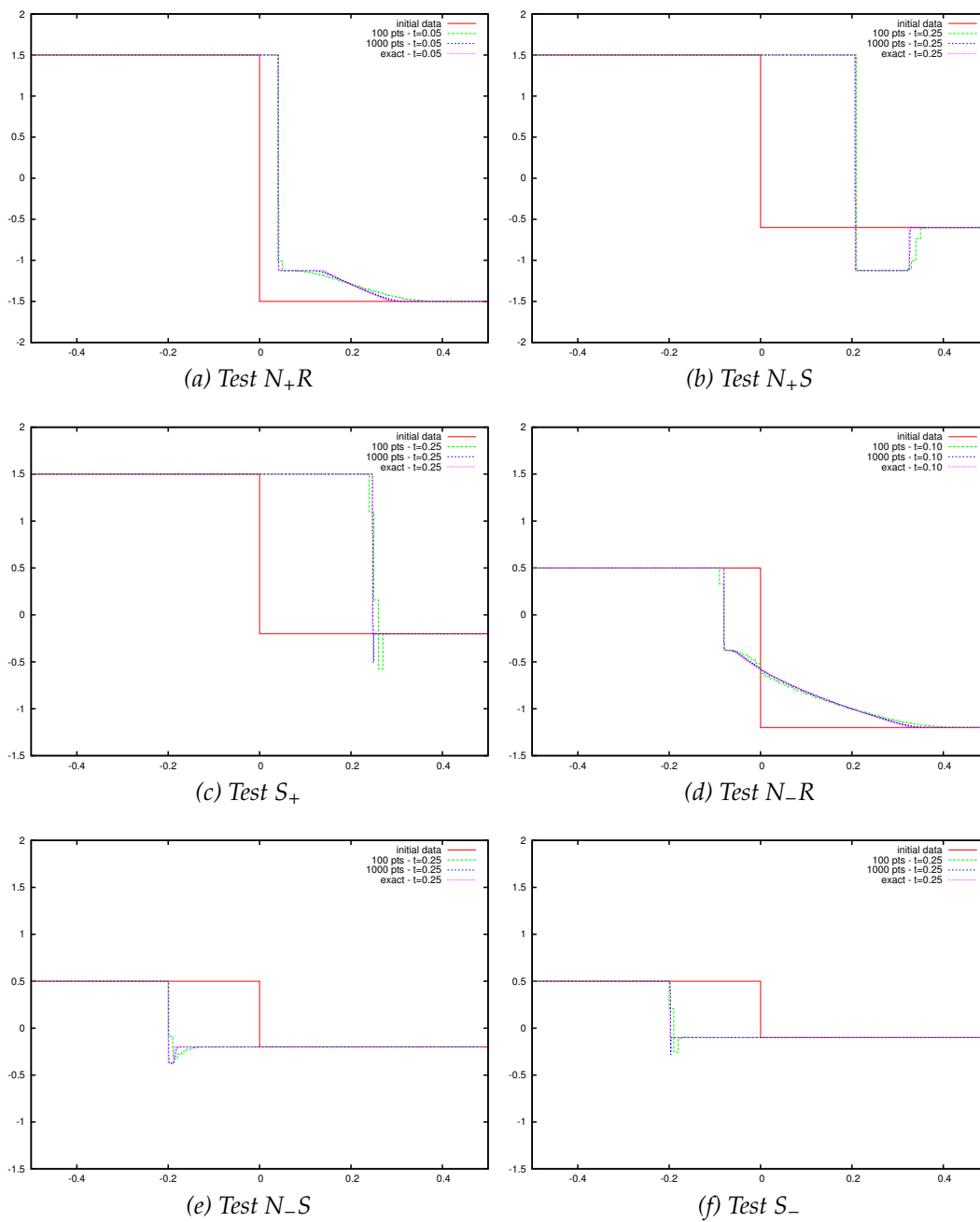
FIGURE 7.5: Problèmes de Riemann non classiques.
