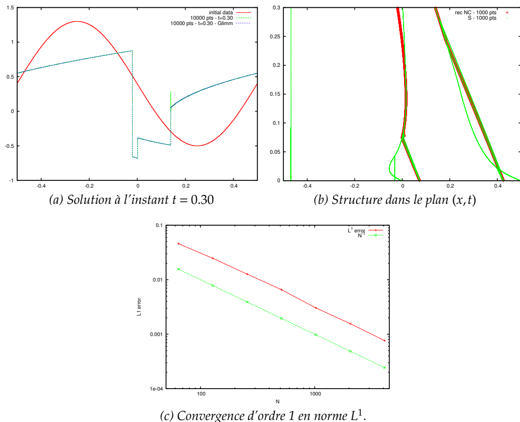
FIGURE 7.8: Problème de Cauchy périodique avec des chocs non classiques.
