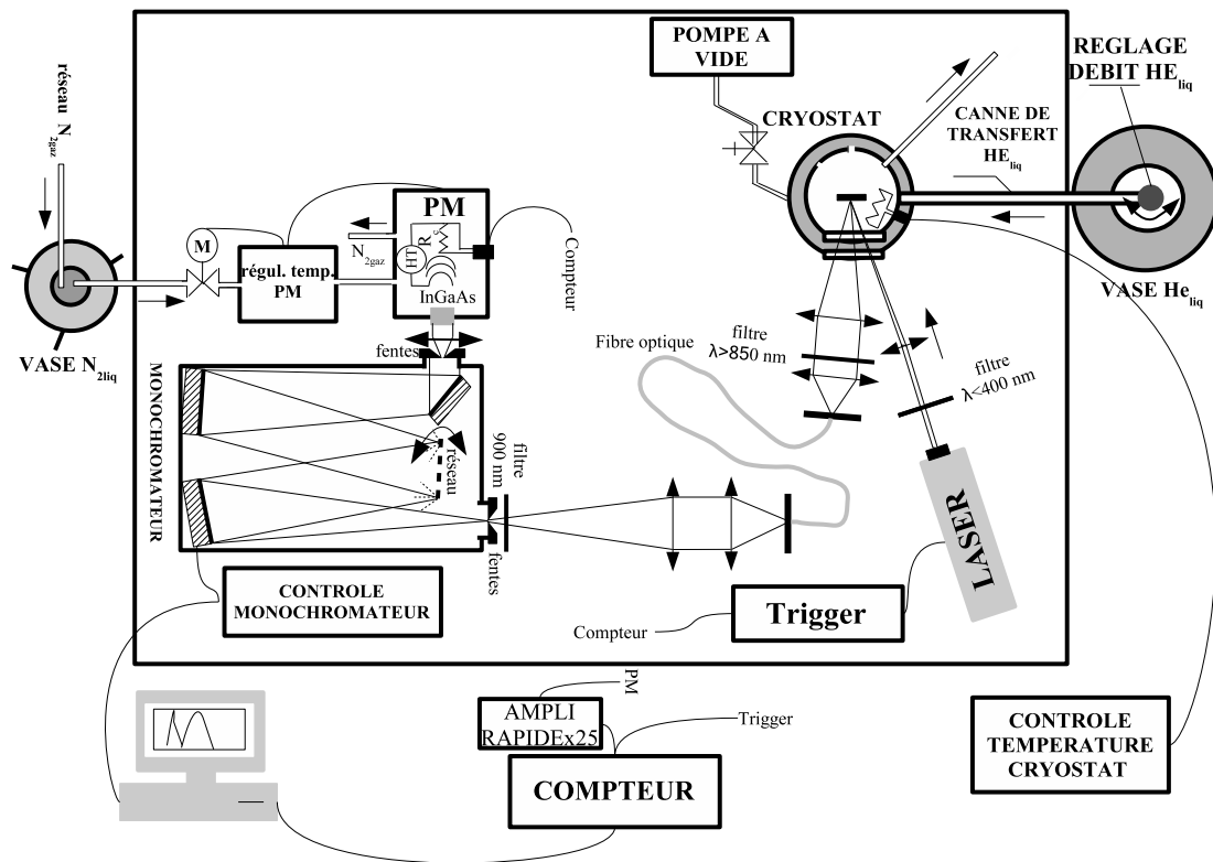
FIG. 2.15 – Montage expérimental de photoluminescence résolue en temps.
