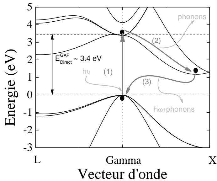
FIG. 2.3 – Représentation d’une expérience de photoluminescence d’un point de vue électronique : (1) un électron de la bande de valence est excité optiquement ( h\nu > 3.43 \text{ eV} ) vers la bande de conduction, (2) l’électron se désexcite par émission de phonons jusqu’au bord de la bande de conduction (en quelques picosecondes [34]), (3) enfin il retourne vers son état fondamental dans la bande de valence avec une émission radiative assistée par l’intervention de phonons.
