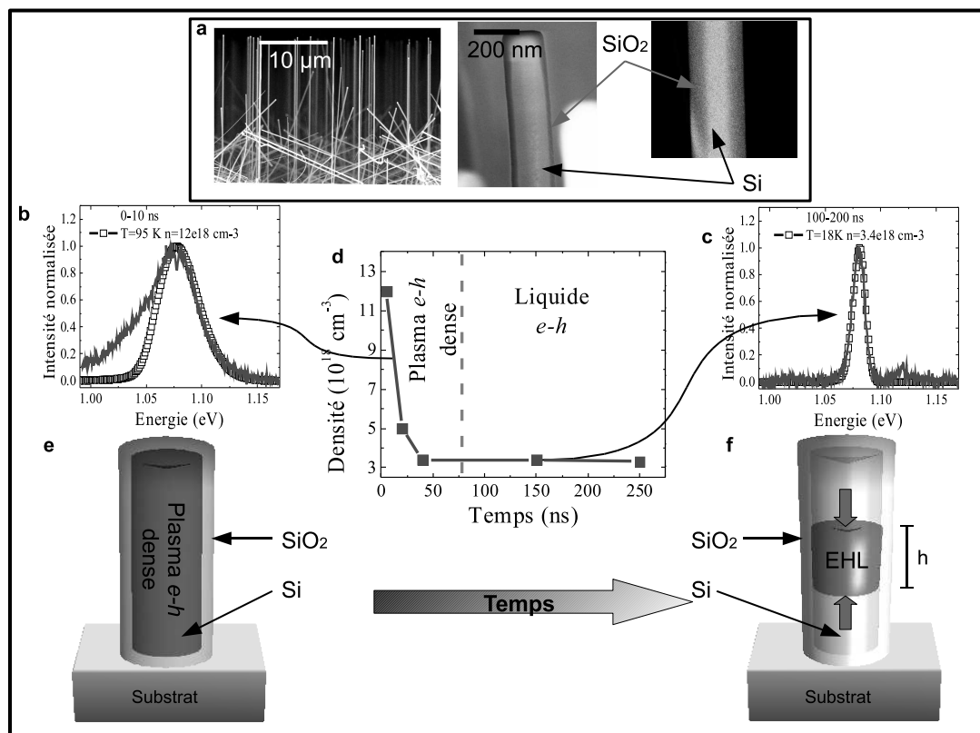
FIG. 3.27 – a Images MEB de nanofils : (gauche) Vue de profil de nanofils de 25 \mu\text{m} de long et de 200 nm de diamètre, (milieu et droite) Nanofils coeur-coquille Si-SiO 2 . b et c : (courbes continues) Spectres résolus en temps acquis sur les fenêtres temporelles : 0–10 ns et 100–200 ns après le pulse laser. (Carrés noirs) Spectres d'émission simulés d'un plasma e-h dont les paramètres sont indiqués en insert. L'ajustement des paramètres du plasma permet de faire coïncider les spectres d'émission simulés avec les spectres expérimentaux pour chaque fenêtre temporelle, et donne accès à l'évolution temporelle de la densité et de la température du plasma e-h . d : Dépendance temporelle de la densité du plasma e-h . Après 50 ns, le système atteint la densité d'un liquide e-h à partir d'où la densité reste constante. e : Représentation schématique du système électronique qui est initialement un plasma dense occupant tout le volume du nanofil. La recombinaison des porteurs engendre une réduction de la densité du plasma jusqu'à atteindre la densité du liquide e-h . f : Ensuite, seul le volume occupé par le liquide e-h décroît au cours du temps.
