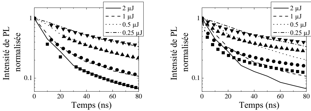
(a) Dynamique de recombinaison des porteurs selon un mécanisme de type Auger assisté par des pièges (symboles) pour différentes puissances d'excitation.
