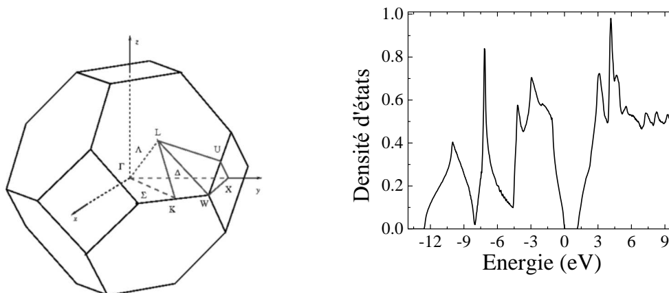
(a) Première zone de Brillouin de la maille cubique face centrée avec les points de hautes symétries.
