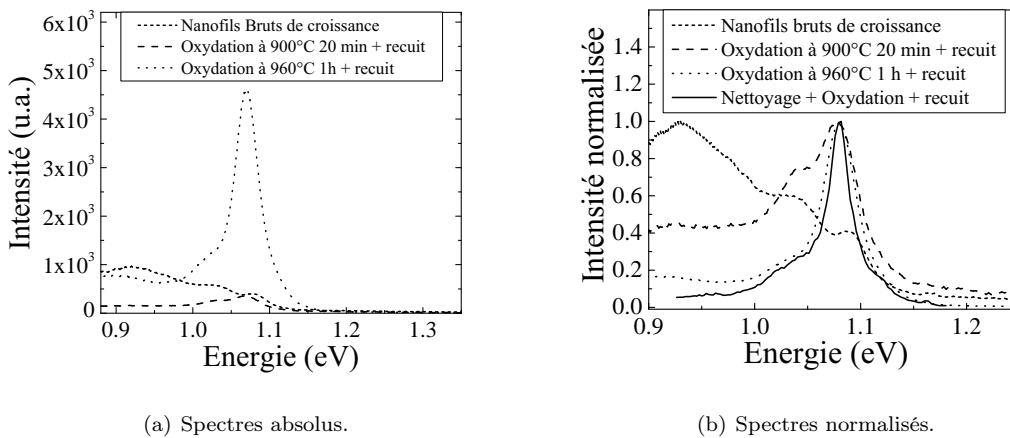
FIG. 3.13 – Spectres de photoluminescence de nanofils bruts de croissance et passivés. Les spectres sont obtenus à 10 K sous une excitation de 3 \cdot 10^4 \text{ W.cm}^{-2} par pulse laser.
