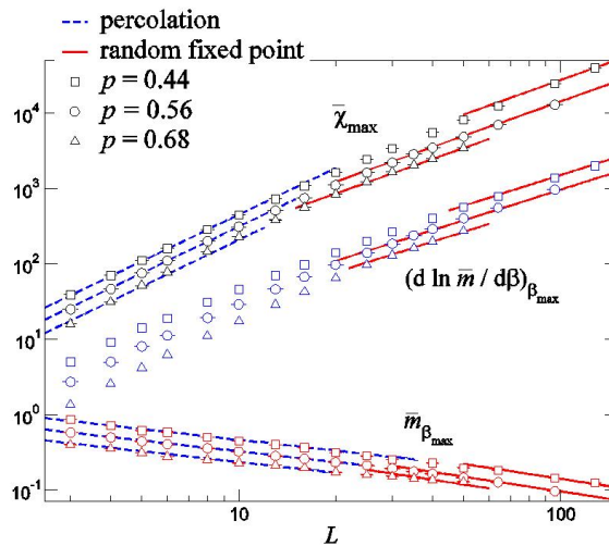
Figure 17. Comportement par effets de taille finie de la susceptibilité, de l'aimantation et de \beta L^{-d} d \ln \overline{m} / d \beta à \beta_{\max} (les grandeurs ont été décalées dans la direction verticale par souci de clarté). Le comportement aux petites tailles du réseau est probablement gouverné par le point fixe de percolation (indiqué par les lignes en tirets et caractérisé par les rapports d'exposants \gamma/\nu \simeq 2,05 et \beta/\nu \simeq 0,475 ). Au-dessus d'une taille de cross-over caractéristique, un nouveau point fixe désordonné est atteint (indiqué par les lignes continues avec les rapports d'exposants \gamma/\nu \simeq 1,535 , 1/\nu \simeq 1,34 et \beta/\nu \simeq 0,73 ).
