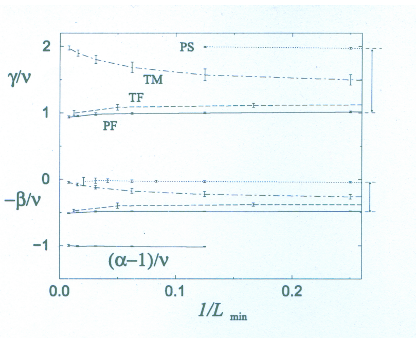
Figure 6. Exposants effectifs dépendant de la taille associés à la susceptibilité, l'aimantation et la différence de densité d'énergie (en pointillés, le système périodique (PS), en points-tirets, la séquence TM, en tirets longs, la séquence TF et en trait continu, la séquence PF) pour r = 5 . Les flèches sur la droite de la figure indiquent la séparation entre les courbes de \gamma/\nu et de -\beta/\nu .
