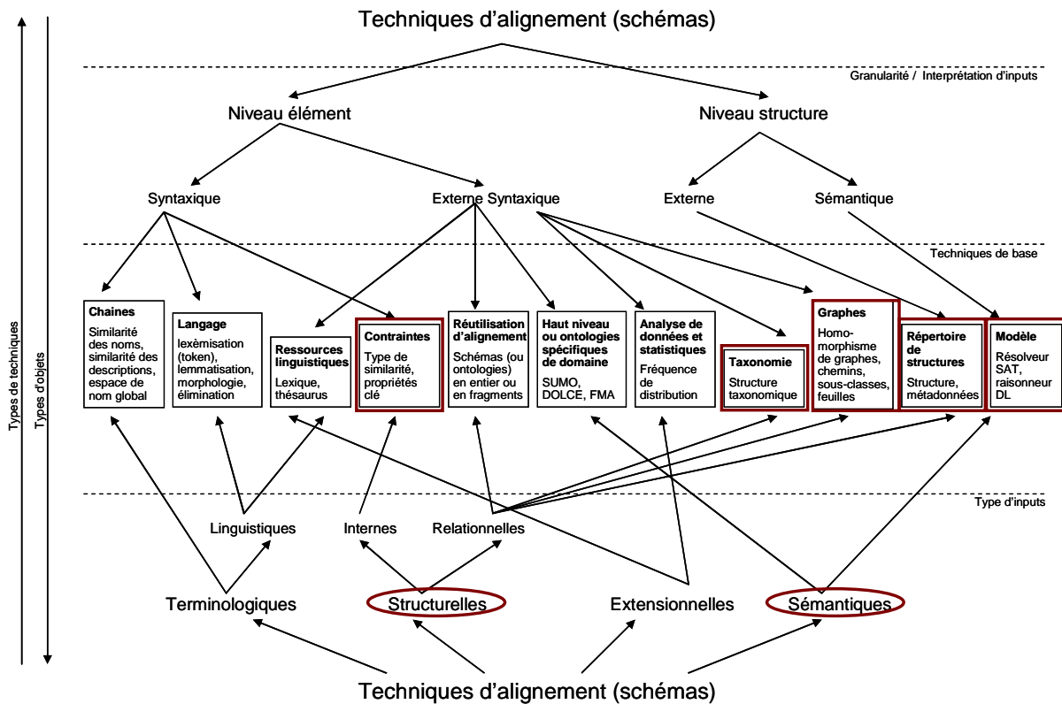
Figure 1. Classification des techniques d'alignement de schémas d'ontologie.
