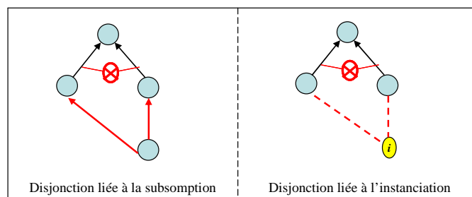
Figure 6. Illustration d'une disjonction liée à une subsumption et d'une disjonction liée à une instanciation.
