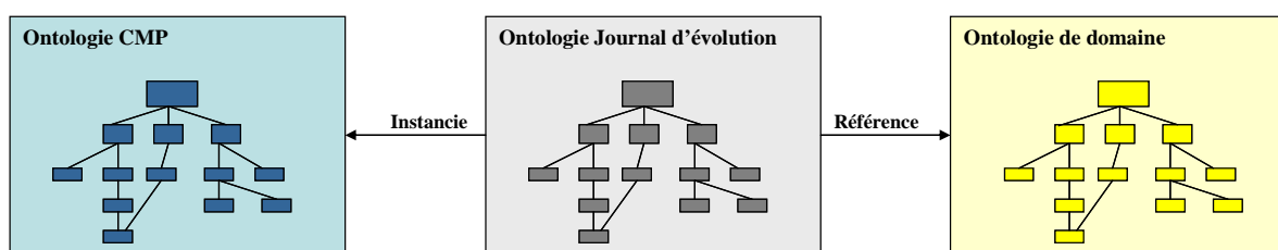
Figure 5. Liens entre l'ontologie journal d'évolution, l'ontologie CMP et l'ontologie de domaine.
