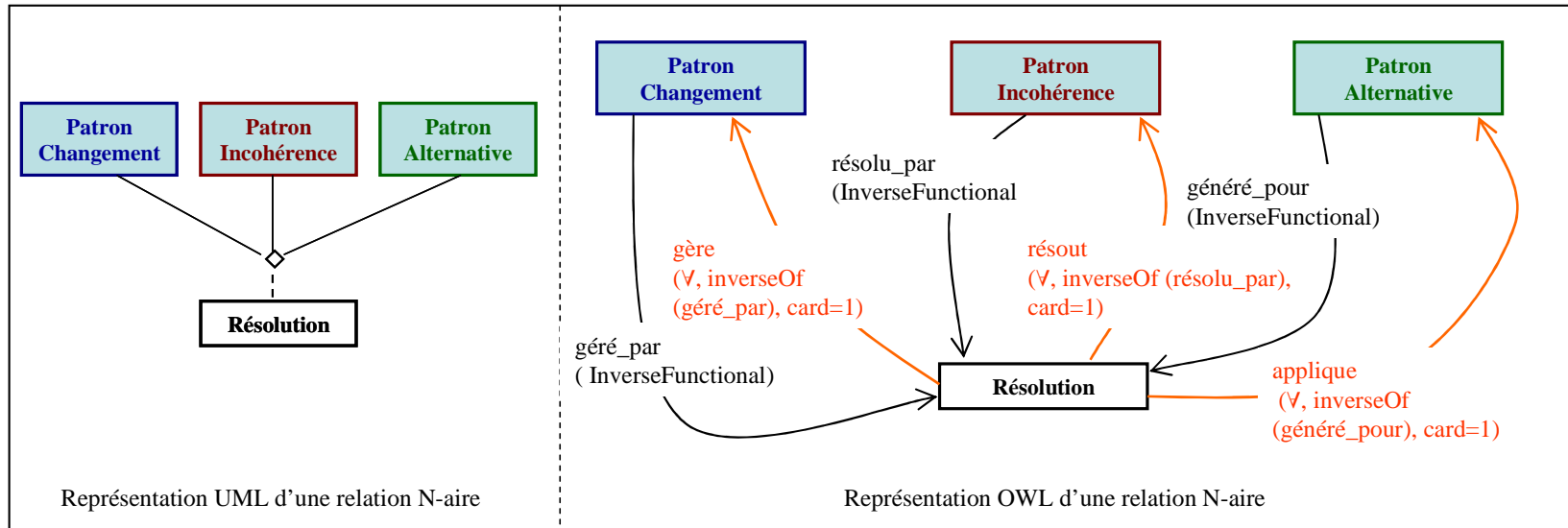
Figure 9. Représentation en UML et en OWL d'une relation N-aire.
