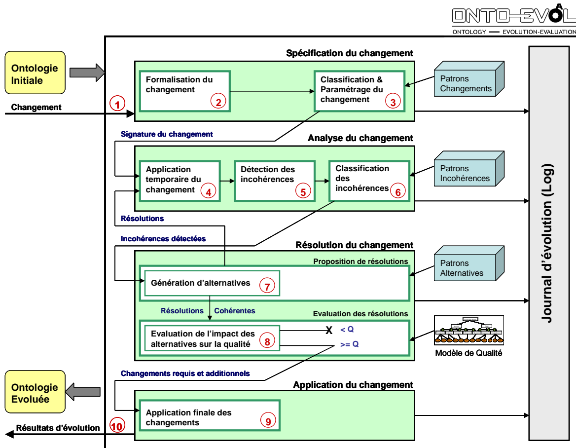
Figure 3. Processus d'évolution de l'approche Onto-Evo al .
