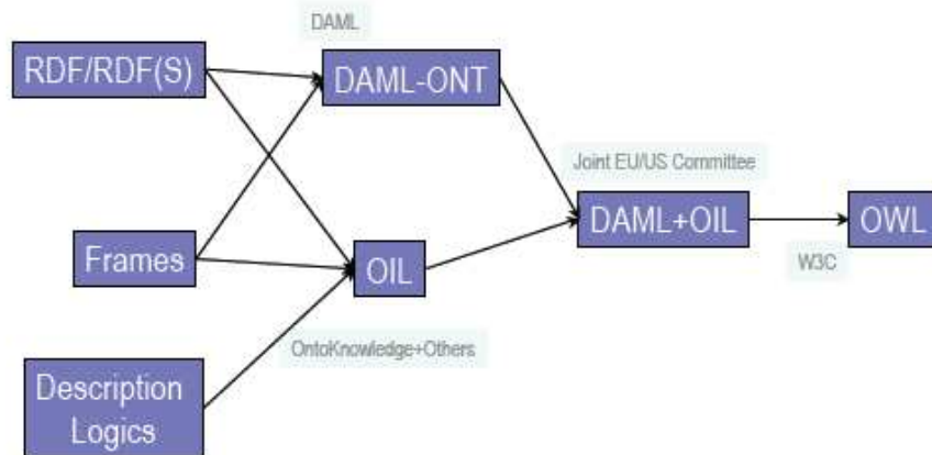
Figure 1. Arborescence de la famille du langage OWL 17 .
