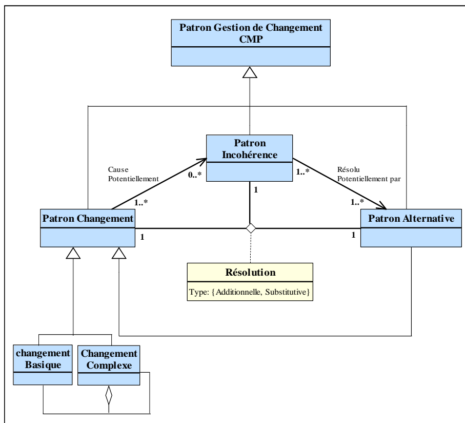
Figure 1. Modèle conceptuel des patrons de gestion de changement CMP.
