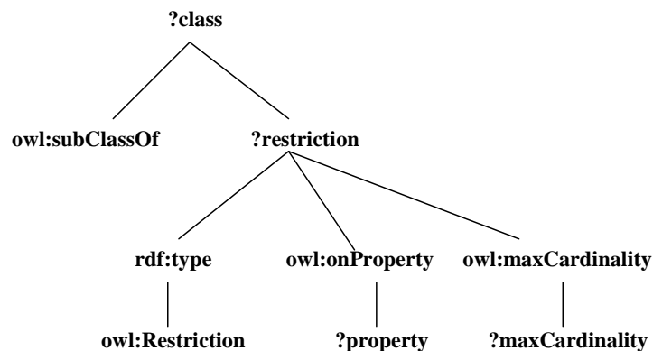
Figure 17. Illustration d'un exemple de patron d'ajout de cardinalité maximale proposé dans (Auer et Herre, 2007).
