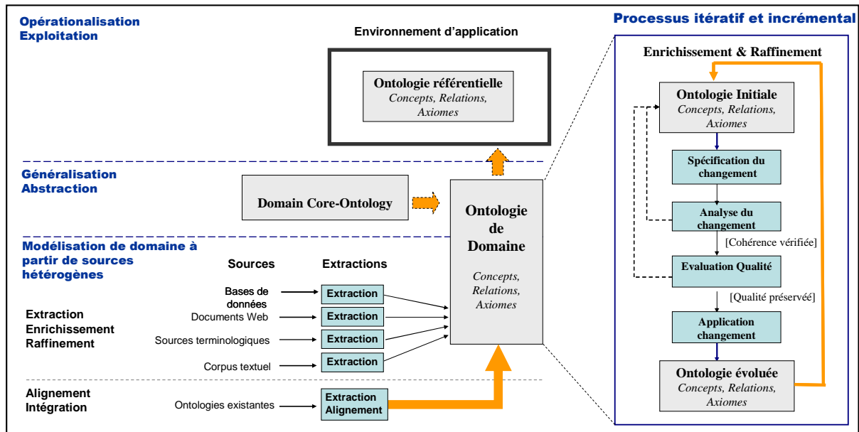
Figure 1. Proposition d'une approche générique de construction d'ontologie à partir de sources hétérogènes.
