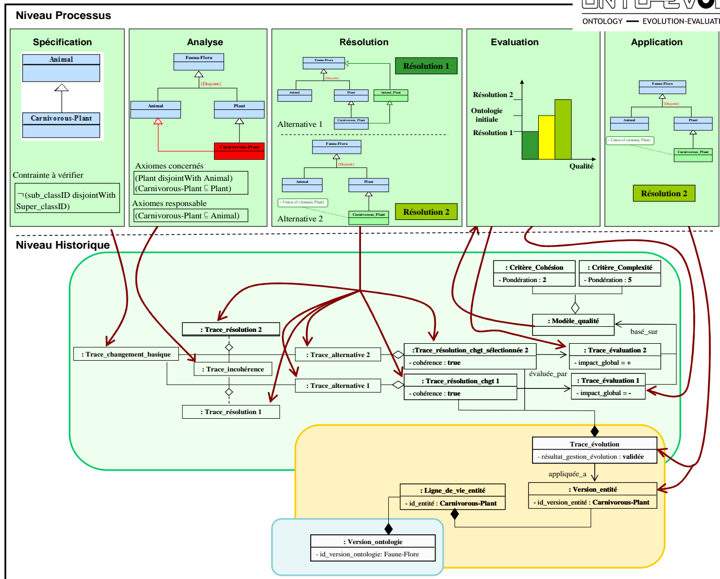
Figure 2. Architecture globale par rapport aux artefacts produits.
