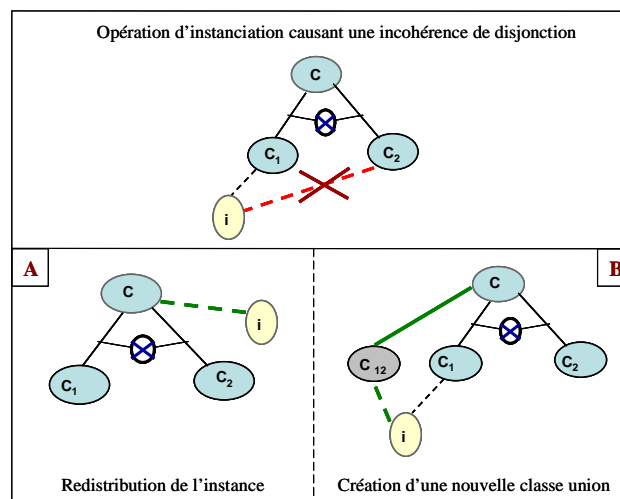
Figure 4. Les alternatives de résolution d'une incohérence de disjonction causée par une instanciation.
