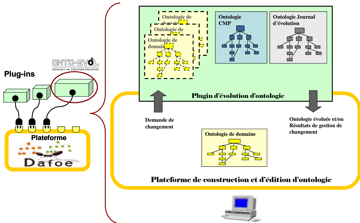
Figure 3. Système d'évolution comme plugin de la plateforme DAFOE.
