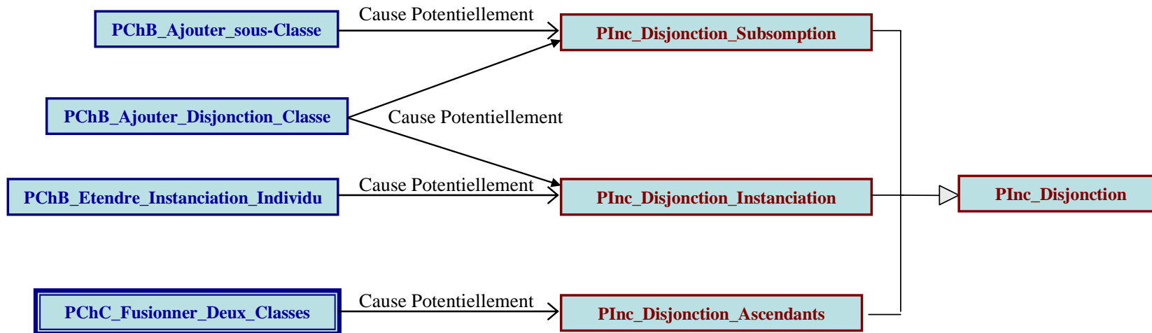
Figure 14. Représentation graphique en UML de la modélisation d'un exemple de patron de d'incohérence de disjonction avec ses spécialisations et les patrons de changements qui leurs sont liés.
