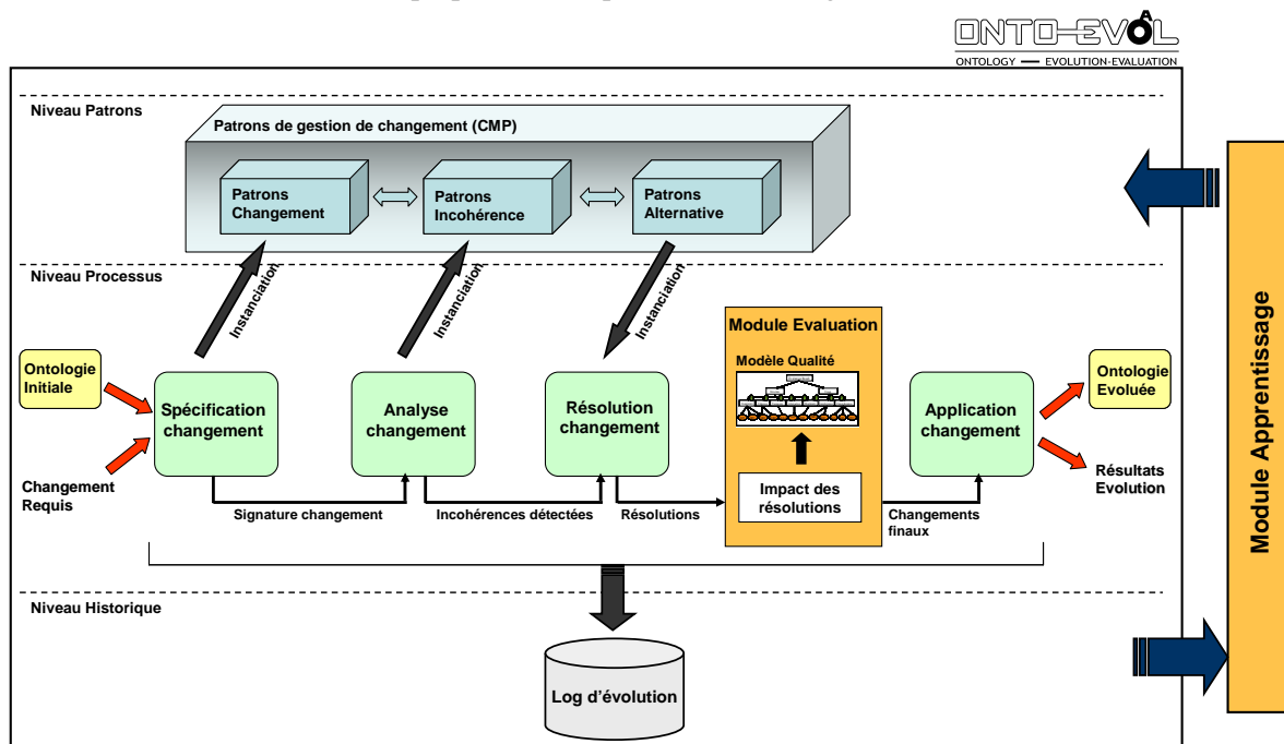
Figure 2. Architecture générale de l'approche Onto-Evo al .
