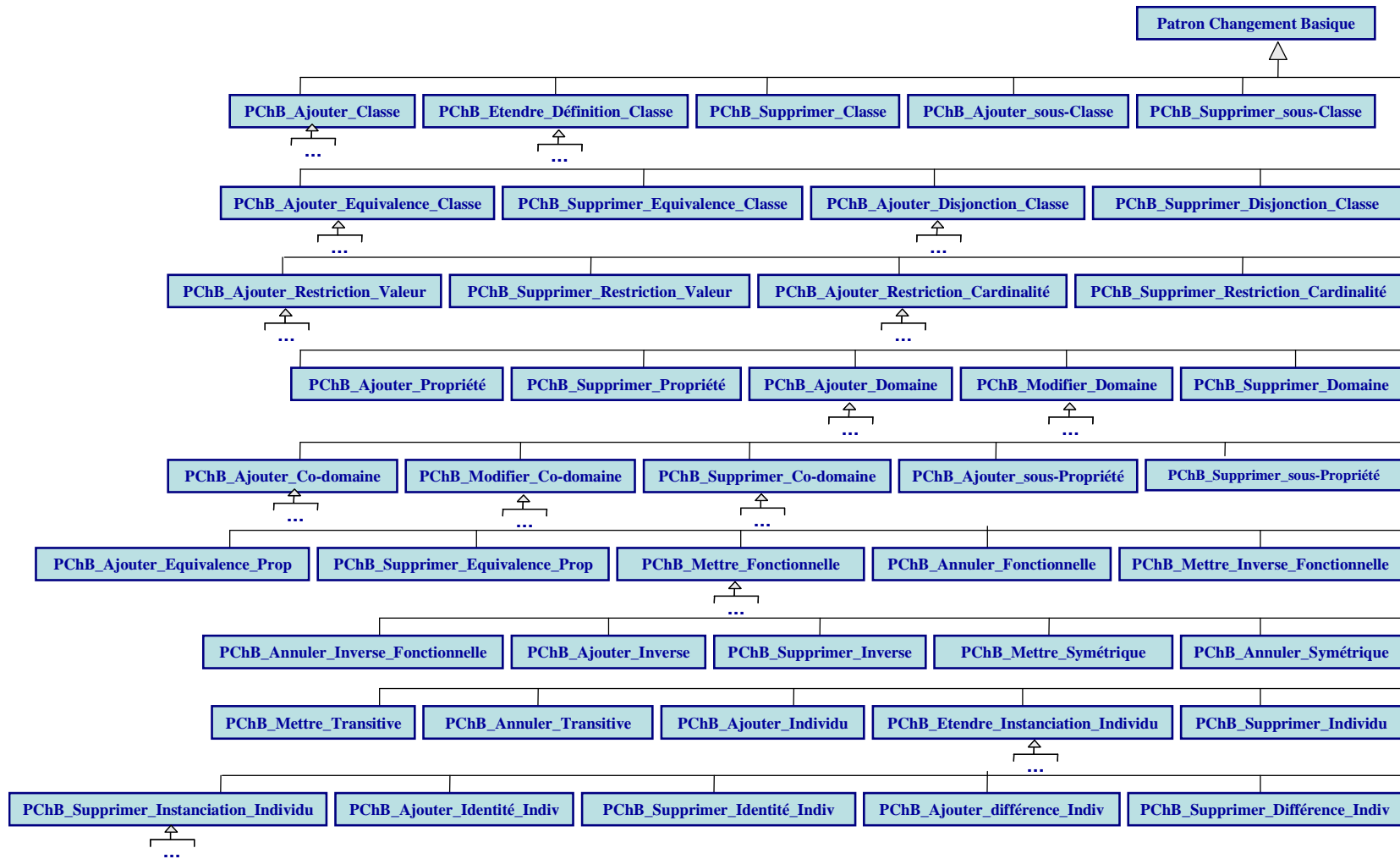
Figure 11. Représentation graphique en UML de la hiérarchie des patrons de changements basiques.
