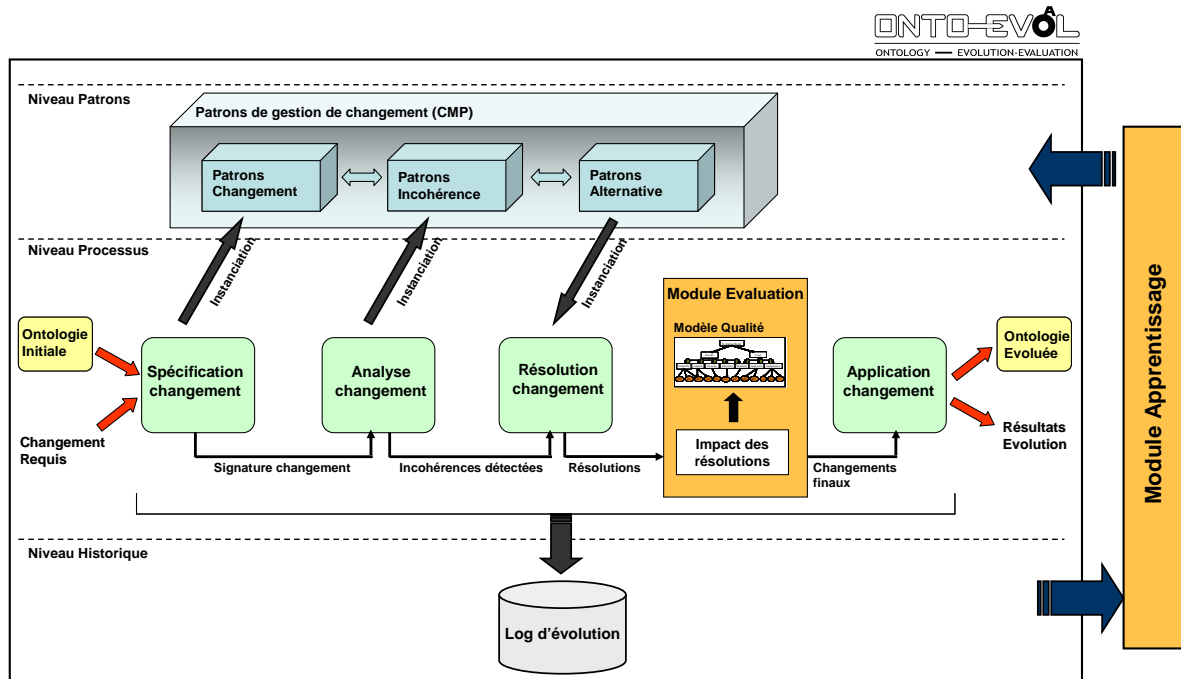
Figure 1. Architecture générale de l'approche Onto-Evo al .
