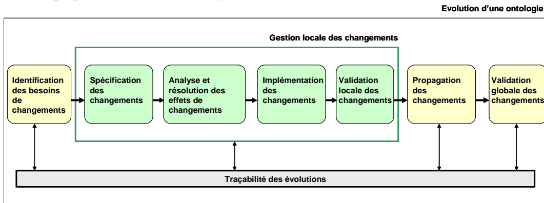
Figure 1. Besoins en évolution d'ontologie.
