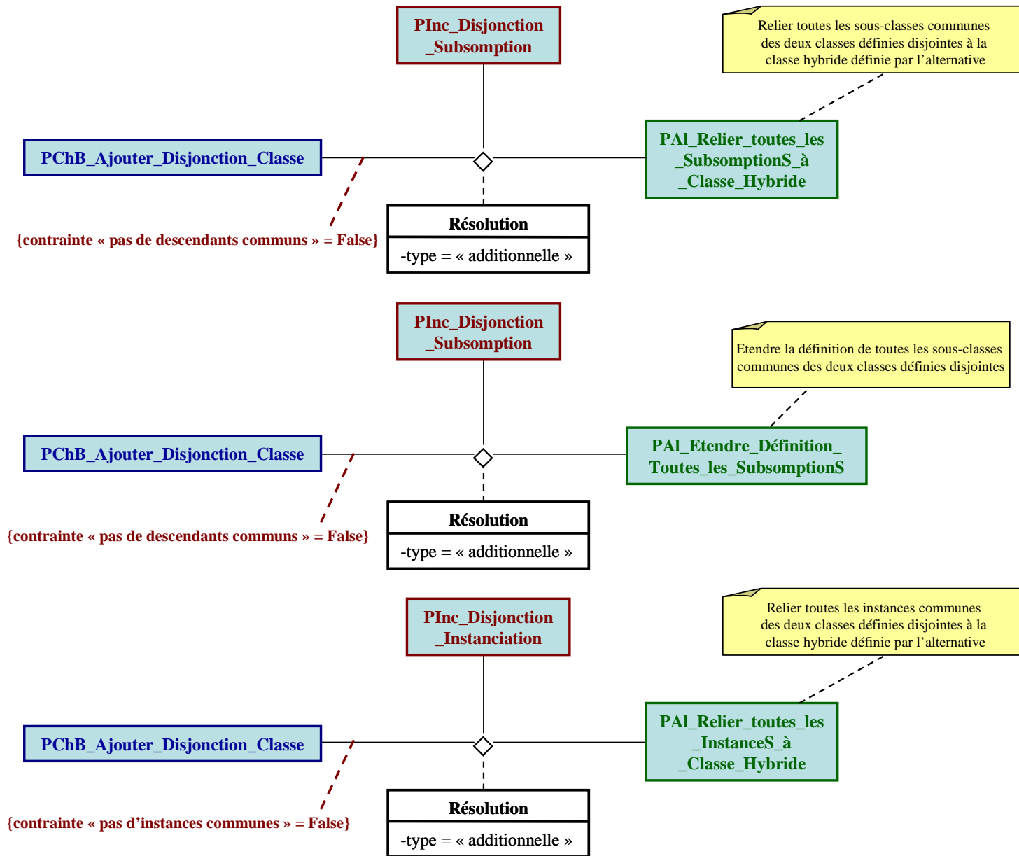
Figure 16. Représentation graphique en UML de la modélisation des résolutions du patron de changement « Ajouter disjonction de classe » pour chacun des patrons d'incohérences qu'il peut causer : « Disjonction de subsumption » et « disjonction d'instanciation ».
