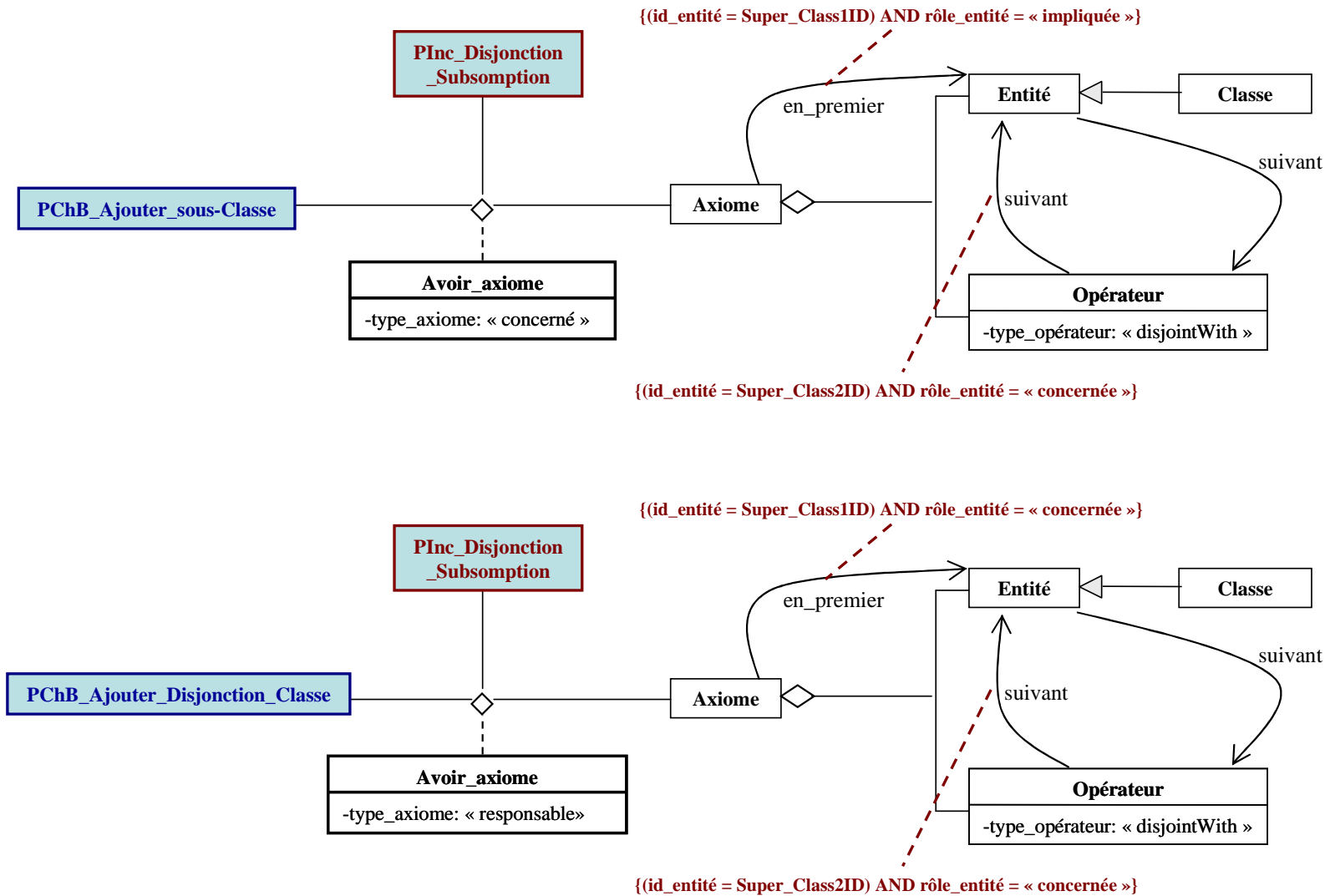
Figure 15. Représentation graphique en UML de la modélisation de la dépendance du type des axiomes des patrons d'incohérences aux changements qui les ont causés et illustration de la description d'un axiome.
