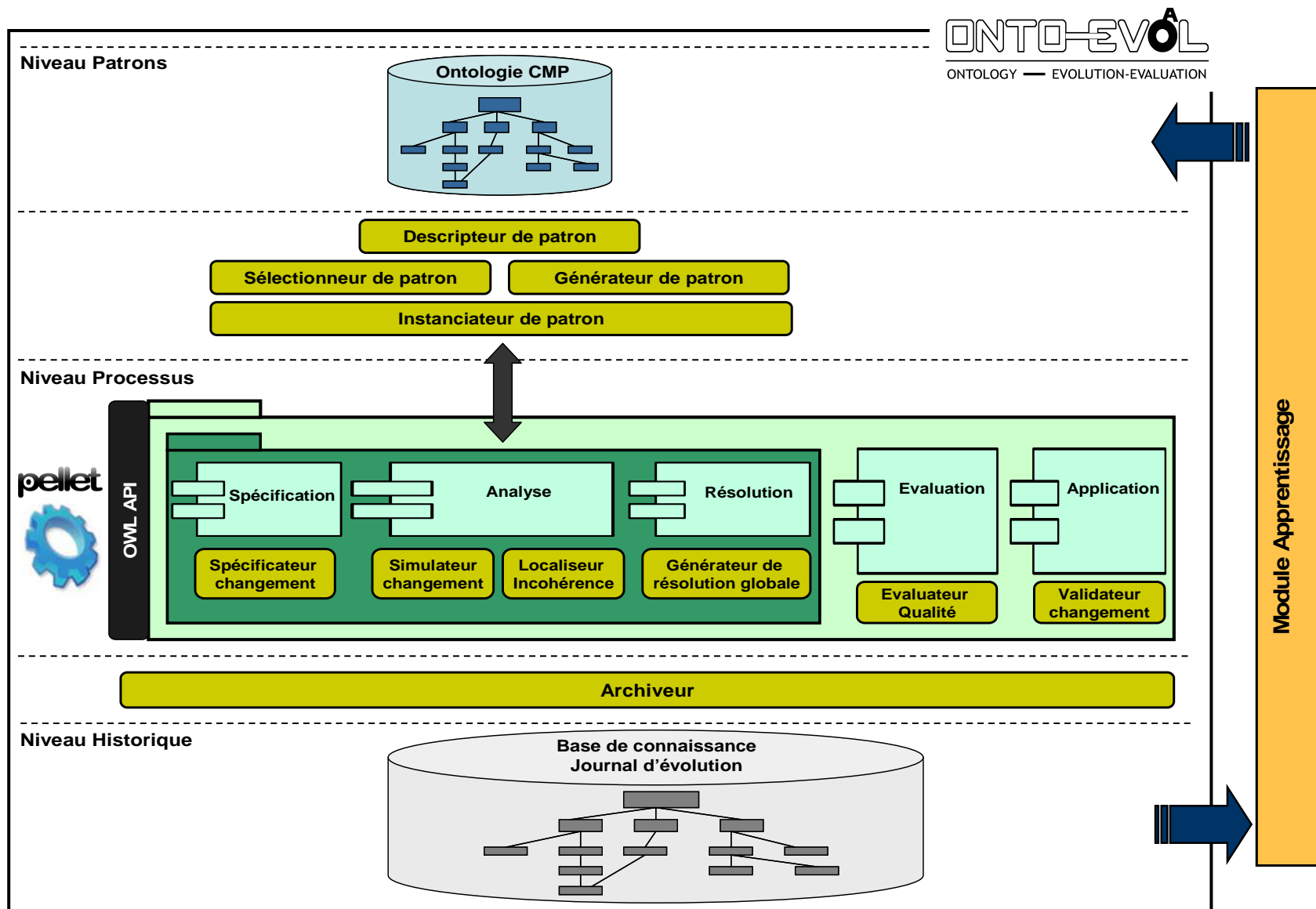
Figure 1. Architecture globale par rapport aux composants logiciels.
