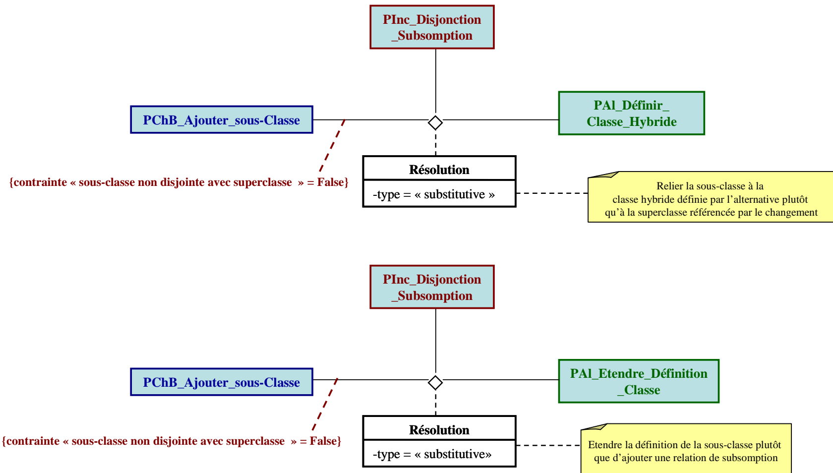
Figure 2. Représentation graphique en UML de la modélisation des résolutions du patron de changement « Ajouter sous-classe » pour le patron d'incohérences qu'il peut causer : « Disjonction de subsumption ».
