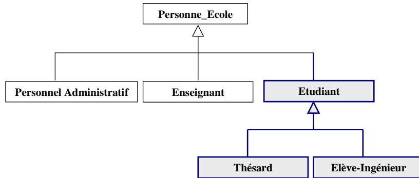
Figure 4. Exemple d'application d'une composition de changement.
