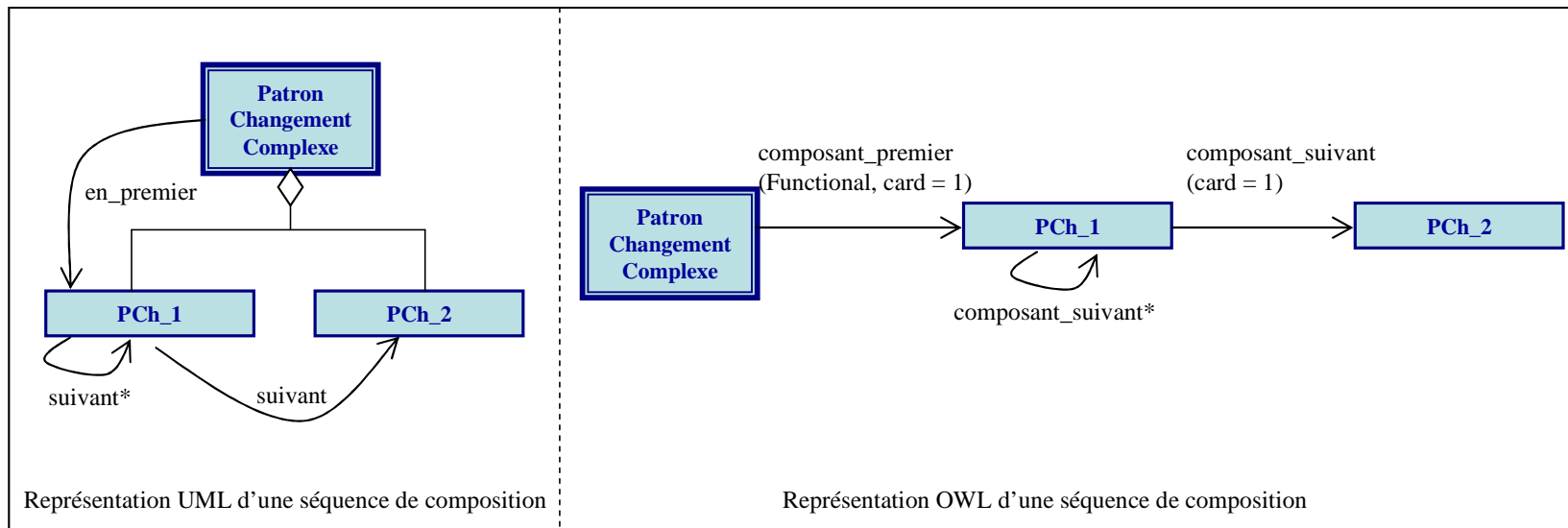
Figure 10. Représentation en UML et en OWL d'une séquence de composition.
