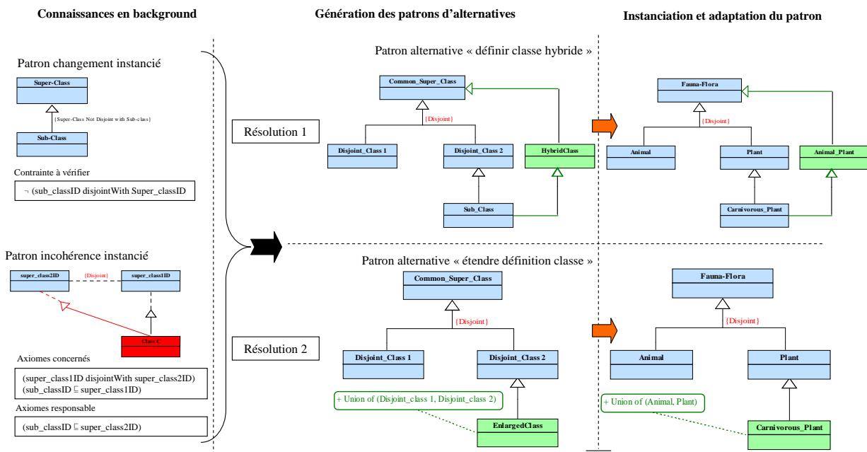
Figure 5. Application d'un patron d'alternatives.
