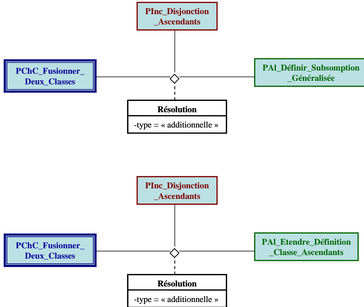
Figure 3. Représentation graphique en UML de la modélisation des résolutions du patron de changement « Fusionner deux classes » pour le patron d'incohérences qu'il peut causer : « Disjonction d'ascendants »
