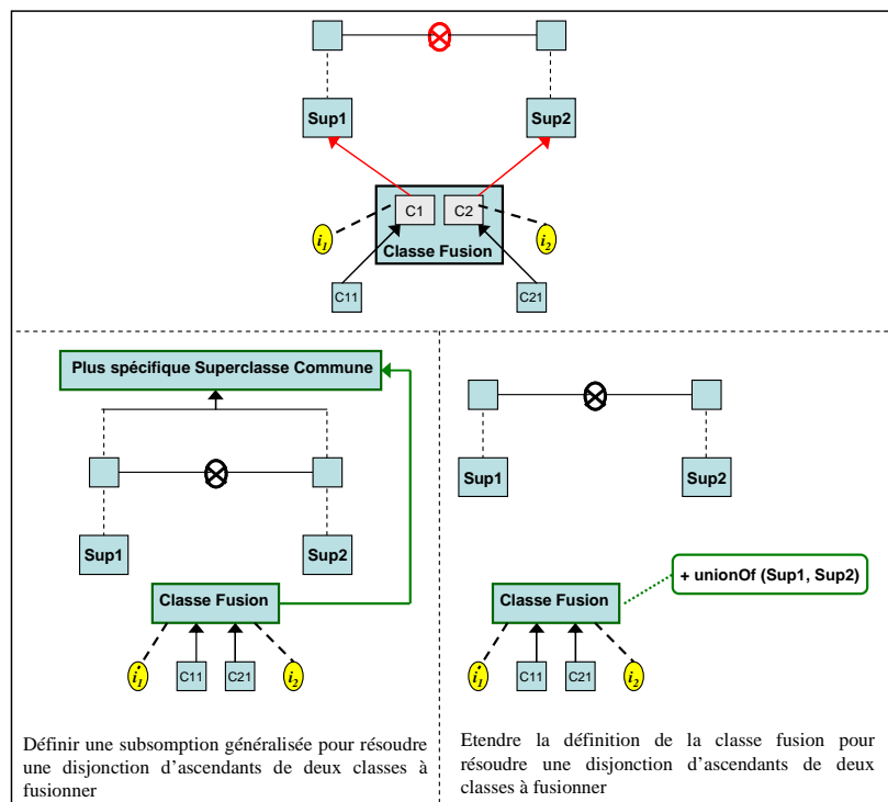
Figure 7. Illustration graphique des patrons de résolution de disjonction d'ascendants due à la fusion de deux classes.
