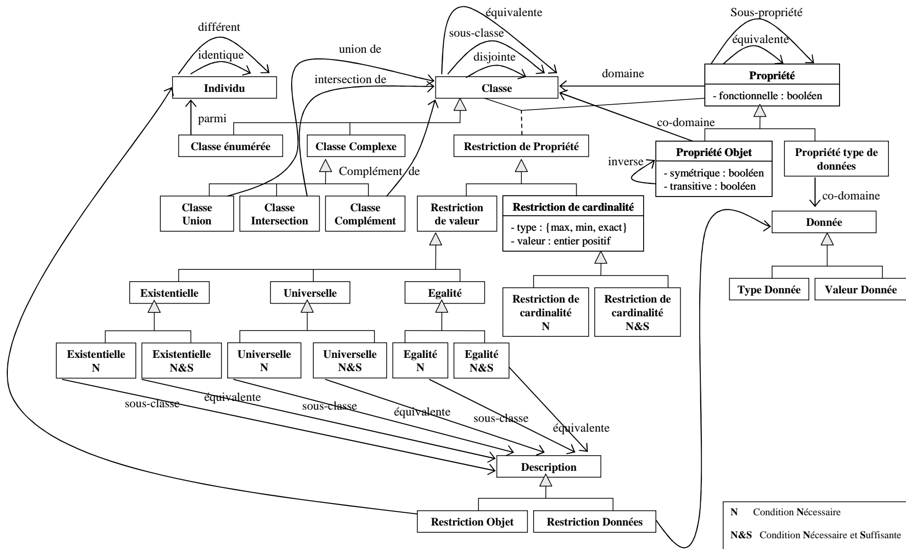
Figure 2. Représentation en UML du méta-modèle OWL.
