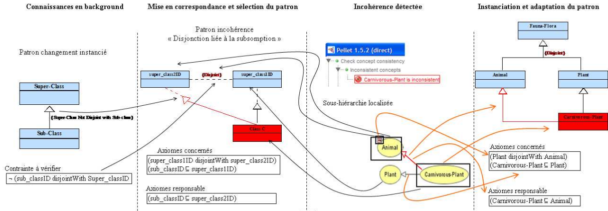
Figure 4. Application d'un patron d'incohérences.
