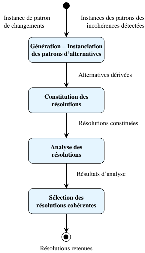
Figure 6. Diagramme d’activités de la procédure de proposition de résolutions.
