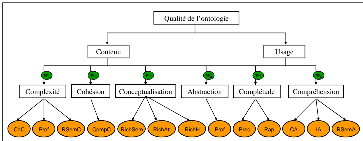
Figure 2. Représentation hiérarchique du modèle de qualité.
