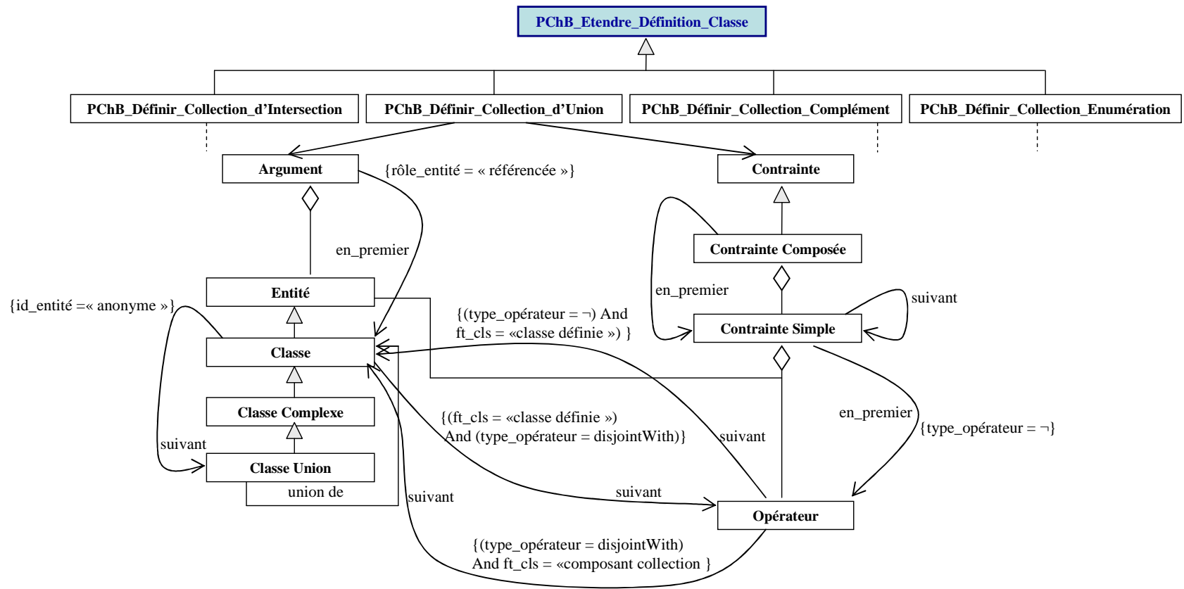
Figure 12. Représentation graphique en UML de la modélisation d'un exemple de patron de changement basique « Etendre la définition d'une classe ».
