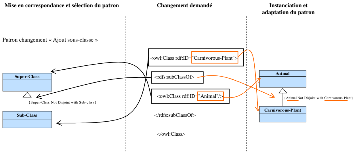
Figure 3. Application d'un patron de changements.
