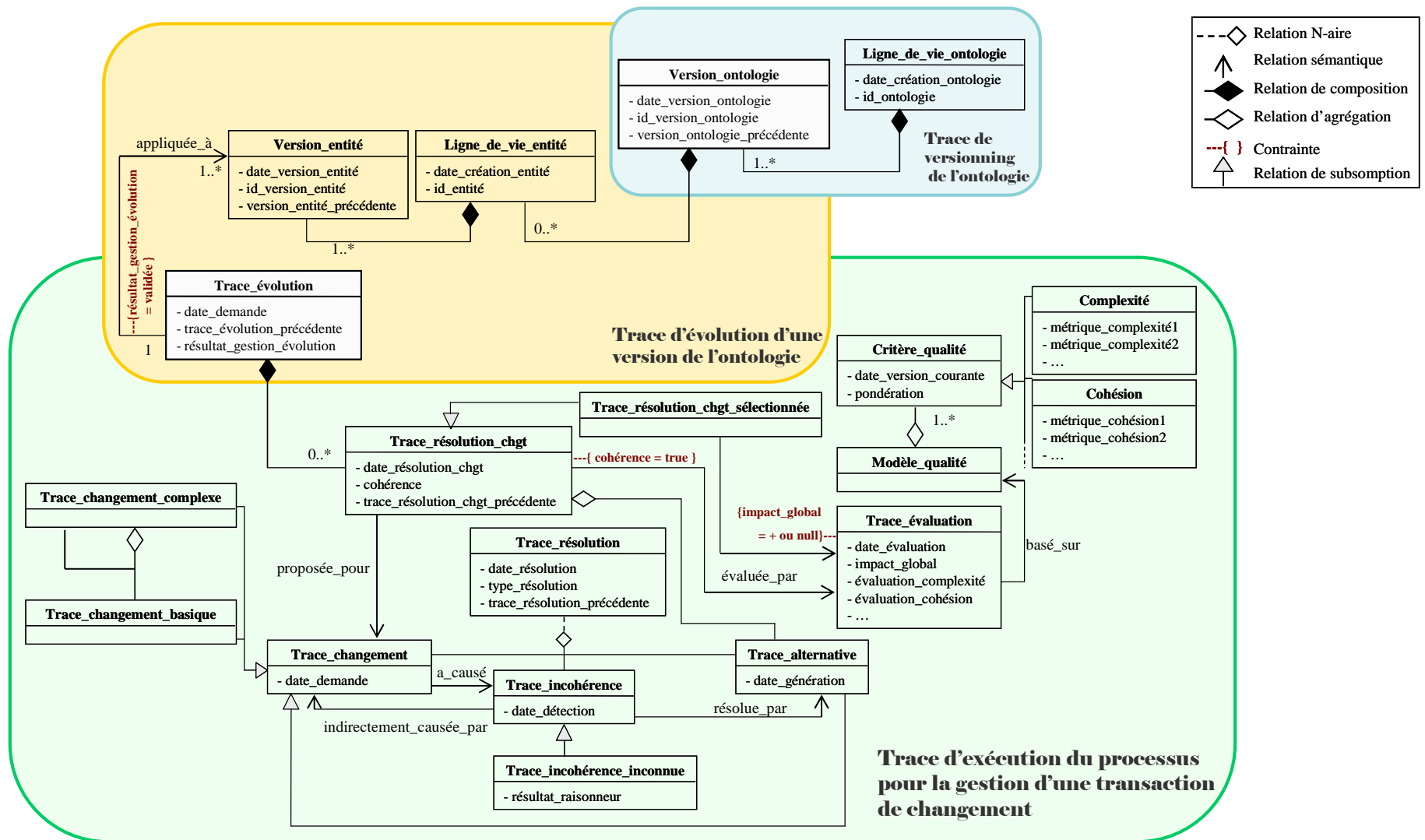
Figure 6. Représentation graphique en UML de l'ontologie journal d'évolution.
