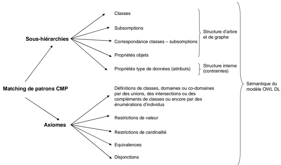
Figure 1. Matching des sous-hiérarchies et des axiomes.
