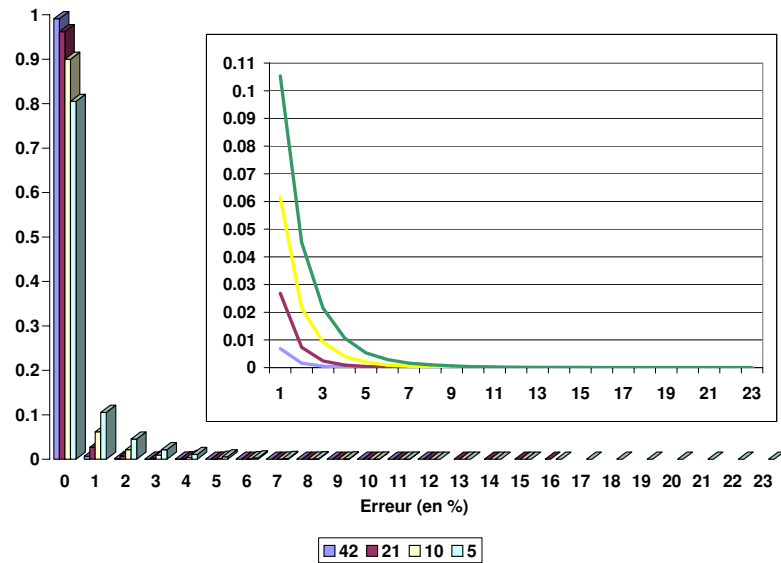
FIG. 4.19: Évaluation de l'erreur d'approximation suite à un rejet de primitives. Moyennes issues de plusieurs points de vue pour l'ensemble SPX . On exprime les erreurs normalisées en pourcentage sur l'axe des abscisses et leur quantité en ordonnée. L'histogramme et les courbes représentent la même chose, les courbes étant à une échelle grossie afin de mettre en valeur les petites erreurs. Les couleurs sont attribuées en fonction de l'appel au rejet des primitives toutes les i fois. On note ainsi que le rejet de primitives détériore peu le rendu final.
