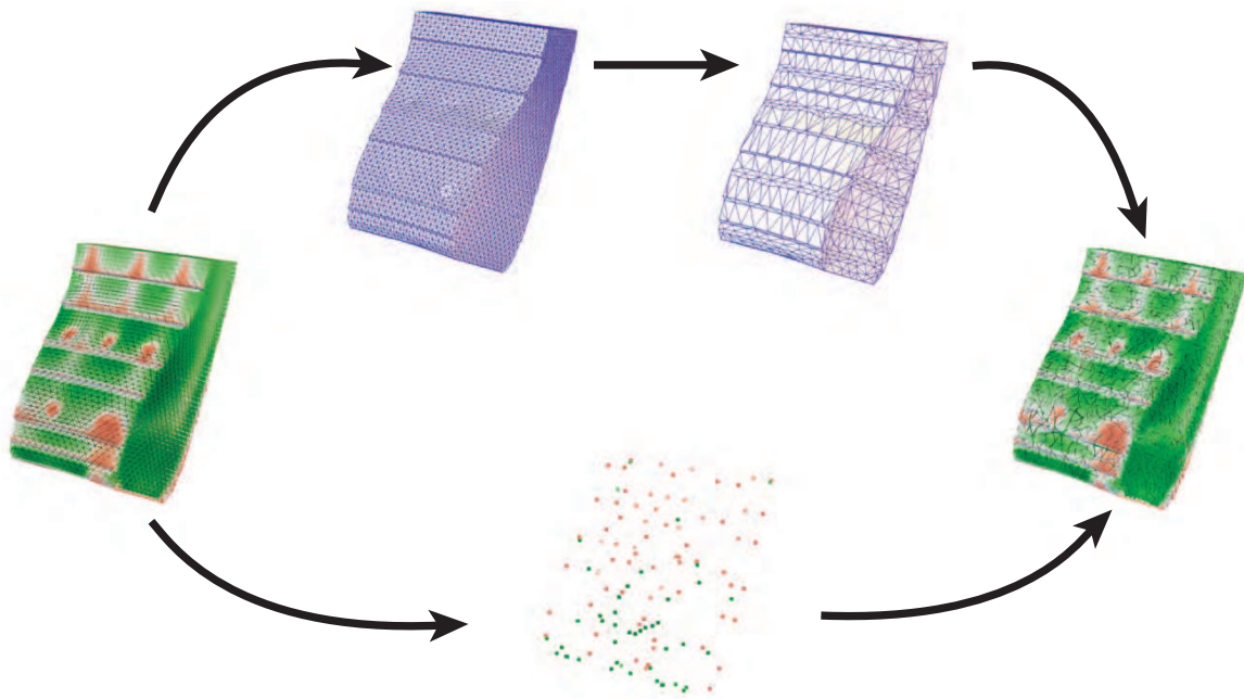
FIG. 2.10: Étapes de la simplification des maillages tétraédriques : Maillage fin à gauche ( Comb : 215\ 040 tétraèdres) représenté en tétraèdres écorchés avec une colorisation en fonction du champ scalaire. Au centre, décomposition du maillage fin en deux sous-ensembles distincts. En haut, extraction de la surface de bord et sa simplification ; en bas, extraction des points critiques. Les points sont coloriés en fonction de leur valeur scalaire. Ces deux ensembles sont utilisés pour générer le maillage grossier de droite via une CDT ( 38\ 115 tétraèdres).
