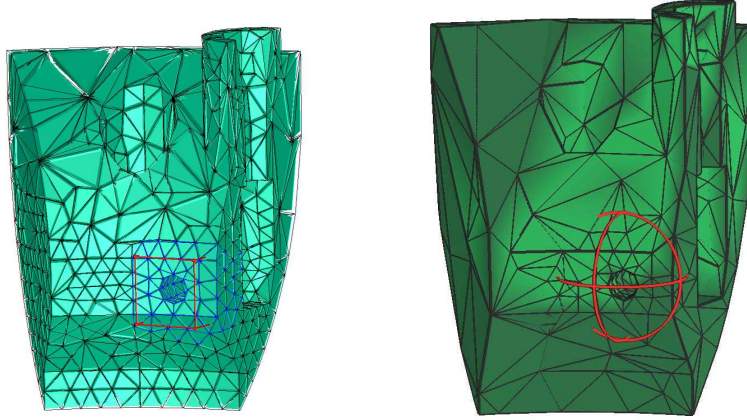
FIG. 3.5: Localité de l'extraction. À gauche en utilisant MT [CDFM + 04]. À droite avec notre méthode BiRes . Contrairement aux précédentes approches multirésolution, notre raffinement est guidé par le maillage grossier et non par les dépendances entre les opérations locales de décimation. Il en résulte que la région fine extraite est plus localisée par rapport à la définition de la boule d'intérêt.
