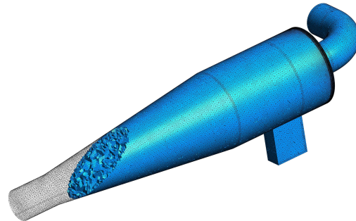
FIG. 1.4: Maillage hexaédrique pour la simulation de gaz (Fourni par John F. Porter). Lors de l'évaluation de la faisabilité de la construction d'une centrale électrique basée sur la combustion des déchets, le cyclone séparateur entre le gaz et les particules néfastes qu'il véhicule est étudié via la simulation de la loi de Stokes. Le maillage va permettre de valider le comportement du gaz sale arrivant par l'entrée rectangulaire, son échappement par le tuyau incurvé alors que les particules seront rejetées par l'autre extrémité [CPHM04]. Il a été généré via l'outil GMSH .
