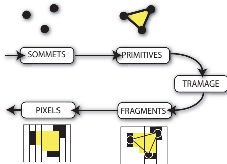
FIG. 1.15: Pipeline graphique. Le pipeline graphique est composé essentiellement de cinq phases. La première considère les sommets individuellement, la deuxième construit les primitives géométriques sous forme de lignes ou de triangles, la troisième est le tramage (ou rasterisation ) convertissant la géométrie en fragments (pixels tridimensionnels), la quatrième effectue les opérations de colorisation, de textures et de profondeur au niveau des fragments, enfin la cinquième affiche les pixels à l'écran.
