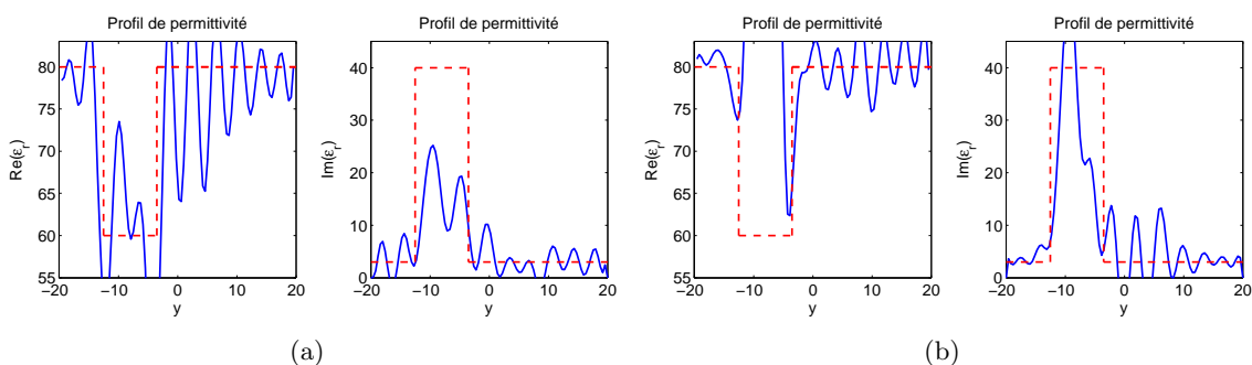
FIG. 4.15 – Comparaison des profils pour différentes erreurs sur la partie réelle de la permittivité de l'eau. La figure (a) représente l'inversion pour une estimation \mathcal{Re}(\varepsilon_r) = 79 et (b) pour une estimation \mathcal{Re}(\varepsilon_r) = 81 , la partie imaginaire étant supposée parfaitement connue.
