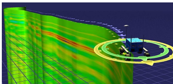
FIG. 1.2 – Simulation de reconstruction d'une structure de sous-sol à partir d'un sondage avec un GPR.
