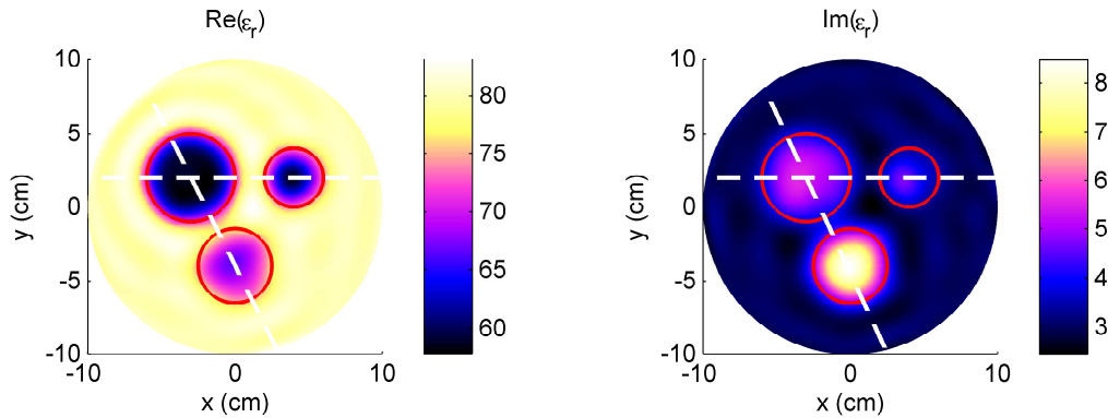
FIG. 4.10 – Carte de permittivité relative de l'inversion de données synthétiques issues de la diffraction de trois tubes diélectriques plongés dans de l'eau. À gauche, nous représentons la partie réelle, à droite, la partie imaginaire. Les cercles rouges représentent les positions exactes des tubes, les pointillés représentent les axes que nous choisissons pour comparer les profils.
