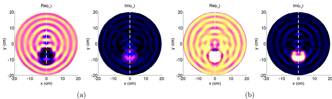
FIG. 4.14 – Comparaison des cartes de permittivité pour différentes erreurs sur la partie réelle de la permittivité de l'eau. La figure (a) représente l'inversion pour une estimation \mathcal{Re}(\varepsilon_r) = 79 et (b) pour une estimation \mathcal{Re}(\varepsilon_r) = 81 , la partie imaginaire étant supposée parfaitement connue.
