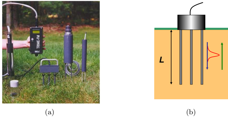
FIG. 1.1 – Exemple de sondes TDR
