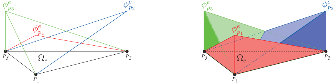
FIG. 2.4 – Fonctions de base sur une maille élémentaire \Omega_e de \Omega .
