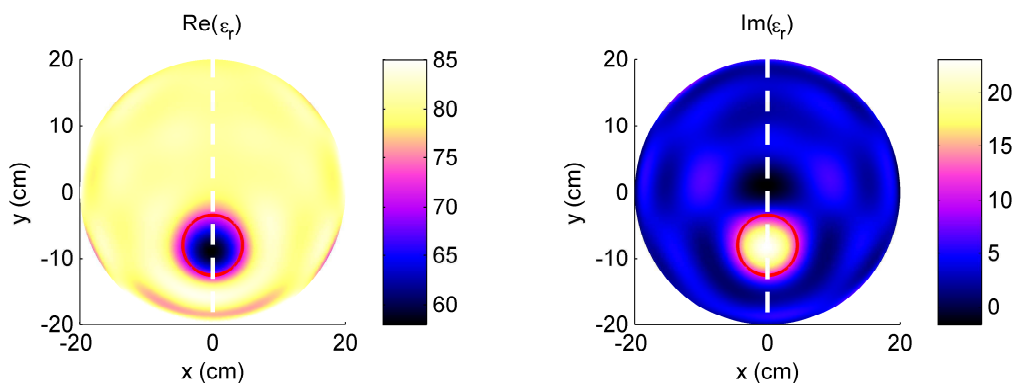
FIG. 6.5 – Carte de la permittivité reconstruite pour des données issues du scanner circulaire, en utilisant une projection d'ordre 10 sur la base de Zernike . (a) et (b) représentent respectivement la partie réelle et la partie imaginaire de la permittivité.
