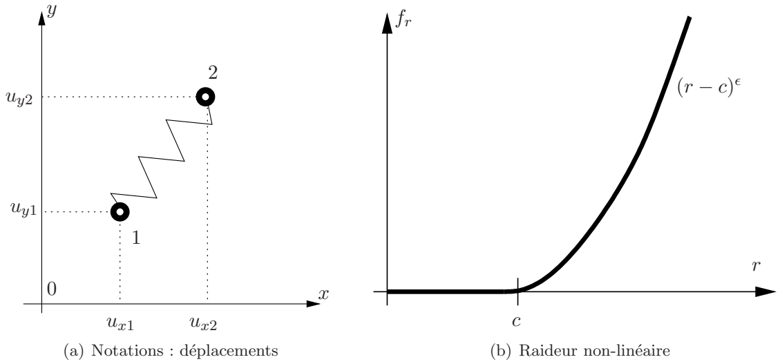
FIG. 2.14 – Elément de raideur radiale non-linéaire axisymétrique
