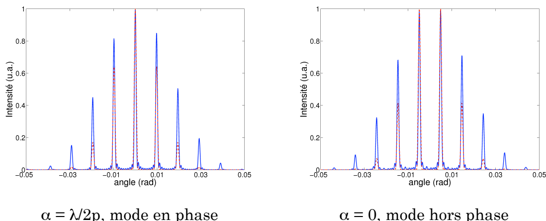
Figure II-25 : Profils en champ lointain des modes hors phase et en phase (bleu) comparés avec les profils théoriques de l'équation (II-12) obtenus avec des émetteurs gaussiens de largeur 2w = 30 \mu\text{m} (pointillés rouges) – I = 3,8 \text{ A} ( = 3,2 \times I_{\text{seuil}} ), R = 40\% , 2L_{\text{ext}} = Z_T/2 .
