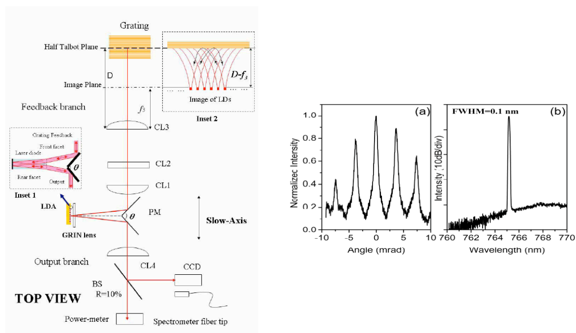
Figure I-37 – gauche : schéma expérimental de la cavité réalisée par [Liu 08] droite : Profil en champ lointain et spectre d'émission en fonctionnement cohérent – I = 50 A, P = 9 W.
