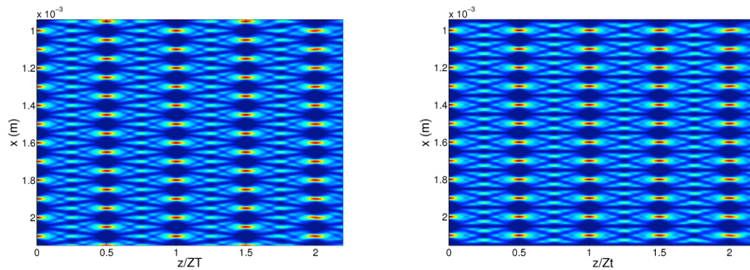
Figure I-33 : Carte d'intensité de la propagation du mode en phase (gauche) et du mode hors phase (droite).
