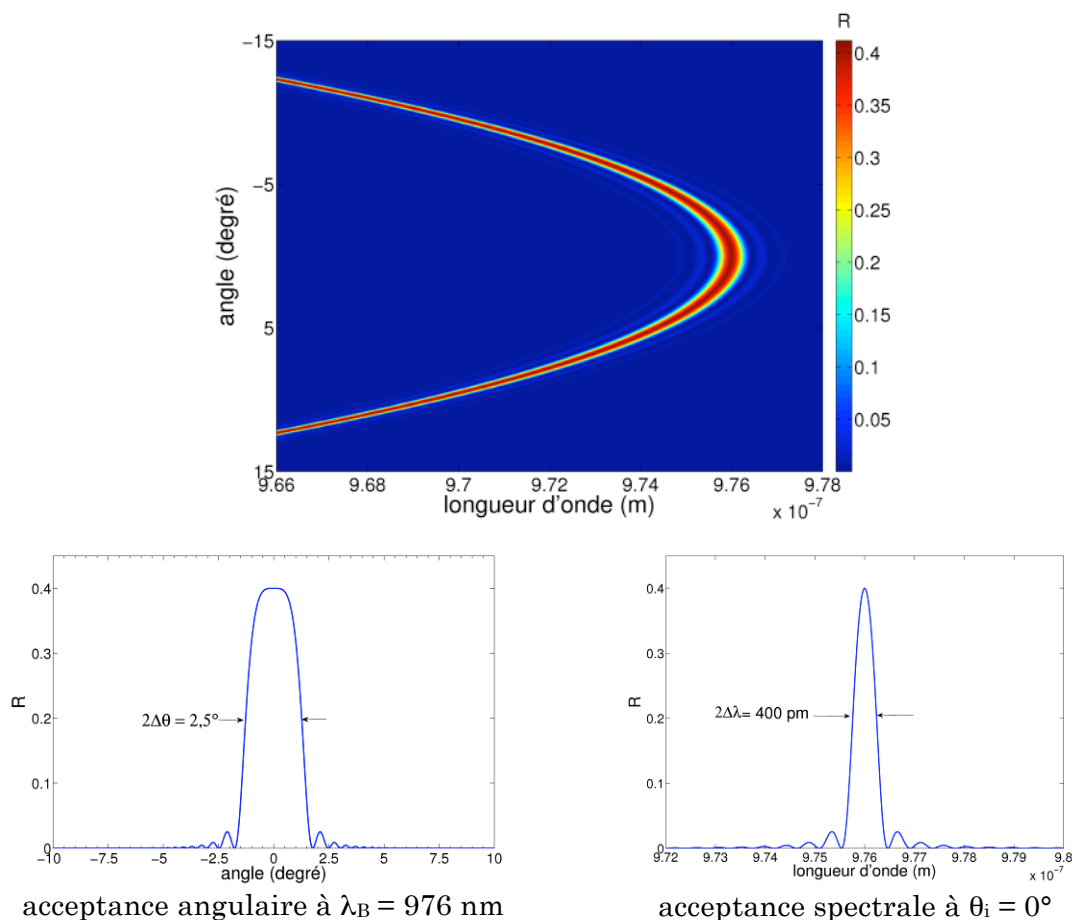
Figure II-3 : Efficacité de diffraction d'un réseau de Bragg en réflexion (caractéristiques données dans le Tableau II-1) et mise en évidence des acceptances angulaire (bas – gauche) et spectrale (bas – droite)
