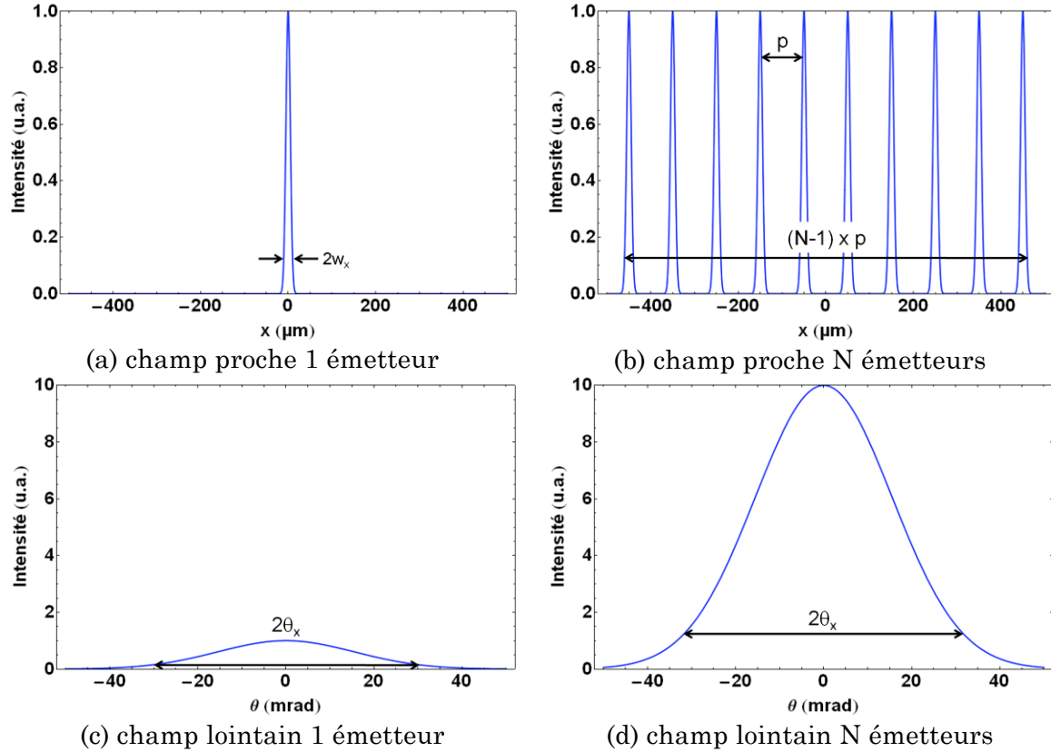
Figure I-17 : Comparaison des profils en champ proche et champ lointain d'une diode laser seule et d'une barrette de N diodes laser de même puissance espacées
