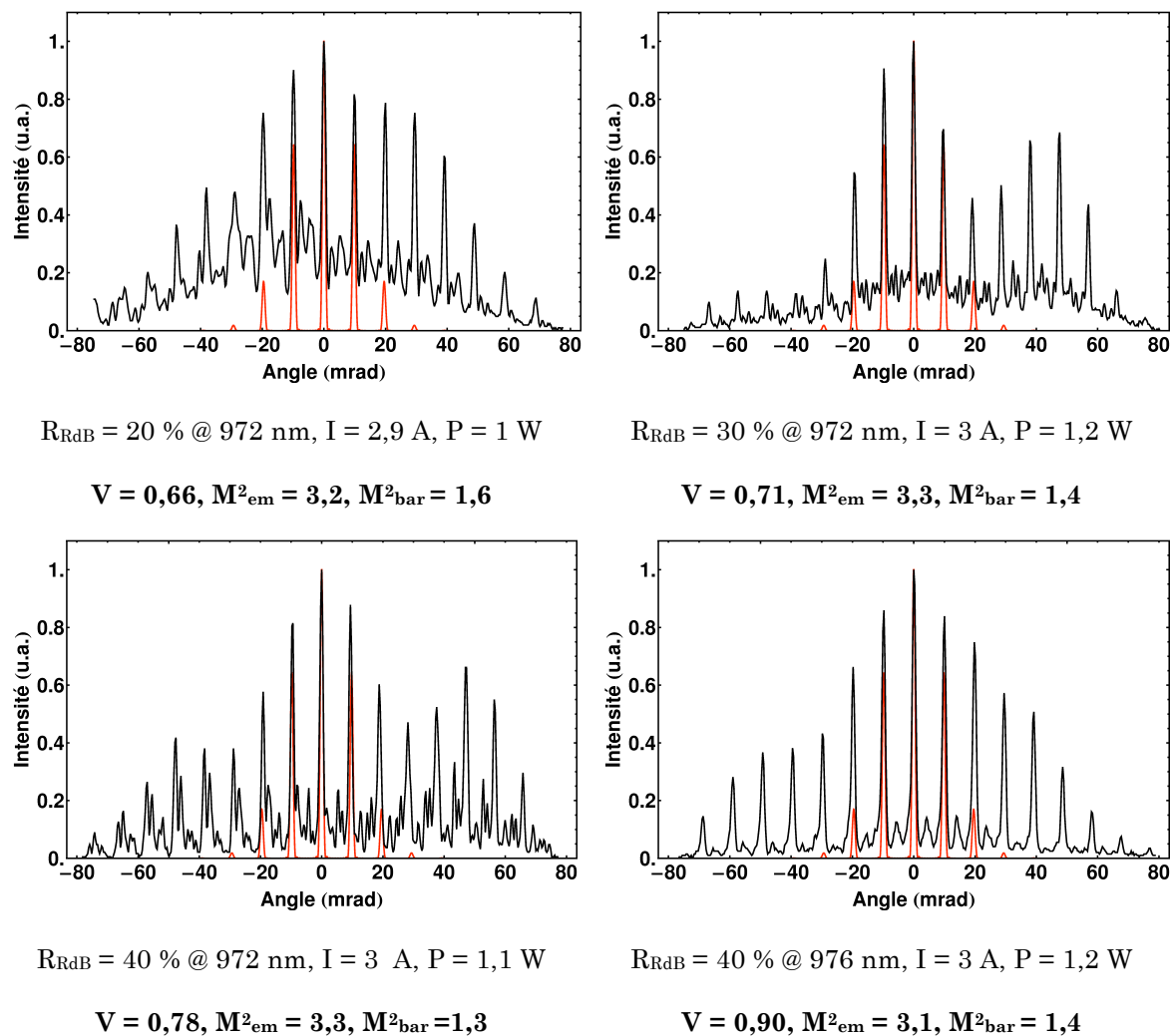
Figure III-16 : Comparaison des profils en champ lointain du mode en phase en fonction du coefficient de réflexion du réseau de Bragg – noir : mesures expérimentales, rouge : champs lointains théoriques – barrette 10IG1-I-5.
