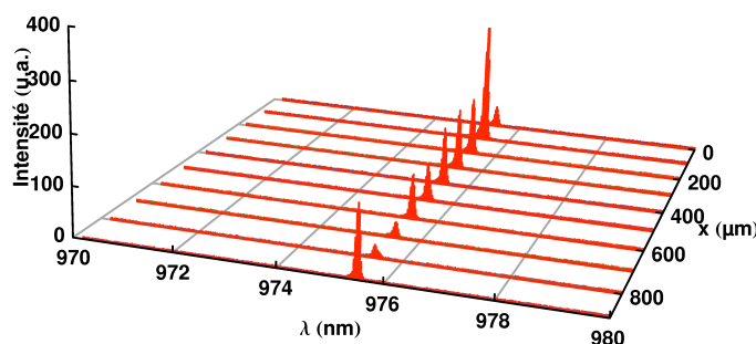
Figure III-13 : Champ proche spectralement résolu avec le réseau de Bragg – R_{dB} = 40 \% @ 976 nm, barrette 10IG1-I-5, I = 4 \text{ A} , P = 1,7 \text{ W} , mode en phase.
