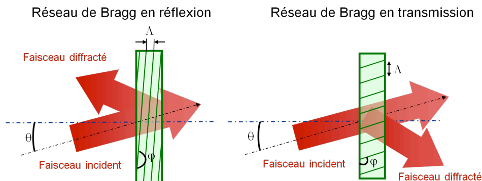
Figure I-12 : Schéma de principe d'un réseau de Bragg en réflexion (gauche) et d'un réseau de Bragg en transmission (droite).
