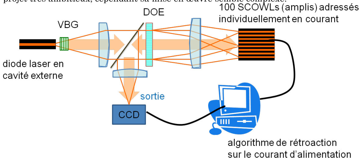
Figure I-39 : Schéma de principe de la configuration de [Huang 09].
