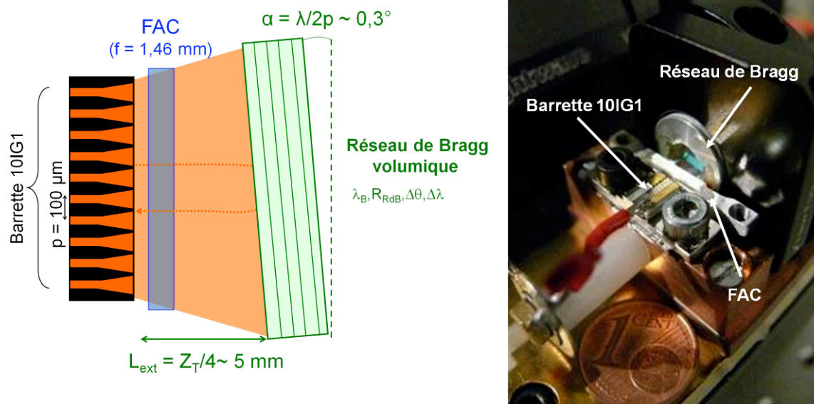
Figure III-10 : gauche – schéma de la cavité Talbot réalisée avec la barrette 10IG1 droite – photographie du prototype, FAC : lentille cylindrique de collimation de la direction verticale.
