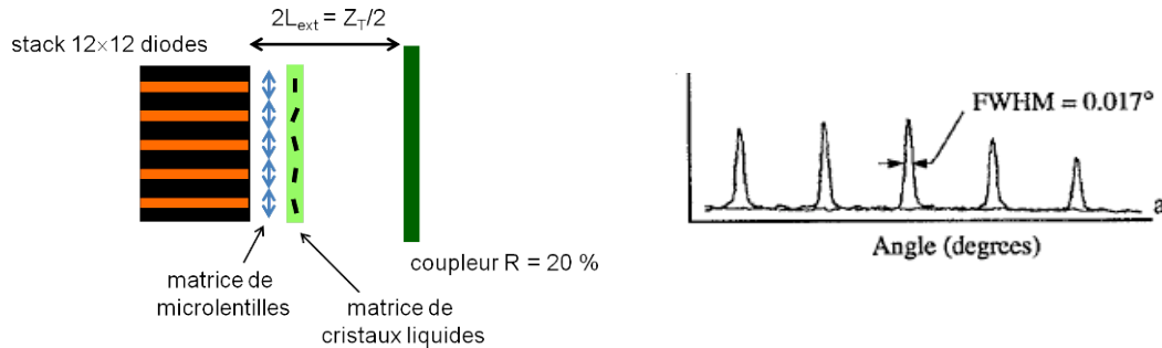
Figure I-38 : Schéma expérimental (gauche) de la cavité réalisée par [Sanders 94] et champ lointain (droite) mesuré pour I = 8 A et P = 1,4 W.
