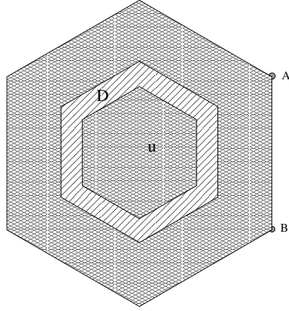
FIGURE 3.4 – Sur les hexagones horizontaux ( z = 0 et z = |a_3|/3 ) on creuse les parties limitées par les deux petits hexagones ( D et D' en hachuré) d'une profondeur égale à \epsilon .
