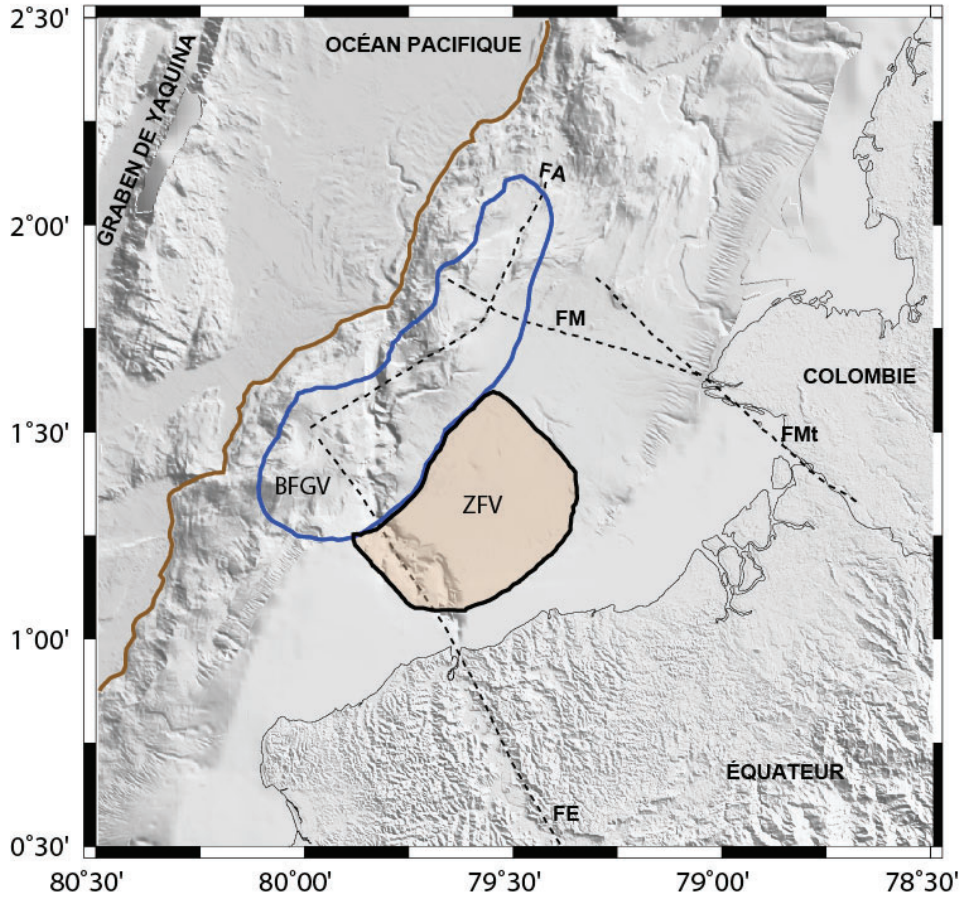
Figure 5.6. Localisation de la zone à faible vitesse sismique (ZFV) en rose. Le contour bleu représente le butoir à faible gradient de vitesse (BFGV). Pour les abréviations voir la légende de la figure 4.13
