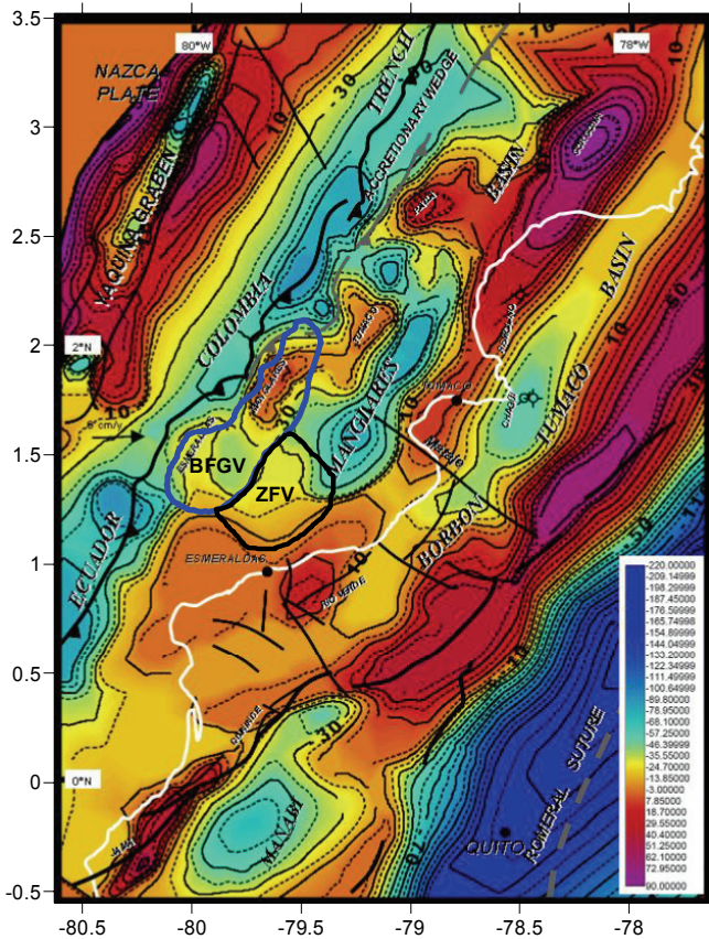
Figure 5.6. Localisation de la zone à faible vitesse sismique (ZFV) en rose. Le contour bleu représente le butoir à faible gradient de vitesse (BFGV). Pour les abréviations voir la légende de la figure 4.13
