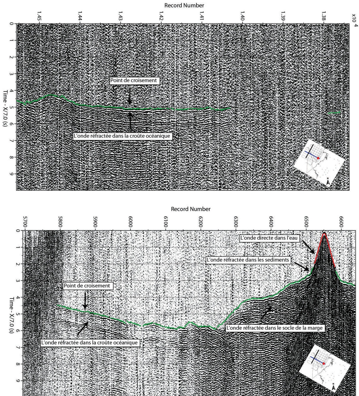
Figure 2.13. Exemple d'un profil en éventail: les données correspondent au profil 28 (ligne épaisse noire dans la carte) enregistré par l'OBS 26 qui voit les tirs en éventail (en haut). L'offset est de 114 km vers le NE et 96 km vers le SW. Notez la bonne qualité de la section sismique malgré la distance entre l'OBS et le profil de tirs. Pour l'identification du type d'ondes enregistrées il faut regarder le point d'intersection avec un profil en ligne (ligne bleue dans la carte, figure en bas) qui correspond à offset de 80 km. Les sections sont représentées en temps réduit à 7 \text{ km s}^{-1} et filtrées avec un filtre Butterworth entre 5 Hz et 15 Hz.
