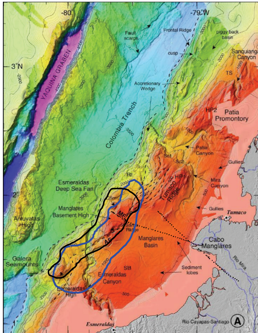
Figure 5.3. Localisation du butoir à faible vitesse (contour bleu) et de l'OBH ( contour noir ) (Collot et al., 2004) sur la carte bathymétrique détaillée (Modifié d'après Collot et al., sous presse). L'OBH défini à partir des données bathymétriques, et de MCS, a une bonne corrélation avec l'extension du butoir à faible gradient de vitesse.
