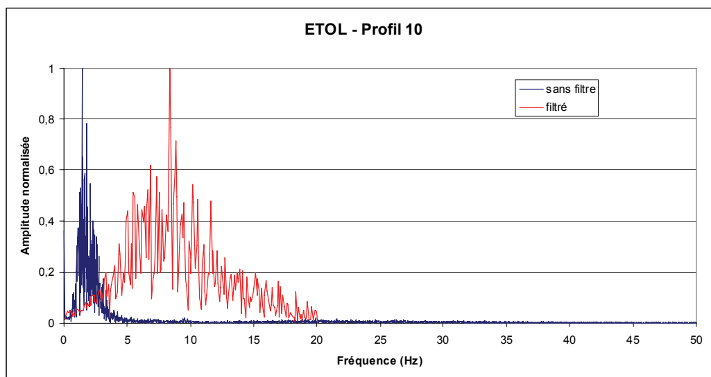
Figure 2.7. Exemple d’un spectre d’amplitude de données du profil 10 enregistrées par la station à terre ETOL, durant la campagne Esmeraldas. En bleu le signal brut, et en rouge sous l’influence du filtre de cohérence entre 4 Hz et 16 Hz.
