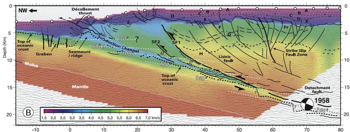
Figure 4.9. Superposition du modèle de vitesse "en bloc" final et l'image migrée mixte du profil MCS SIS44. L'image met en évidence les rapports entre les vitesses sismiques et les structures sismiques. Les cercles blancs indiquent la position des OBS. SF1 et SF2 sont des failles secondaires. Les lettres de A à E marquent les différentes couches sédimentaires du bassin avant-arc, F à H les couches du socle de la marge. D'après Collot et al., 2008.
