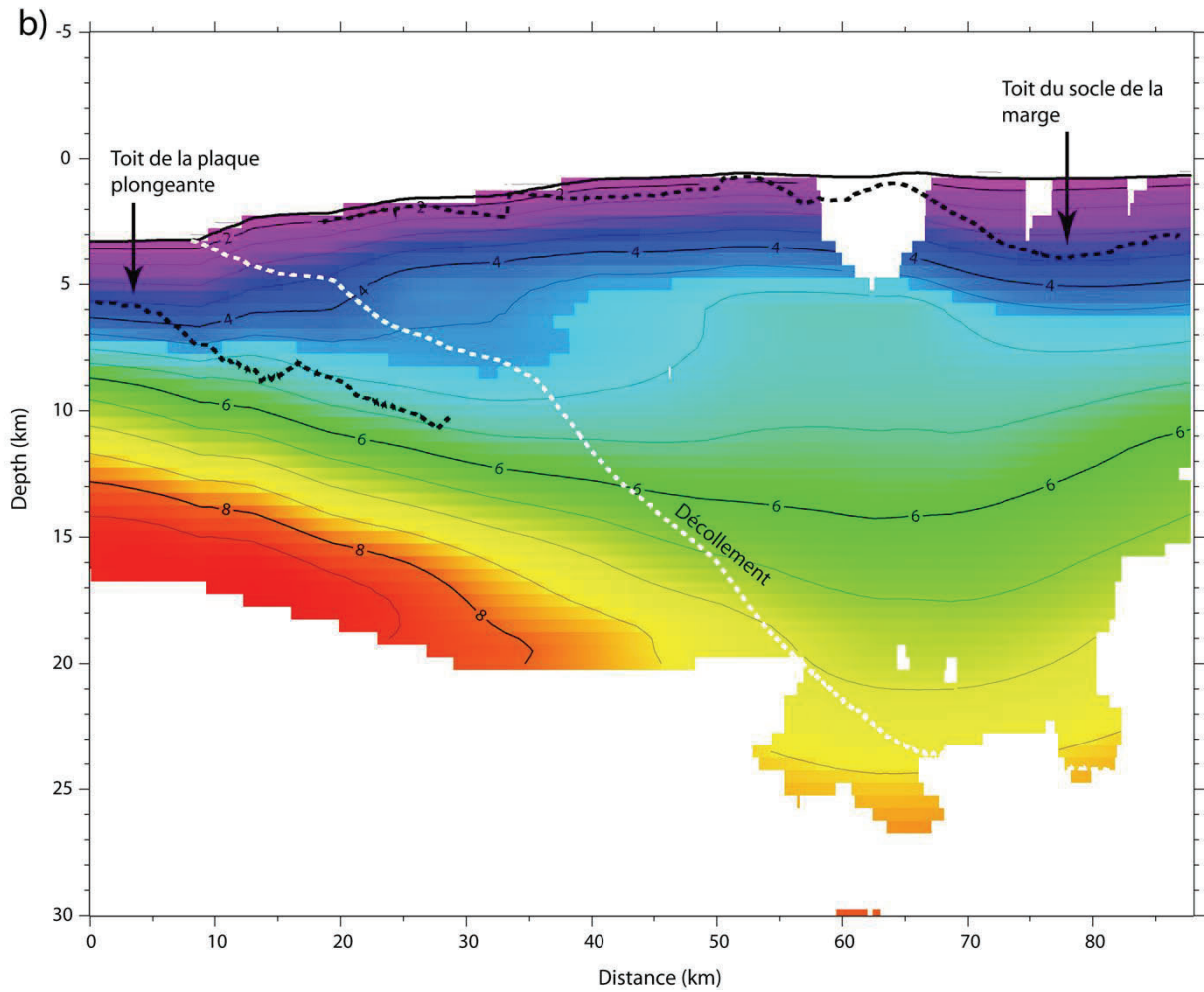
Figure 4.11. Même chose que la figure 4.7 le long du profil SIS47
