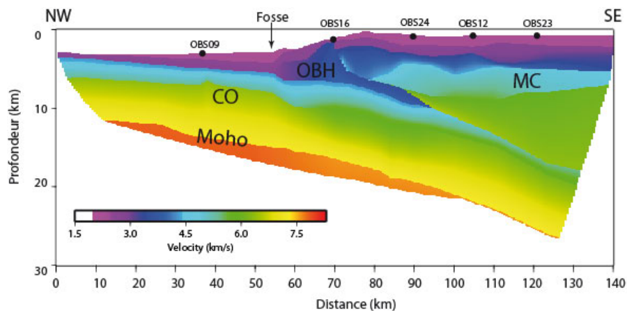
Figure A3.2.3. Modèle de vitesse final du profil 16, obtenu par modélisation directe ( rms = 0.103 \text{ s} ). CO croûte océanique de la plaque plongeante, MC marge de la plaque chevauchante, OBH outer basement high . Les cercles noirs représentent les OBS utilisés pour la modélisation.
