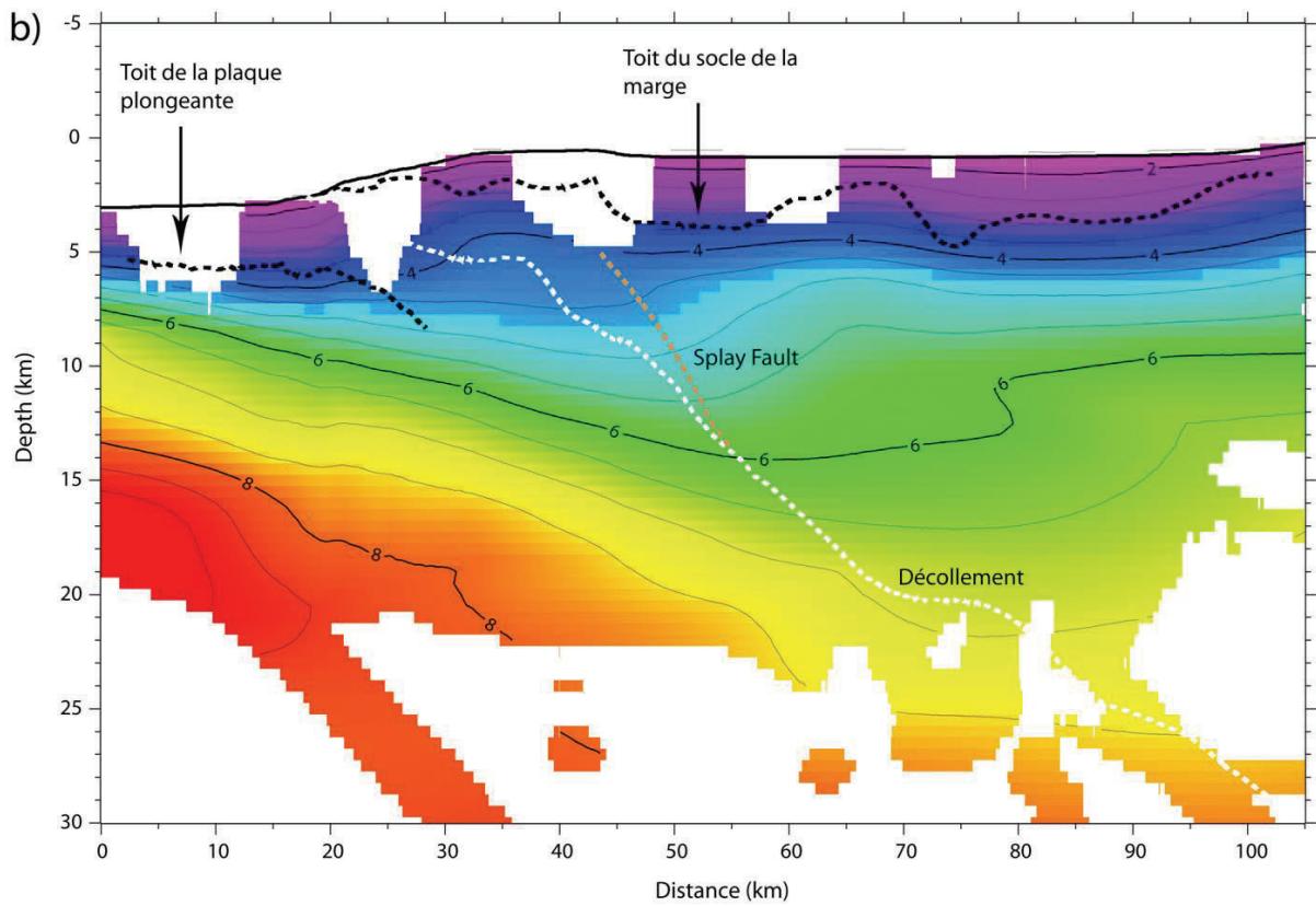
Figure 4.10. Même chose que la figure 4.7 le long du profil SIS45
