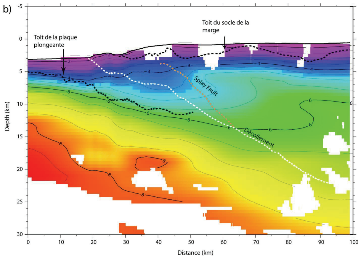
Figure 4.8. Même chose que la figure 4.7 le long du profil SIS44
