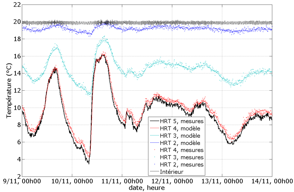
FIG. 4.2 : Température sur le pare- pluie, dans la paroi Est, et à l'intérieur, du 9 au 14 novembre 2008 ; h_{c,int} = 6 \text{ W/m}^2\text{K}
