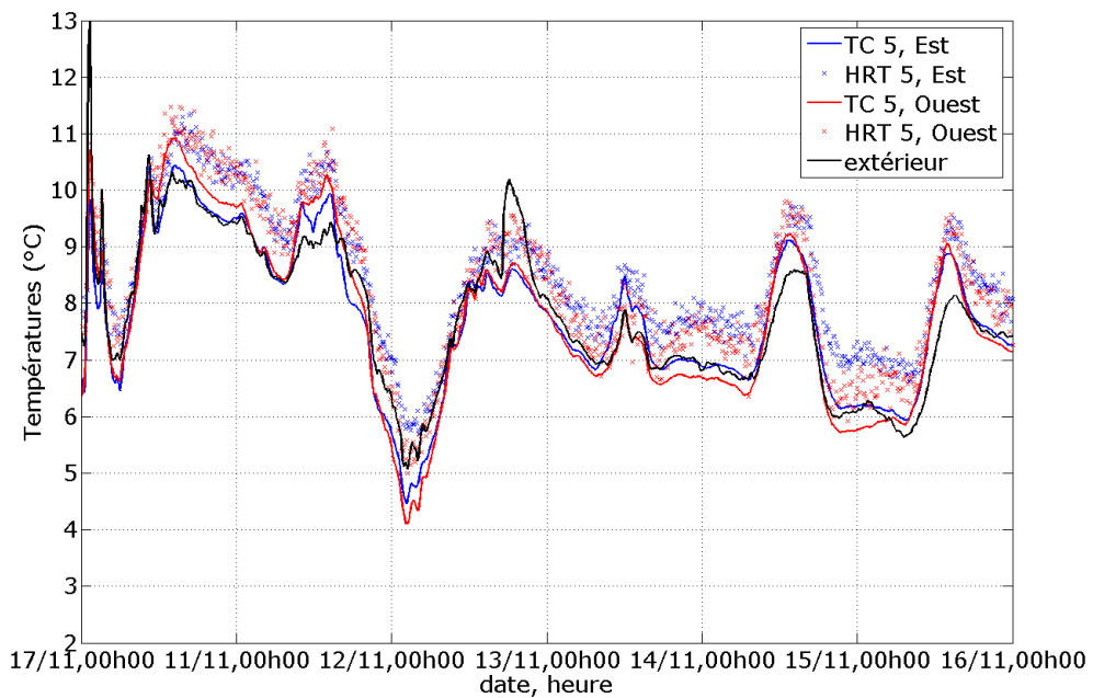
FIG. 2.18 : Températures à l'arrière du bardage (TC 5) et sur le pare-pluie (HRT 5), en parois Est et Ouest, et température extérieure, du 6 novembre au 17 novembre 2008
