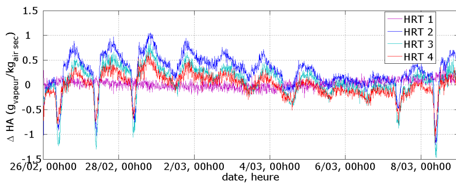
FIG. 4.7 : Écarts entre les résultats de calculs et les mesures d'humidité absolue dans la paroi Est, du 26 février au 9 mars 2009
