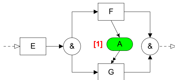
FIGURE 7.3 – Modèle comportant une panne sur le niveau initial d'un flux
