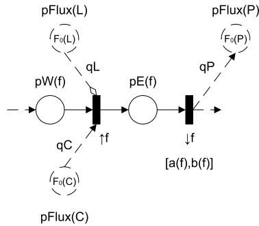
FIGURE 5.8 – Motif d'une fonction à sortie simple f
