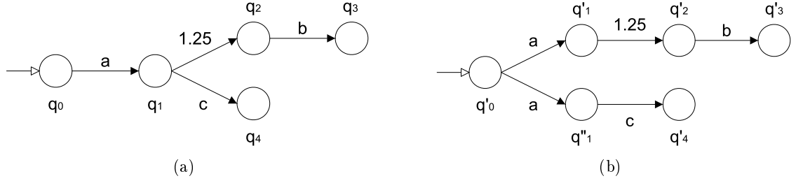
FIGURE 2.2 – Équivalence de langage temporisé
