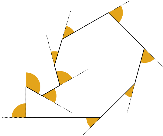
FIG. B.2 – La somme des angles des tangentes d'un polygone du plan est égale à 2\pi
