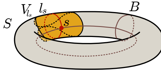
FIG. 3.3 – Voisinage topologique V_{l_s} d'un sommet s appartenant à l'ensemble des points base B sur la surface S .
