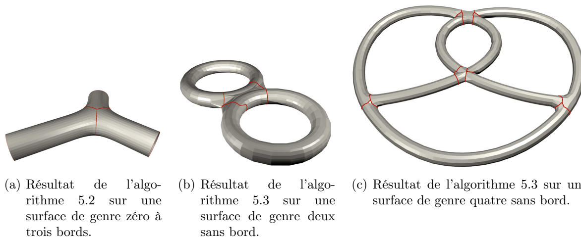
FIG. 5.6 – Pavages en cylindre de surfaces par 3-cets et recuit simulé.
