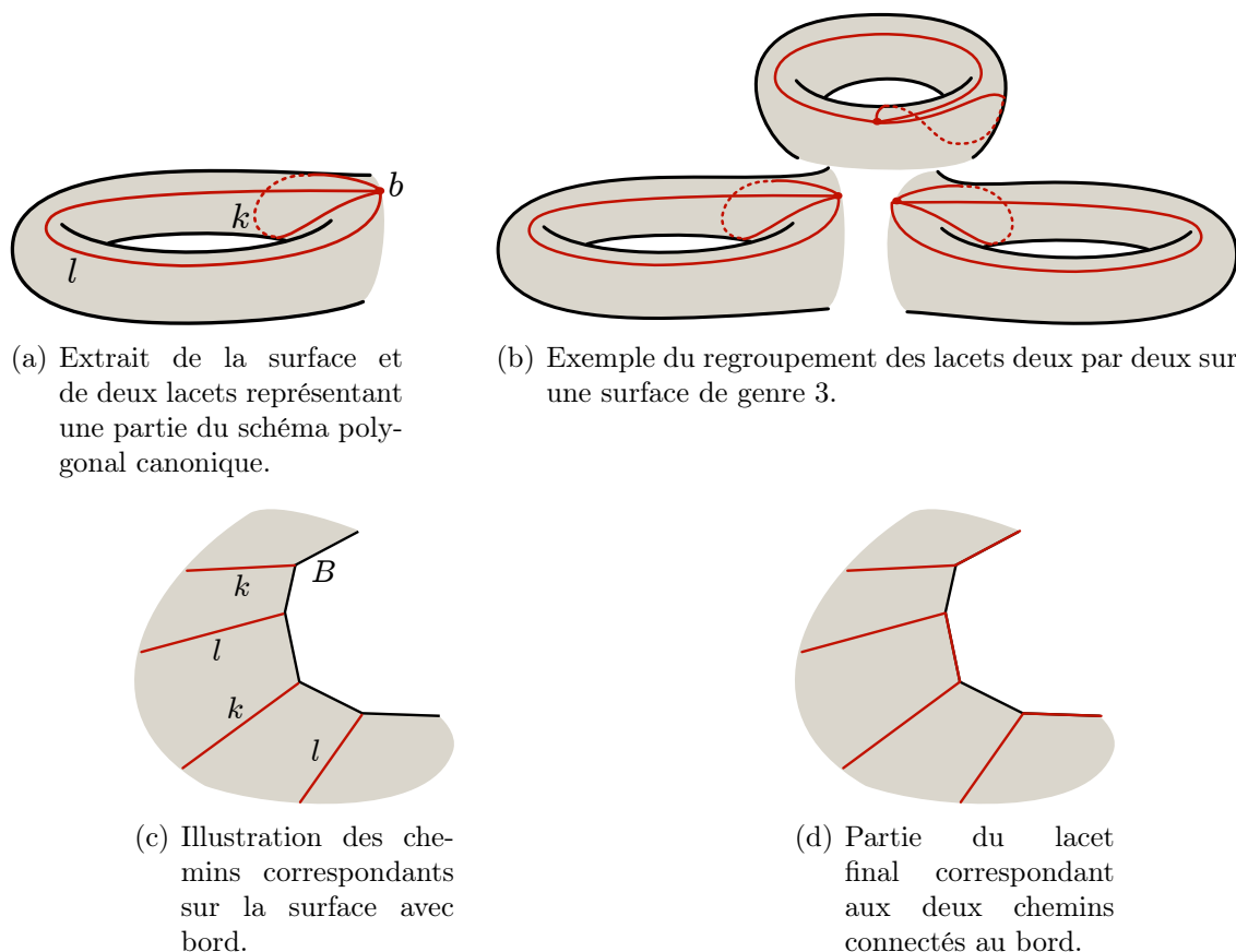
FIG. 3.1 – Illustration de la preuve du lemme 3.1.
